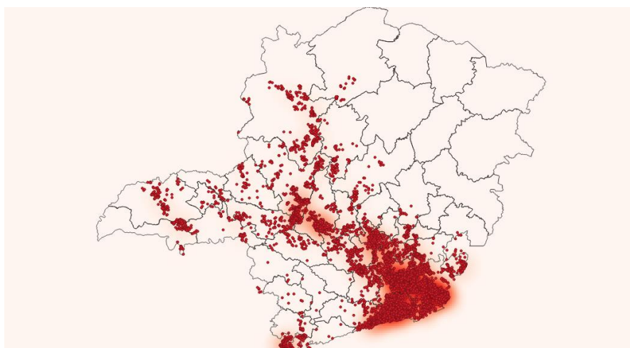
Figura 9 - Raios registrados no dia 02/02/2020. Fonte: RINDAT.
