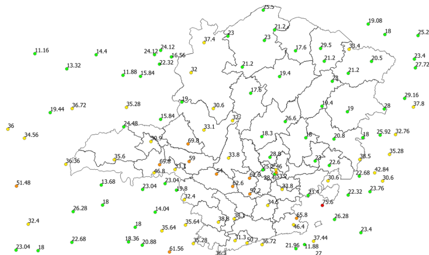
Figura 5 - Rajadas de vento registradas no dia 01/02/2020. Fonte: INMET.
