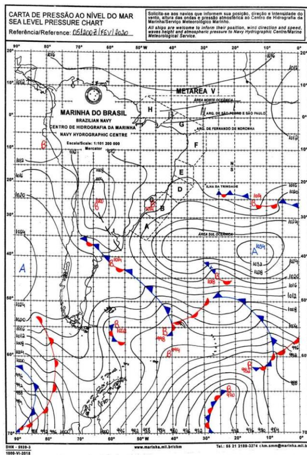
Figura 22 - Carta Sinótica do Dia 05/02/2020. Fonte: Marinha Brasileira.
