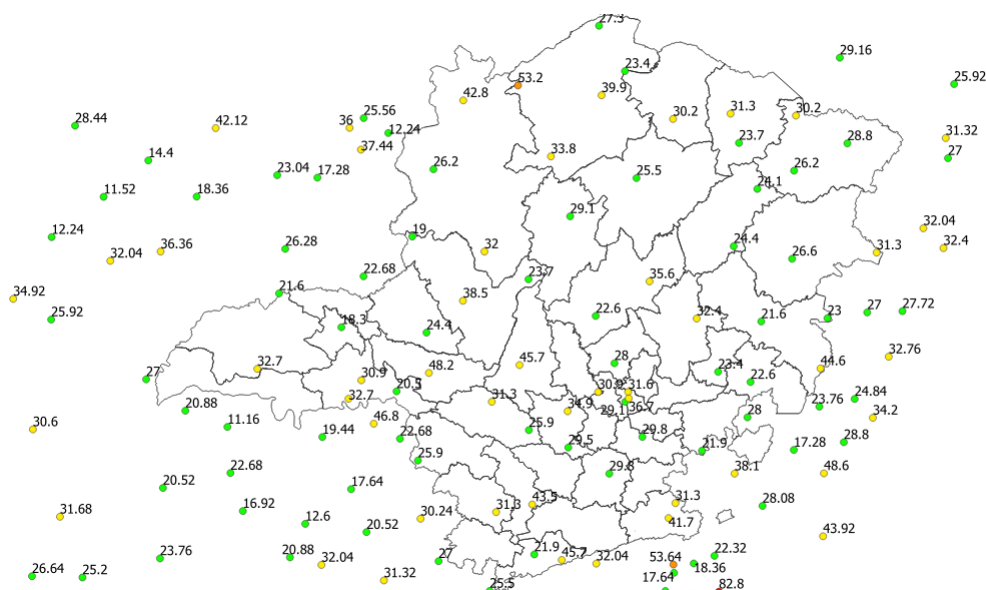
Figura 25 - Rajadas de vento registradas no dia 05/02/2020. Fonte: INMET.
