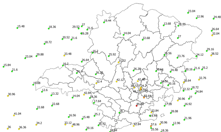
Figura 10 - Rajadas de vento registradas no dia 02/02/2020. Fonte: INMET.
