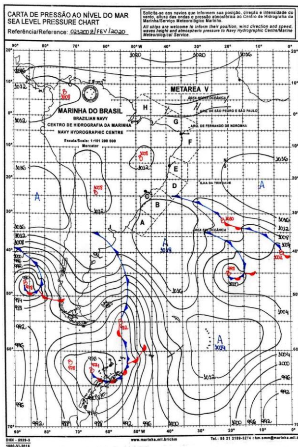
Figura 7 - Carta Sinótica do Dia 02/02/2020. Fonte: Marinha Brasileira.
