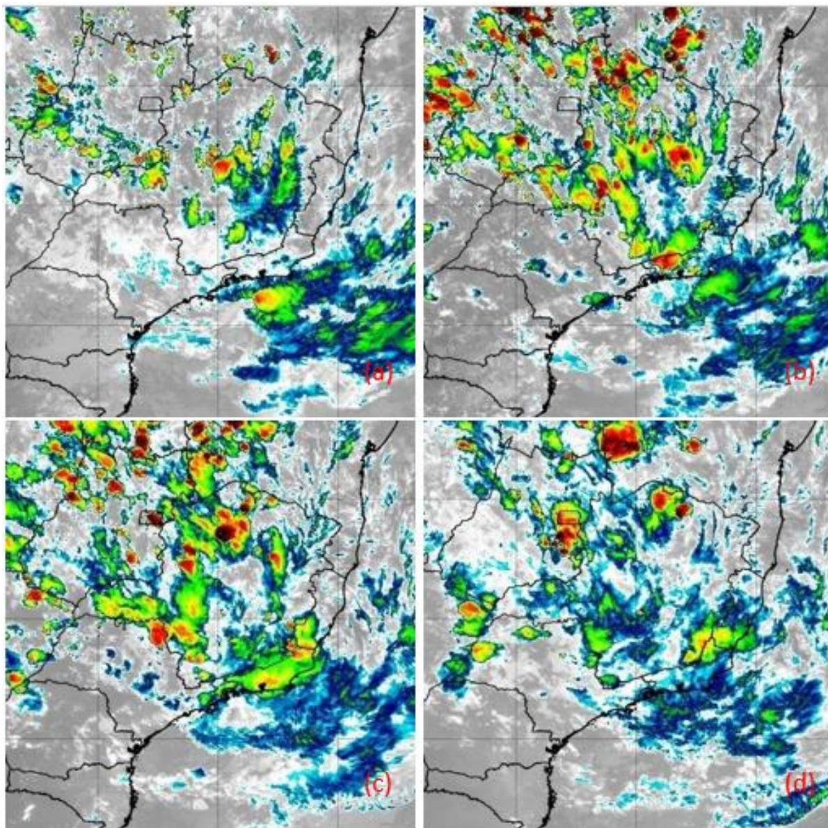
Figura 23 - Imagens do satélite GOES-16 do dia 05/02/2020 as 12:00 (a), 15:00 (b), 18:00 (c) e 21:00 horas local. Fonte: INPE.
