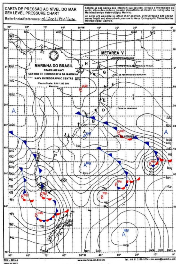
Figura 2 - Carta Sinótica do Dia 01/02/2020. Fonte: Marinha Brasileira.
