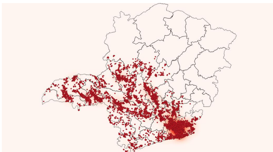
Figura 4 - Raios registrados no dia 01/02/2020. Fonte: RINDAT.
