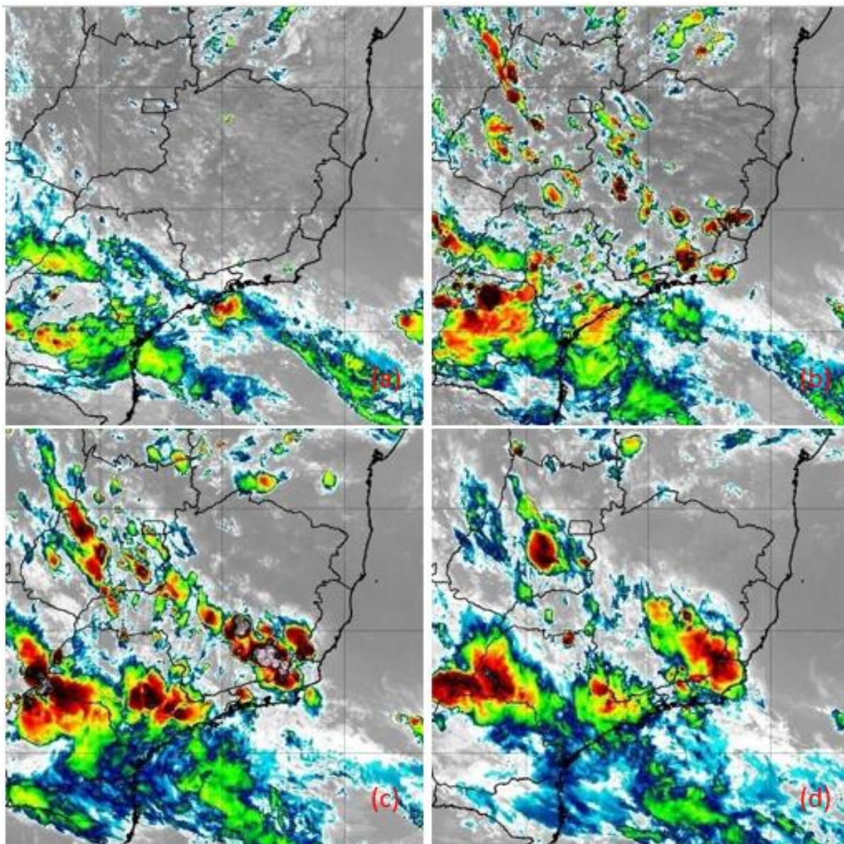
Figura 8 - Imagens do satélite GOES-16 do dia 02/02/2020 as 12:00 (a), 15:00 (b), 18:00 (c) e 21:00 horas local. Fonte: INPE.
