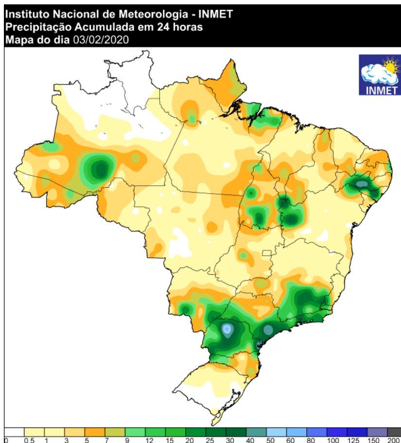
Figura 11 - Precipitação ocorrida no dia 02/02/2020. Fonte: INMET.
