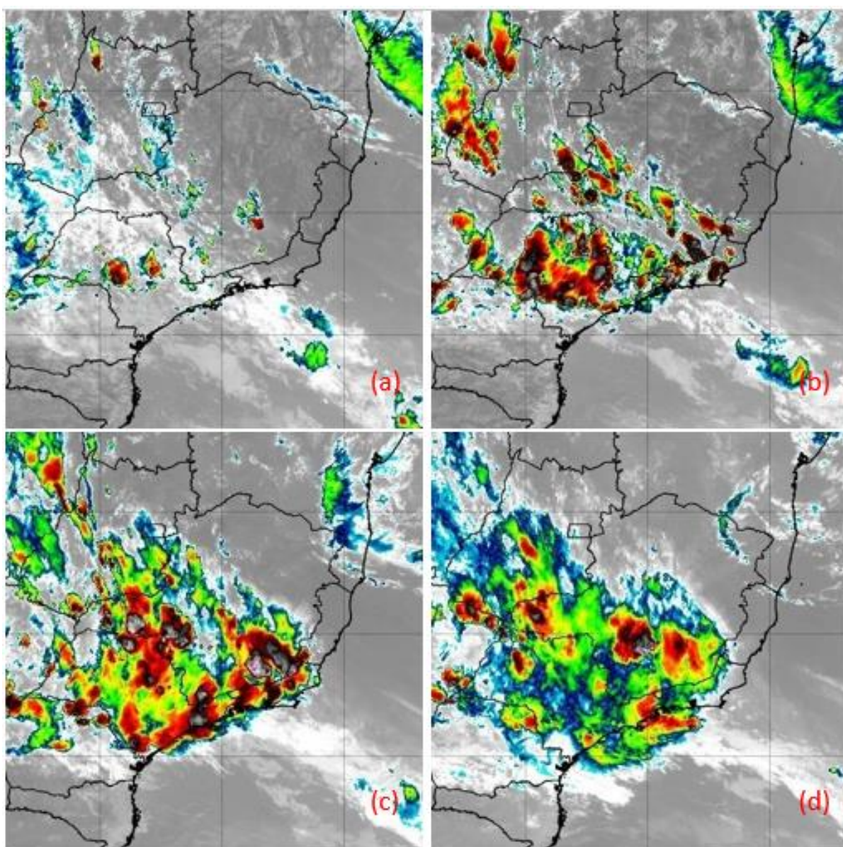
Figura 3 - Imagens do satélite GOES-16 do dia 01/02/2020 as 12:00 (a), 15:00 (b), 18:00 (c) e 21:00 horas local. Fonte: INPE.
