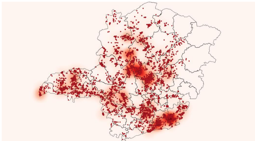
Figura 24 - Raios registrados no dia 05/02/2020. Fonte: RINDAT.
