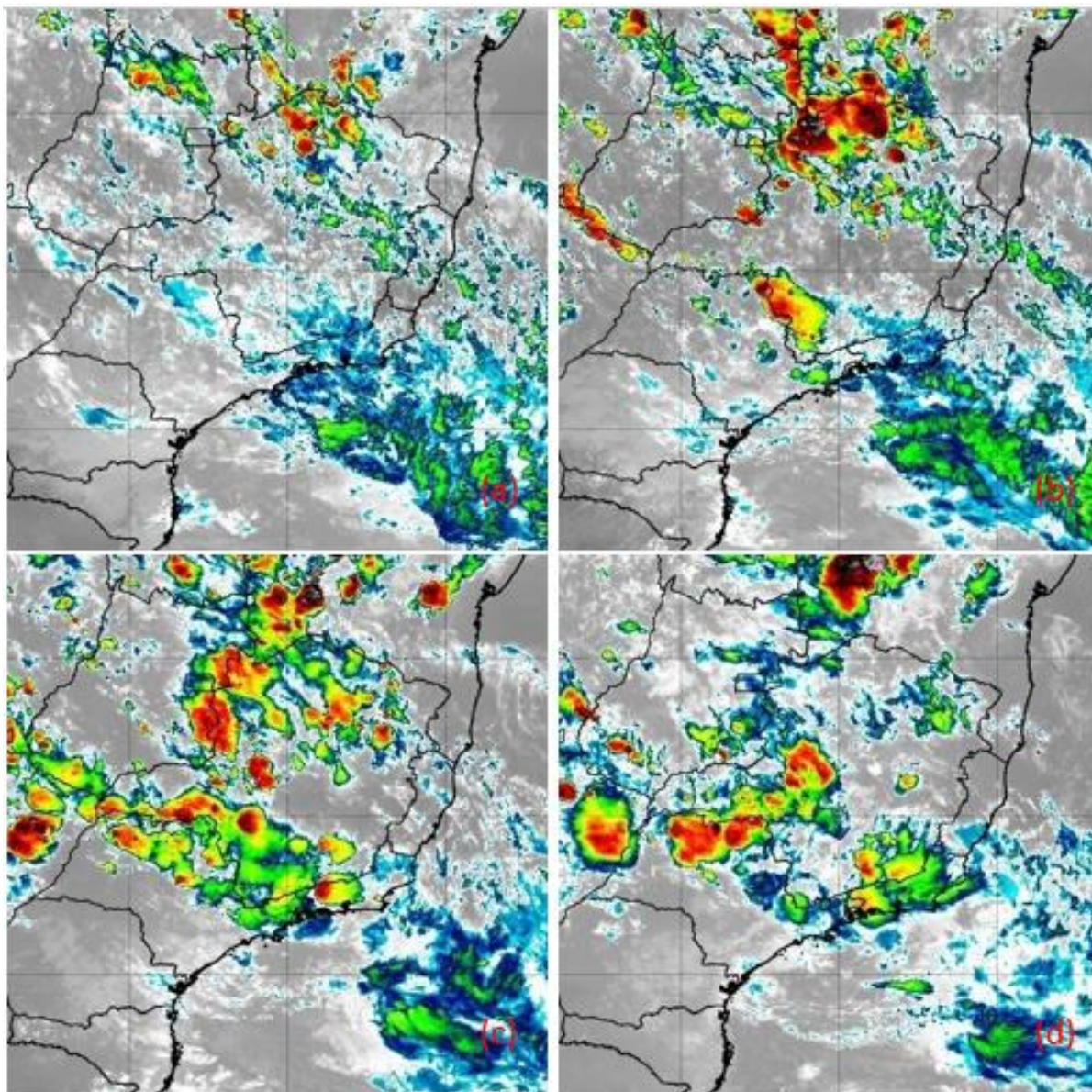
Figura 18 - Imagens do satélite GOES-16 do dia 04/02/2020 as 12:00 (a), 15:00 (b), 18:00 (c) e 21:00 horas local. Fonte: INPE.
