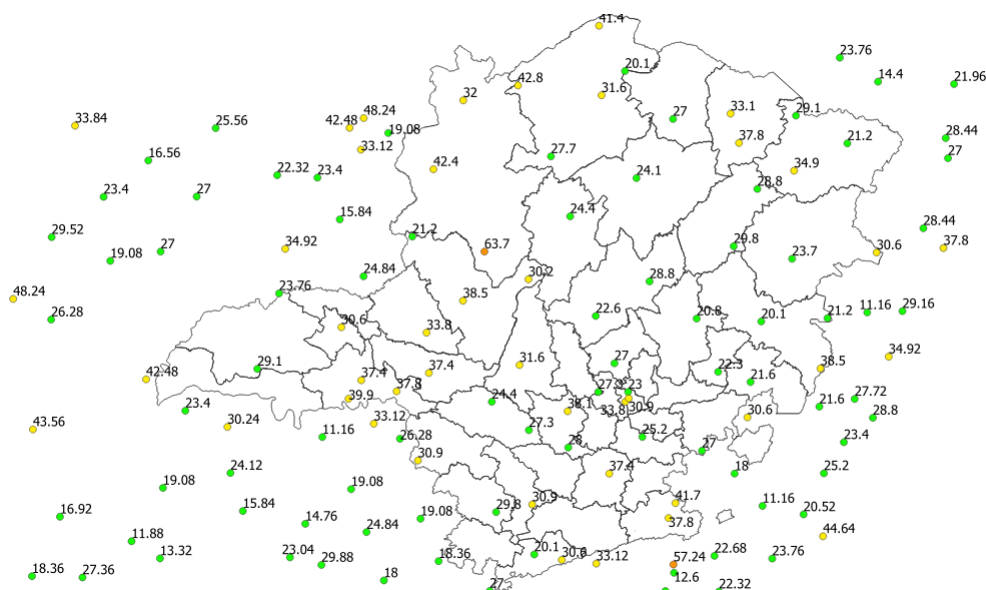
Figura 20 - Rajadas de vento registradas no dia 04/02/2020. Fonte: INMET.
