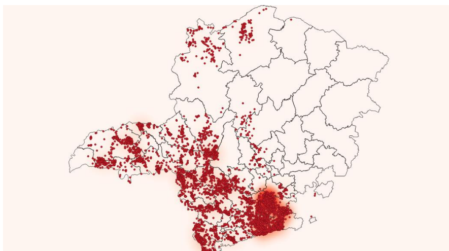
Figura 14 - Raios registrados no dia 03/02/2020. Fonte: RINDAT.
