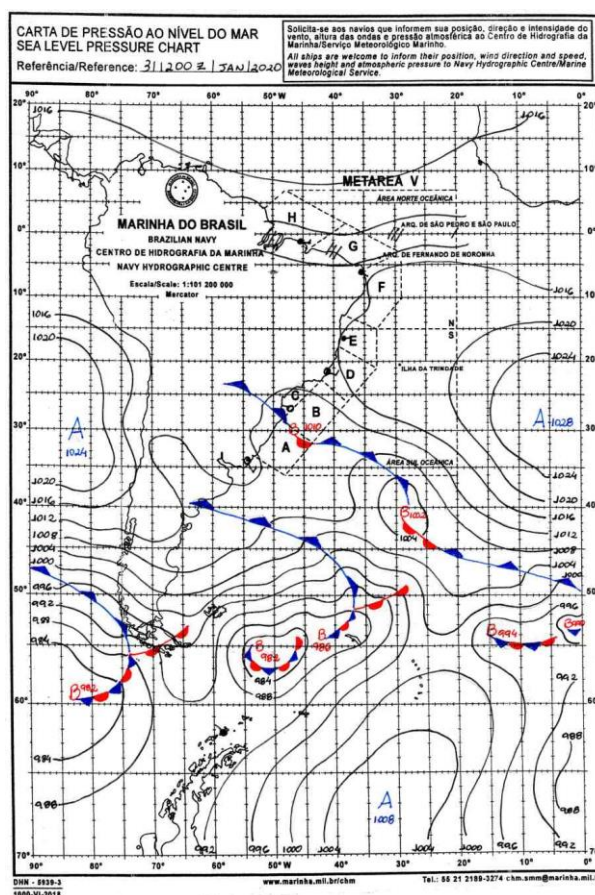
Figura 1 - Carta Sinótica do Dia 31/01/2020. Fonte: Marinha Brasileira.
