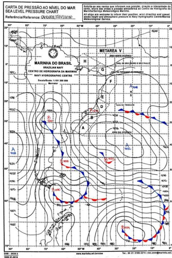
Figura 17 - Carta Sinótica do Dia 04/02/2020. Fonte: Marinha Brasileira.
