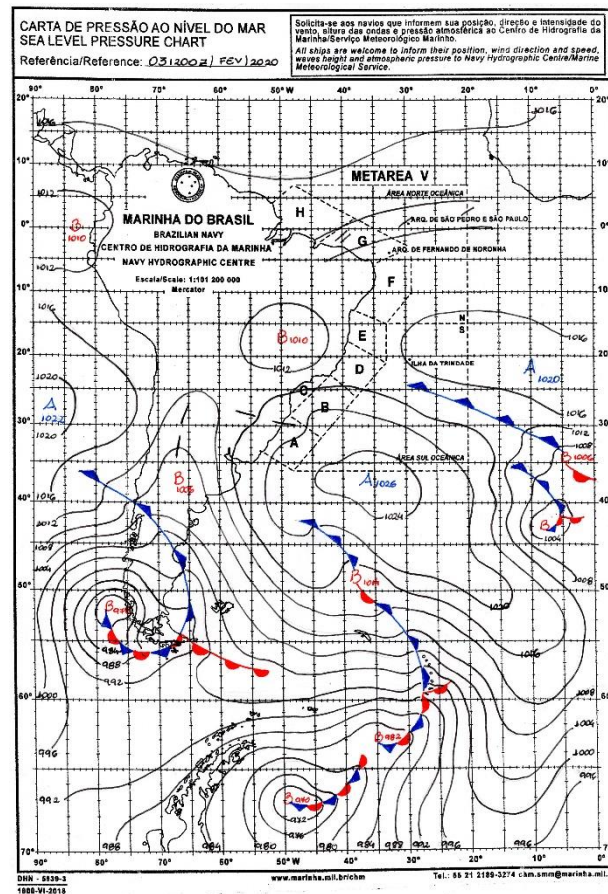
Figura 12 - Carta Sinótica do Dia 03/02/2020. Fonte: Marinha Brasileira.
