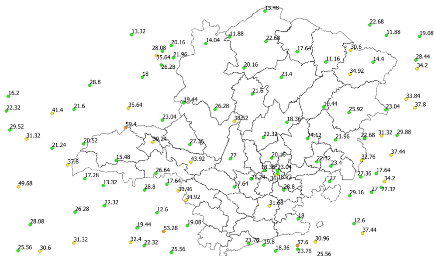
Figura 15 - Rajadas de vento registradas no dia 03/02/2020. Fonte: INMET.
