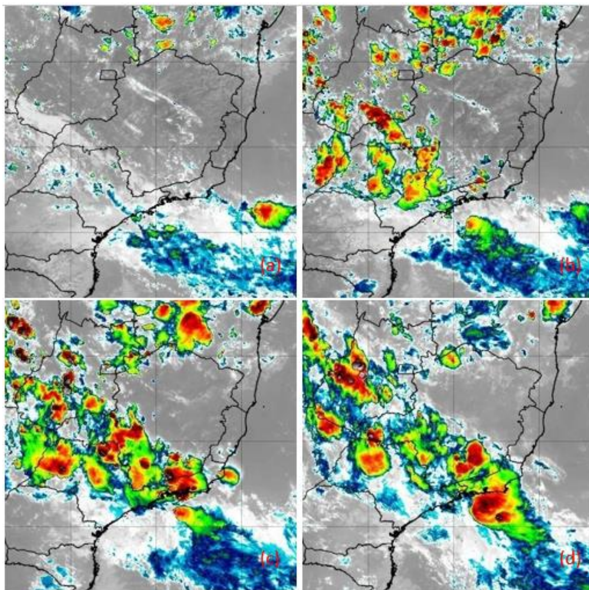
Figura 13 - Imagens do satélite GOES-16 do dia 03/02/2020 as 12:00 (a), 15:00 (b), 18:00 (c) e 21:00 horas local. Fonte: INPE.
