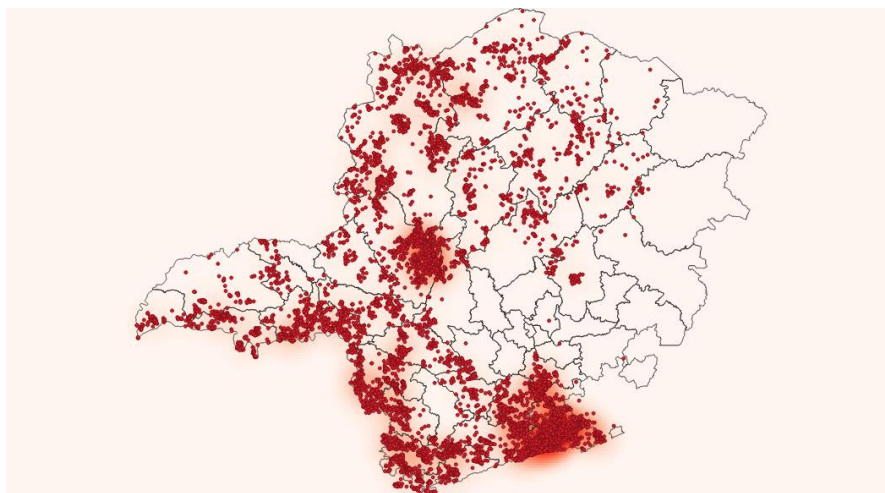
Figura 19 - Raios registrados no dia 04/02/2020. Fonte: RINDAT.
