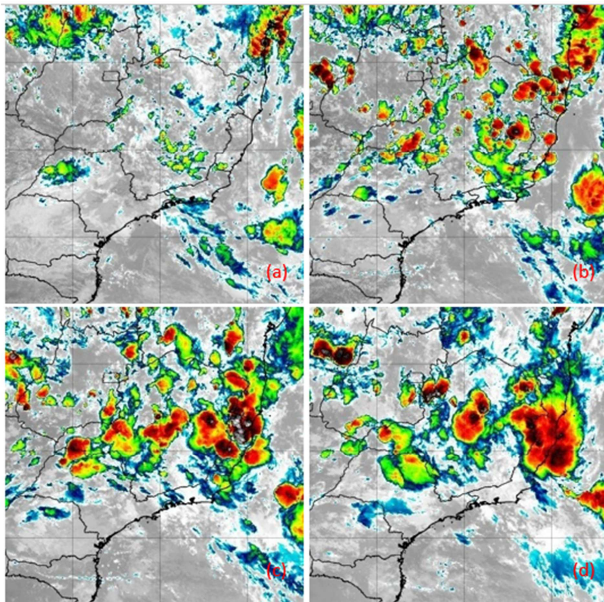
Figura 8 - Imagens do satélite GOES-16 do dia 03/01/2020 as 12:00 (a), 15:00 (b), 18:00 (c) e 21:00 horas local. Fonte: INPE.
