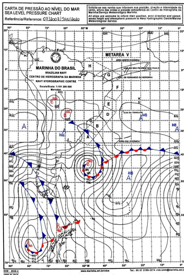
Figura 27 - Carta Sinótica do Dia 07/01/2020. Fonte: Marinha Brasileira.
