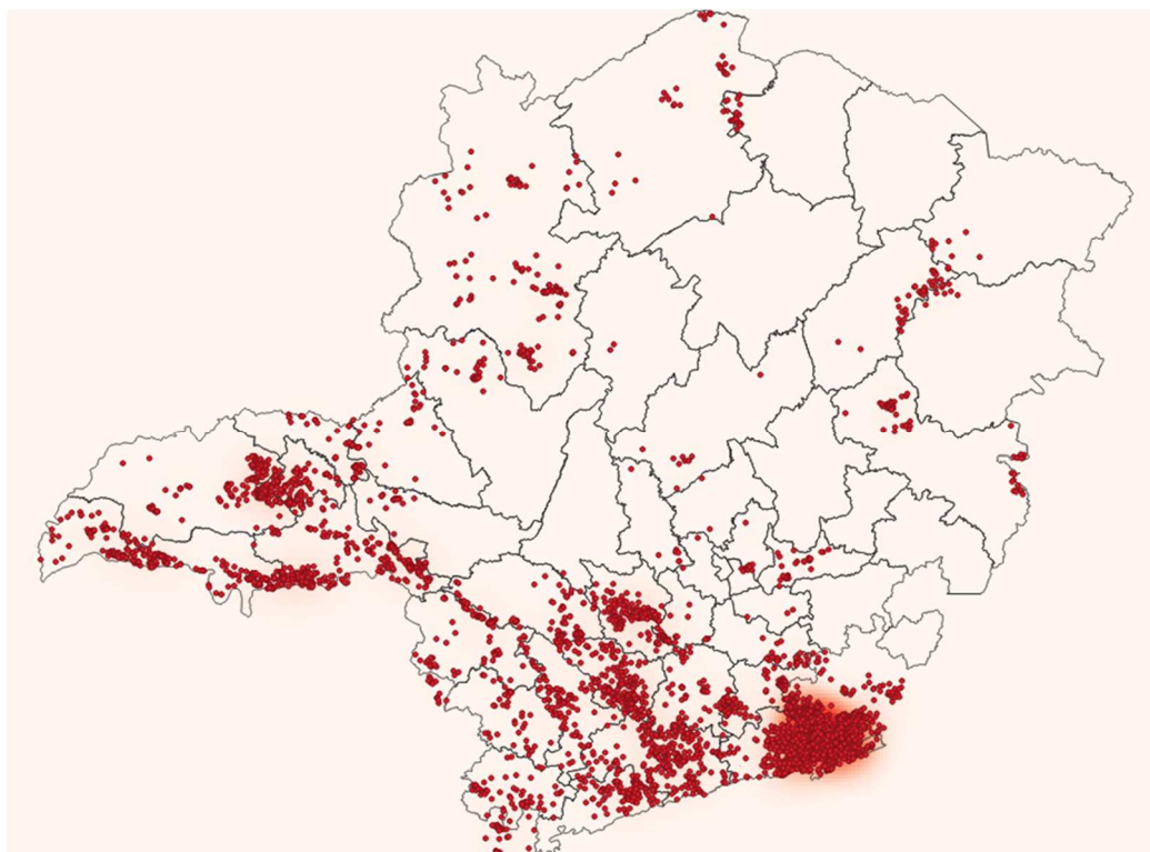
Figura 69 - Raios registrados no dia 05/01/2020. Fonte: RINDAT.
