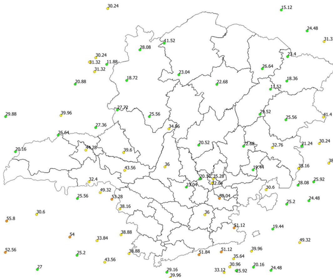
Figura 30 - Rajadas de vento registradas no dia 07/01/2020. Fonte: INMET.
