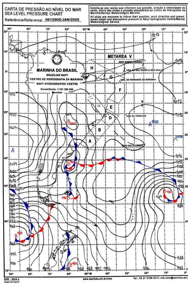
Figura 22 - Carta Sinótica do Dia 06/01/2020. Fonte: Marinha Brasileira.
