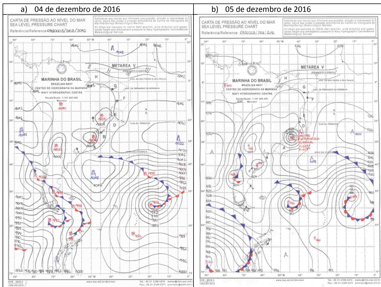
Figura 1 - Cartas Sinóticas elaboradas pelo Centro de Previsão de Tempo e Estudos Climáticos - CPTEC para os dias 04 a 08 de dezembro de 2016.
