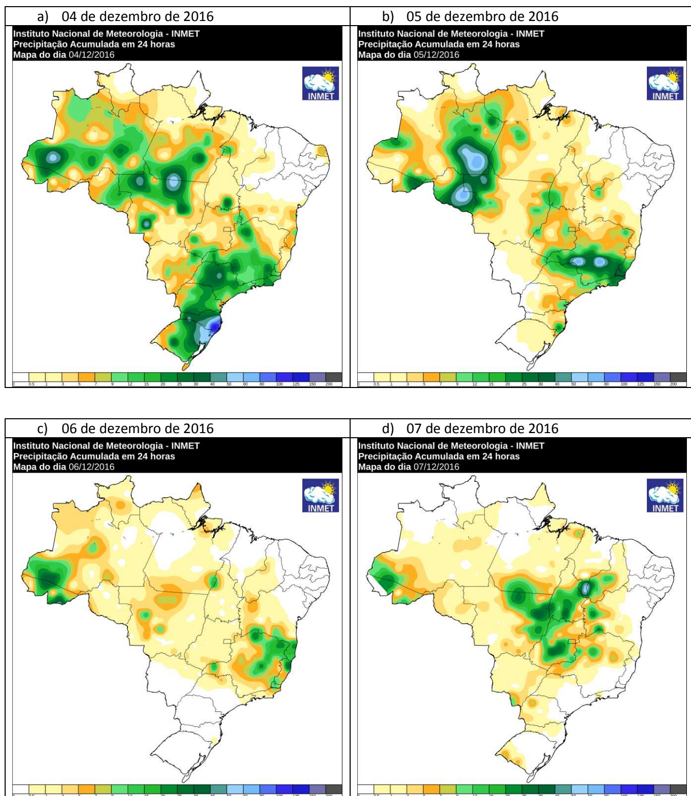
Figura 2 – Acumulado de precipitação (mm) nos dias 04 a 08 de dezembro de 2016.
