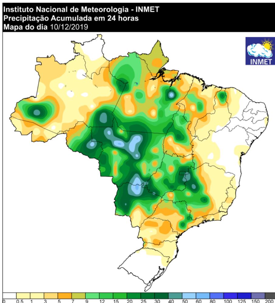
Figura 21 - Precipitação ocorrida no dia 09/12/2019. Fonte: INMET.
