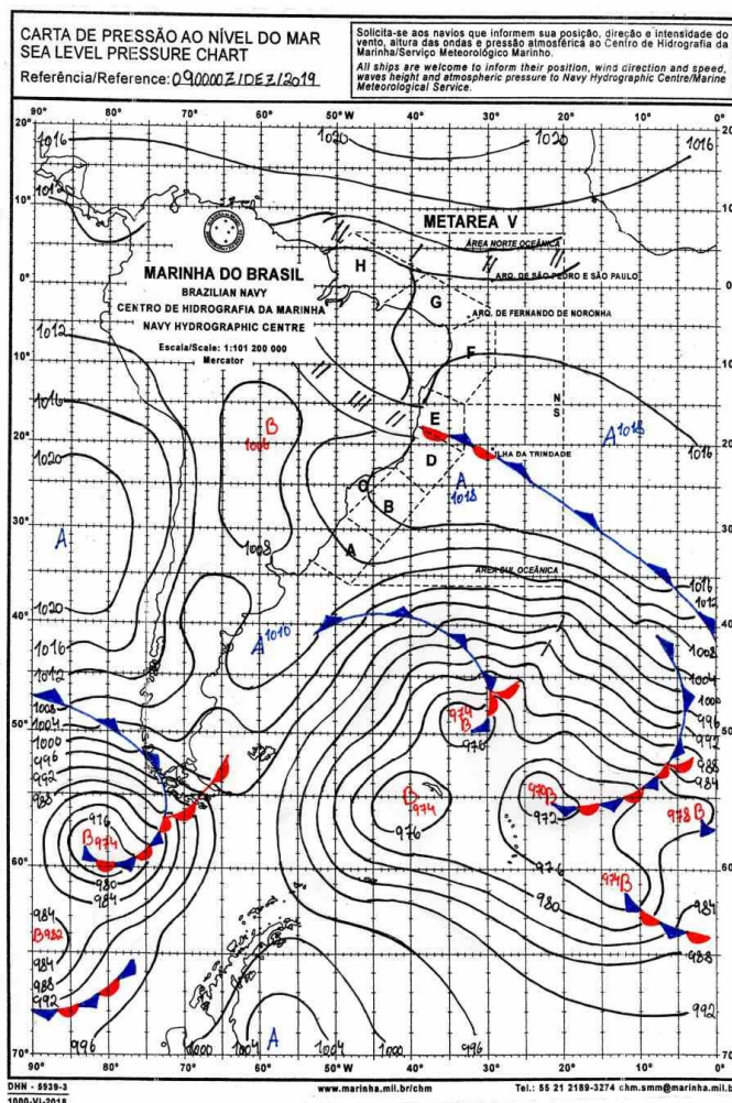
Figura 17 - Carta Sinótica do Dia 09/12/2019. Fonte: Marinha Brasileira.
