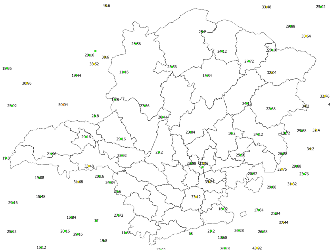
Figura 25 - Rajadas de vento registradas no dia 10/12/2019. Fonte: INMET.
