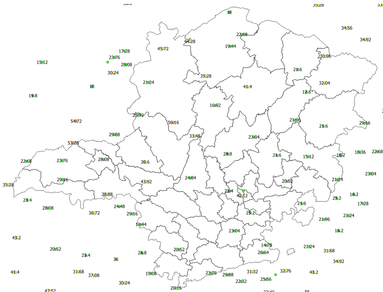
Figura 20 - Rajadas de vento registradas no dia 09/12/2019. Fonte: INMET.
