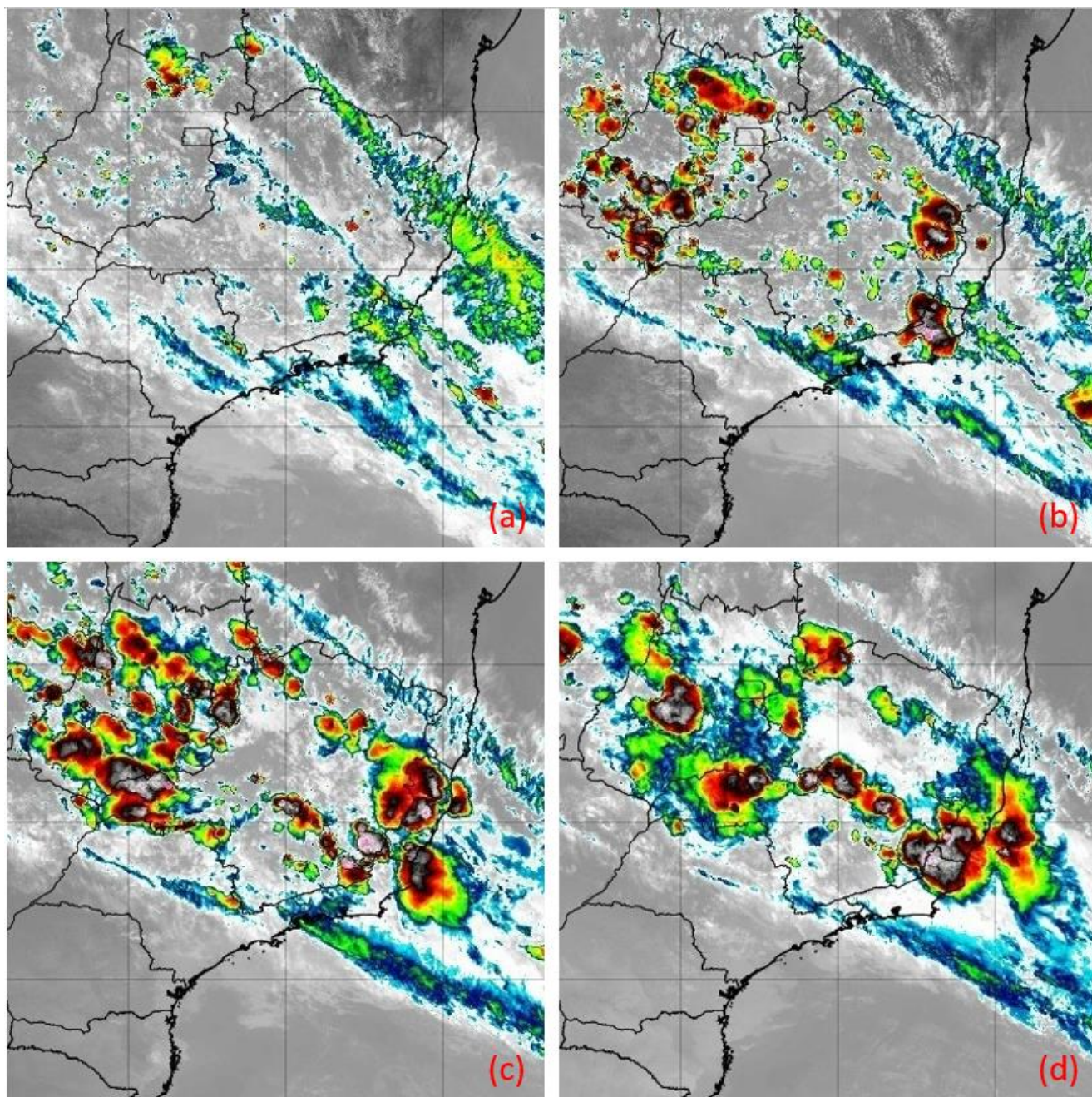
Figura 3 - Imagens do satélite GOES-16 do dia 06/12/2019 as 12:00 (a), 15:00 (b), 18:00 (c) e 21:00 horas local. Fonte: INPE.
