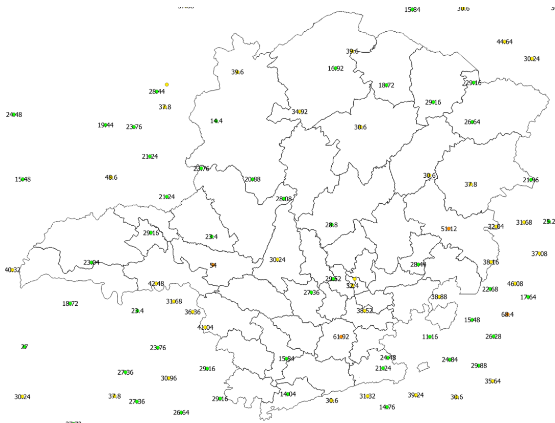
Figura 5 - Rajadas de vento registradas no dia 06/12/2019. Fonte: INMET.
