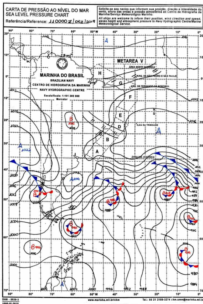
Figura 277 - Carta Sinótica do Dia 11/12/2019. Fonte: Marinha Brasileira.
