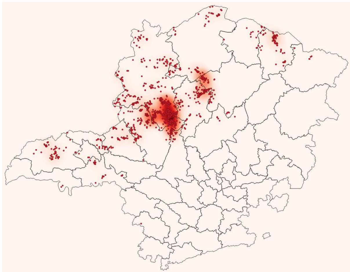
Figura 14 - Raios registrados no dia 08/12/2019. Fonte: RINDAT.
