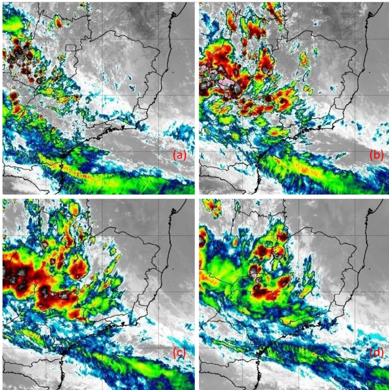
Figura 18 - Imagens do satélite GOES-16 do dia 09/12/2019 as 12:00 (a), 15:00 (b), 18:00 (c) e 21:00 horas local. Fonte: INPE.
