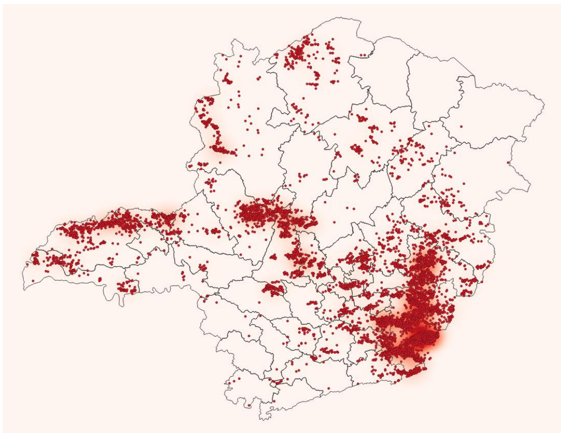
Figura 4 - Raios registrados no dia 06/12/2019. Fonte: RINDAT.
