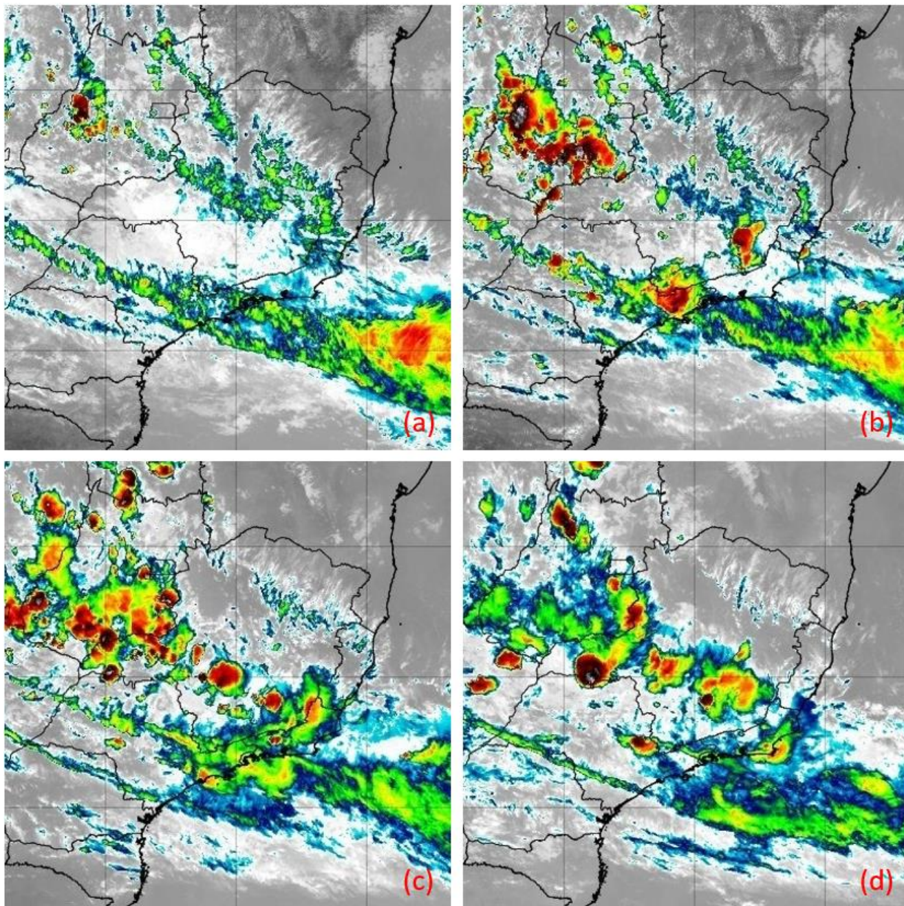
Figura 23 - Imagens do satélite GOES-16 do dia 10/12/2019 as 12:00 (a), 15:00 (b), 18:00 (c) e 21:00 horas local. Fonte: INPE.
