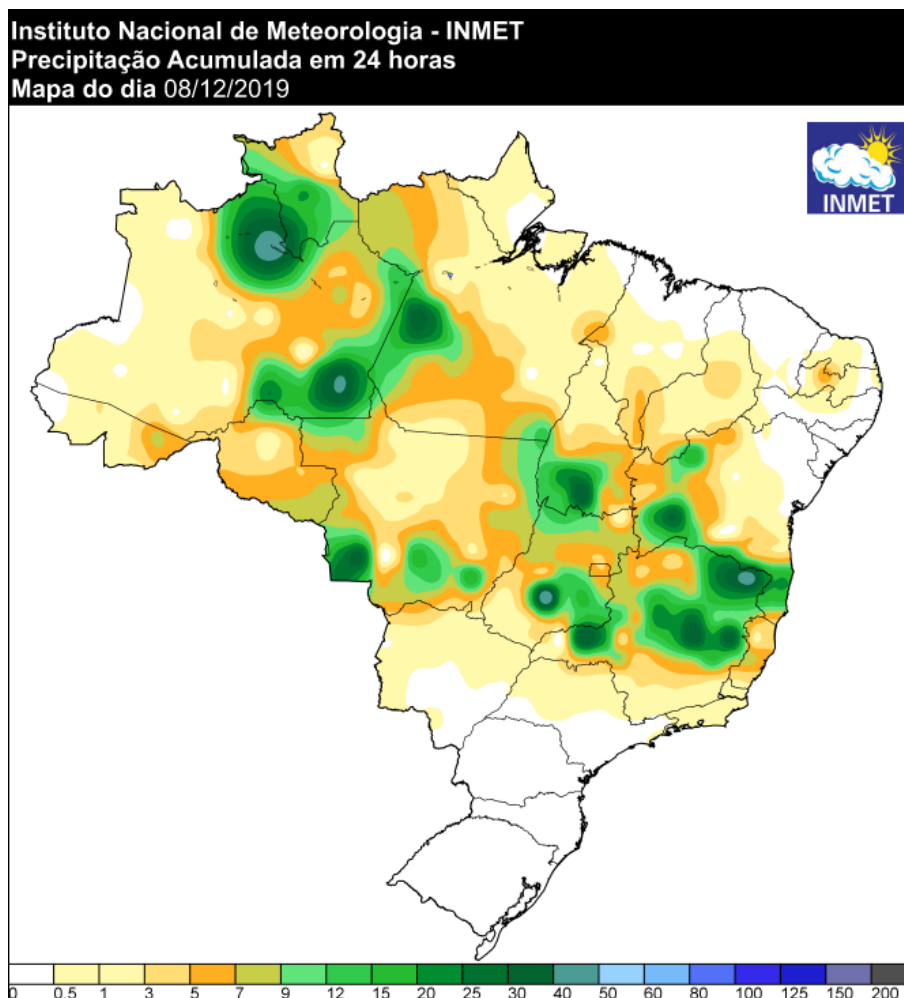
Figura 11 - Precipitação ocorrida no dia 07/12/2019. Fonte: INMET.
