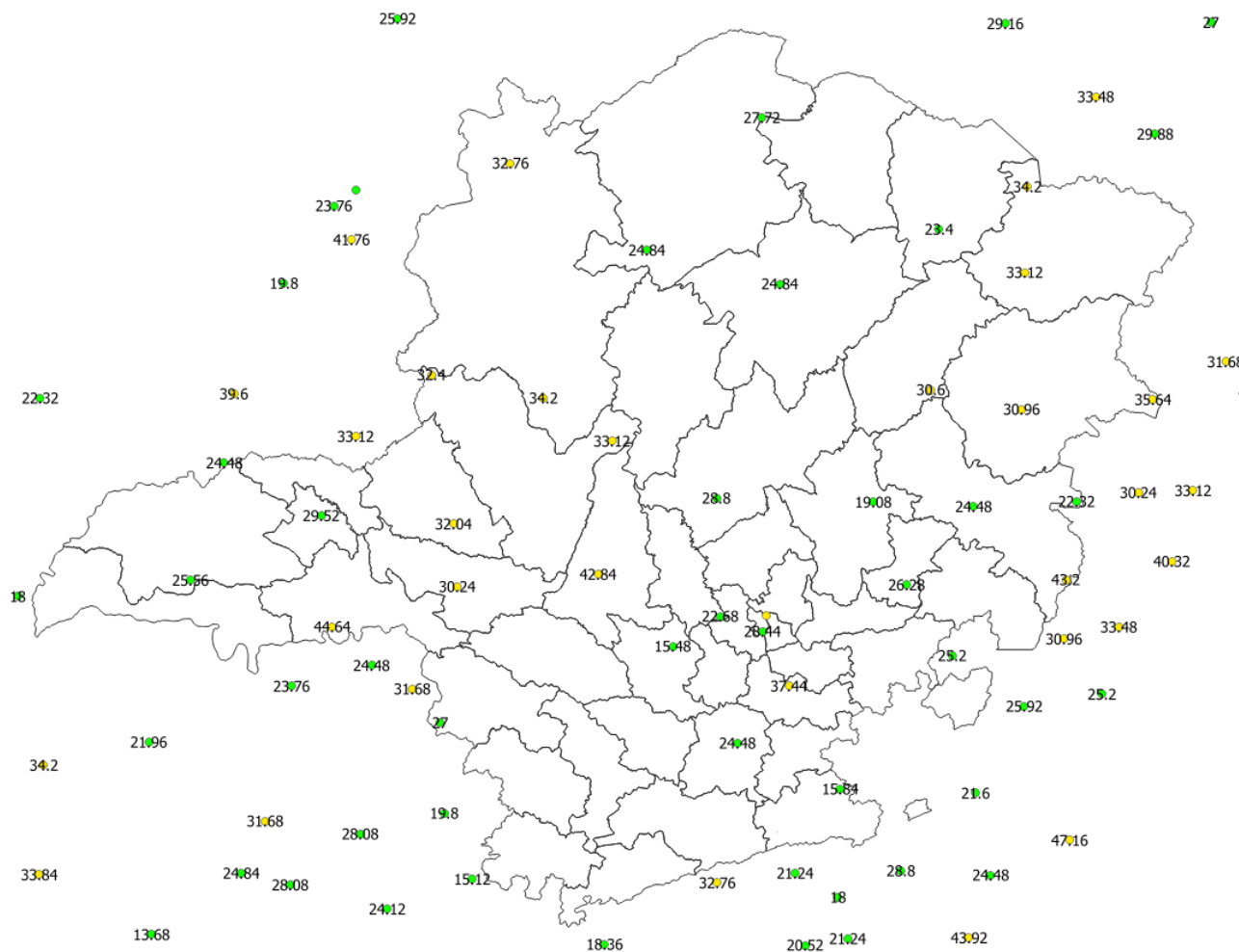
Figura 30 - Rajadas de vento registradas no dia 11/12/2019. Fonte: INMET.
