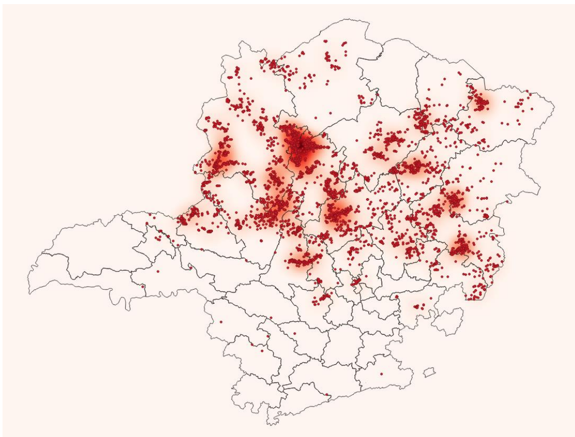
Figura 9 - Raios registrados no dia 07/12/2019. Fonte: RINDAT.
