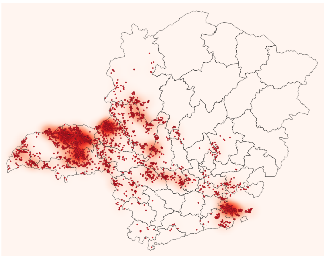
Figura 299 - Raios registrados no dia 11/12/2019. Fonte: RINDAT.
