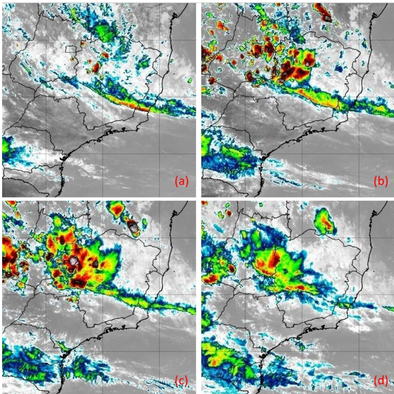
Figura 13 - Imagens do satélite GOES-16 do dia 08/12/2019 as 12:00 (a), 15:00 (b), 18:00 (c) e 21:00 horas local. Fonte: INPE.
