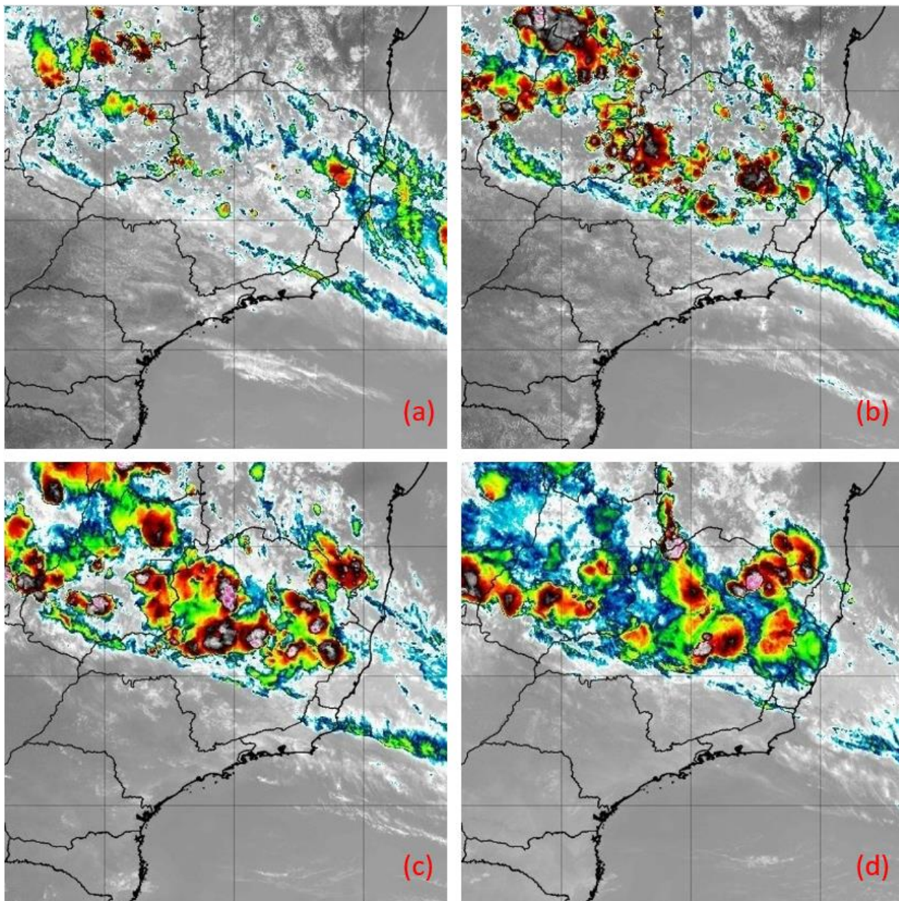
Figura 8 - Imagens do satélite GOES-16 do dia 07/12/2019 as 12:00 (a), 15:00 (b), 18:00 (c) e 21:00 horas local. Fonte: INPE.
