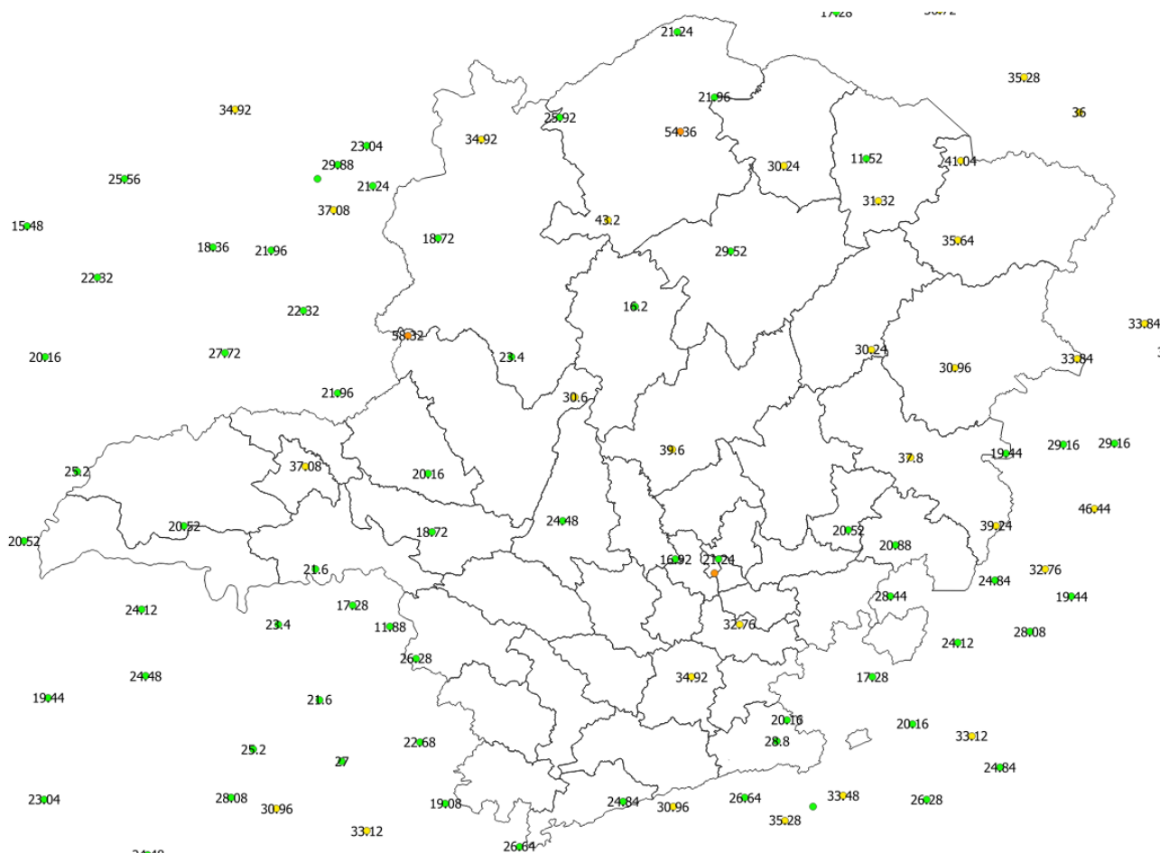
Figura 10 - Rajadas de vento registradas no dia 07/12/2019. Fonte: INMET.
