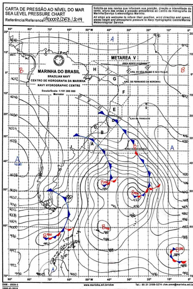
Figura 7 - Carta Sinótica do Dia 07/12/2019. Fonte: Marinha Brasileira.
