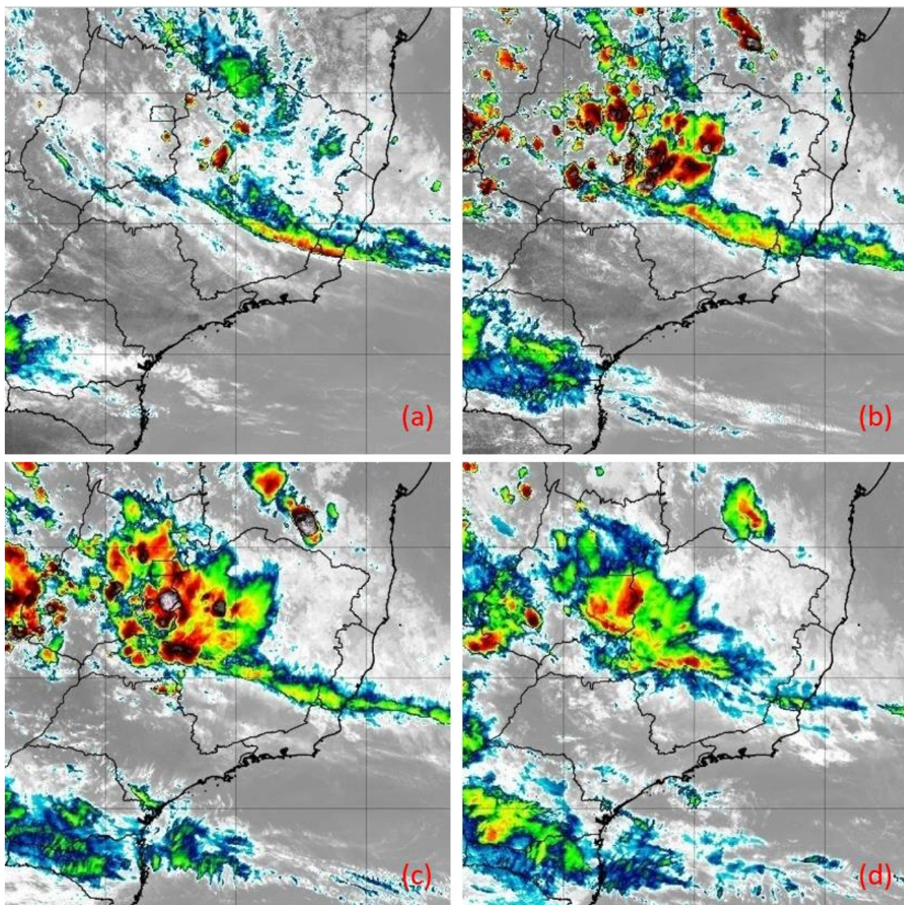
Figura 13 encontra-se as imagens de satélite do dia 30/11, onde pode-se ver o desenvolvimento de diversos núcleos convectivos em diversas regiões do estado, mas notadamente entre o Triângulo Mineiro, Sul e Noroeste de Minas. Estes sistemas iniciaram-se desde o final da manhã no Triângulo e
