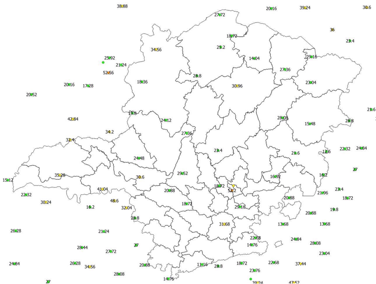
Figura 15 - Rajadas de vento registradas no dia 08/12/2019. Fonte: INMET.
