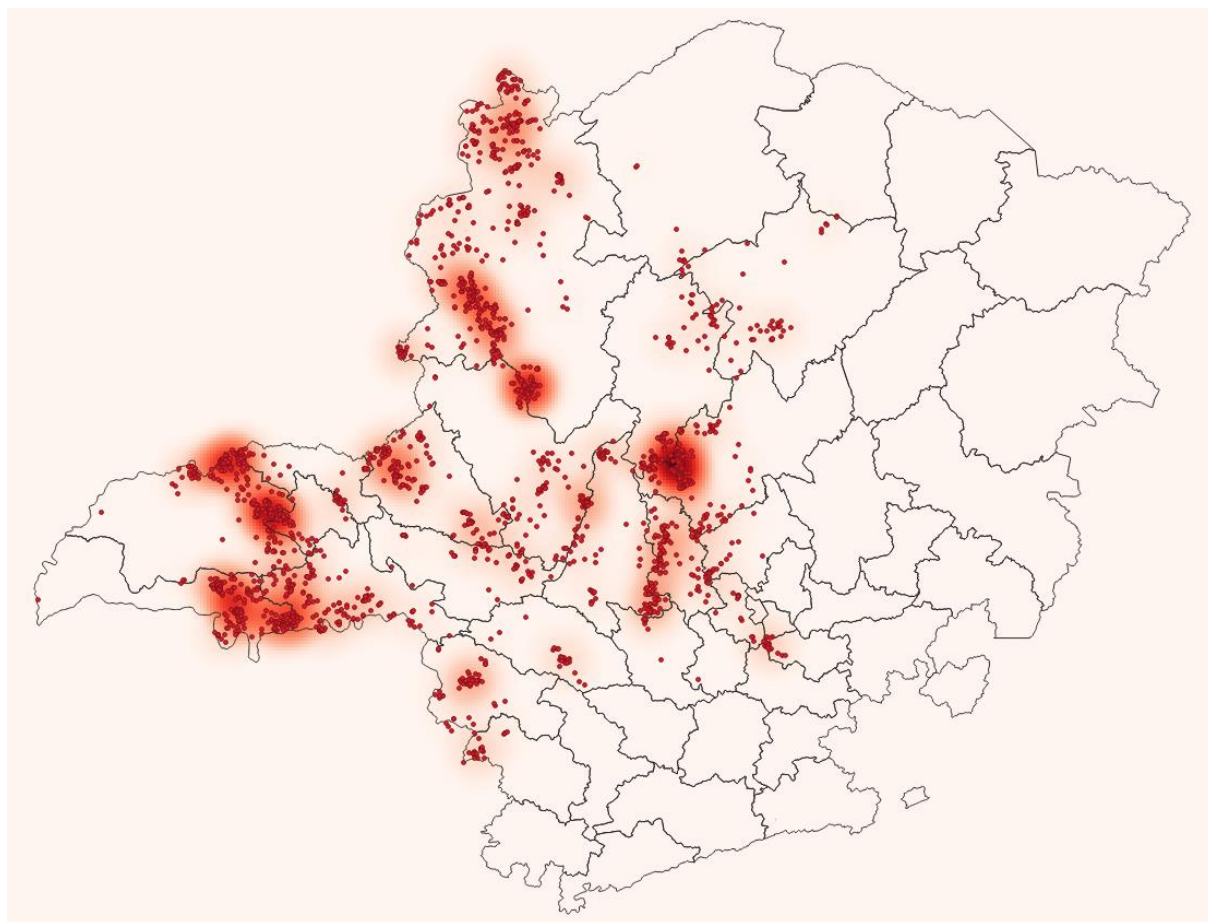
Figura 19 - Raios registrados no dia 09/12/2019. Fonte: RINDAT.
