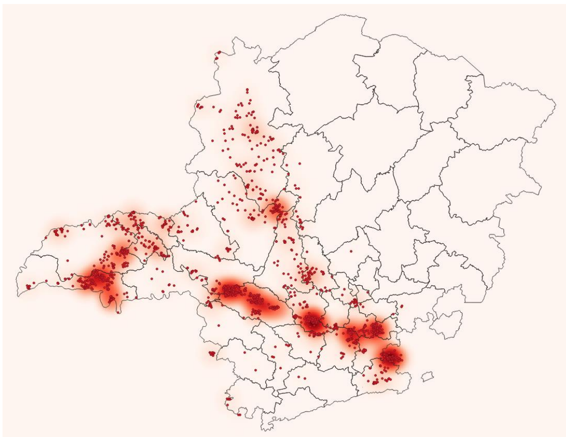
Figura 24 - Raios registrados no dia 10/12/2019. Fonte: RINDAT.
