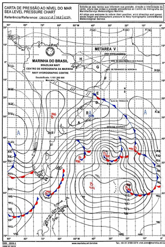
Figura 12 - Carta Sinótica do Dia 08/12/2019. Fonte: Marinha Brasileira.
