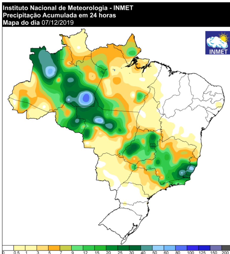
Figura 6 - Precipitação ocorrida no dia 06/12/2019. Fonte: INMET.
