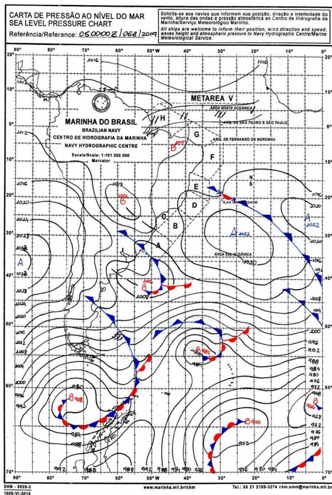
Figura 1 - Carta sinótica do dia 05/12/2019. Fonte: Marinha Brasileira.
