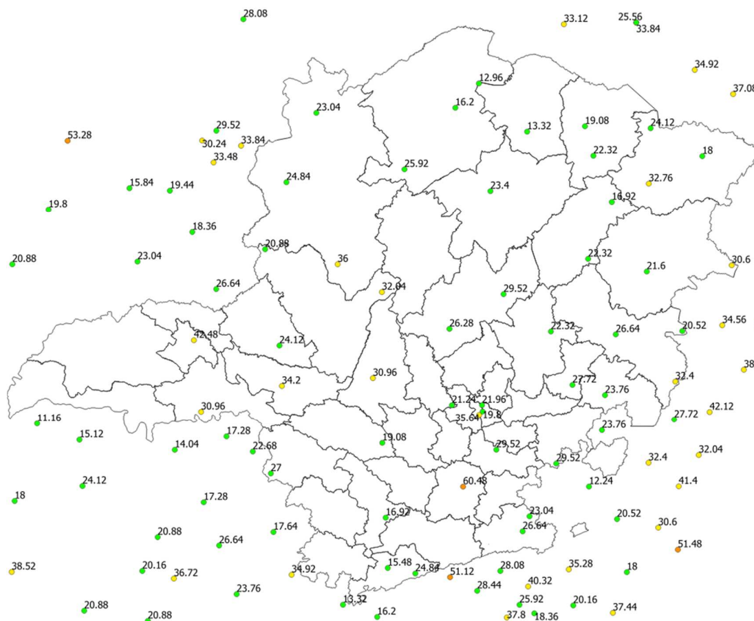
Figura 20 - Rajadas de vento registradas no dia 11/01/2020. Fonte: INMET.
