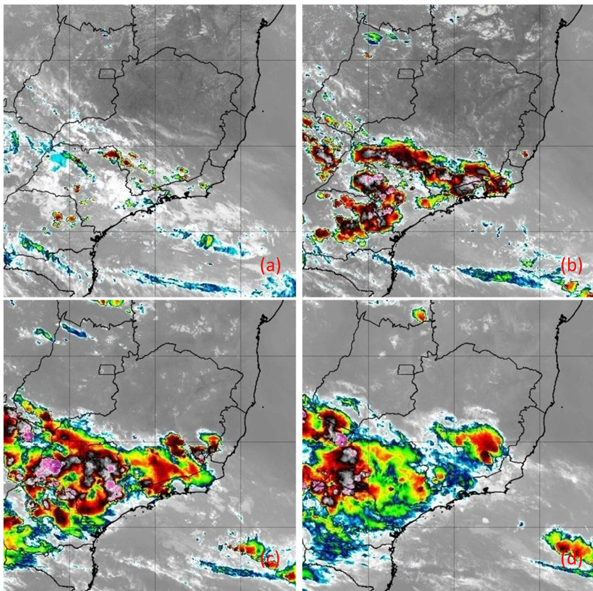
Figura 23 - Imagens do satélite GOES-16 do dia 12/01/2020 as 15:00 (a), 18:00 (b), 21:00 (c) e 24:00 horas local (d). Fonte: INPE.
