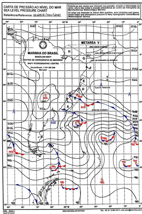
Figura 22 - Carta Sinótica do Dia 12/01/2020. Fonte: Marinha Brasileira.
