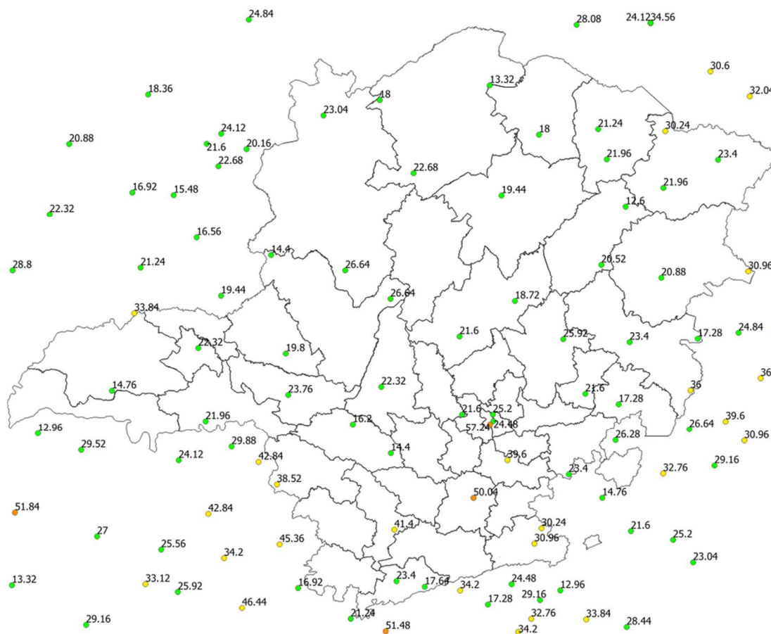
Figura 25 - Rajadas de vento registradas no dia 12/01/2020. Fonte: INMET.
