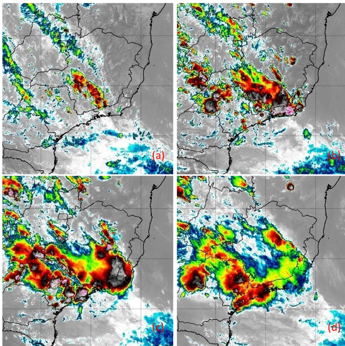
Figura 3 - Imagens do satélite GOES-16 do dia 08/01/2020 as 15:00 (a), 18:00 (b), 21:00 (c) e 24:00 horas local (d). Fonte: INPE.
