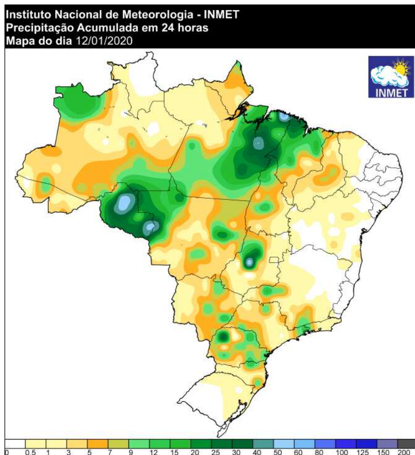
Figura 21 - Precipitação ocorrida no dia 11/01/2020. Fonte: INMET.
