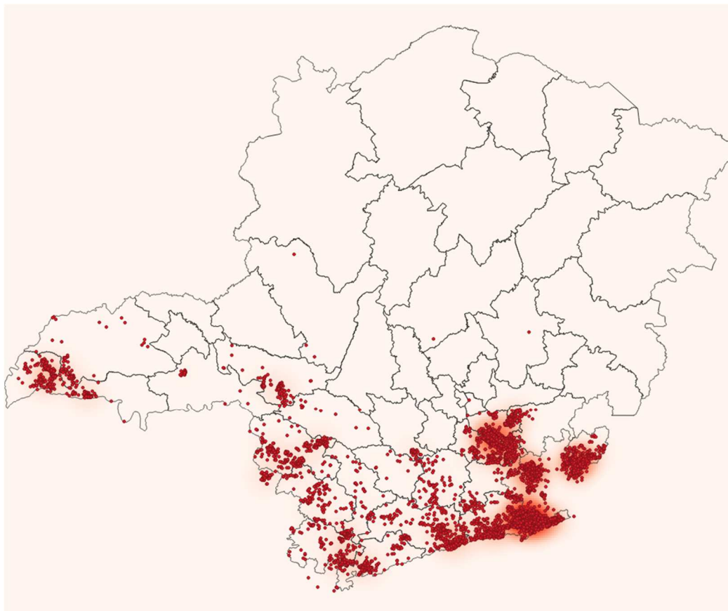
Figura 24 - Raios registrados no dia 12/01/2020. Fonte: RINDAT.
