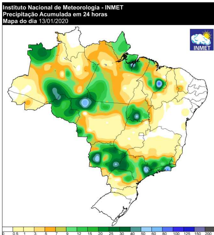
Figura 26 - Precipitação ocorrida no dia 12/01/2020. Fonte: INMET.
