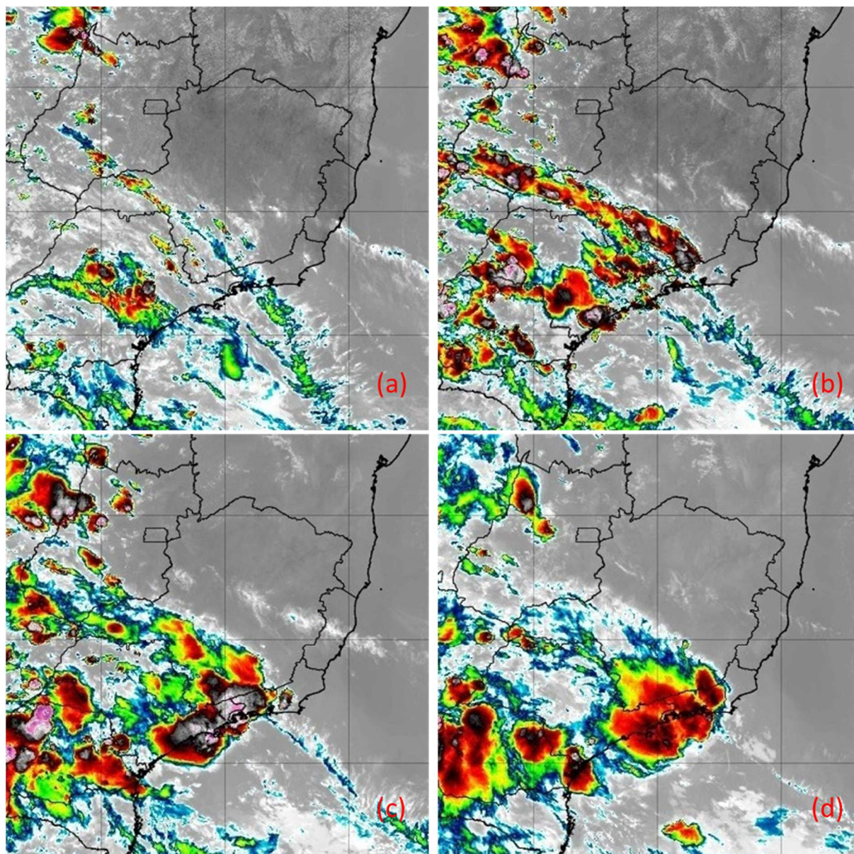
Figura 18 - Imagens do satélite GOES-16 do dia 11/01/2020 as 15:00 (a), 18:00 (b), 21:00 (c) e 24:00 horas local (d). Fonte: INPE.
