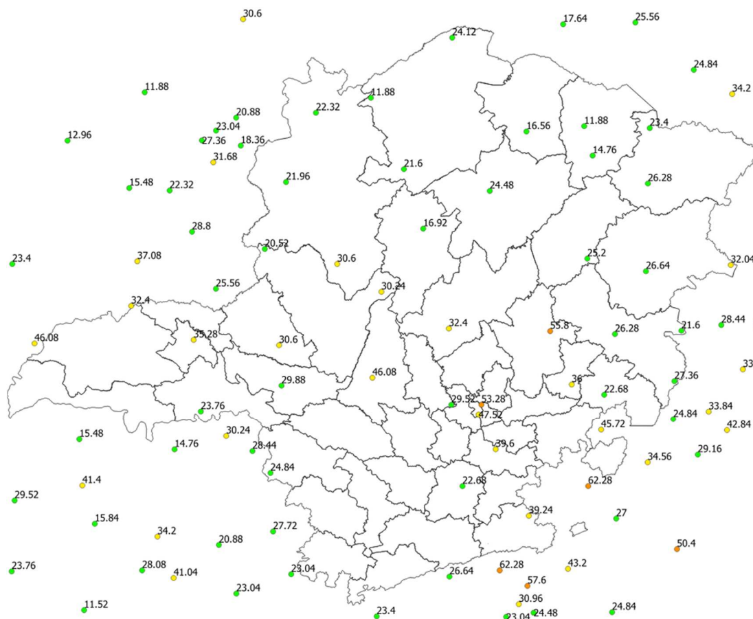
Figura 5 - Rajadas de vento registradas no dia 08/01/2020. Fonte: INMET.
