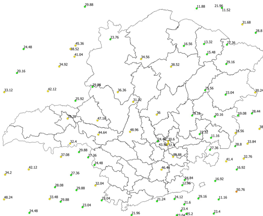
Figura 10 - Rajadas de vento registradas no dia 09/01/2020. Fonte: INMET.
