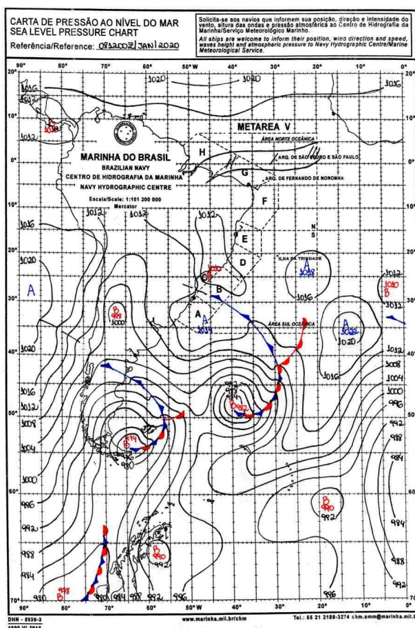
Figura 2 - Carta Sinótica do Dia 08/01/2020. Fonte: Marinha Brasileira.
