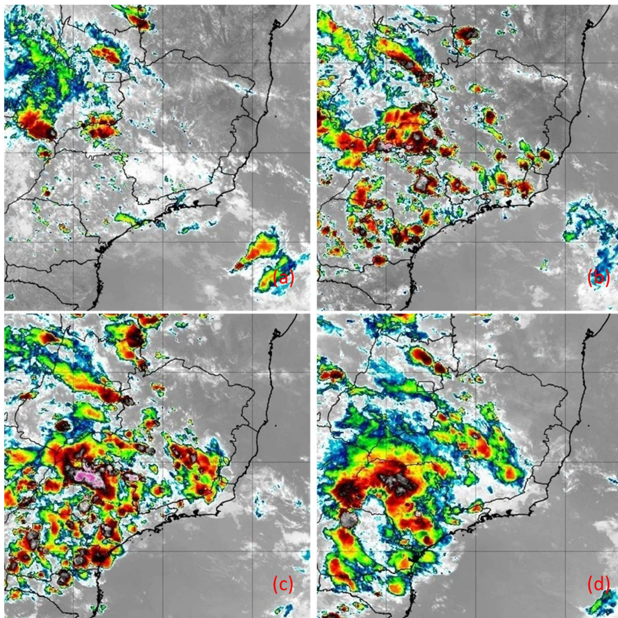
Figura 8 - Imagens do satélite GOES-16 do dia 09/01/2020 as 15:00 (a), 18:00 (b), 21:00 (c) e 24:00 horas local (d). Fonte: INPE.
