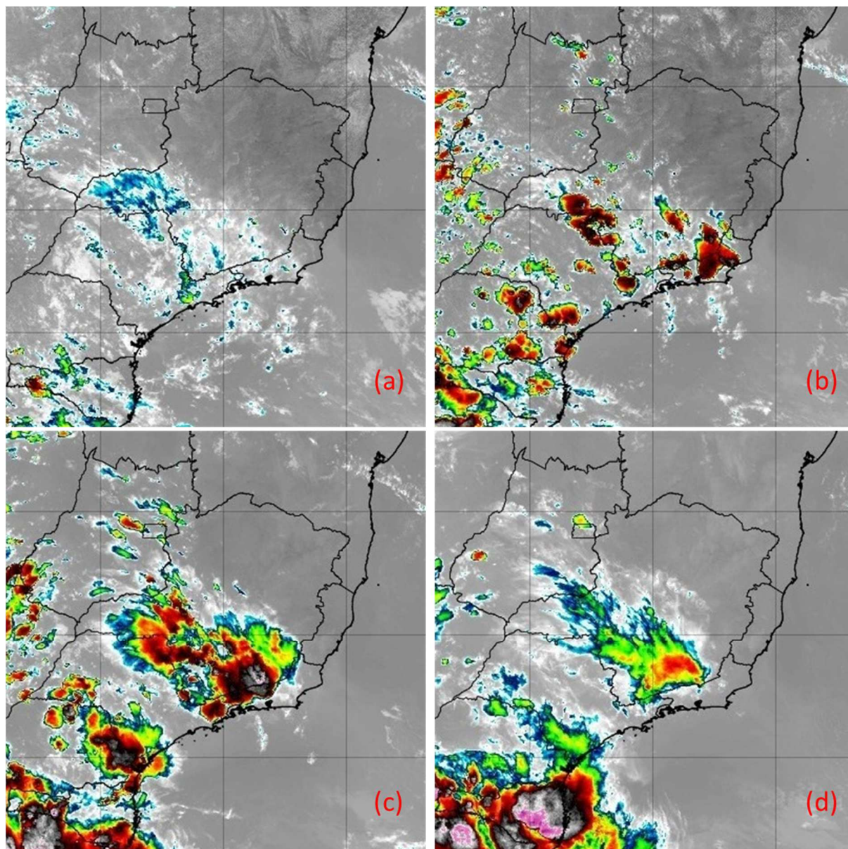
Figura 13 - Imagens do satélite GOES-16 do dia 10/01/2020 as 15:00 (a), 18:00 (b), 21:00 (c) e 24:00 horas local (d). Fonte: INPE.
