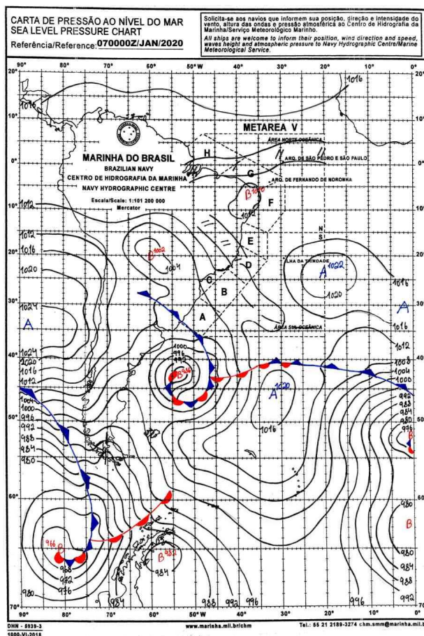
Figura 1 - Carta Sinótica do Dia 07/01/2020. Fonte: Marinha Brasileira.
