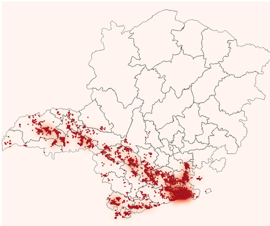
Figura 19 - Raios registrados no dia 11/01/2020. Fonte: RINDAT.
