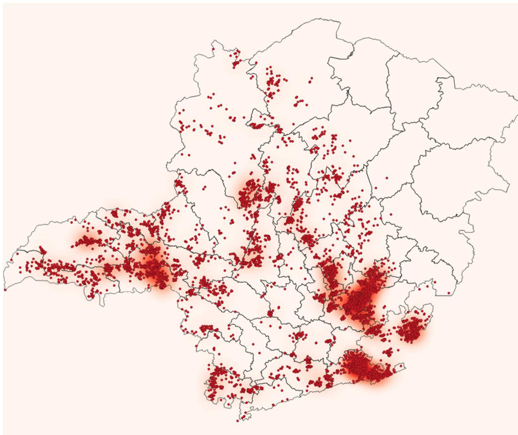
Figura 9 - Raios registrados no dia 09/01/2020. Fonte: RINDAT.
