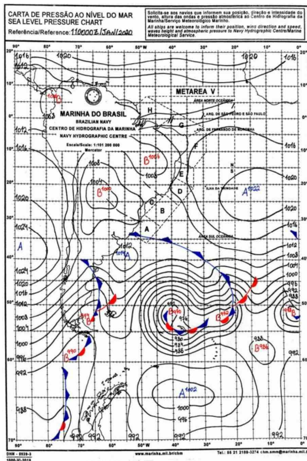
Figura 17 - Carta Sinótica do Dia 11/01/2020. Fonte: Marinha Brasileira.
