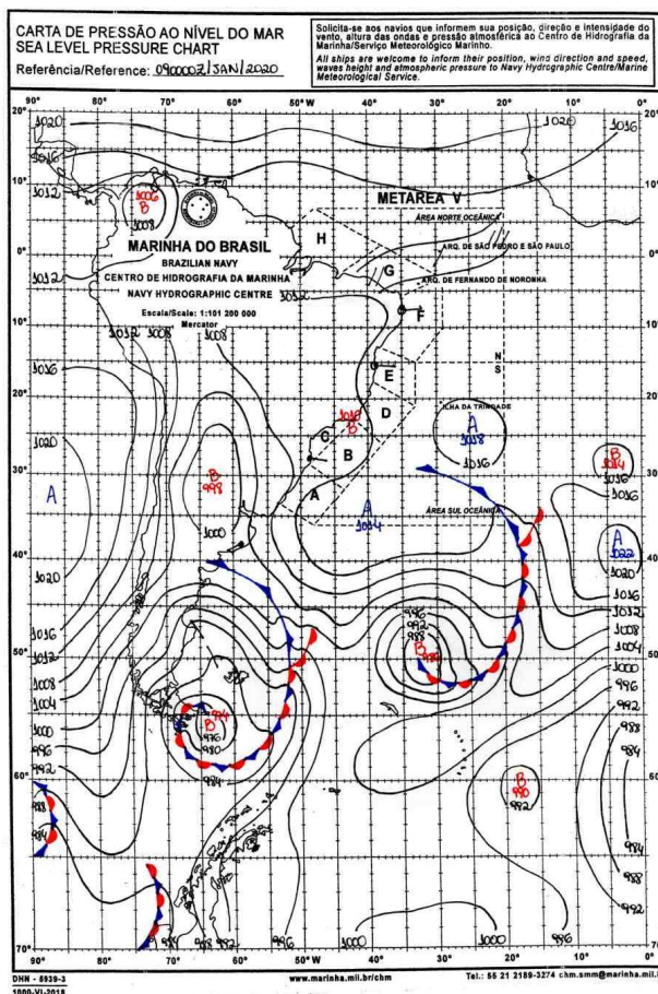
Figura 7 - Carta Sinótica do Dia 09/01/2020. Fonte: Marinha Brasileira.
