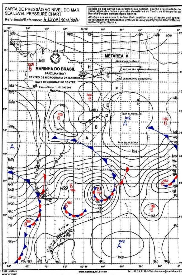
Figura 12 - Carta Sinótica do Dia 10/01/2020. Fonte: Marinha Brasileira.
