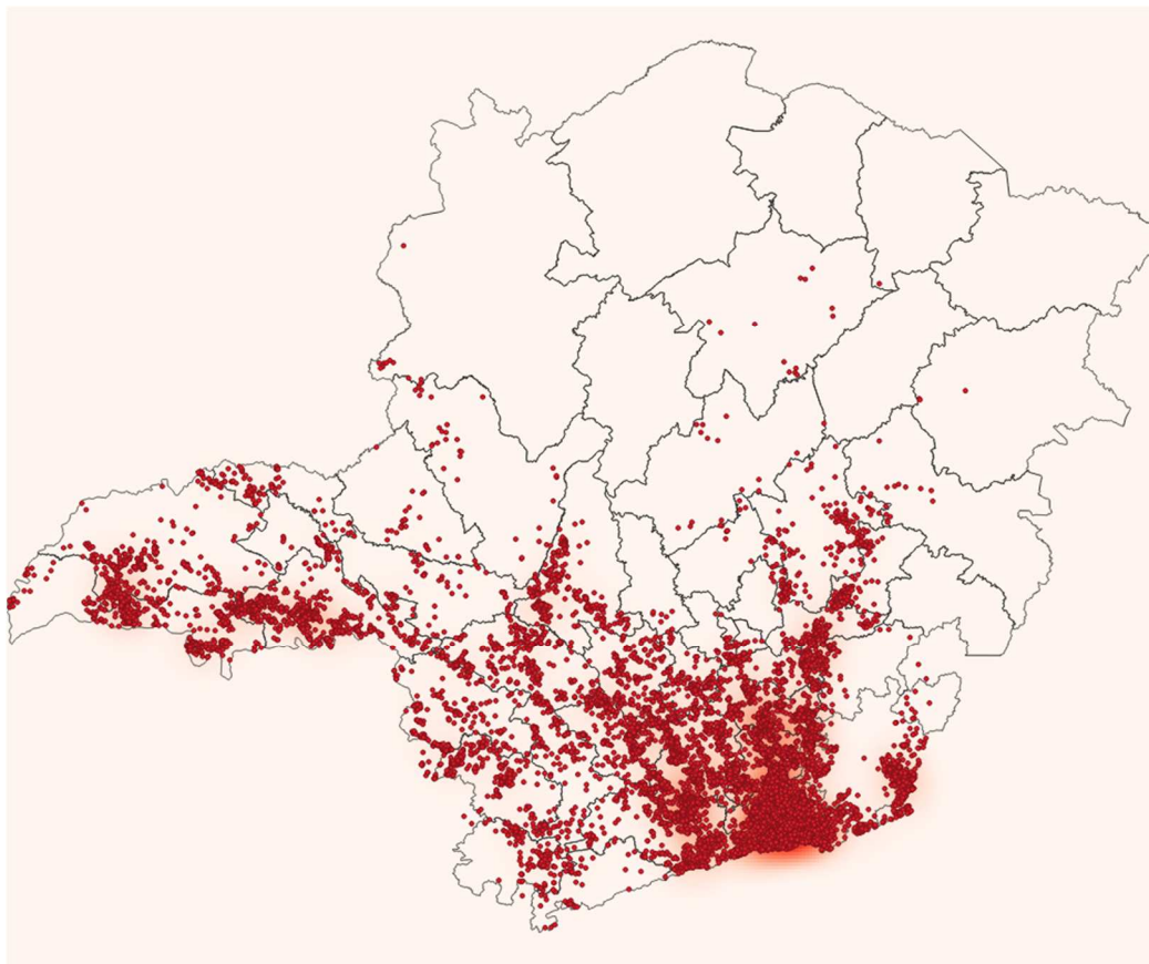
Figura 4 - Raios registrados no dia 08/01/2020. Fonte: RINDAT.
