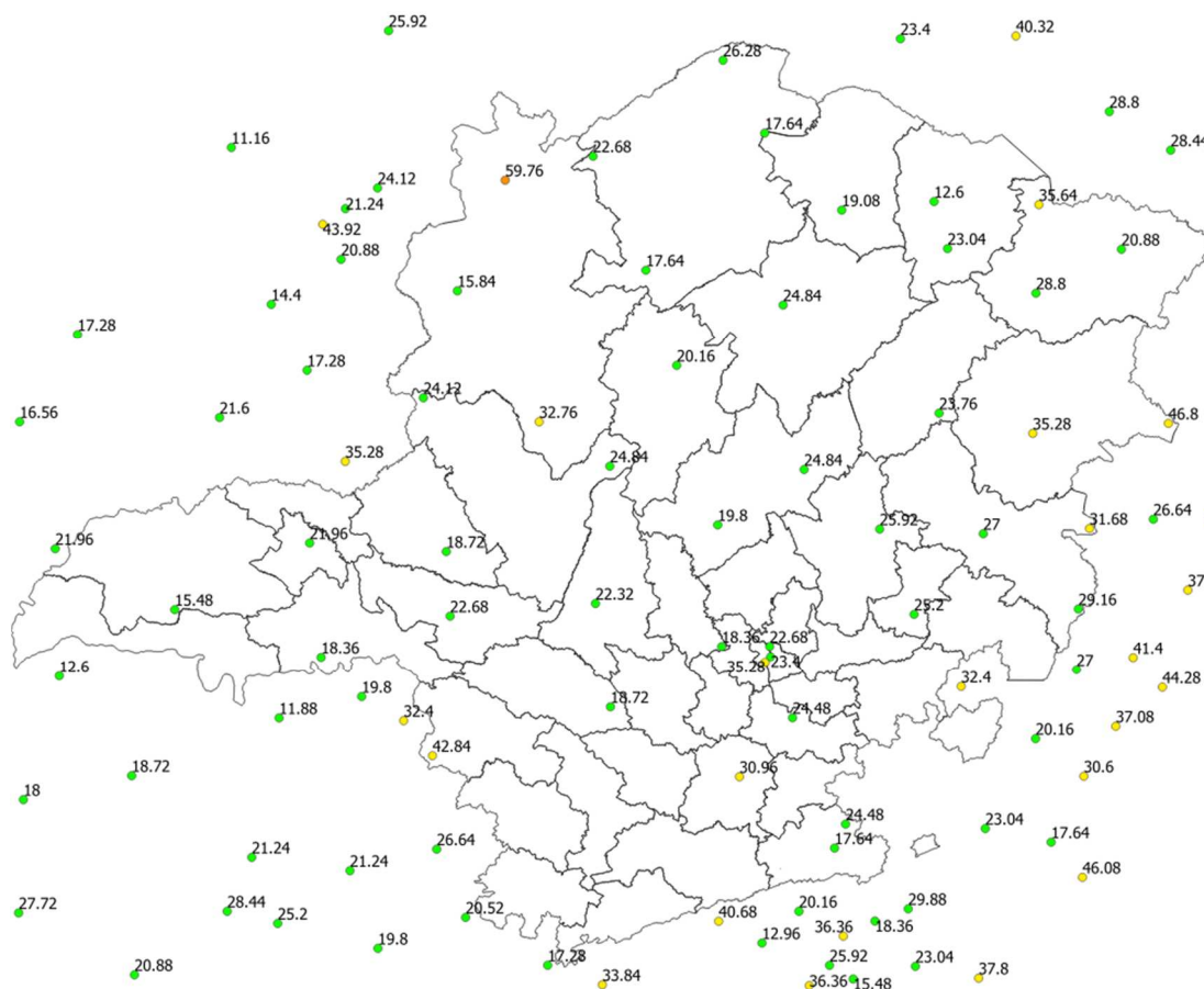
Figura 15 - Rajadas de vento registradas no dia 10/01/2020. Fonte: INMET.
