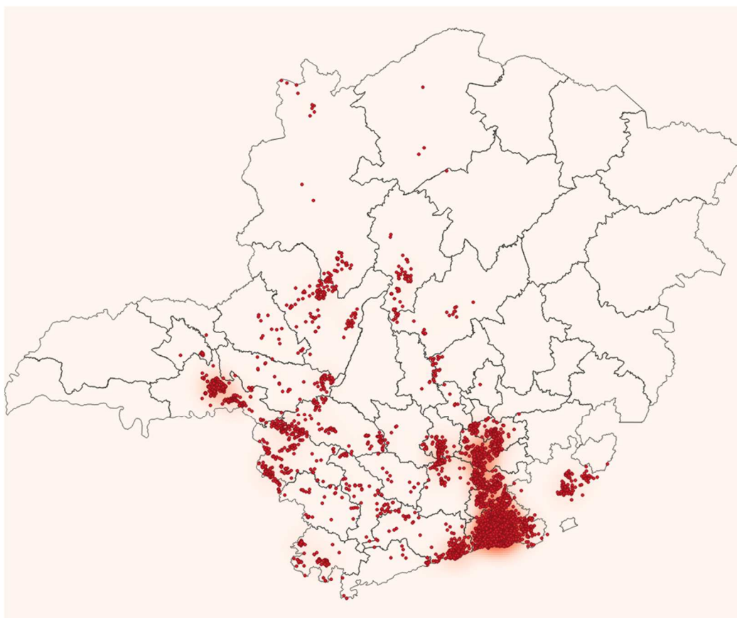
Figura 14 - Raios registrados no dia 10/01/2020. Fonte: RINDAT.
