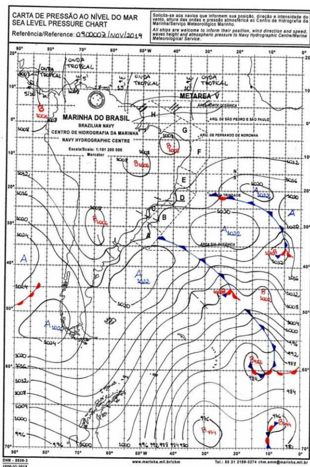
Figura 7 Carta Sinótica do dia 09/11/2019. Fonte: Marinha Brasileira.
