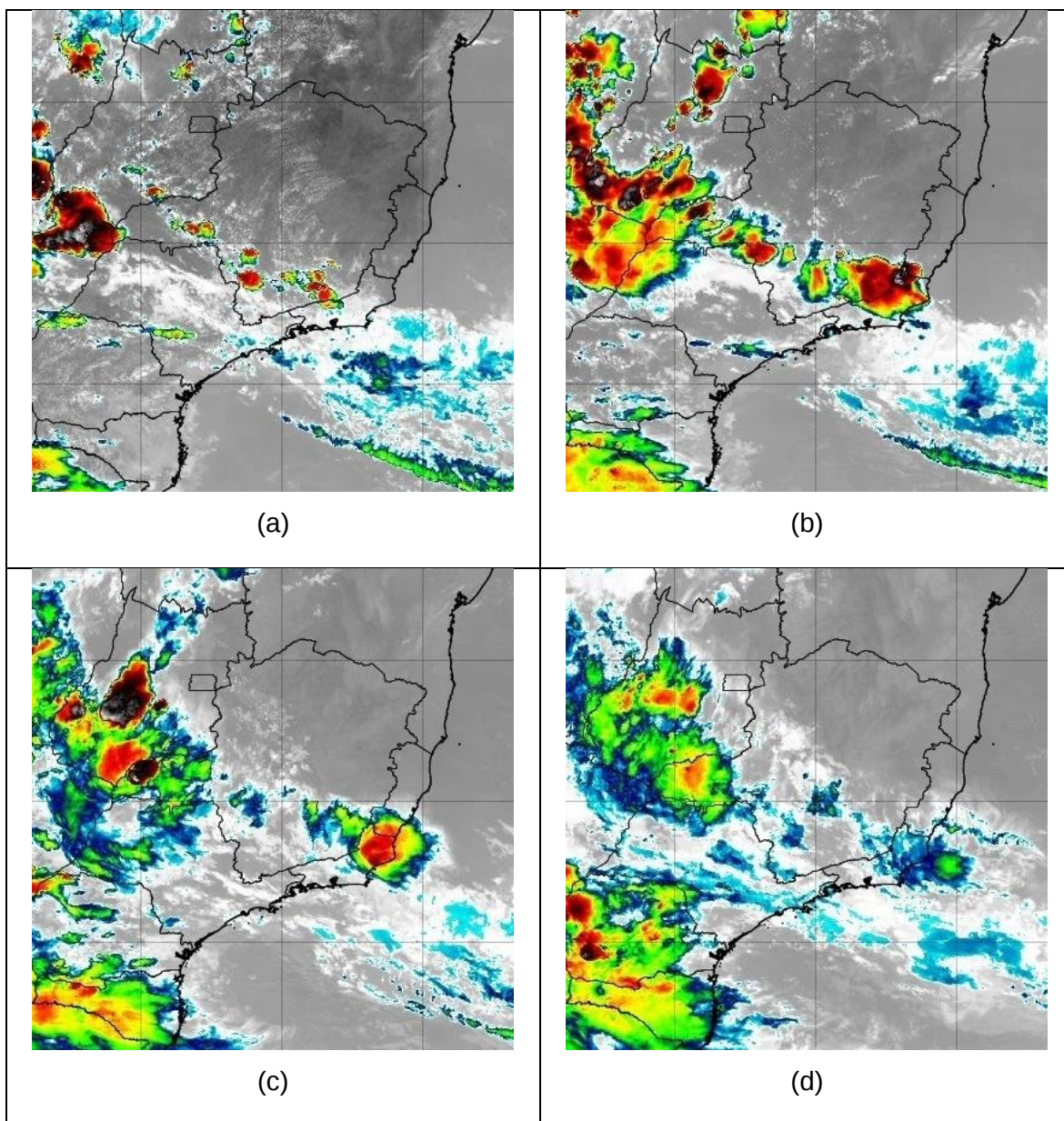
Figura 8 Imagens de Satélite do dia 09/11 as 14:00 (a), 17:00 (b), 20:00 (c) e 23:00 (d). Fonte: INPE
