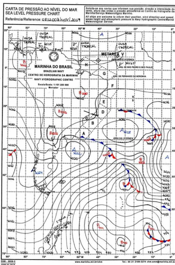
Figura 2 Carta Sinótica do dia 08/11/2019. Fonte: Marinha Brasileira
