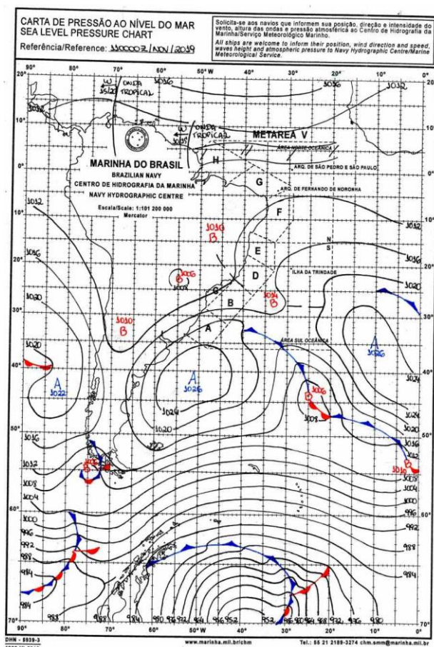
Figura 10 Carta Sinótica do dia 11/11/2019. Fonte: Marinha Brasileira.
