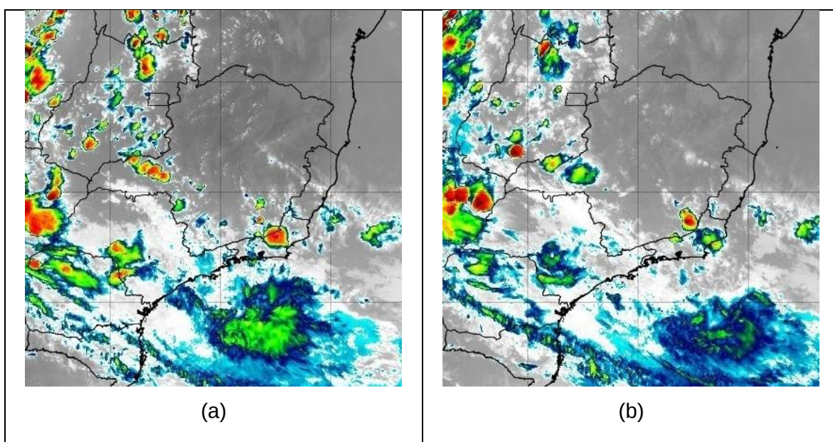
Figura 6 Imagens de Satélite do dia 10/11 as 17:00 (a) e 19:00 (b). Fonte: INPE.
