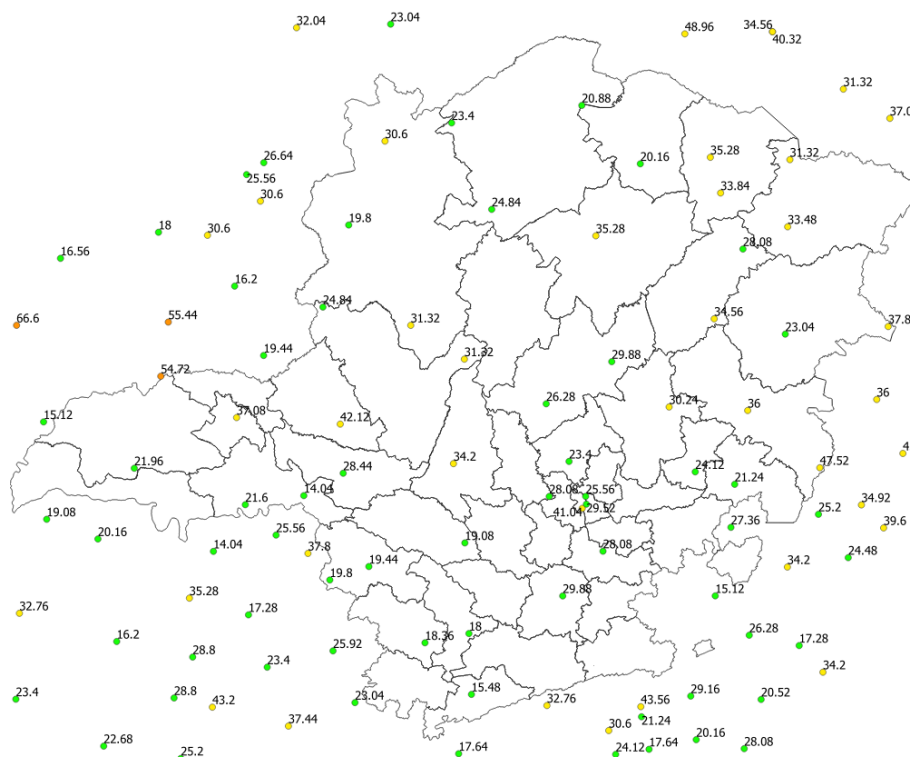
Figura 8 Localização das maiores rajadas de vento registradas no dia 10/11/2019. Fonte: INMET.
