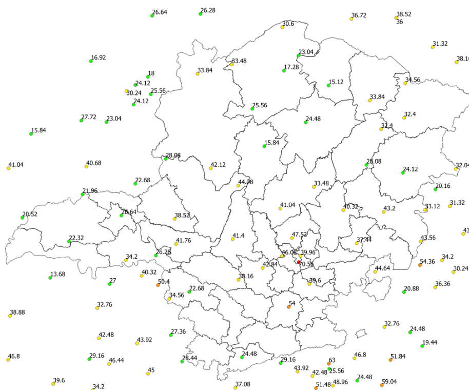
Figura 20 Localização das maiores rajadas de vento registradas no dia 11/11/2019. Fonte: INMET.
