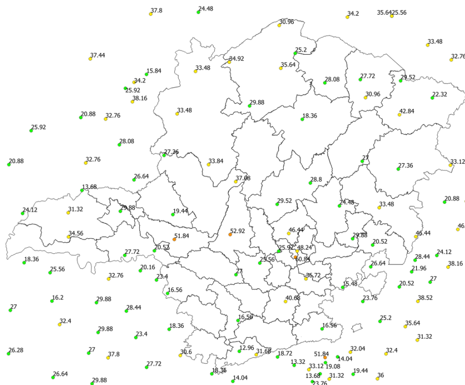
Figura 5 Localização das maiores rajadas de vento registradas no dia 08/11/2019. Fonte: INMET.
