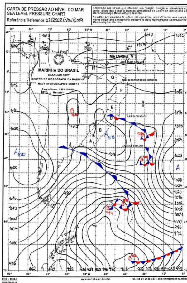
Figura 1 - Carta Sinótica do dia 07/11/2019. Fonte: Marinha Brasileira
