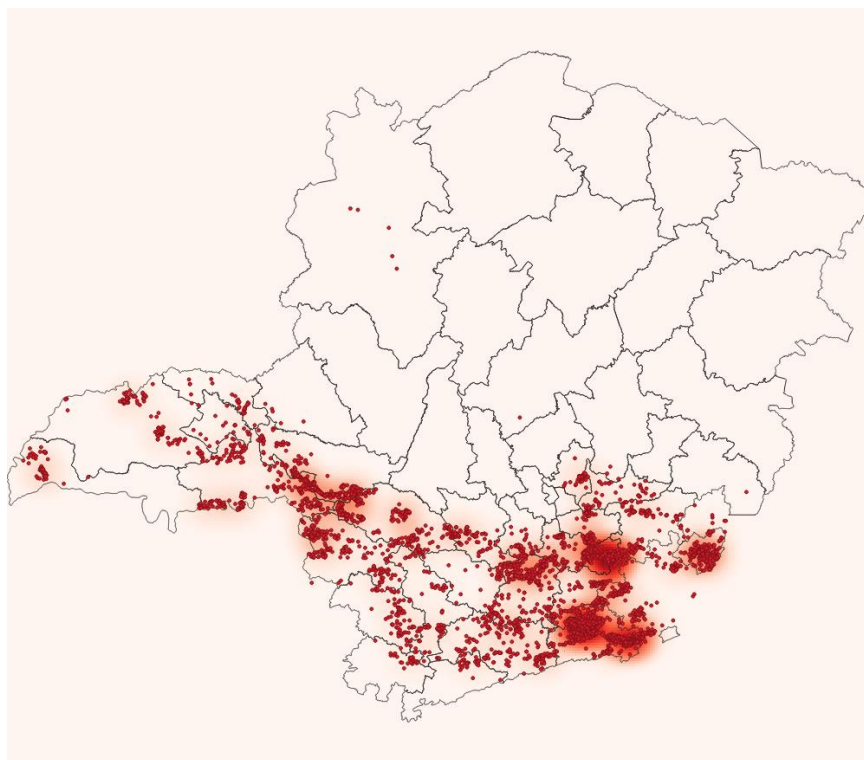
Figura 12 Localização dos raios registrados no dia 11/11/2019
