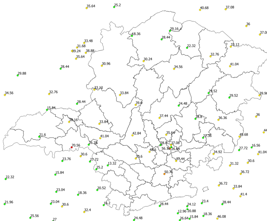
Figura 10 Localização das maiores rajadas de vento registradas no dia 09/11/2019. Fonte: INMET.
