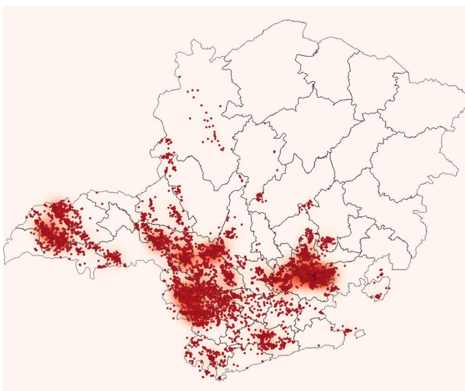
Figura 4 Localização dos raios registrados no dia 08/11/2019. Fonte: RINDAT.
