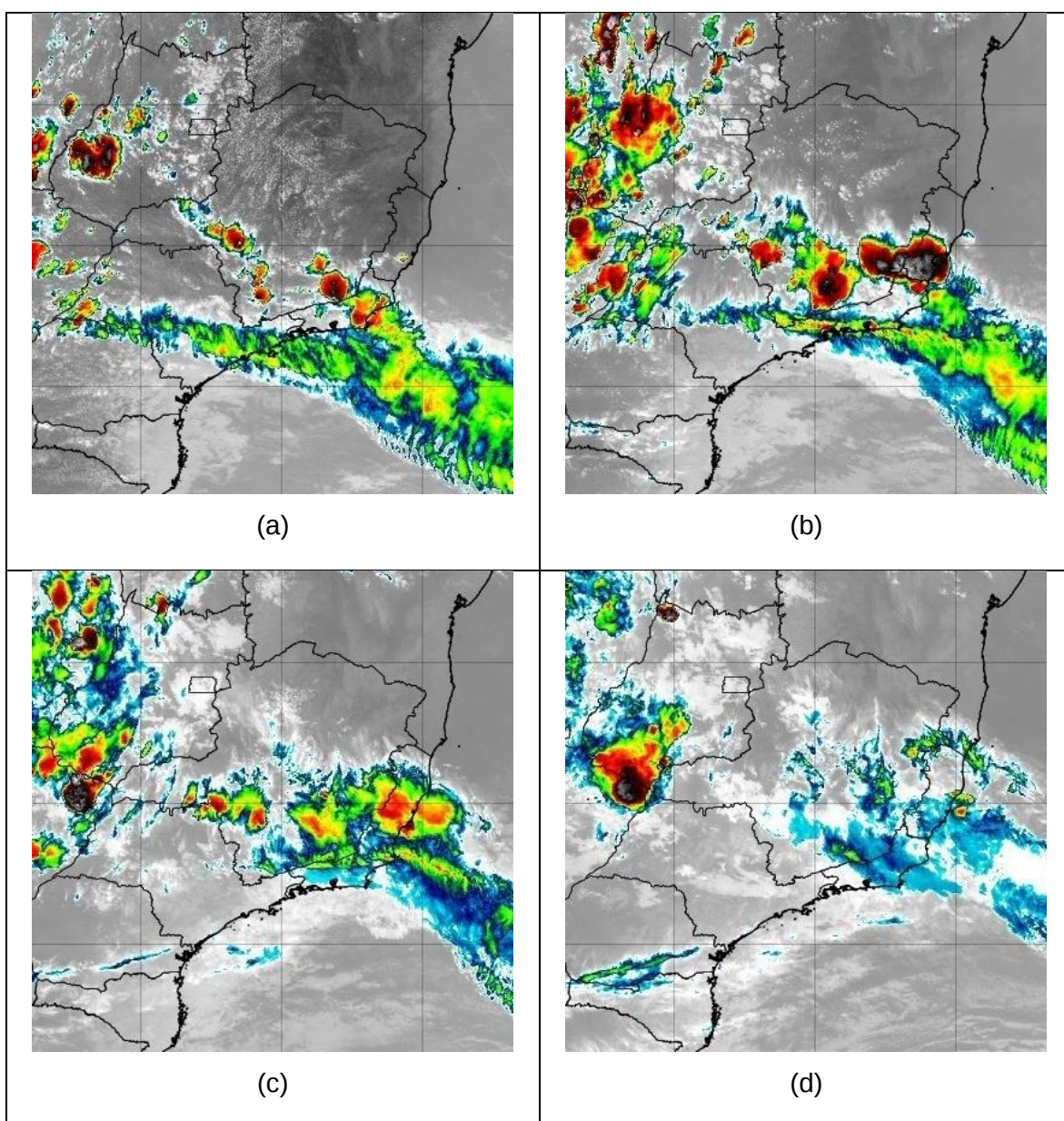
Figura 11 Imagens de Satélite do dia 11/11 as 14:00 (a), 17:00 (b), 20:00 (c) e 23:00 (d). Fonte: INPE.
