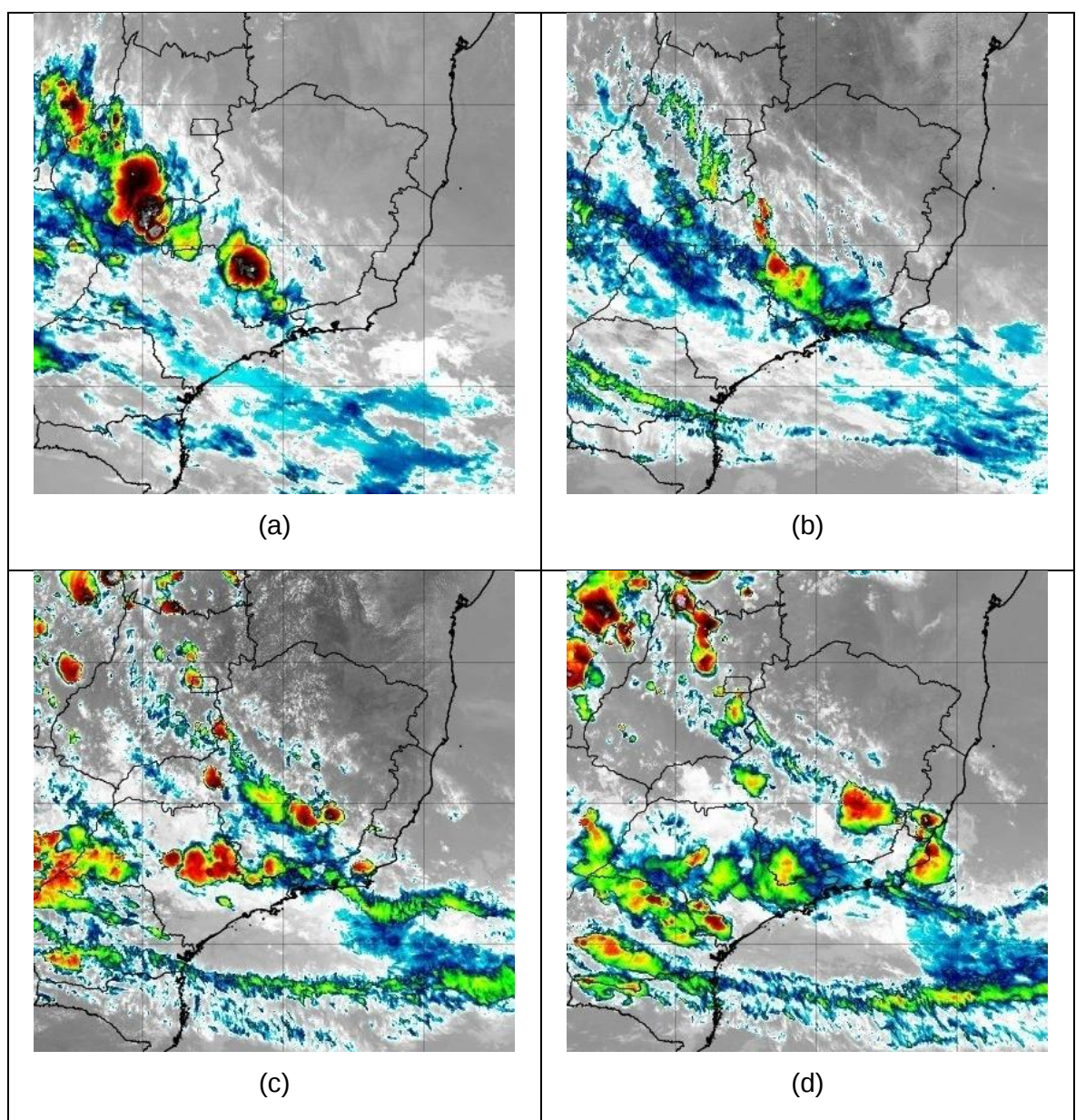
Figura 3 Imagens de Satélite do dia 08/11 as 01:00 (a), 09:00 (b), 15:00 (c) e 18:00 (d). Fonte: INPE
