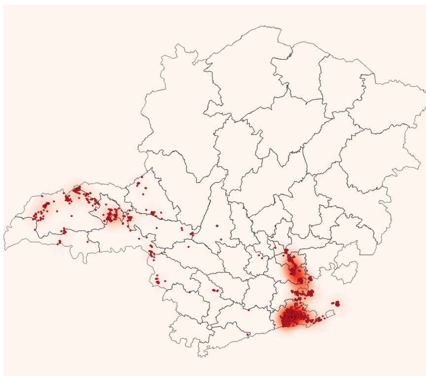
Figura 7 Localização dos raios registrados no dia 10/11/2019. Fonte: RINDAT.
