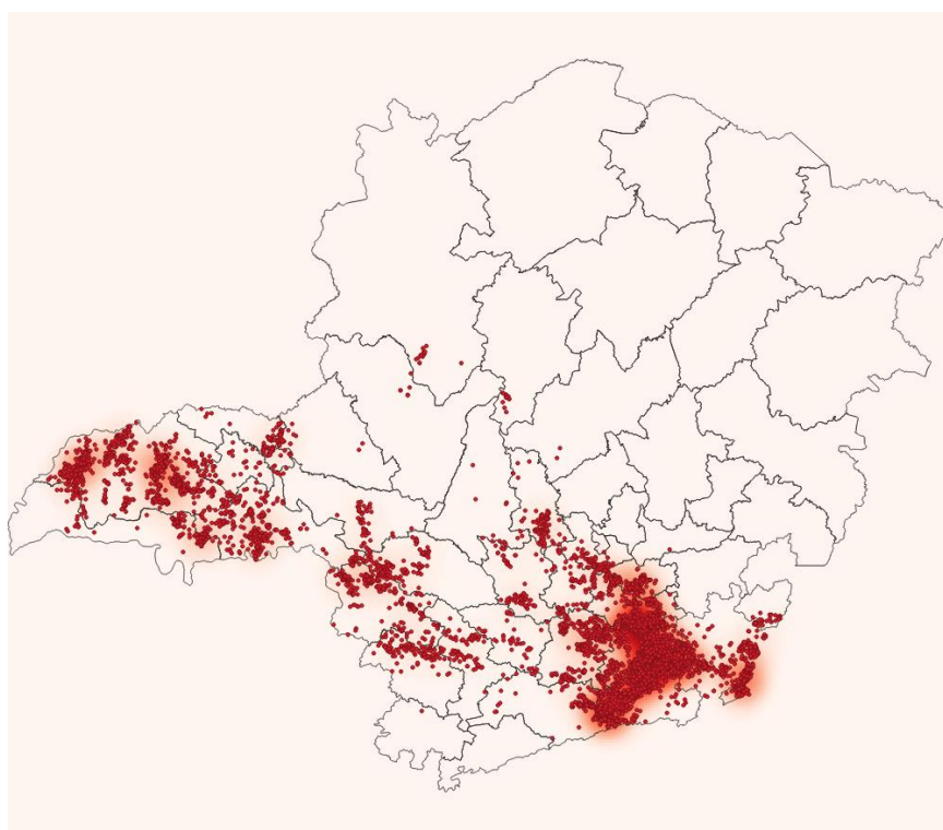
Figura 9 Localização dos raios registrados no dia 09/11/2019
