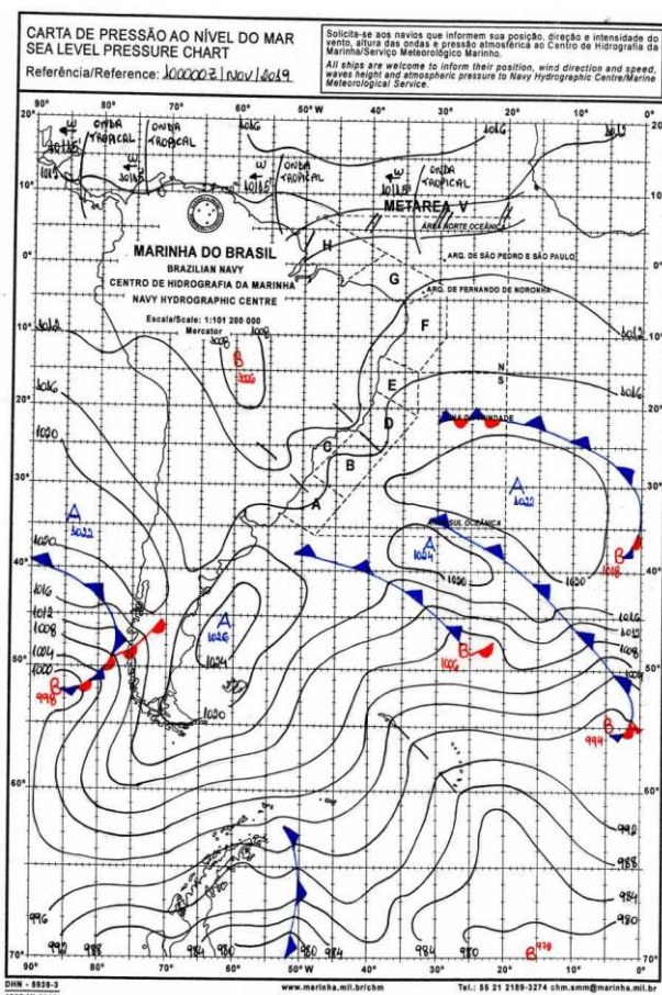
Figura 5 Carta Sinótica do dia 10/11/2019. Fonte: Marinha Brasileira.
