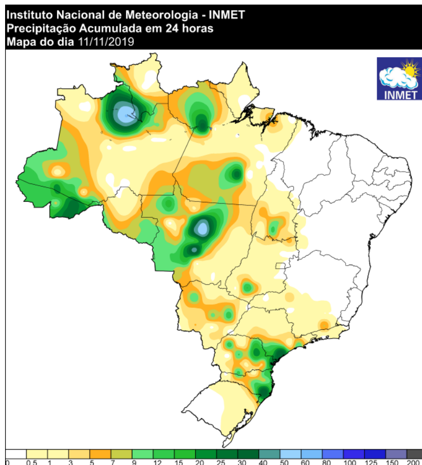
Figura 9 Pluviometria do dia 10/11/2019
