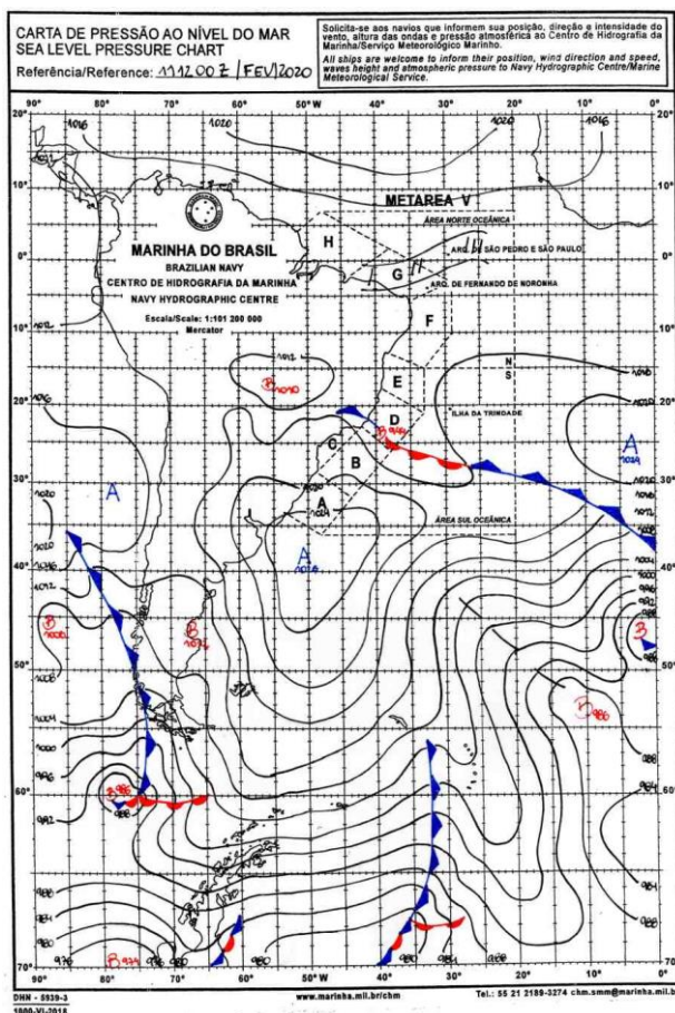
Figura 2 - Carta Sinótica do Dia 11/02/2020. Fonte: Marinha Brasileira.
