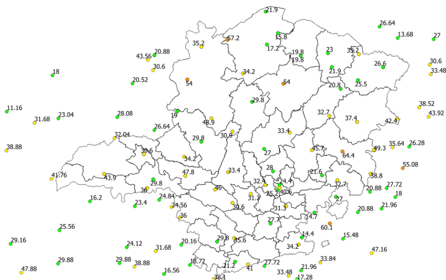
Figura 5 - Rajadas de vento registradas no dia 11/02/2020. Fonte: INMET.
