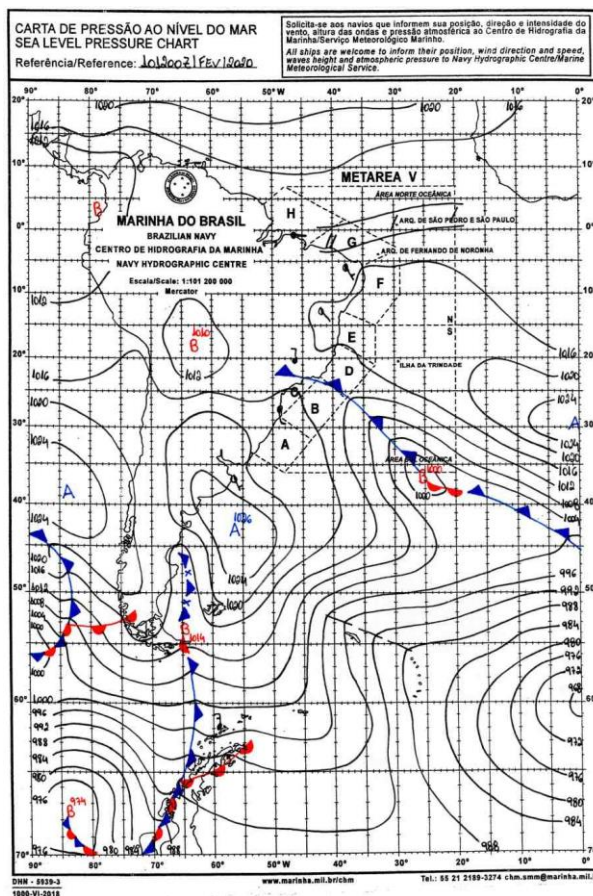
Figura 1 - Carta Sinótica do Dia 10/02/2020. Fonte: Marinha Brasileira.
