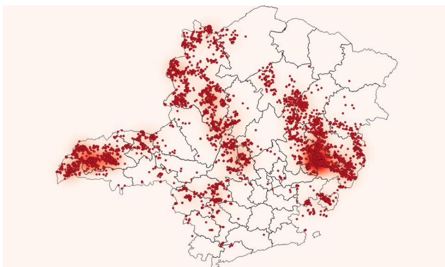
Figura 4 - Raios registrados no dia 11/02/2020. Fonte: RINDAT.
