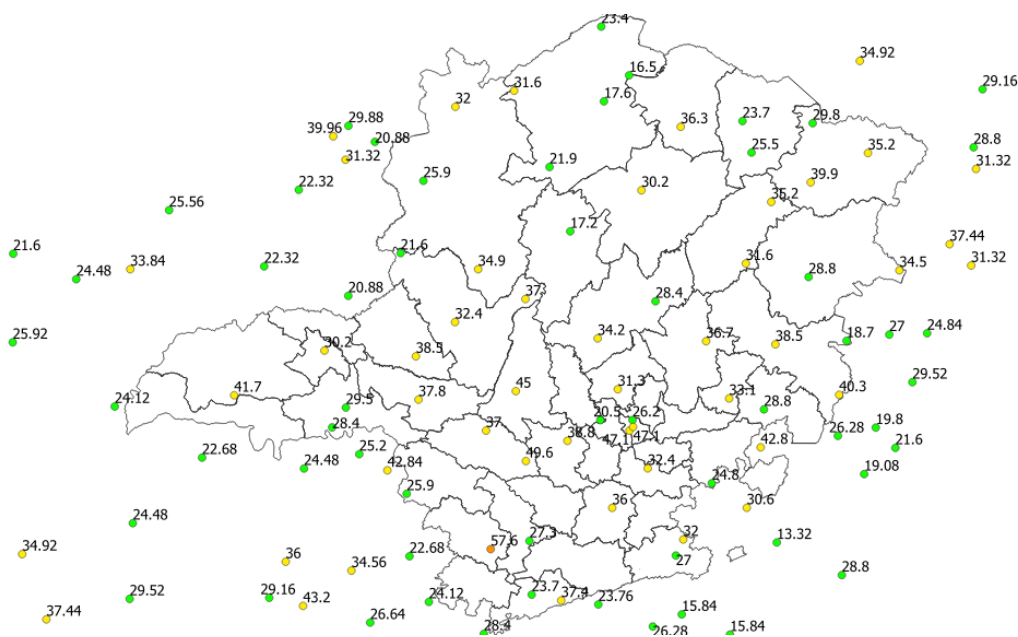
Figura 15 - Rajadas de vento registradas no dia 13/02/2020. Fonte: INMET.
