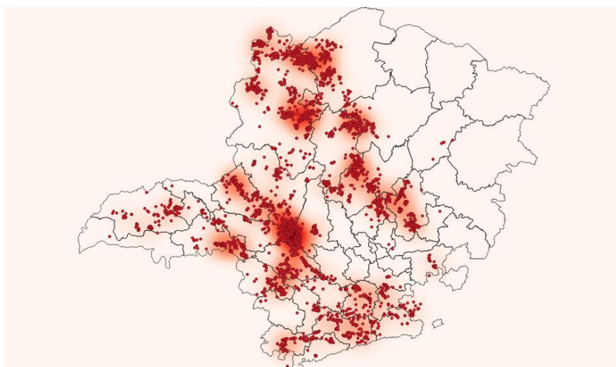
Figura 9 - Raios registrados no dia 12/02/2020. Fonte: RINDAT.
