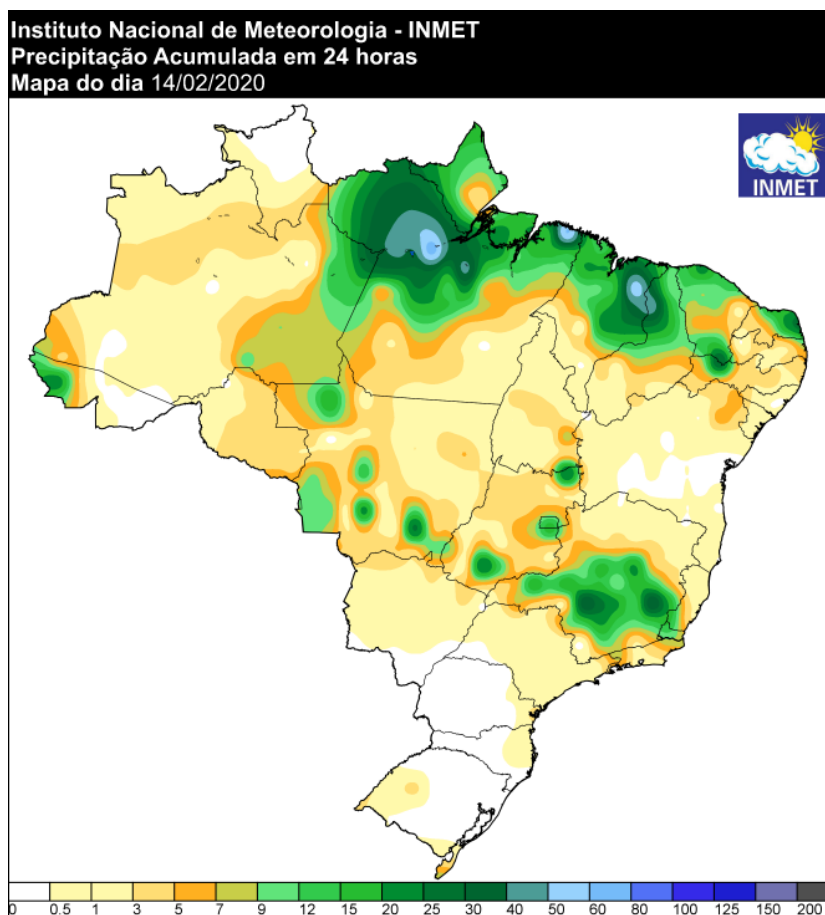
Figura 16 - Precipitação ocorrida no dia 13/02/2020. Fonte: INMET.
