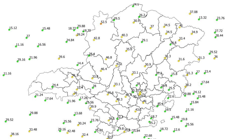
Figura 10 - Rajadas de vento registradas no dia 12/02/2020. Fonte: INMET.
