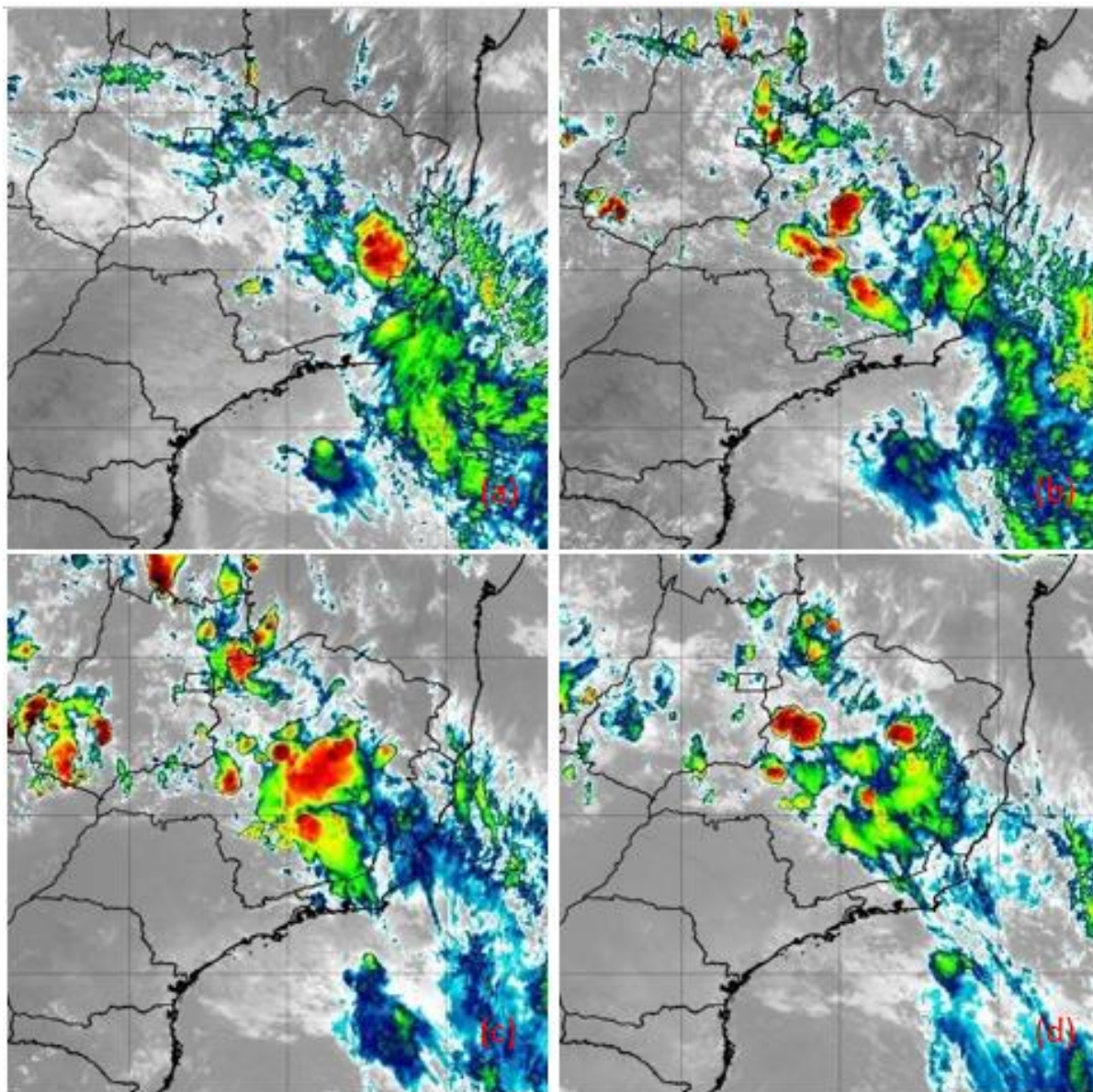
Figura 13 - Imagens do satélite GOES-16 do dia 13/02/2020 as 12:00 (a), 15:00 (b), 18:00 (c) e 21:00 horas local. Fonte: INPE.
