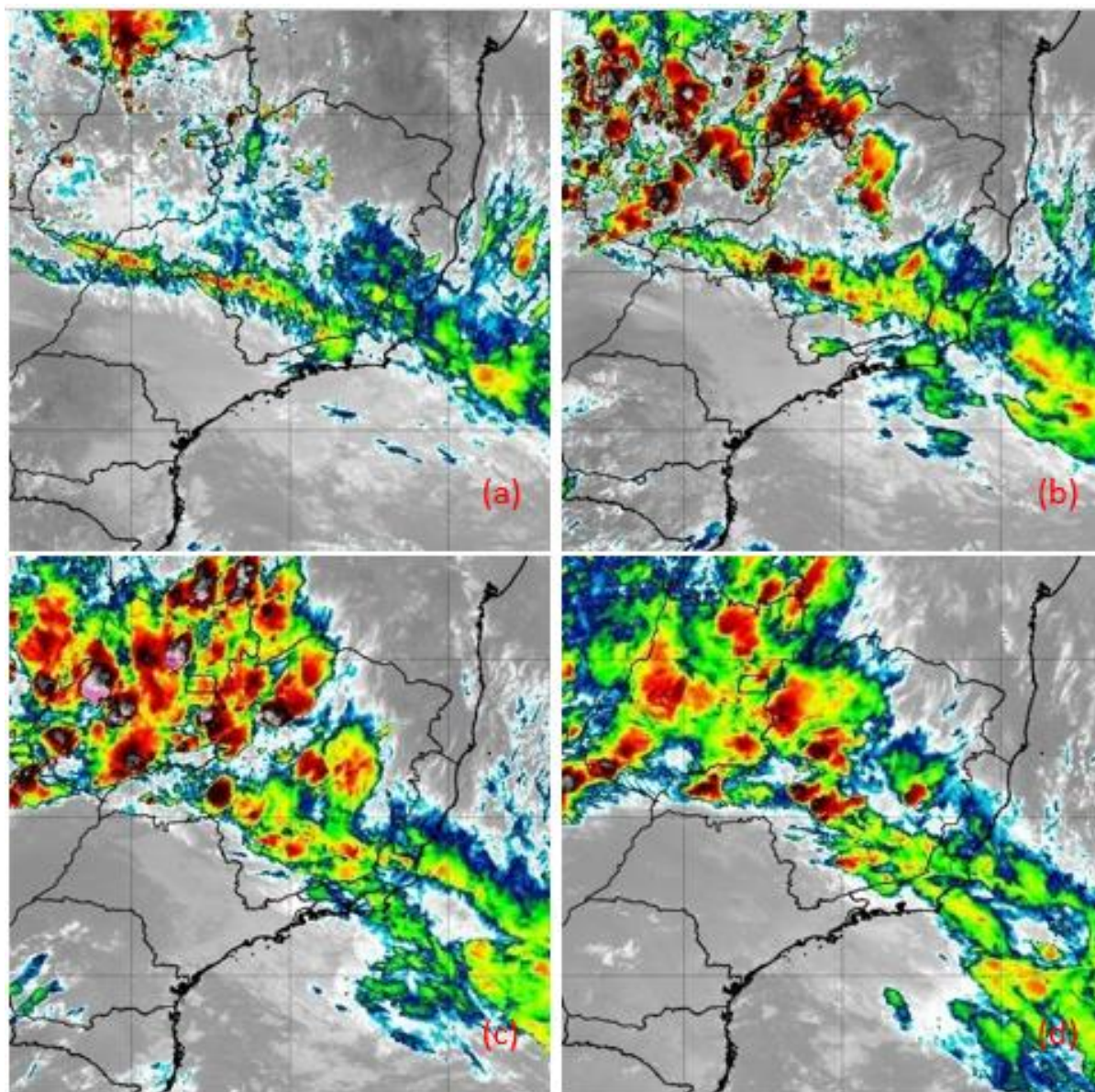
Figura 8 - Imagens do satélite GOES-16 do dia 12/02/2020 as 12:00 (a), 15:00 (b), 18:00 (c) e 21:00 horas local. Fonte: INPE.
