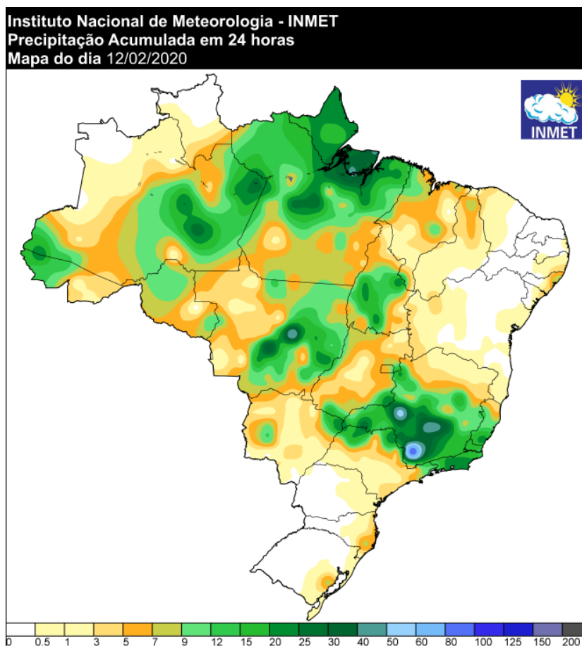
Figura 6 - Precipitação ocorrida no dia 11/02/2020. Fonte: INMET.
