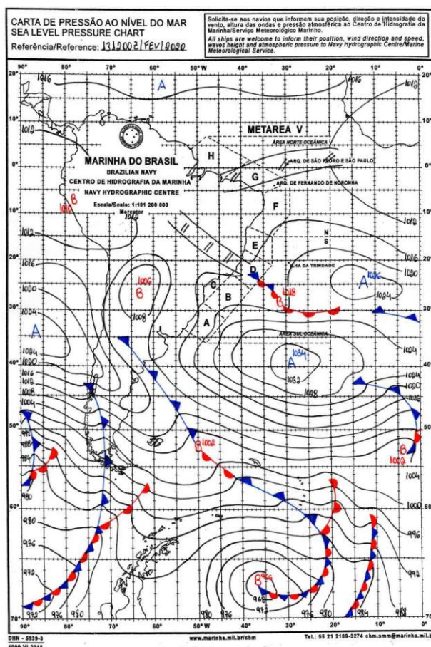
Figura 12 - Carta Sinótica do Dia 13/02/2020. Fonte: Marinha Brasileira.
