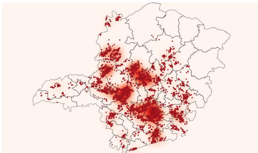
Figura 14 - Raios registrados no dia 13/02/2020. Fonte: RINDAT.
