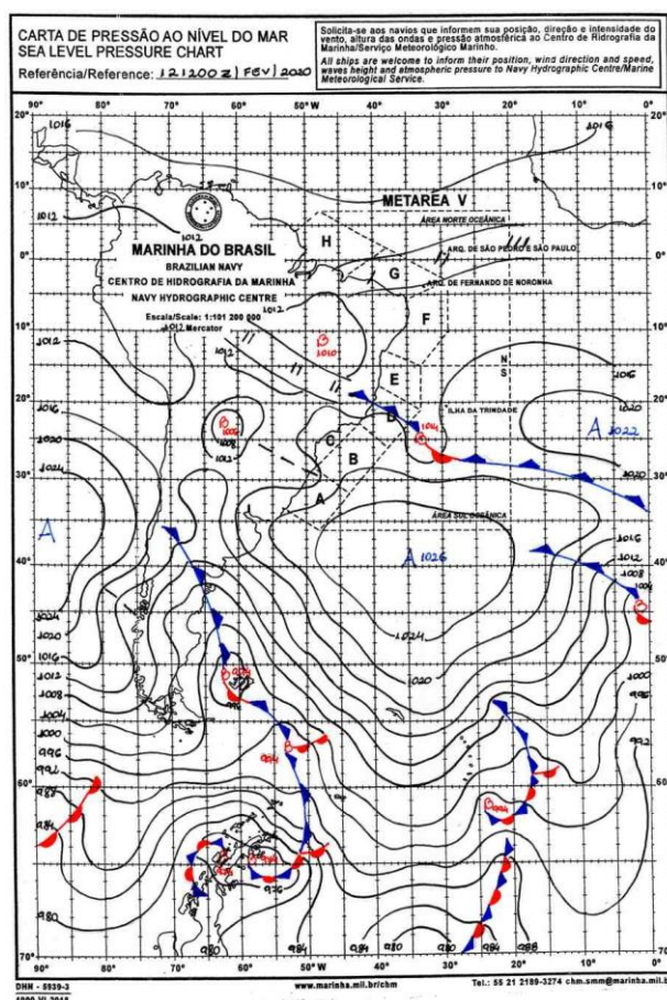
Figura 7 - Carta Sinótica do Dia 12/02/2020. Fonte: Marinha Brasileira.
