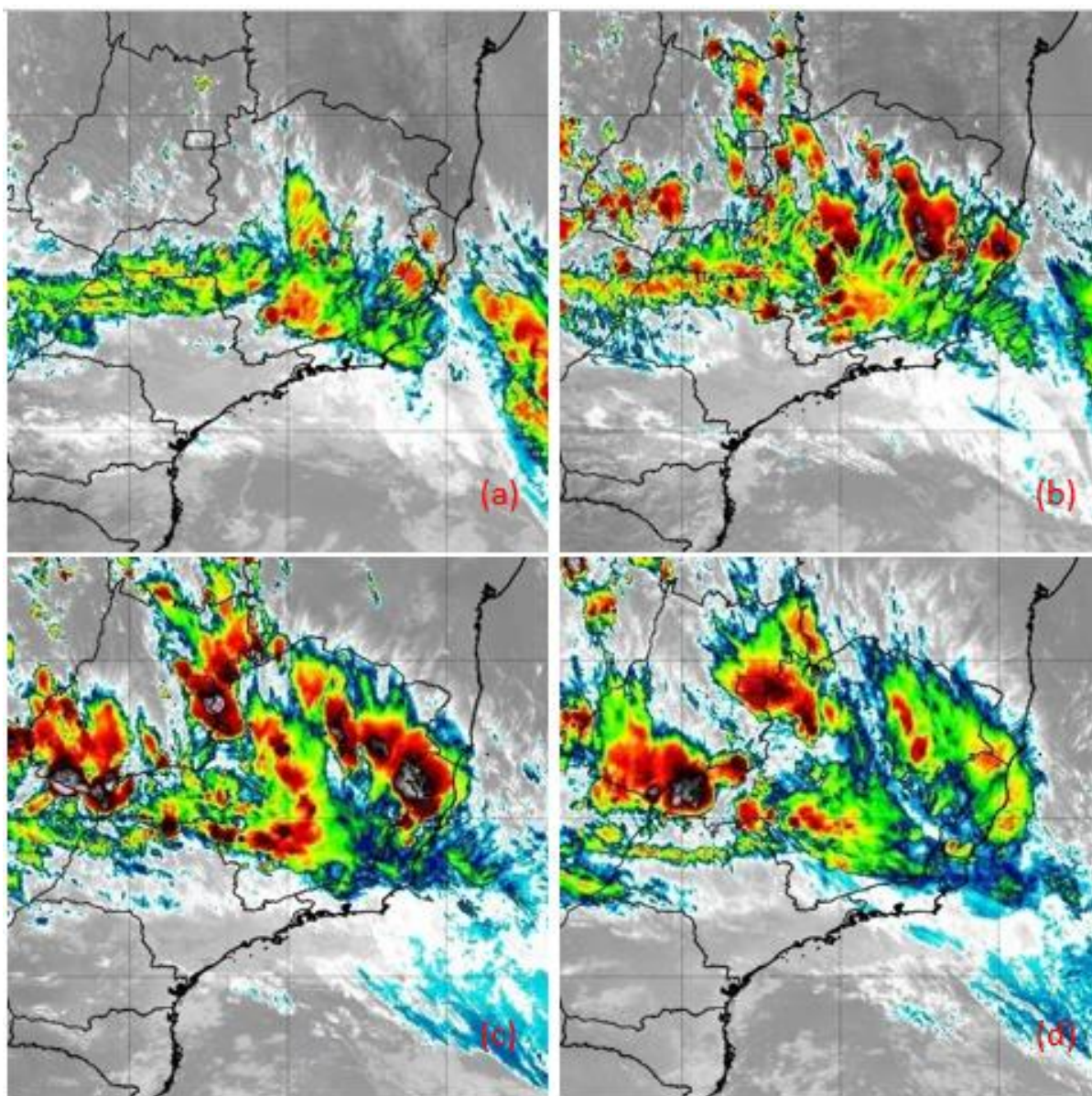
Figura 3 - Imagens do satélite GOES-16 do dia 11/02/2020 as 12:00 (a), 15:00 (b), 18:00 (c) e 21:00 horas local. Fonte: INPE.
