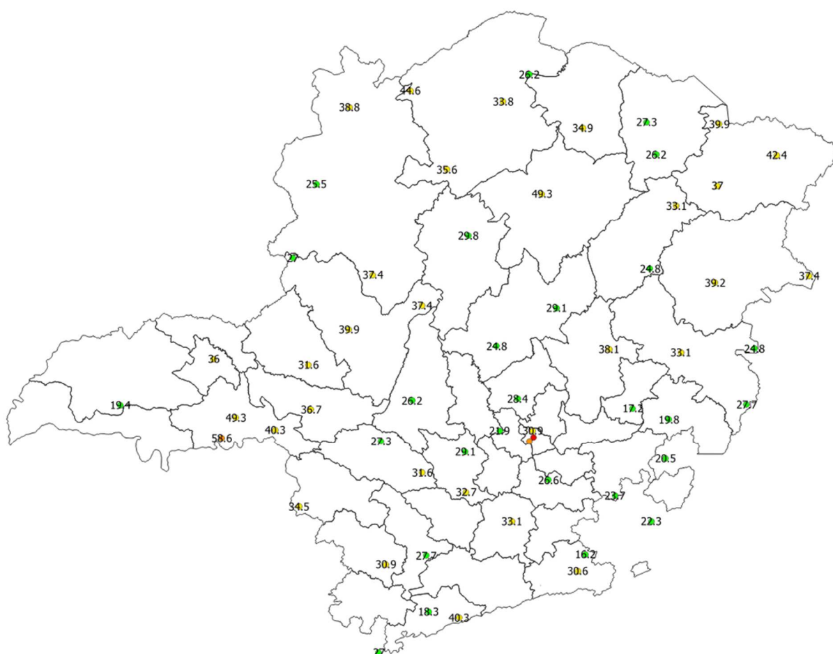
Figura 15 - Rajadas de vento registradas no dia 18/01/2020. Fonte: INMET.
