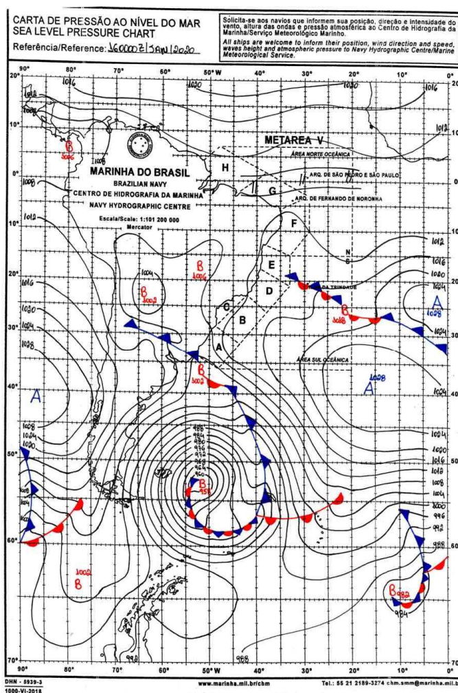
Figura 2 - Carta Sinótica do Dia 16/01/2020. Fonte: Marinha Brasileira.
