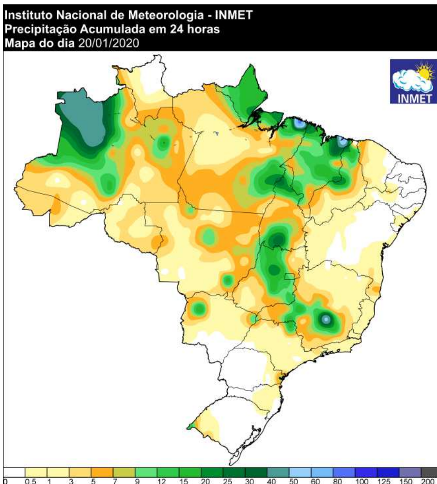
Figura 21 - Precipitação ocorrida no dia 19/01/2020. Fonte: INMET.
