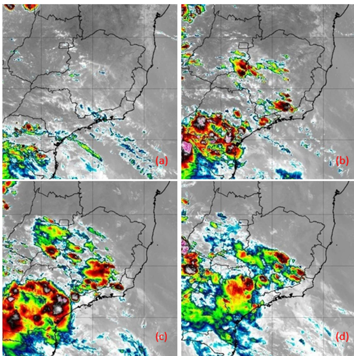
Figura 3 - Imagens do satélite GOES-16 do dia 16/01/2020 as 12:00 (a), 15:00 (b), 18:00 (c) e 21:00 horas local. Fonte: INPE.
