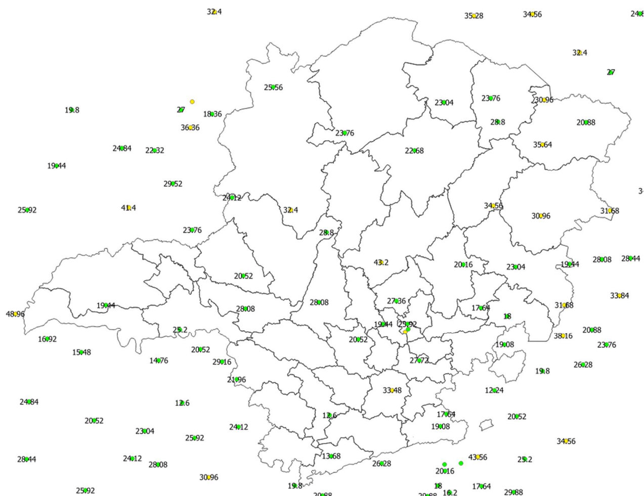
Figura 20 - Rajadas de vento registradas no dia 19/01/2020. Fonte: INMET.
