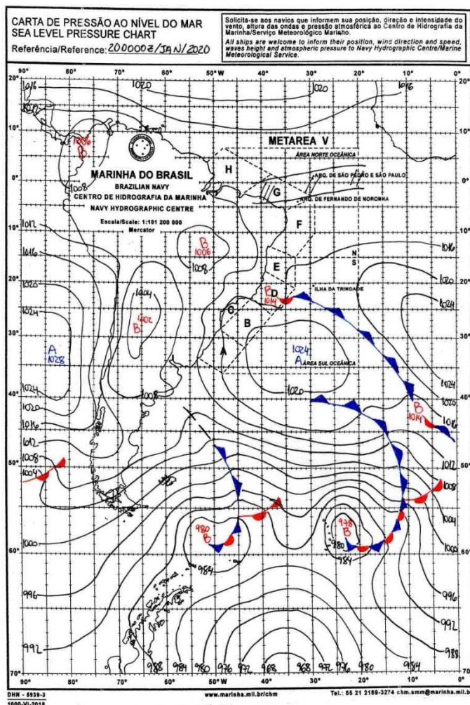
Figura 22 - Carta Sinótica do Dia 20/01/2020. Fonte: Marinha Brasileira.
