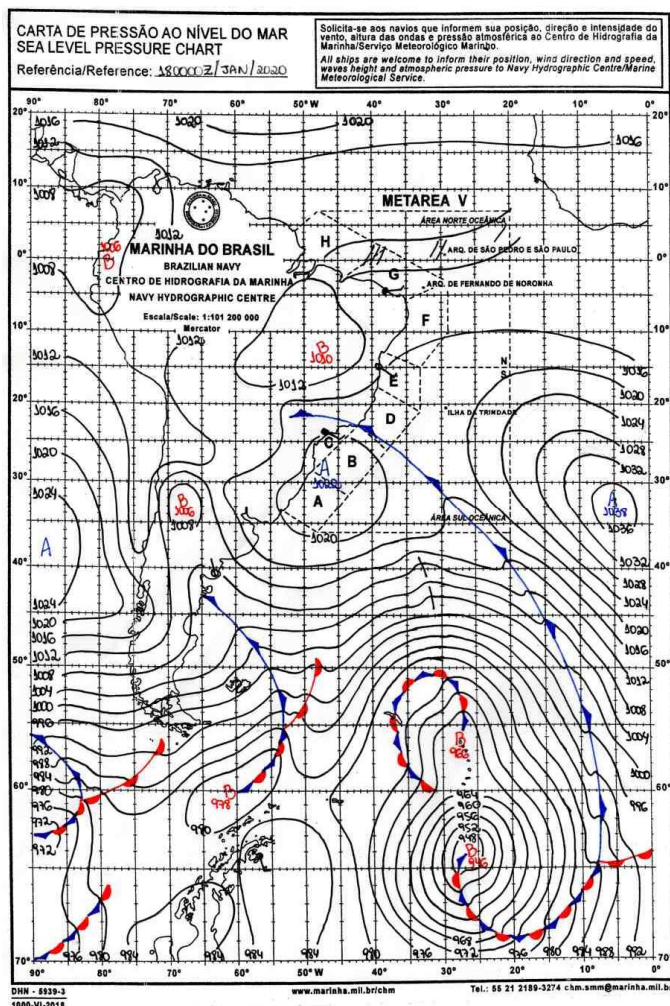
Figura 12 - Carta Sinótica do Dia 18/01/2020. Fonte: Marinha Brasileira.
