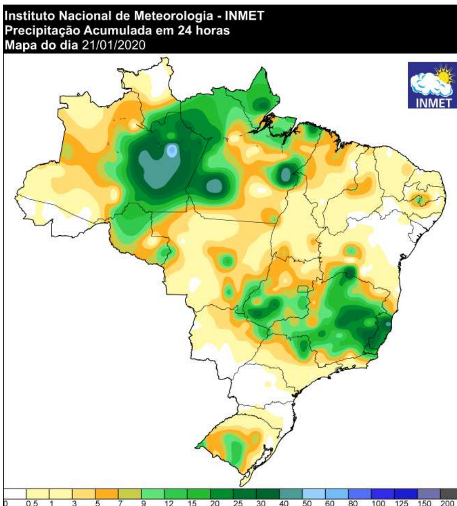
Figura 26 - Precipitação ocorrida no dia 20/01/2020. Fonte: INMET.
