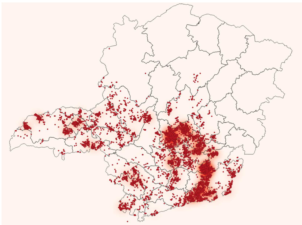
Figura 4 - Raios registrados no dia 16/01/2020. Fonte: RINDAT.
