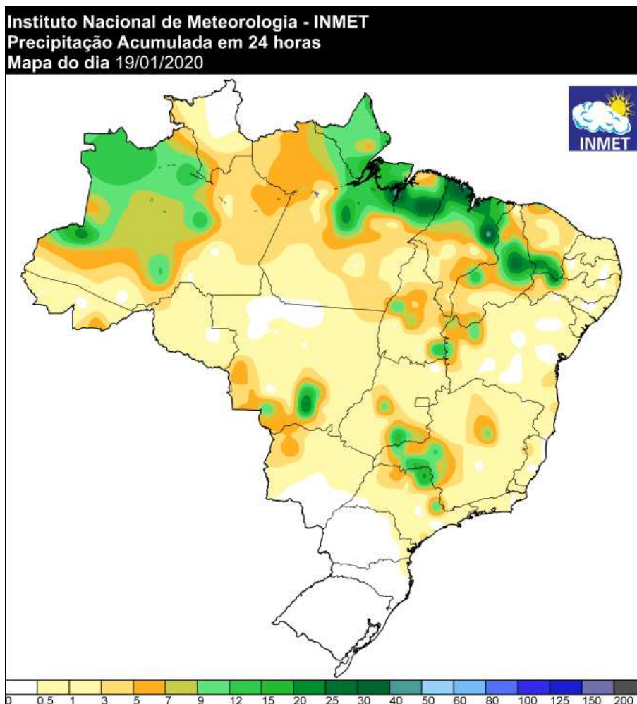
Figura 16 - Precipitação ocorrida no dia 18/01/2020. Fonte: INMET.
