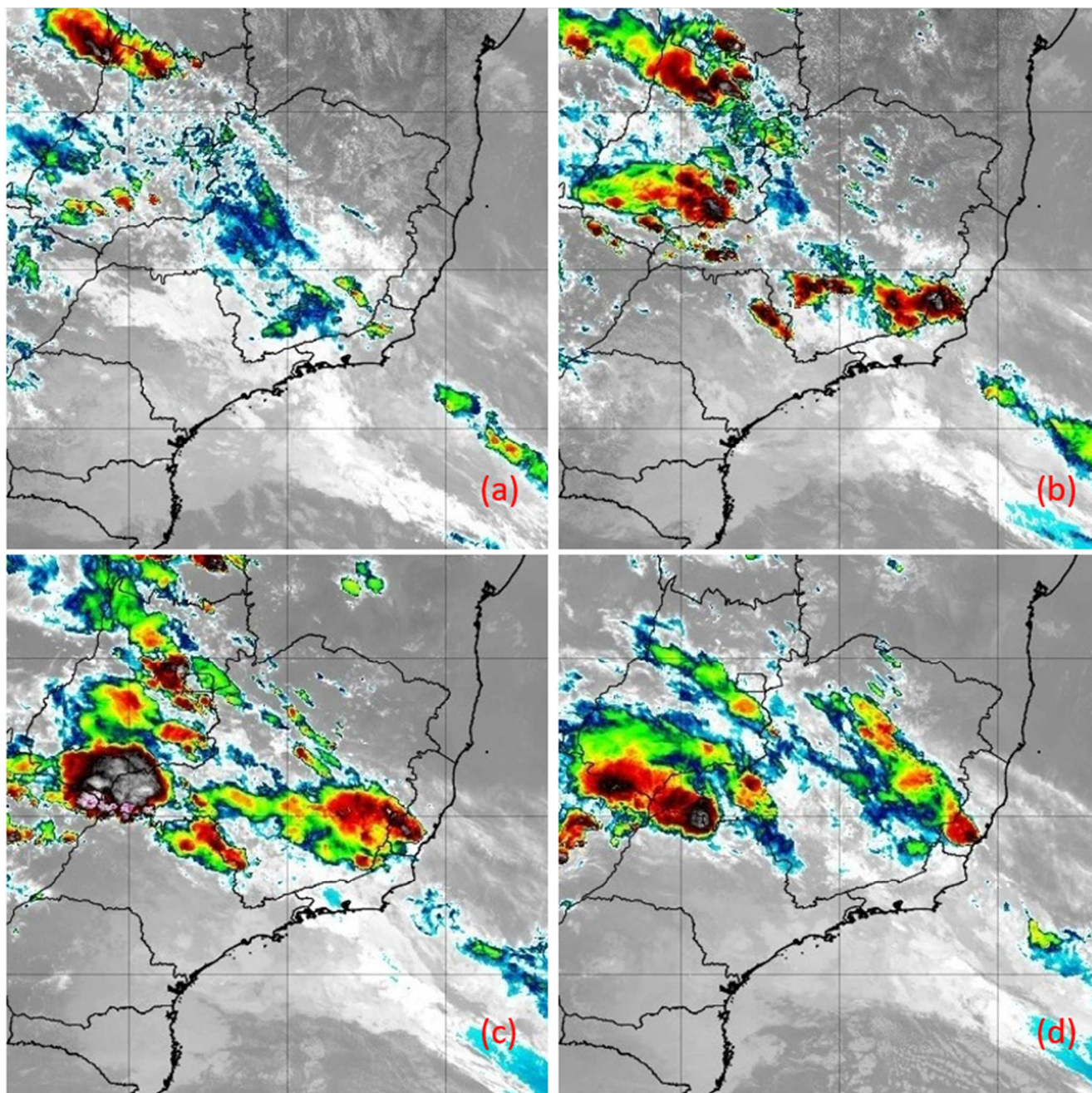
Figura 8 - Imagens do satélite GOES-16 do dia 17/01/2020 as 12:00 (a), 15:00 (b), 18:00 (c) e 21:00 horas local. Fonte: INPE.
