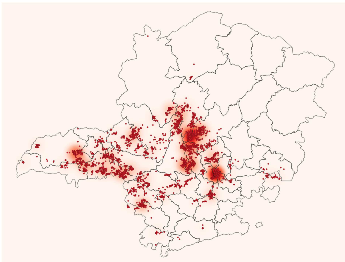
Figura 19 - Raios registrados no dia 19/01/2020. Fonte: RINDAT.
