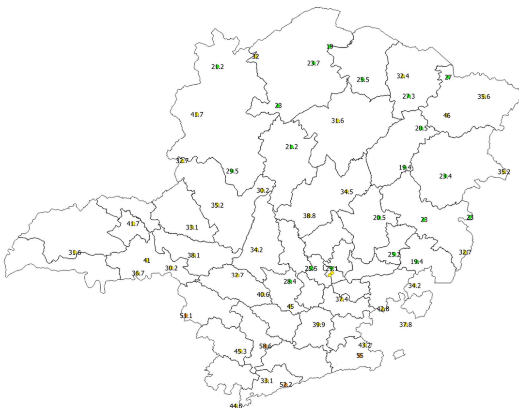
Figura 5 - Rajadas de vento registradas no dia 16/01/2020. Fonte: INMET.
