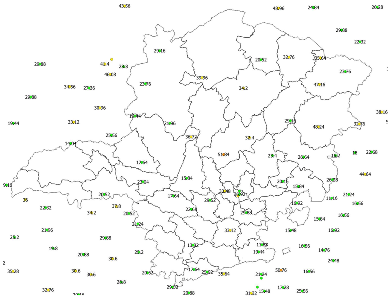
Figura 30 - Rajadas de vento registradas no dia 21/01/2020. Fonte: INMET.
