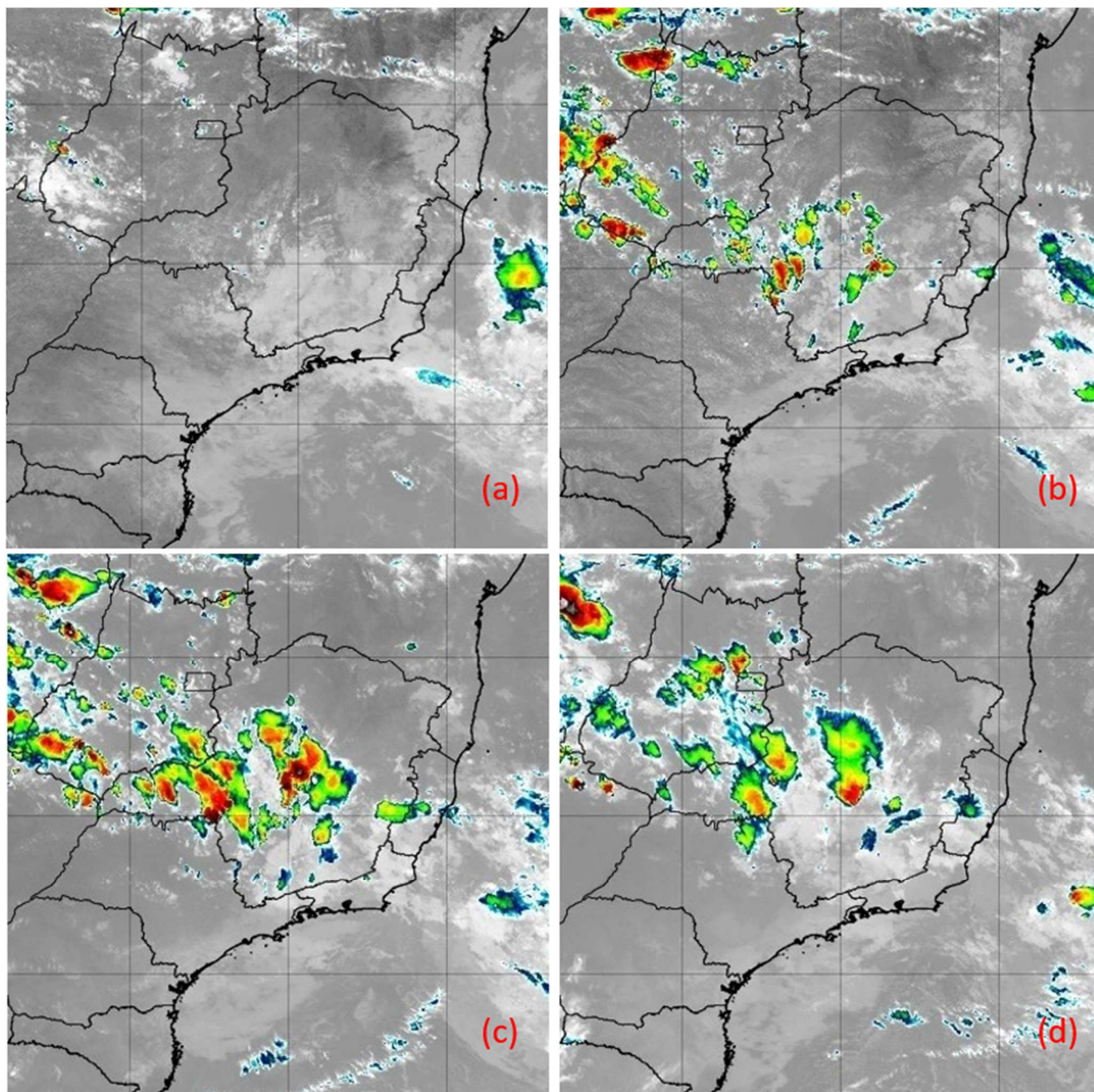
Figura 18 - Imagens do satélite GOES-16 do dia 19/01/2020 as 12:00 (a), 15:00 (b), 18:00 (c) e 21:00 horas local. Fonte: INPE.
