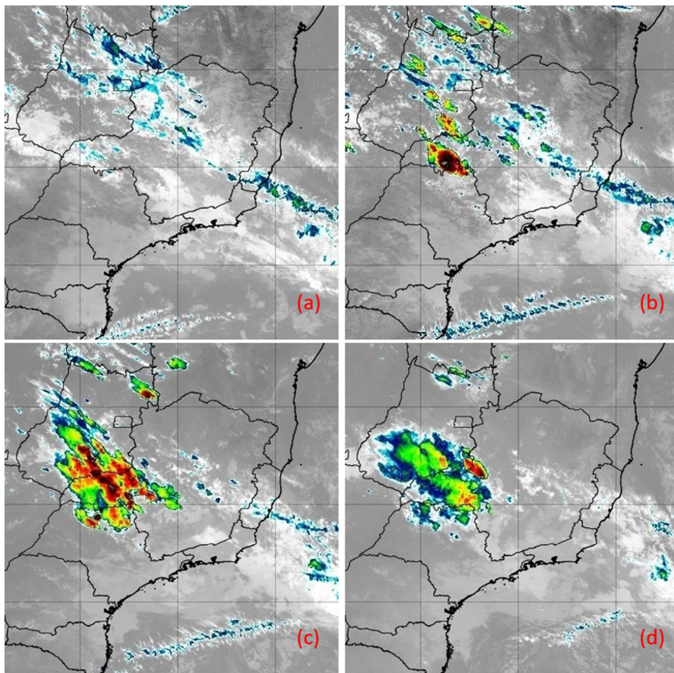
Figura 13 encontra-se as imagens de satélite do dia 18/01, onde pode-se ver o desenvolvimento de núcleos convectivos, sobretudo no Triângulo Mineiro, mas também em partes do centro e norte do estado.
