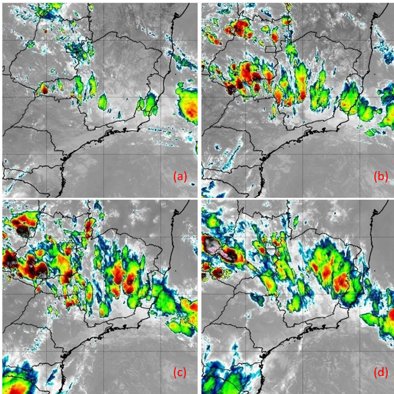
Figura 23 - Imagens do satélite GOES-16 do dia 20/01/2020 as 12:00 (a), 15:00 (b), 18:00 (c) e 21:00 horas local. Fonte: INPE.
