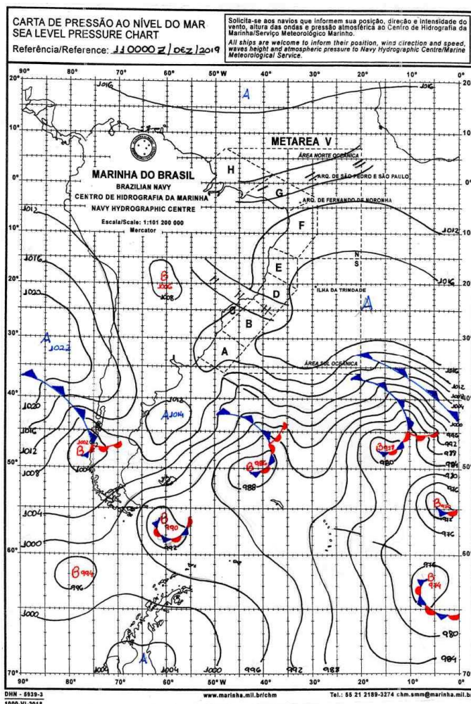
Figura 277 - Carta Sinótica do Dia 21/01/2020. Fonte: Marinha Brasileira.
