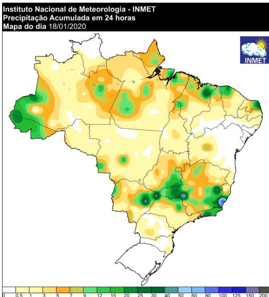
Figura 11 - Precipitação ocorrida no dia 17/01/2020. Fonte: INMET.
