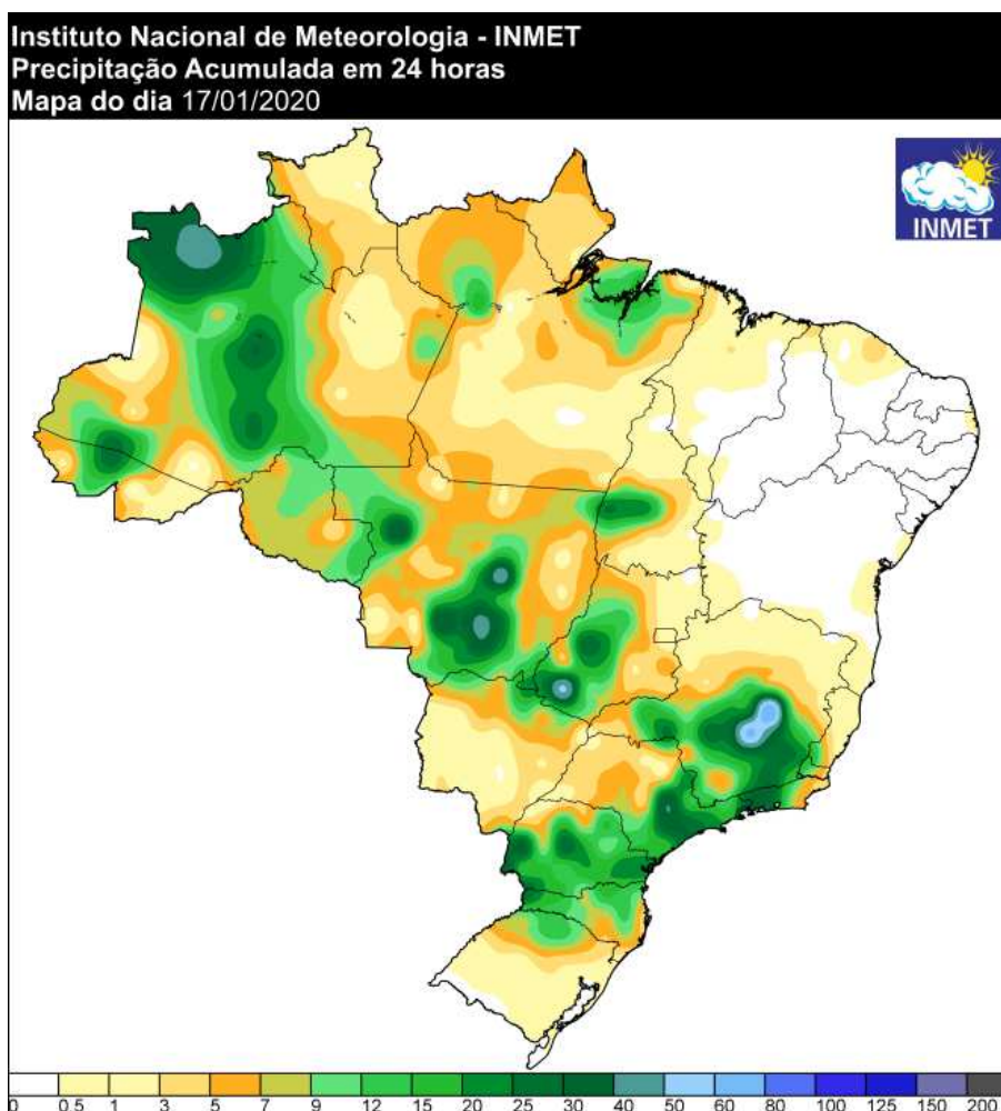
Figura 6 - Precipitação ocorrida no dia 16/01/2020. Fonte: INMET.
