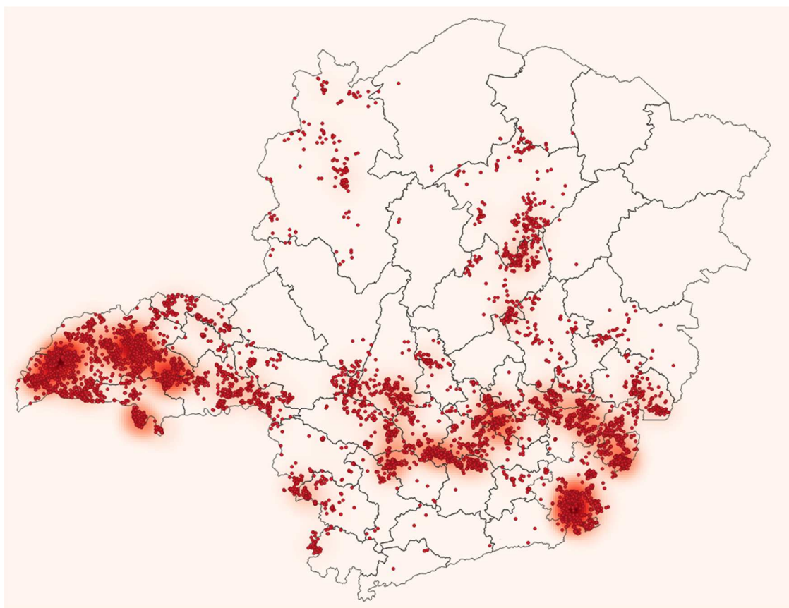
Figura 9 - Raios registrados no dia 17/01/2020. Fonte: RINDAT.
