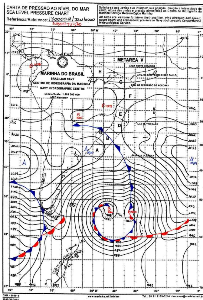
Figura 7 - Carta Sinótica do Dia 17/01/2020. Fonte: Marinha Brasileira.
