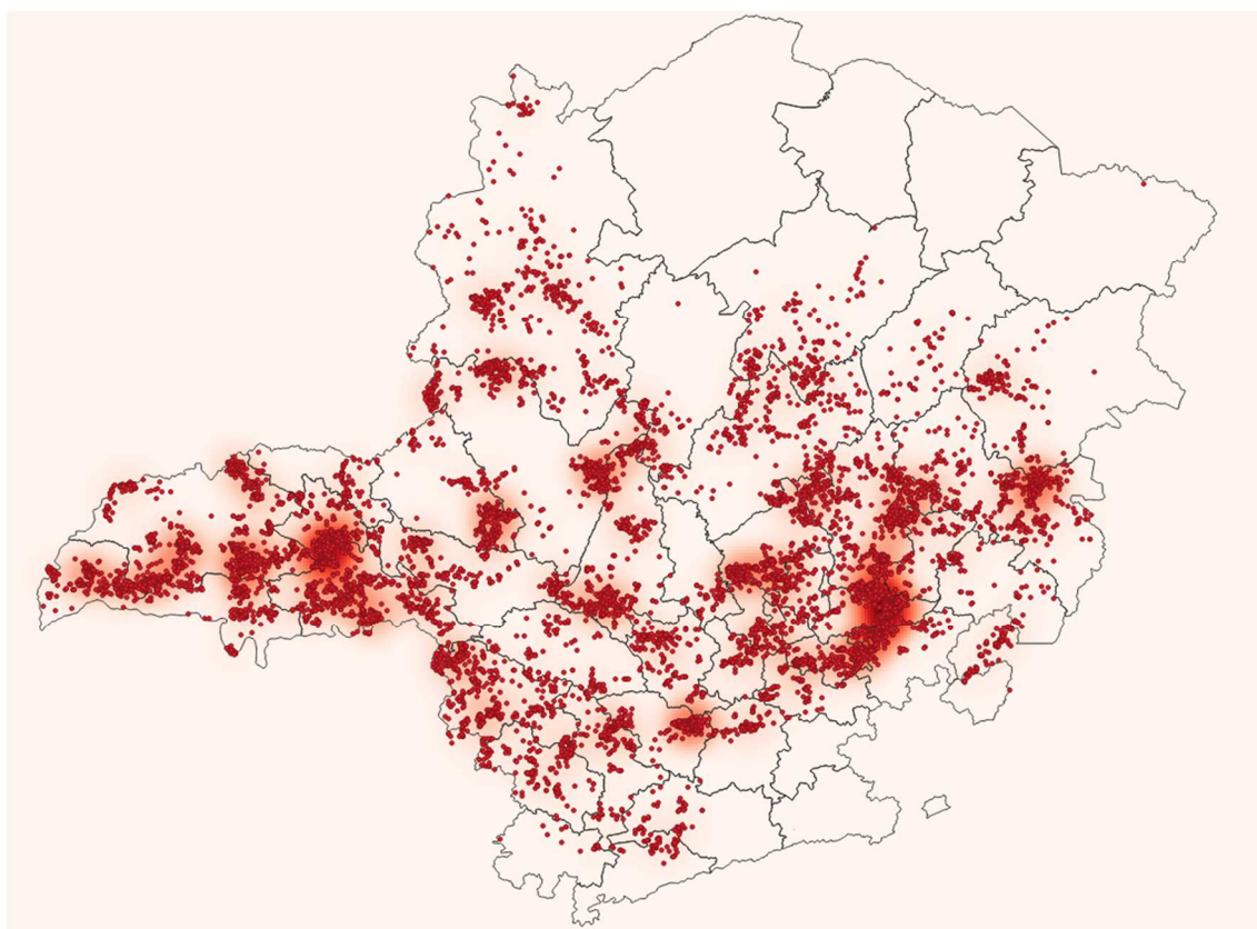
Figura 24 - Raios registrados no dia 20/01/2020. Fonte: RINDAT.
