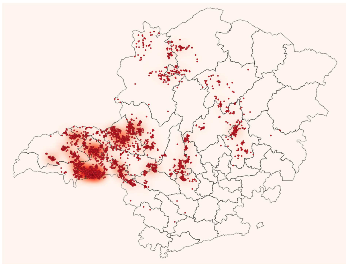
Figura 14 - Raios registrados no dia 18/01/2020. Fonte: RINDAT.
