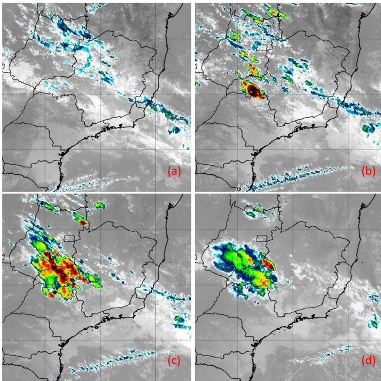
Figura 13 - Imagens do satélite GOES-16 do dia 18/01/2020 as 12:00 (a), 15:00 (b), 18:00 (c) e 21:00 horas local. Fonte: INPE.
