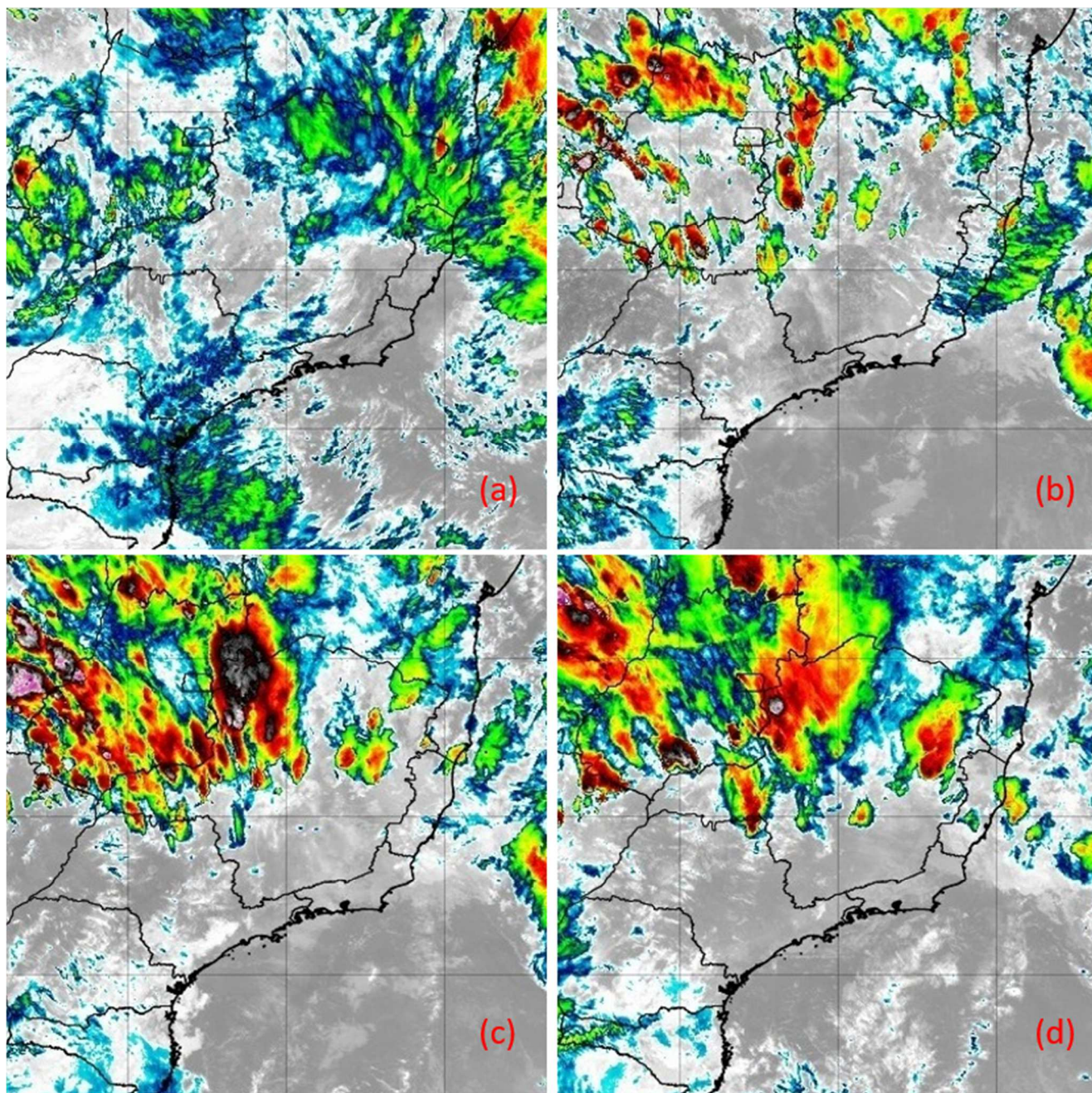
Figura 288 - Imagens do satélite GOES-16 do dia 21/01/2020 as 12:00 (a), 15:00 (b), 18:00 (c) e 21:00 horas local. Fonte: INPE.
