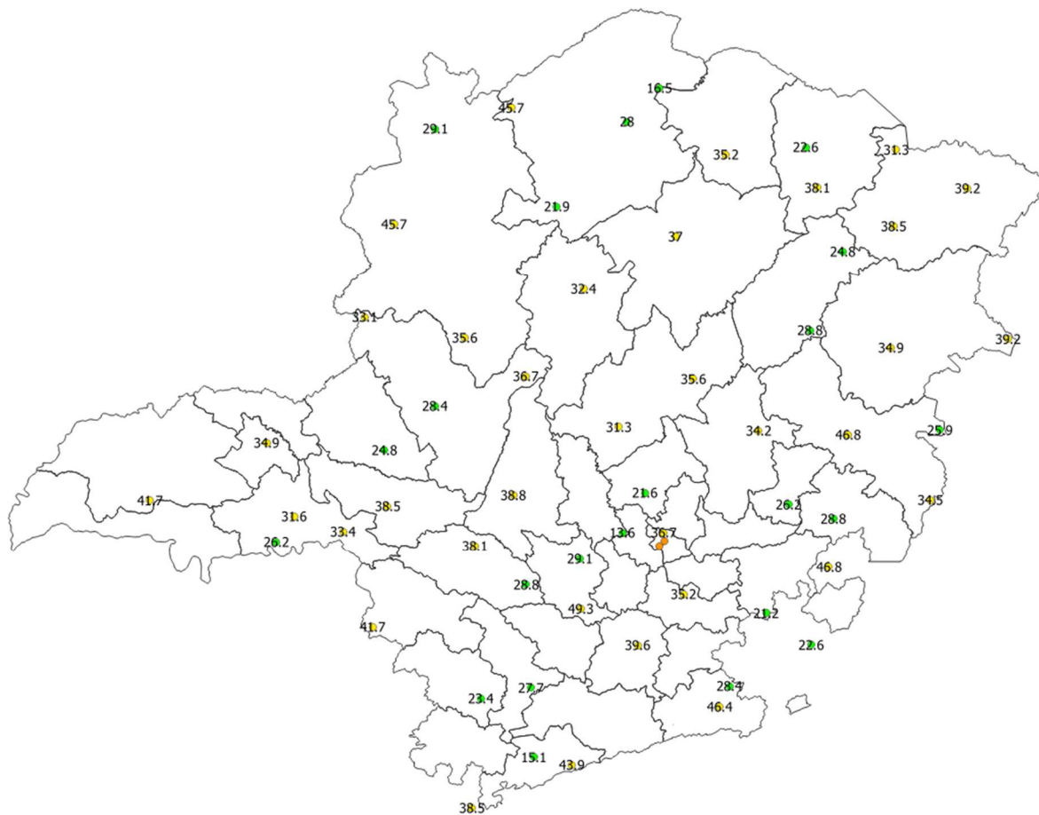
Figura 10 - Rajadas de vento registradas no dia 17/01/2020. Fonte: INMET.
