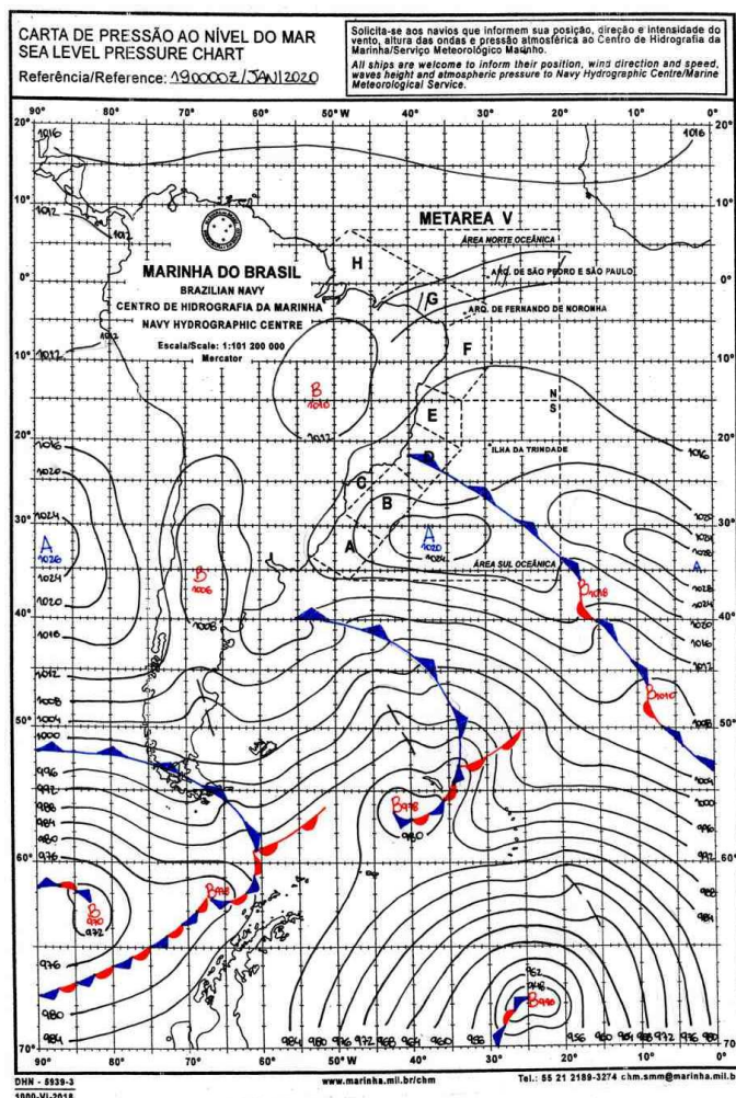
Figura 17 - Carta Sinótica do Dia 19/01/2020. Fonte: Marinha Brasileira.
