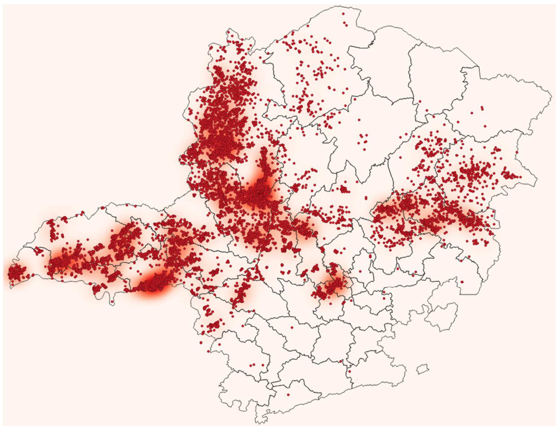
Figura 299 - Raios registrados no dia 21/01/2020. Fonte: RINDAT.
