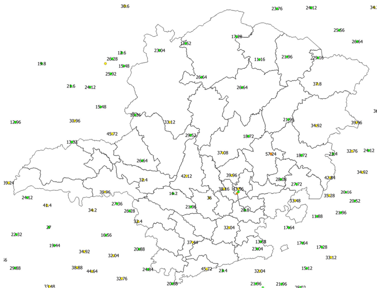
Figura 25 - Rajadas de vento registradas no dia 20/01/2020. Fonte: INMET.
