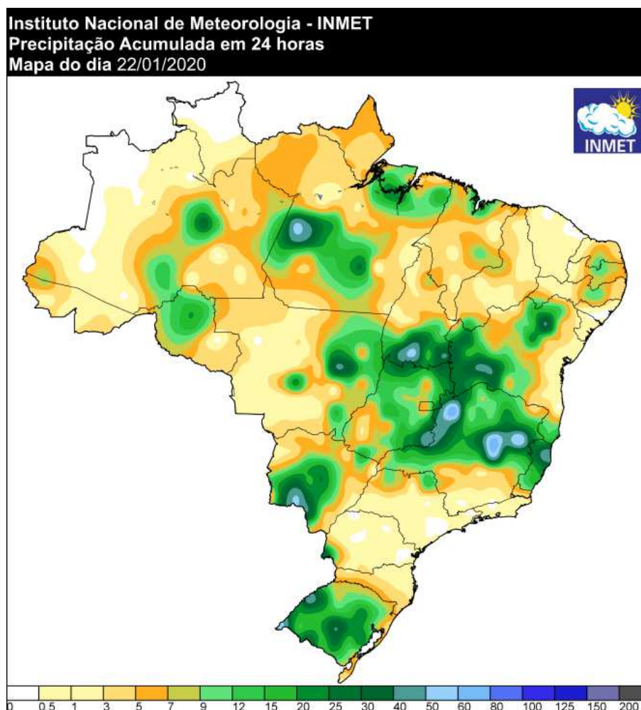
Figura 31 - Precipitação ocorrida no dia 21/01/2020. Fonte: INMET.
