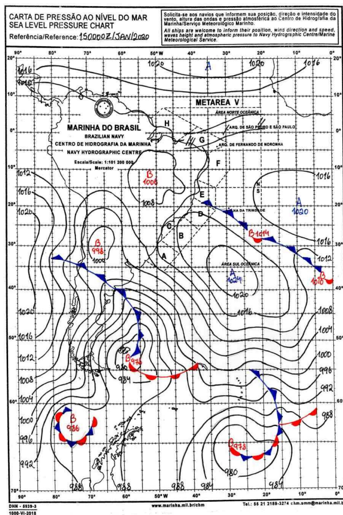
Figura 1 - Carta sinótica do dia 15/01/2020. Fonte: Marinha Brasileira.
