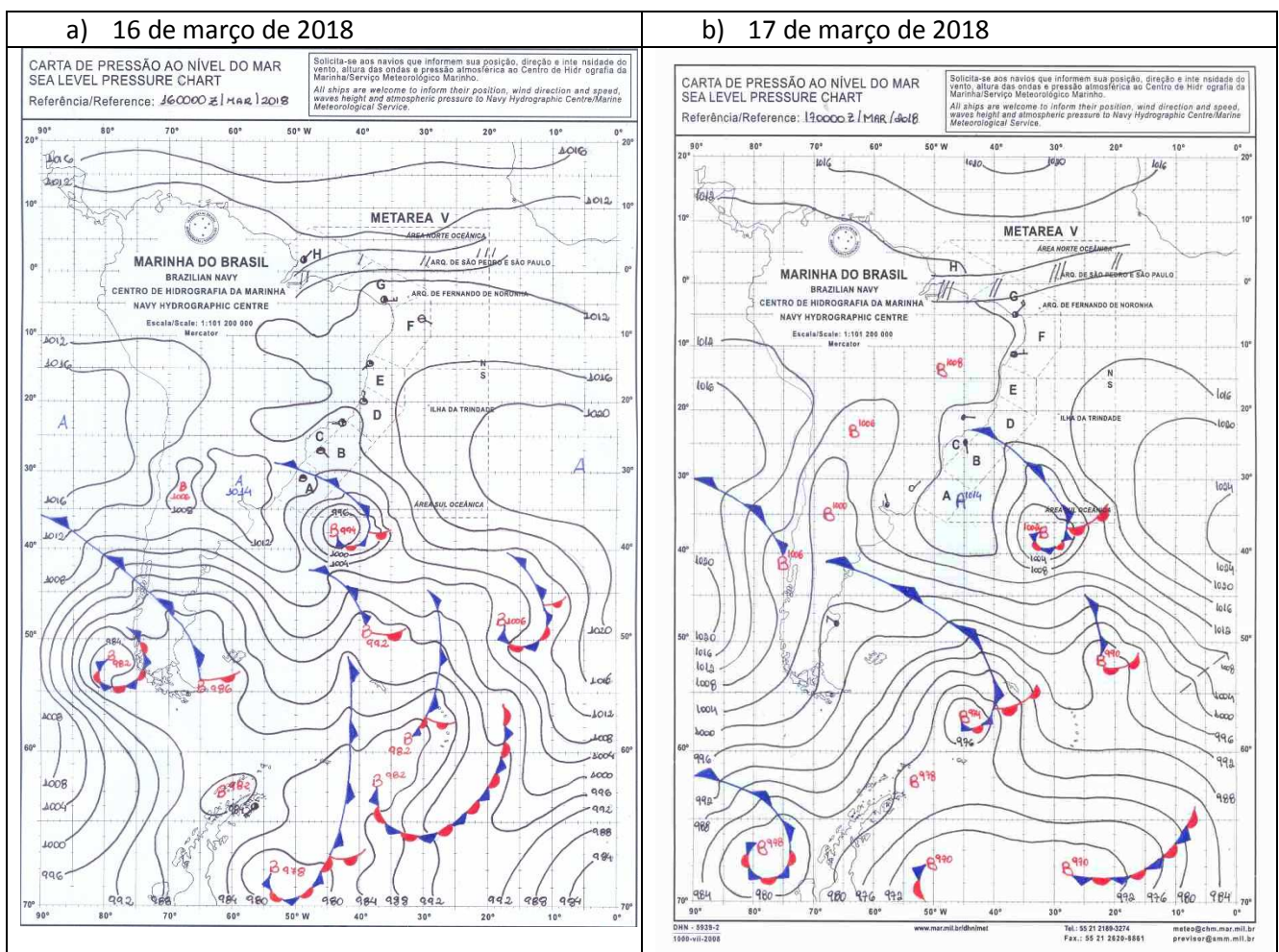
Figura 1 - Cartas Sinóticas elaboradas pela Marinha do Brasil para os dias 16 e 17 de março de 2018.
