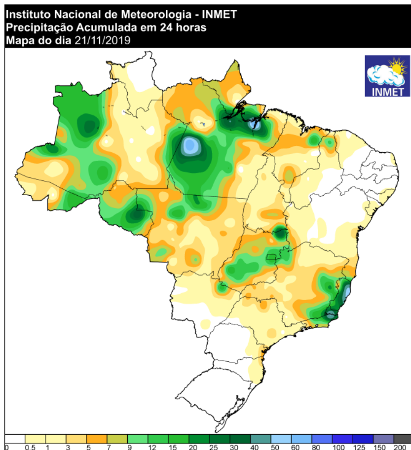
Figura 16 - Precipitação ocorrida no dia 20/11/2019. Fonte: INMET.
