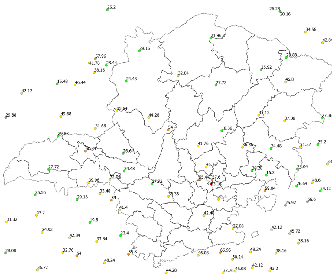
Figura 30 - Rajadas de vento registradas no dia 23/11/2019. Fonte: INMET.
