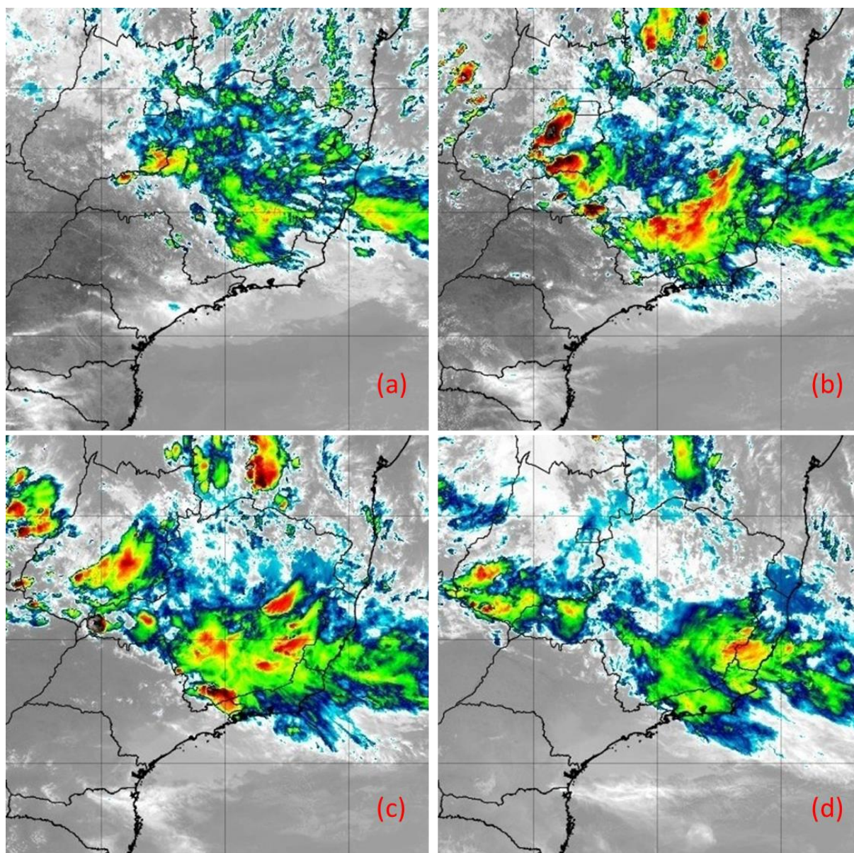
Figura 3 - Imagens do satélite GOES-16 do dia 18/11/2019 as 12:00 (a), 15:00 (b), 18:00 (c) e 21:00 horas local. Fonte: INPE.
