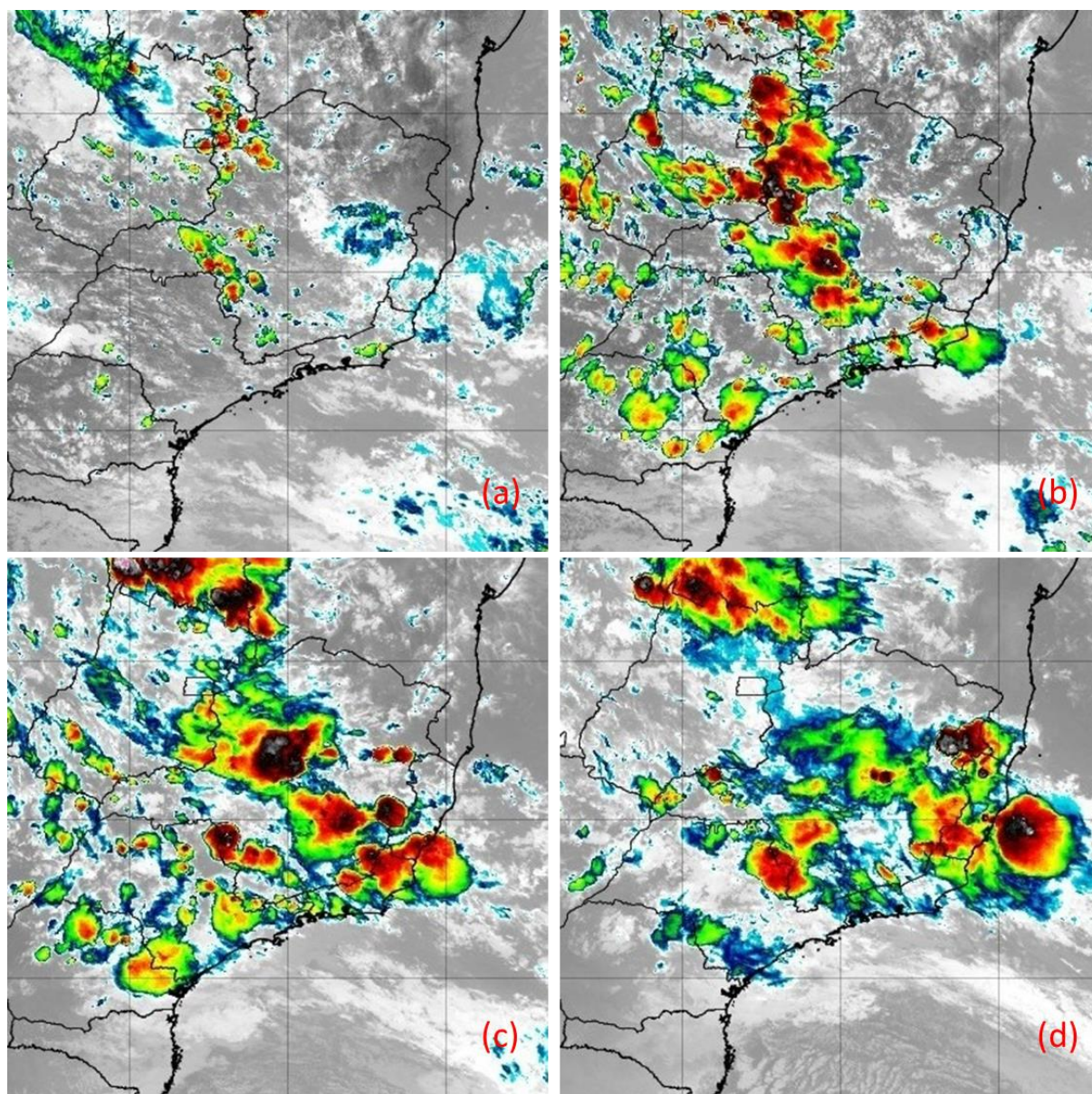
Figura 28 - Imagens do satélite GOES-16 do dia 23/11/2019 as 12:00 (a), 15:00 (b), 18:00 (c) e 21:00 horas local. Fonte: INPE.
