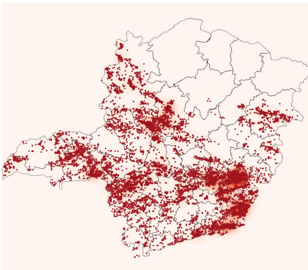
Figura 29 - Raios registrados no dia 23/11/2019. Fonte: RINDAT.
