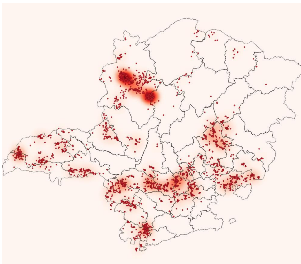
Figura 4 - Raios registrados no dia 18/11/2019. Fonte: RINDAT.
