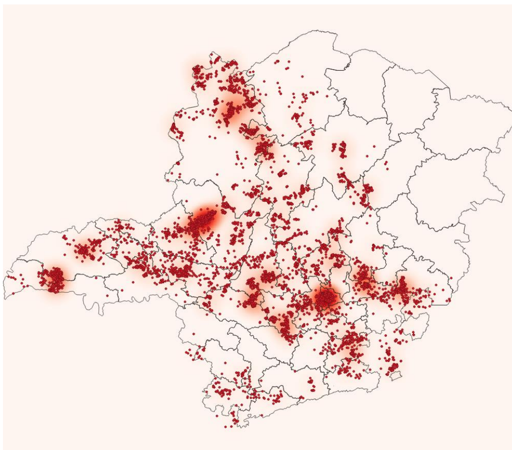
Figura 9 - Raios registrados no dia 19/11/2019. Fonte: RINDAT.
