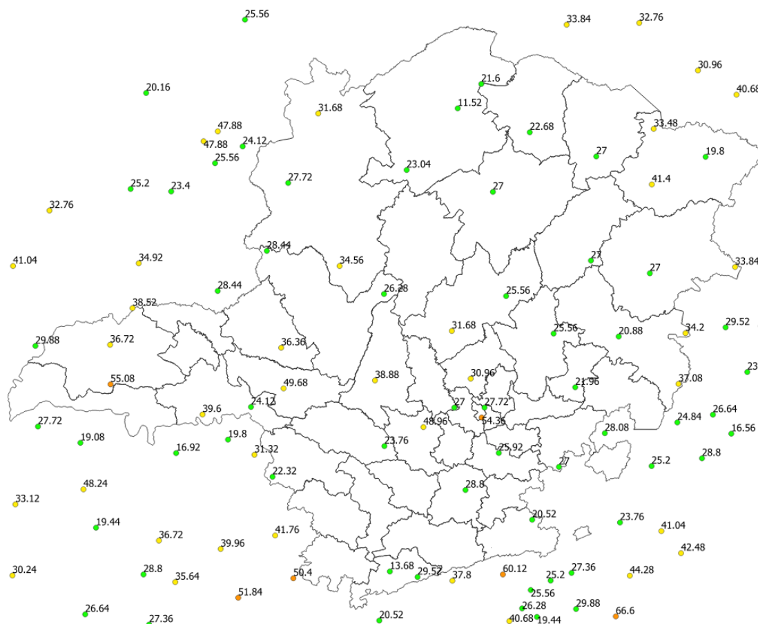
Figura 25 - Rajadas de vento registradas no dia 22/11/2019. Fonte: INMET.
