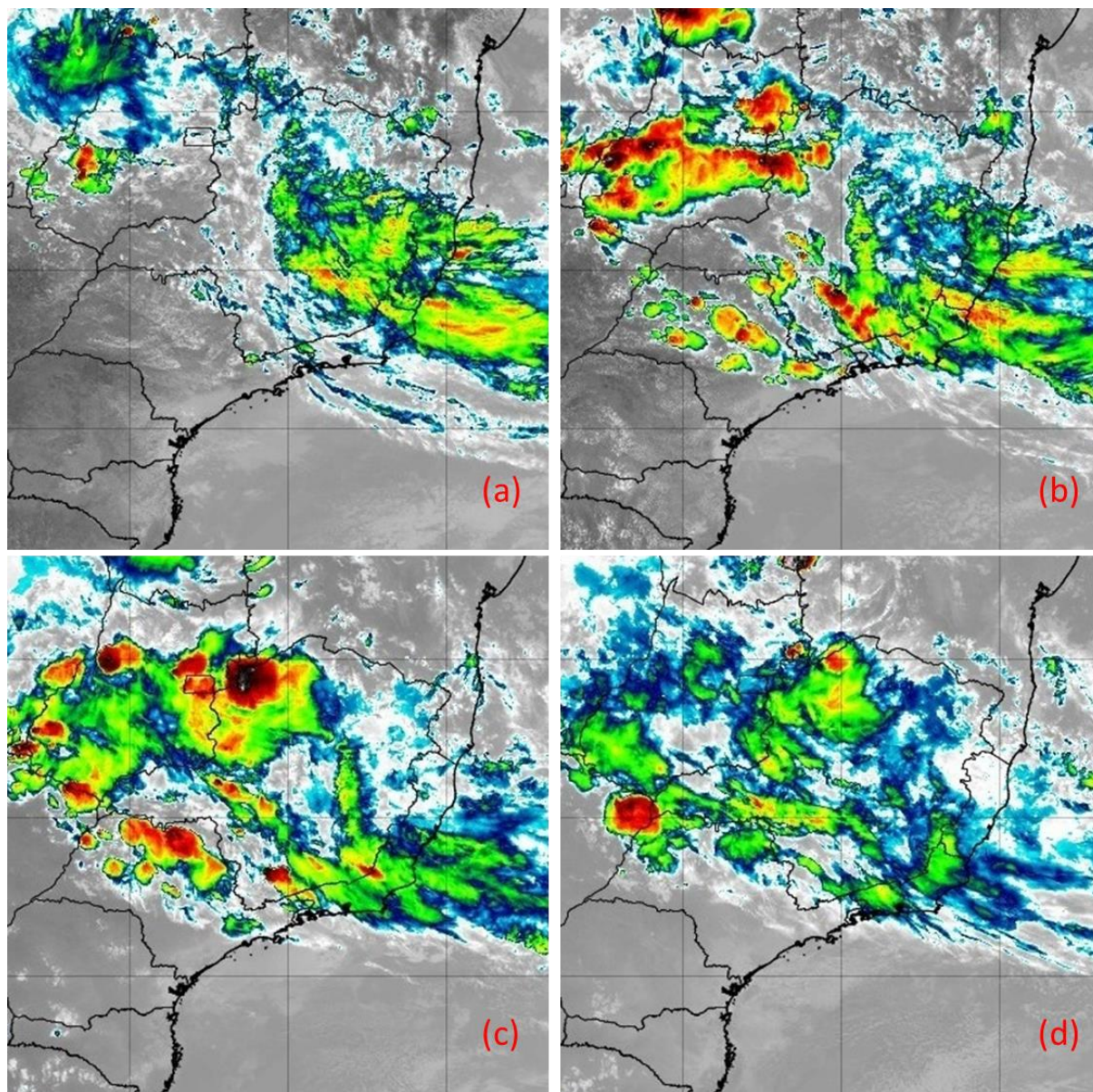
Figura 13 - Imagens do satélite GOES-16 do dia 20/11/2019 as 12:00 (a), 15:00 (b), 18:00 (c) e 21:00 horas local. Fonte: INPE.
