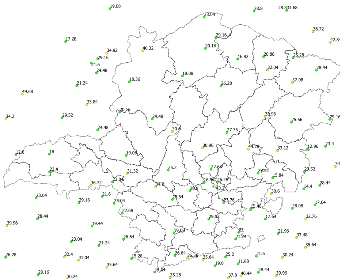
Figura 15 - Rajadas de vento registradas no dia 20/11/2019. Fonte: INMET.
