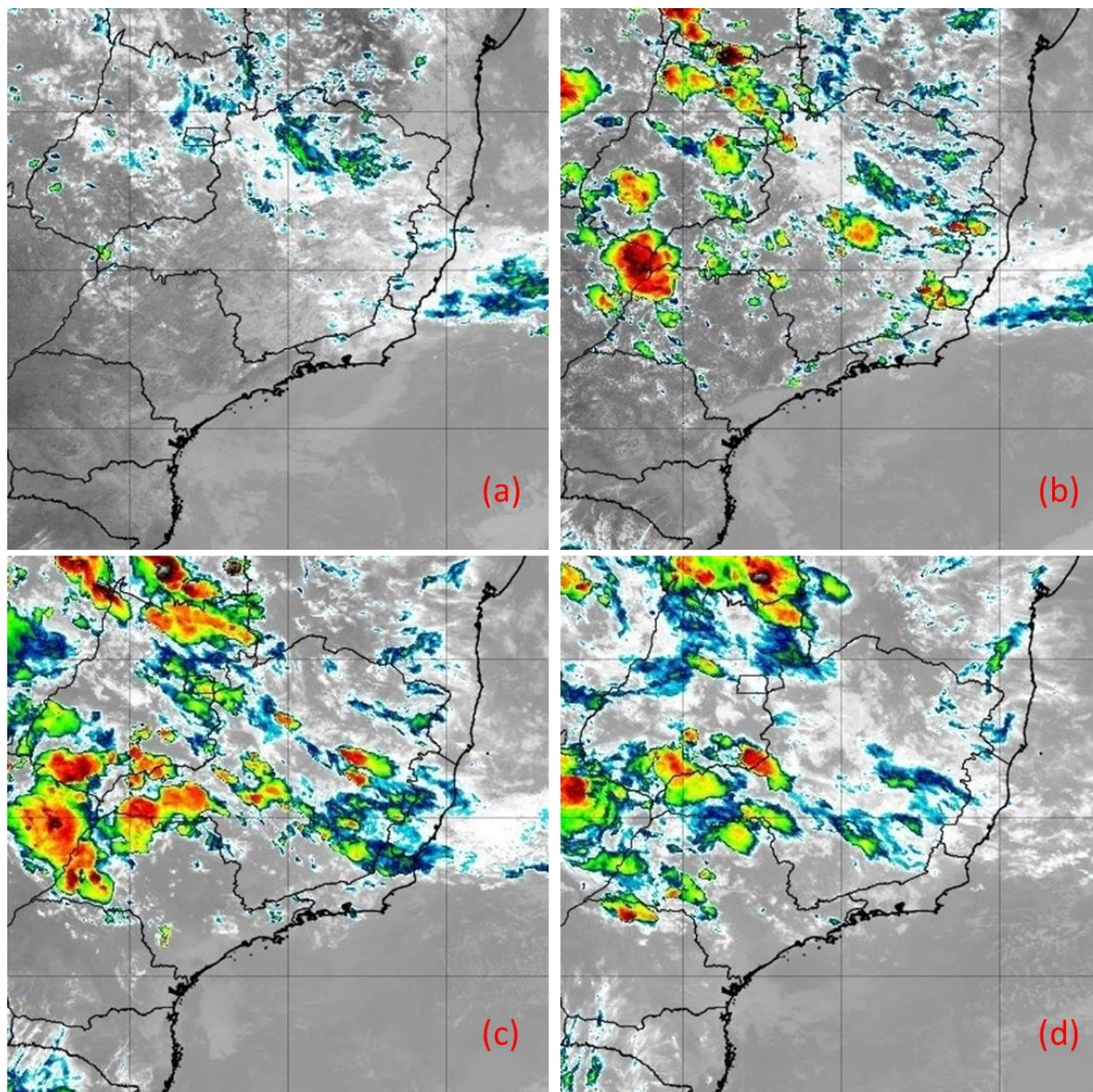
Figura 18 - Imagens do satélite GOES-16 do dia 21/11/2019 as 12:00 (a), 15:00 (b), 18:00 (c) e 21:00 horas local. Fonte: INPE.
