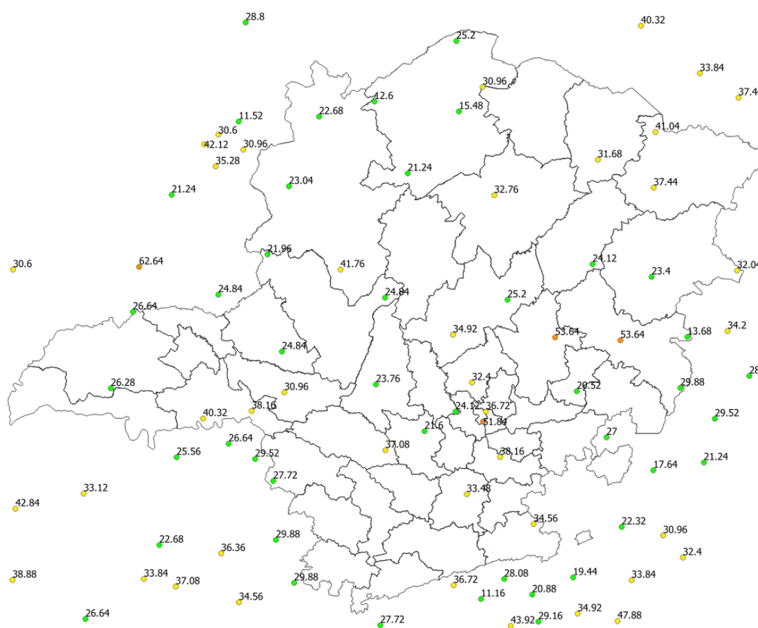
Figura 20 - Rajadas de vento registradas no dia 21/11/2019. Fonte: INMET.
