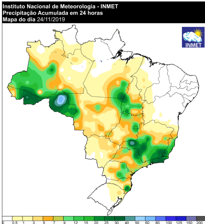
Figura 31 - Precipitação ocorrida no dia 23/11/2019. Fonte: INMET.
