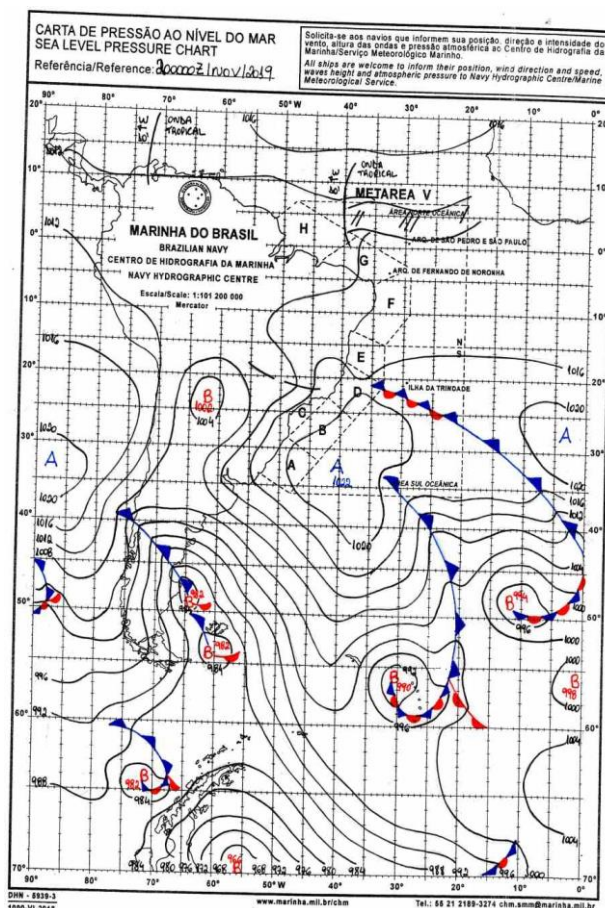
Figura 12 - Carta Sinótica do Dia 20/11/2019. Fonte: Marinha Brasileira.
