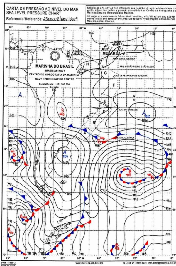
Figura 27 - Carta Sinótica do Dia 23/11/2019. Fonte: Marinha Brasileira.
