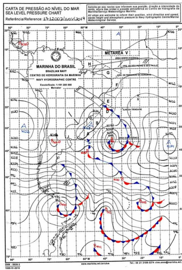
Figura 1 - Carta Sinótica do Dia 17/11/2019. Fonte: Marinha Brasileira.
