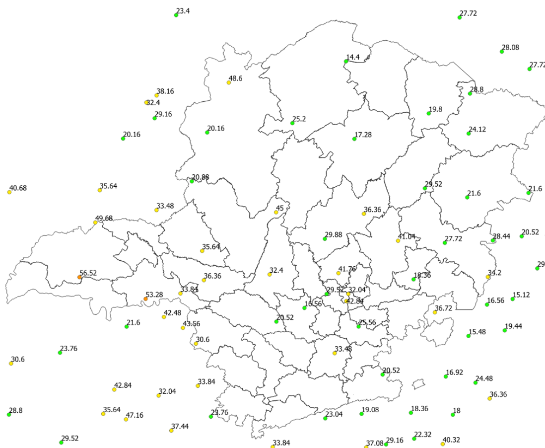
Figura 5 - Rajadas de vento registradas no dia 18/11/2019. Fonte: INMET.
