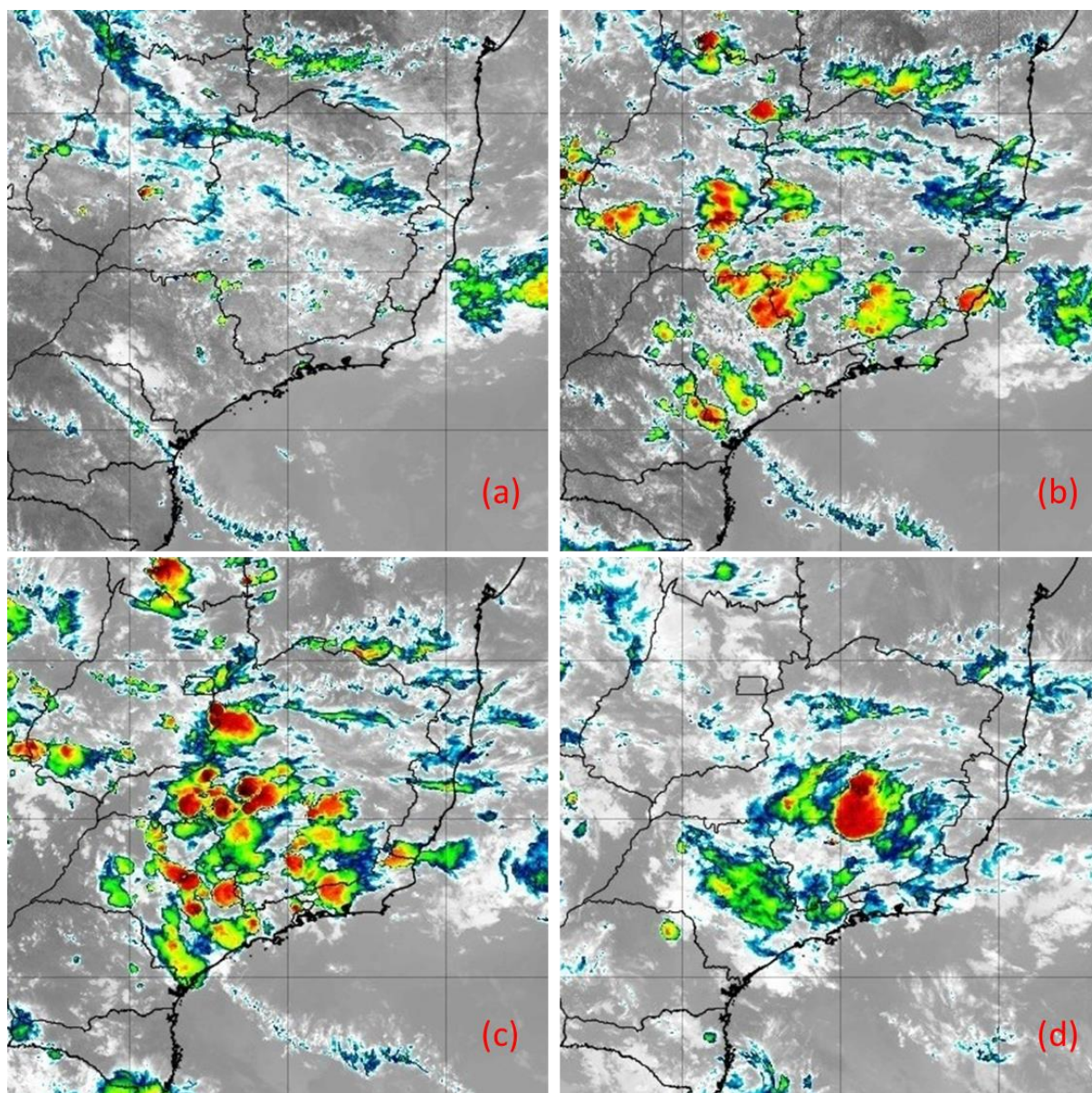
Figura 23 - Imagens do satélite GOES-16 do dia 22/11/2019 as 12:00 (a), 15:00 (b), 17:30 (c) e 21:00 horas local. Fonte: INPE.
