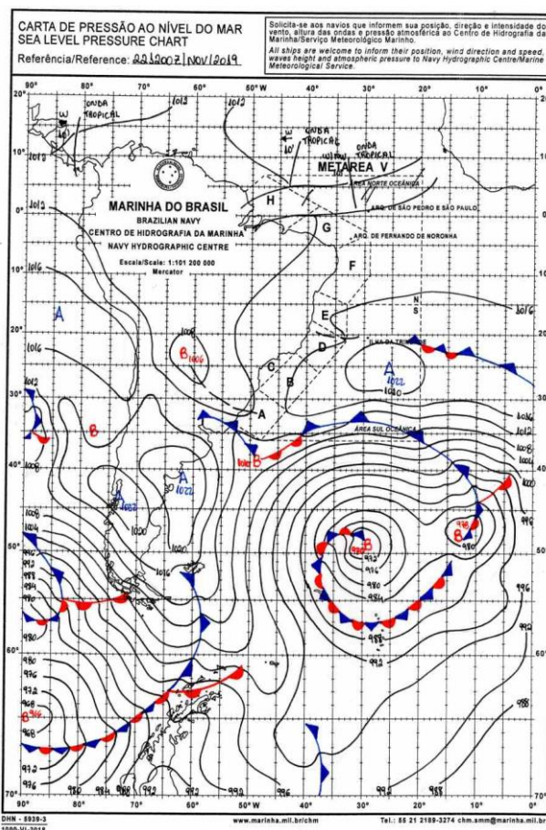
Figura 22 - Carta Sinótica do Dia 22/11/2019. Fonte: Marinha Brasileira.
