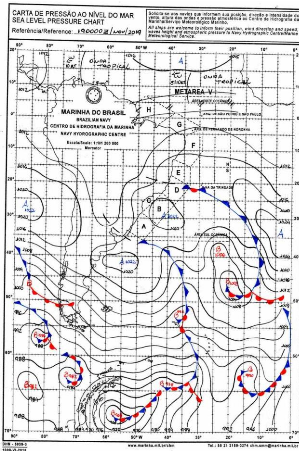
Figura 7 - Carta Sinótica do Dia 19/11/2019. Fonte: Marinha Brasileira.
