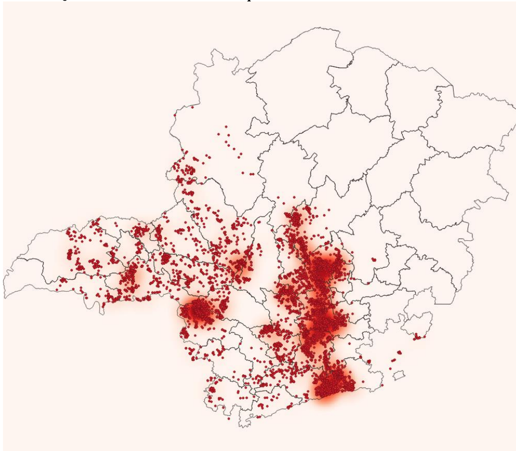
Figura 24 - Raios registrados no dia 22/11/2019. Fonte: RINDAT.
