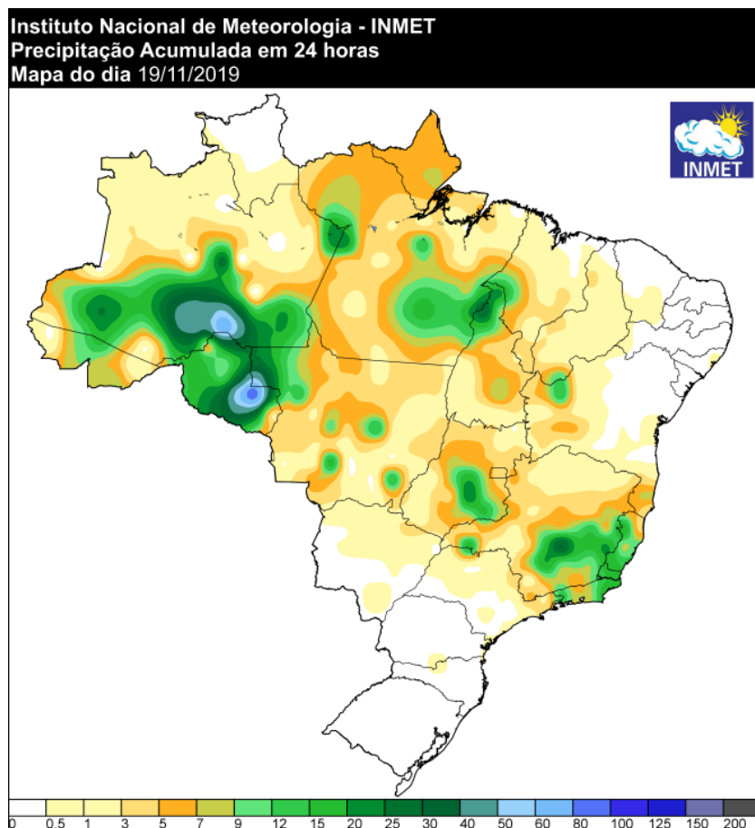
Figura 6 - Precipitação ocorrida no dia 18/11/2019. Fonte: INMET.
