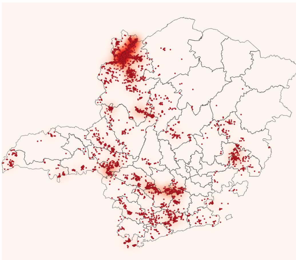
Figura 14 - Raios registrados no dia 20/11/2019. Fonte: RINDAT.
