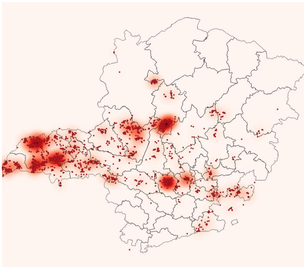
Figura 19 - Raios registrados no dia 21/11/2019. Fonte: RINDAT.
