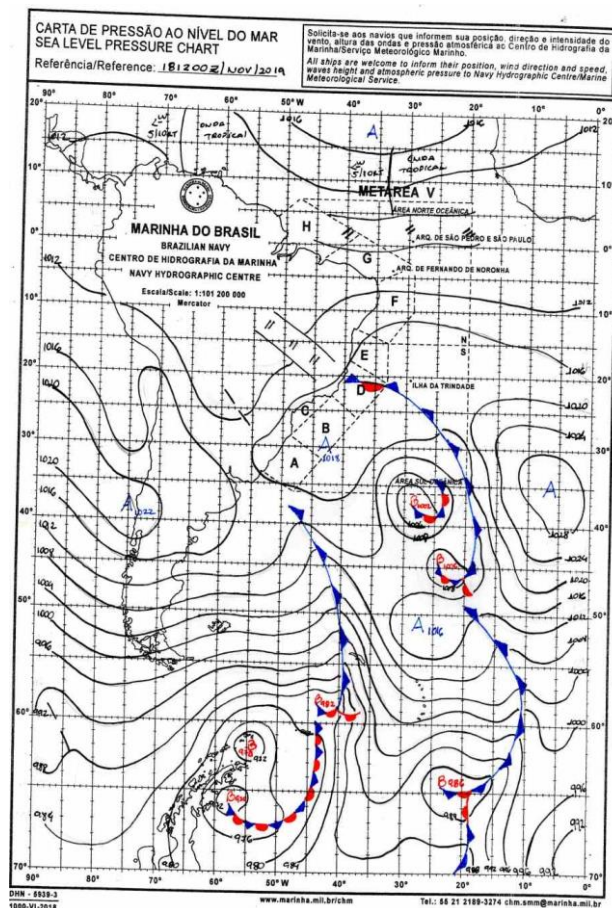
Figura 2 - Carta Sinótica do Dia 18/11/2019. Fonte: Marinha Brasileira.
