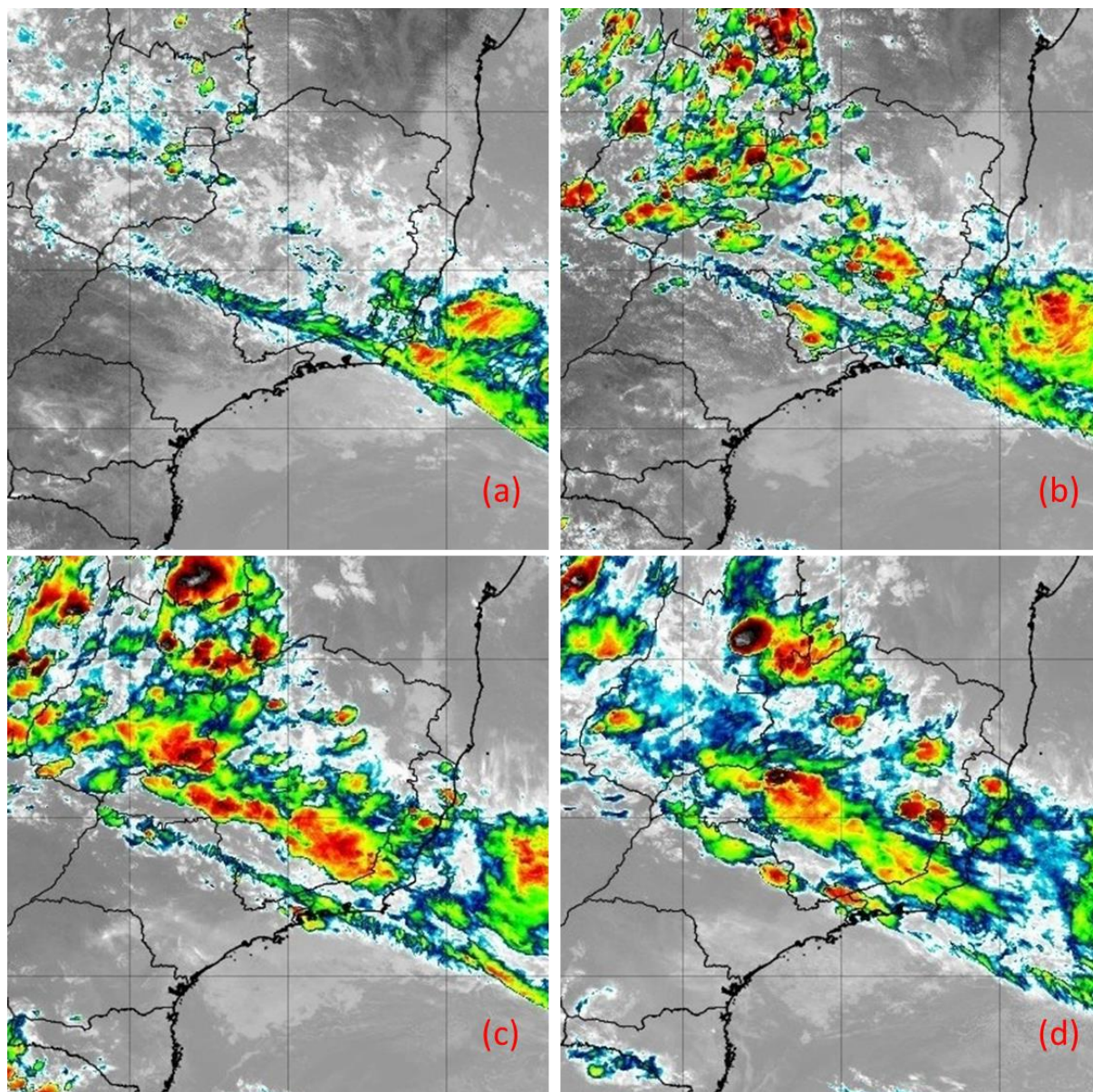
Figura 8 - Imagens do satélite GOES-16 do dia 19/11/2019 as 12:00 (a), 15:00 (b), 18:00 (c) e 21:00 horas local. Fonte: INPE.
