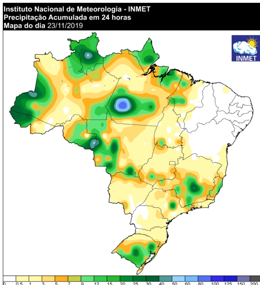
Figura 26 - Precipitação ocorrida no dia 22/11/2019. Fonte: INMET.
