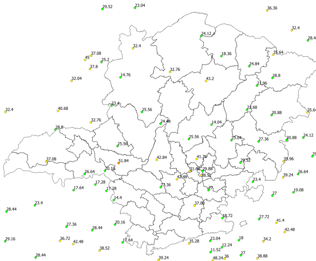
Figura 10 - Rajadas de vento registradas no dia 19/11/2019. Fonte: INMET.
