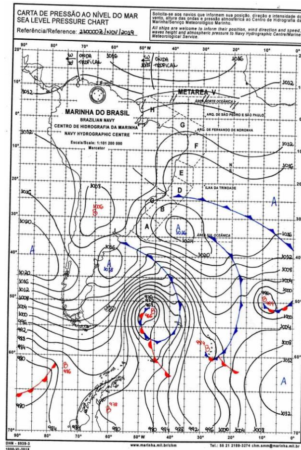
Figura 17 - Carta Sinótica do Dia 21/11/2019. Fonte: Marinha Brasileira.
