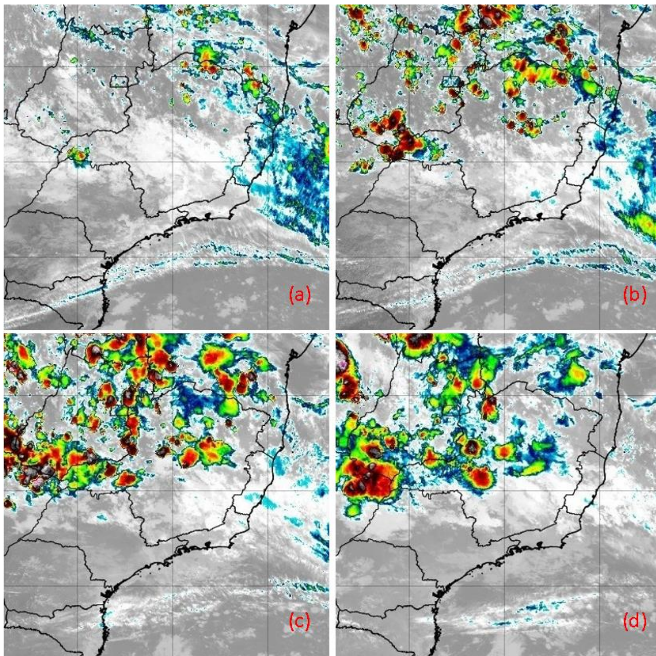
Figura 13 - Imagens do satélite GOES-16 do dia 23/02/2020 as 12:00 (a), 15:00 (b), 18:00 (c) e 21:00 horas local. Fonte: INPE.
