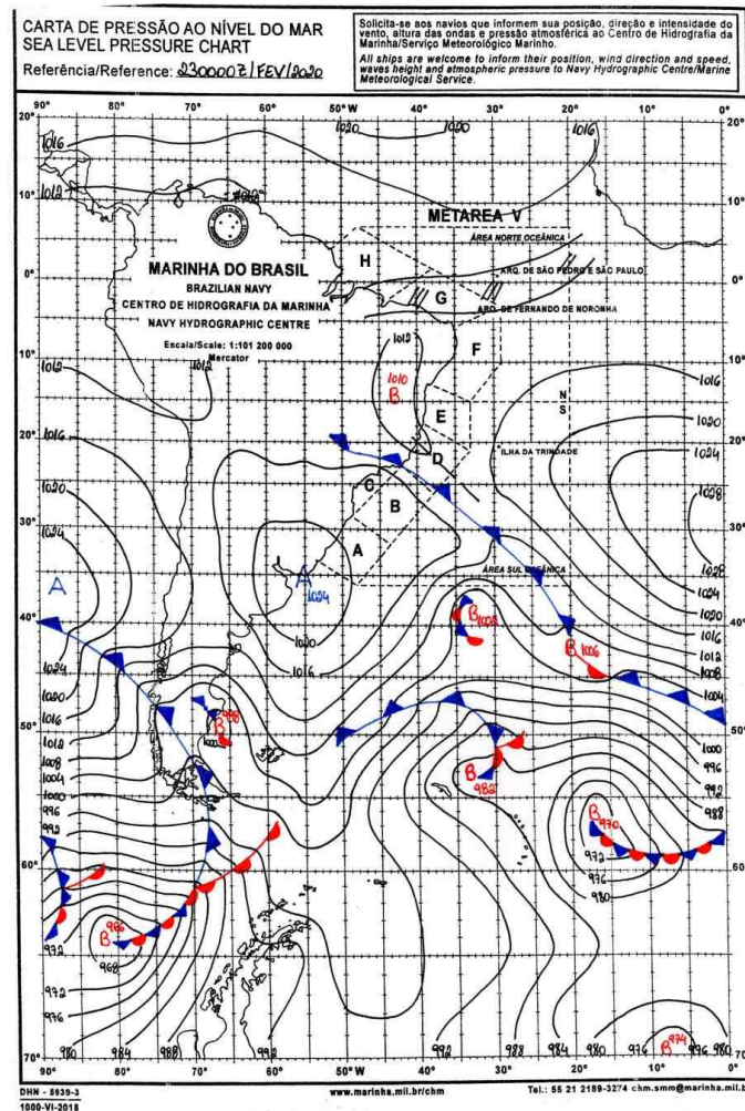
Figura 12 - Carta Sinótica do Dia 23/02/2020. Fonte: Marinha Brasileira.
