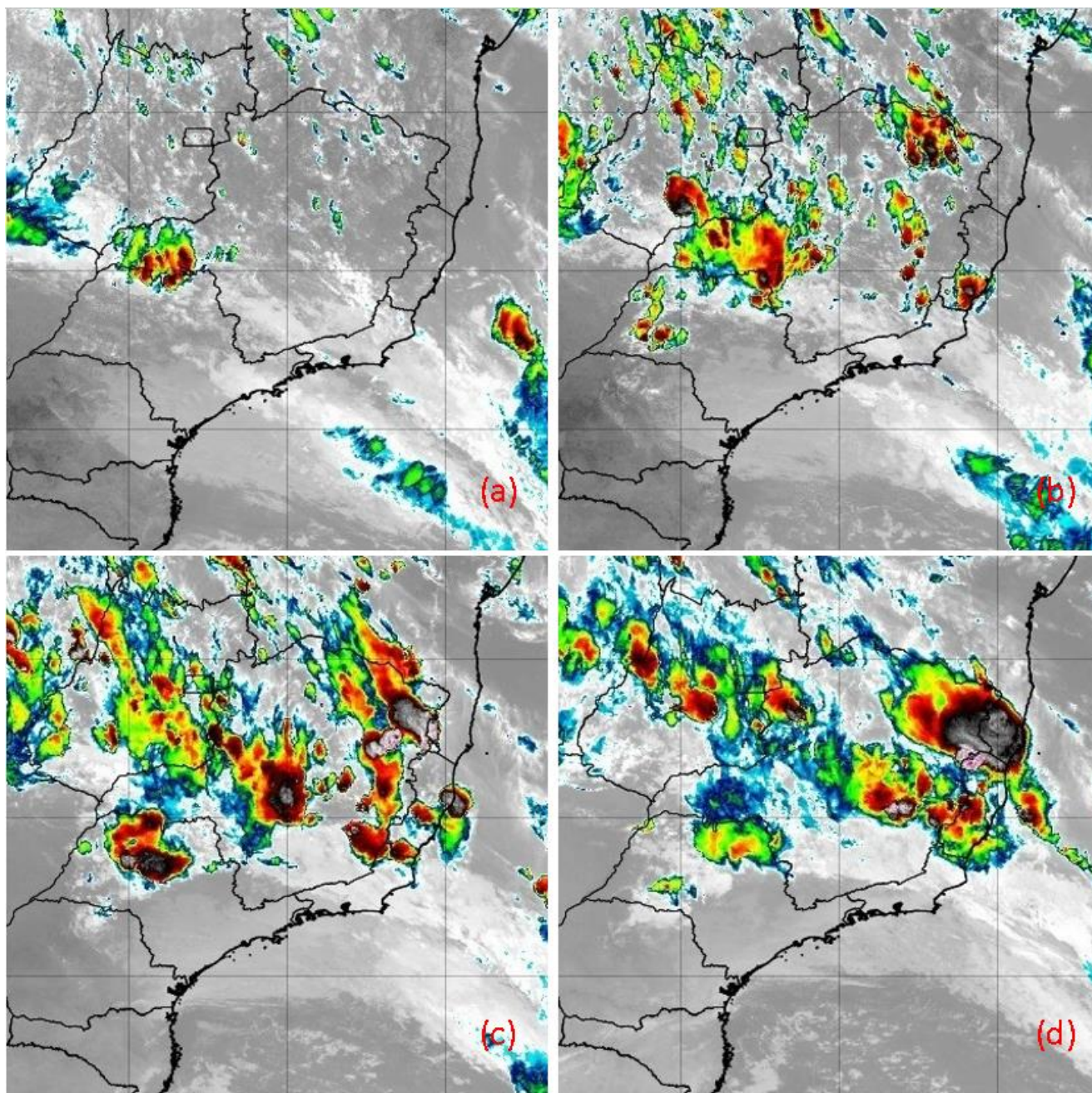
Figura 8 - Imagens do satélite GOES-16 do dia 22/02/2020 as 12:00 (a), 15:00 (b), 18:00 (c) e 21:00 horas local. Fonte: INPE.
