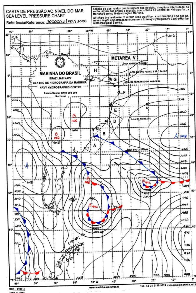
Figura 1 - Carta sinótica do dia 20/02/2020. Fonte: Marinha Brasileira.
