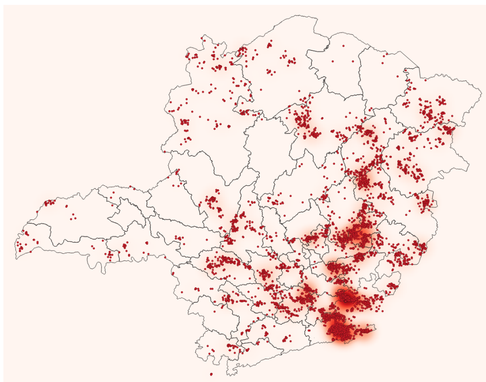
Figura 4 - Raios registrados no dia 21/02/2020. Fonte: RINDAT.
