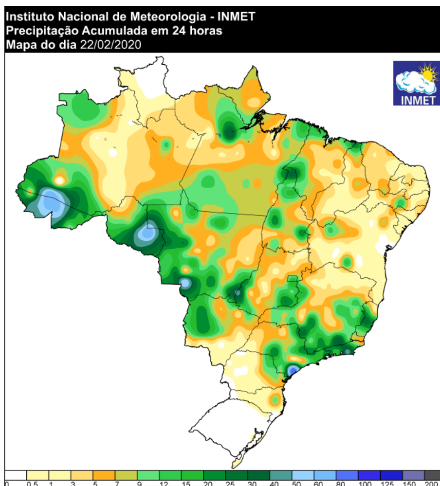
Figura 6 - Precipitação ocorrida no dia 21/02/2020. Fonte: INMET.
