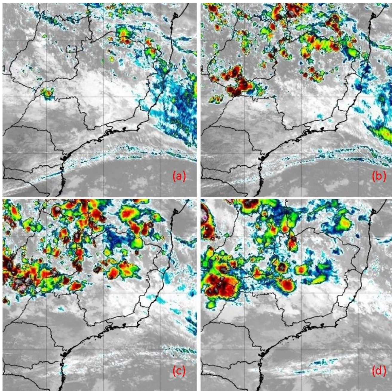
Figura 13, onde pode-se ver o desenvolvimento de núcleos convectivos entre o Triângulo Mineiro, Norte e Leste ao longo da tarde e da noite.
