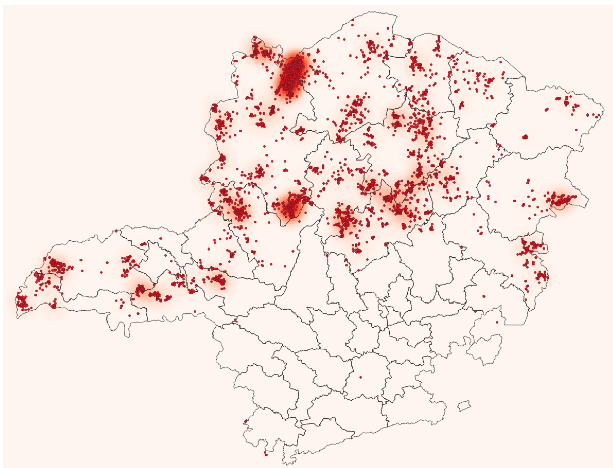
Figura 14 - Raios registrados no dia 23/02/2020. Fonte: RINDAT.
