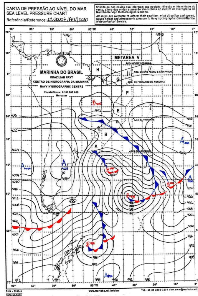
Figura 7 - Carta Sinótica do Dia 22/02/2020. Fonte: Marinha Brasileira.
