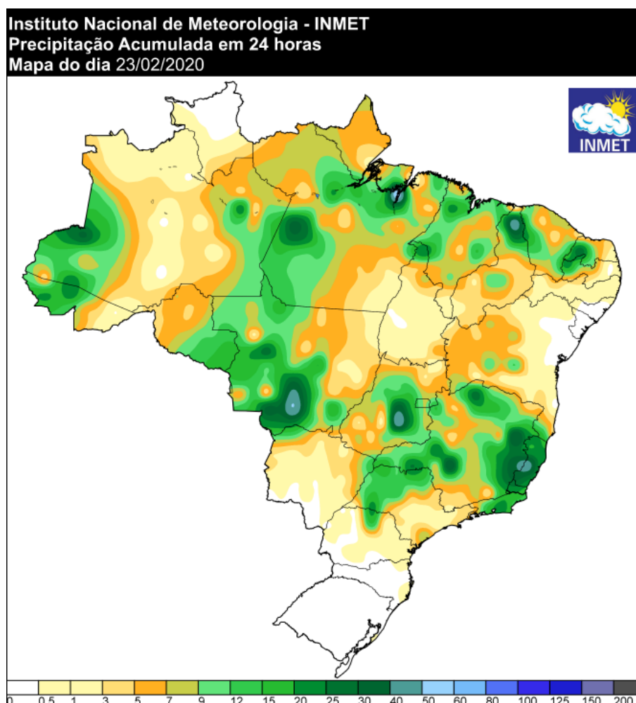
Figura 11 - Precipitação ocorrida no dia 22/02/2020. Fonte: INMET.
