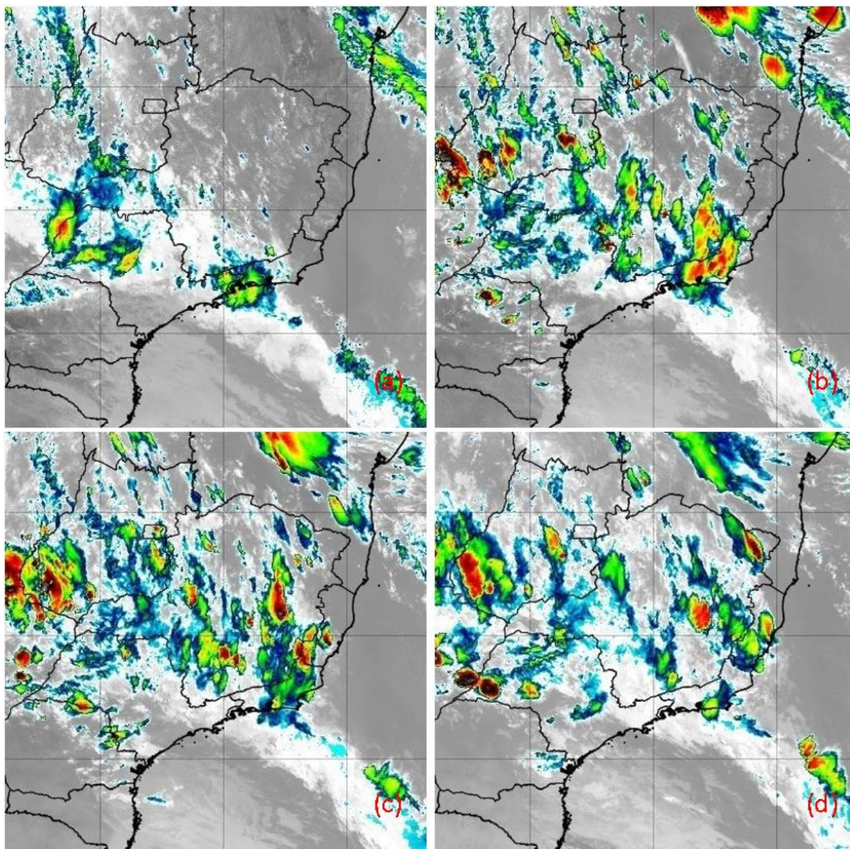
Figura 3 - Imagens do satélite GOES-16 do dia 21/02/2020 as 12:00 (a), 16:00 (b), 18:00 (c) e 21:00 horas local. Fonte: INPE.
