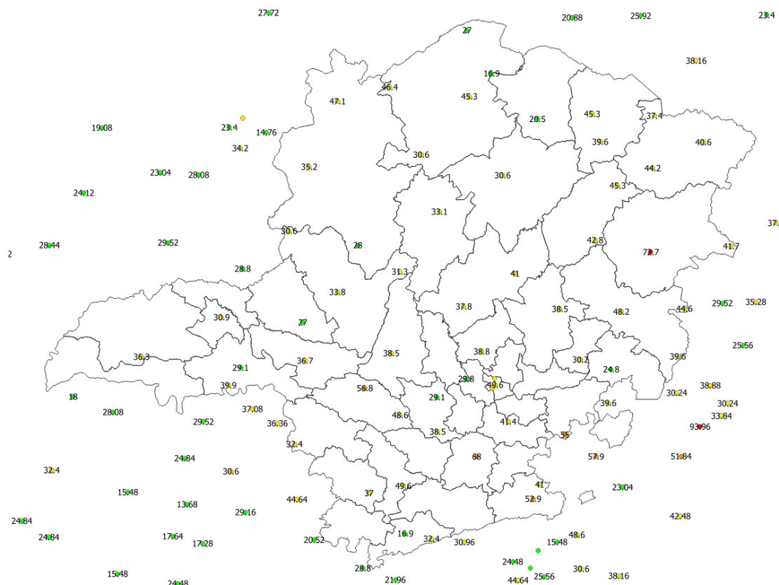
Figura 5 - Rajadas de vento registradas no dia 21/02/2020. Fonte: INMET.
