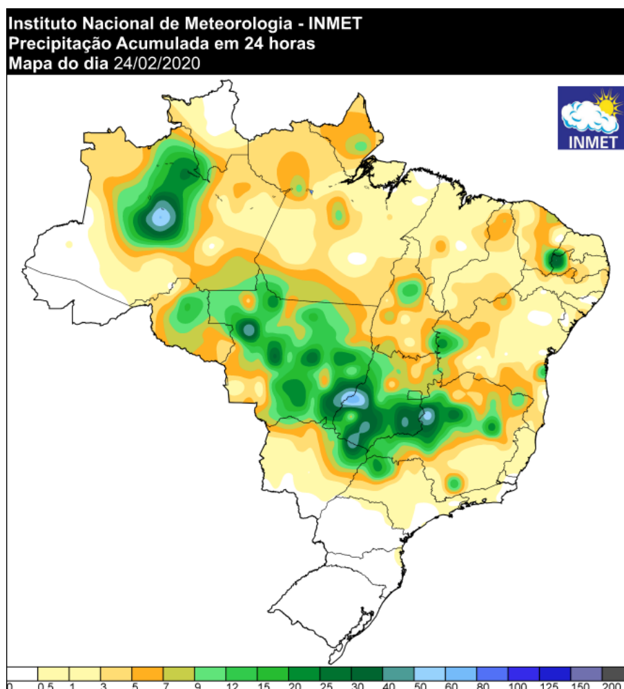
Figura 16 - Precipitação ocorrida no dia 23/02/2020. Fonte: INMET.
