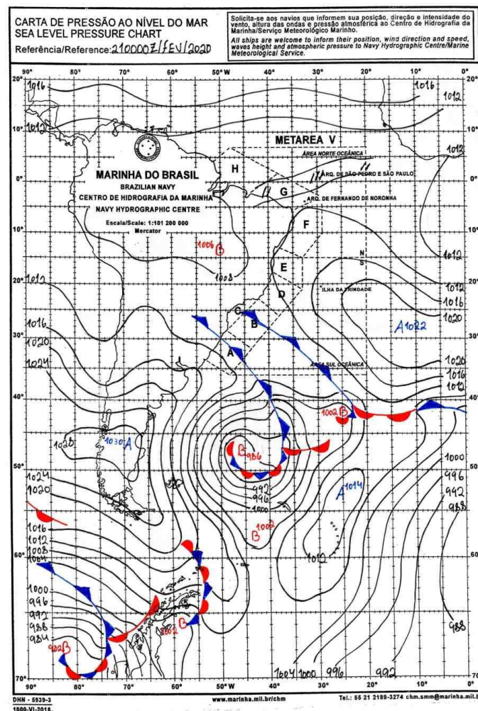
Figura 2 - Carta Sinótica do Dia 21/02/2020. Fonte: Marinha Brasileira.
