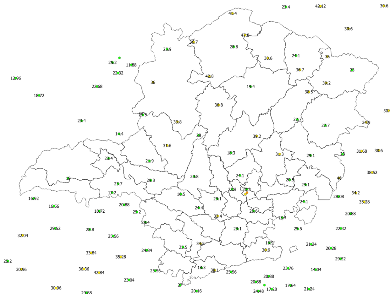
Figura 15 - Rajadas de vento registradas no dia 23/02/2020. Fonte: INMET.
