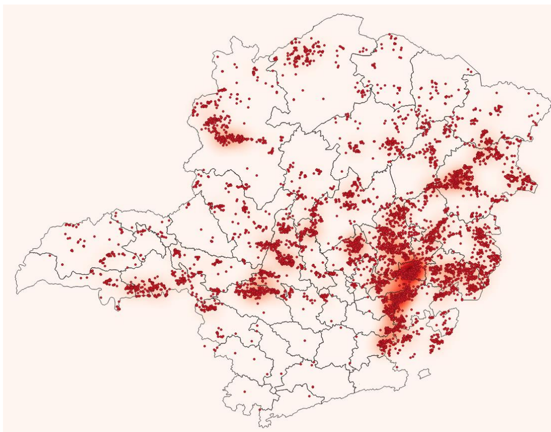
Figura 9 - Raios registrados no dia 22/02/2020. Fonte: RINDAT.
