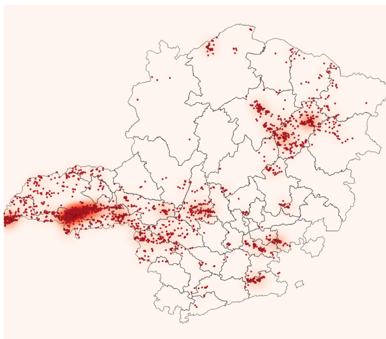
Figura 5 Localização dos raios registrados no dia 21/10/2019. Fonte: RINDAT
