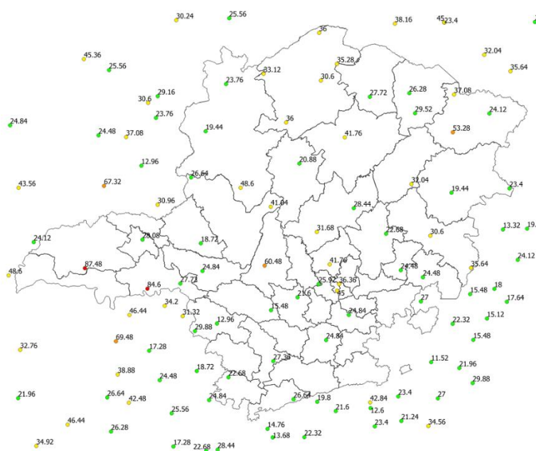
Figura 6 Rajadas de Vento registradas no dia 21/10/2019. Fonte: INMET.
