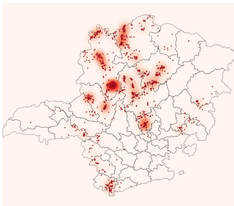
Figura 15 Localização dos raios registrados no dia 23/10/2019. Fonte RINDAT.
