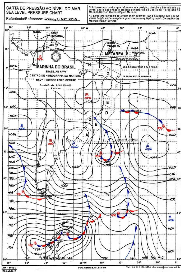
Figura 1 - Carta Sinótica do dia 20/10/2019. Fonte: Marinha Brasileira
