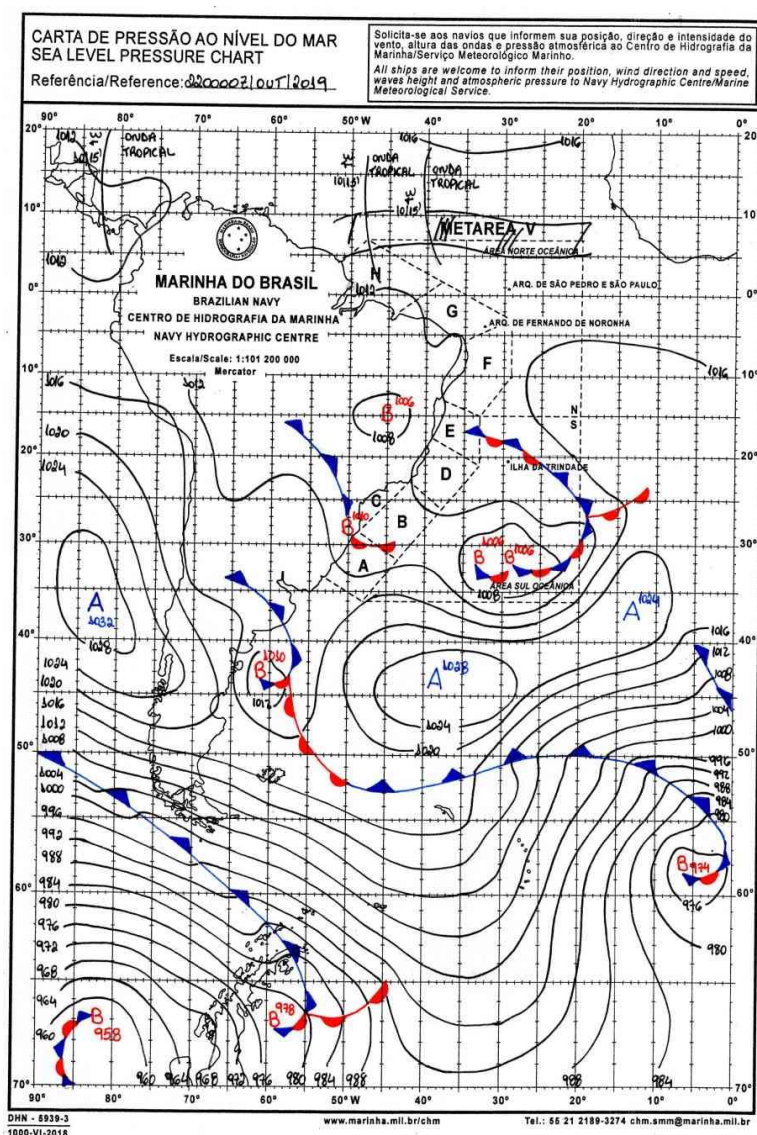
Figura 8 Carta Sinótica do dia 22/10/2019. Fonte: Marinha Brasileira.
