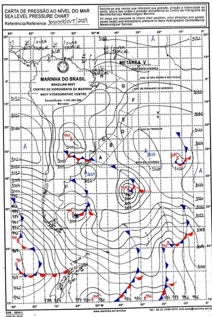
Figura 23 Carta Sinótica do dia 23/10/2019. Fonte: Marinha Brasileira.
