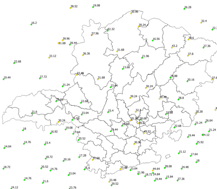
Figura 11 Rajadas de Vento registradas no dia 22/10/2019
