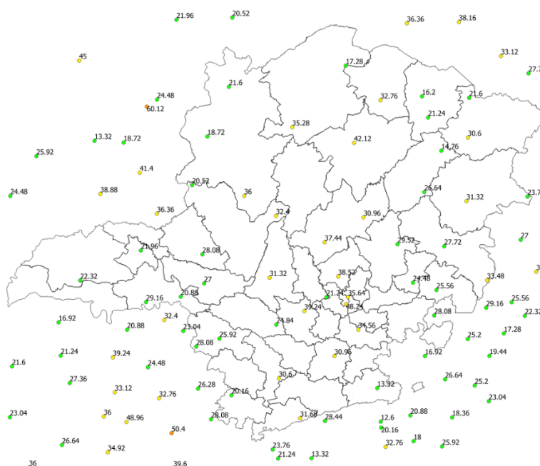
Figura 16 Rajadas de vento observadas no dia 23/10/2019. Fonte: INMET.
