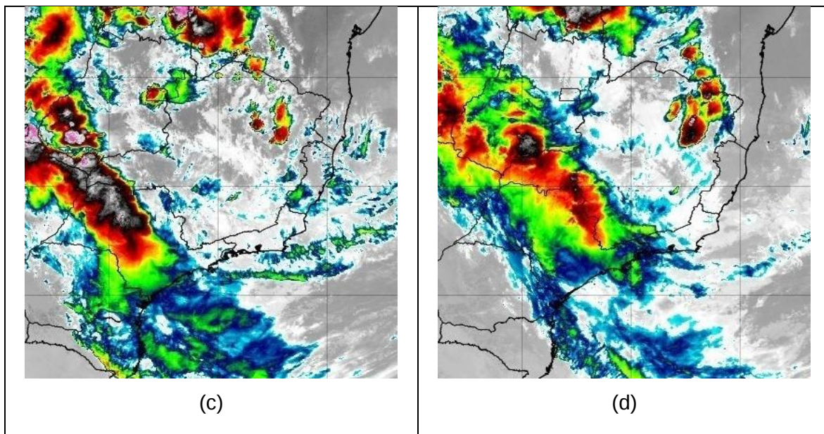
Figura 4 Imagens de Satélite do dia 21/10 as 09:30 (a), 12:30 (b), 16:00 (c) e 19:00 (d). Fonte: INPE
