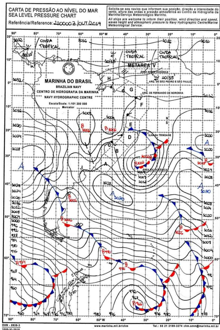
Figura 3 Carta Sinótica do dia 21/10/2019. Fonte: Marinha Brasileira
