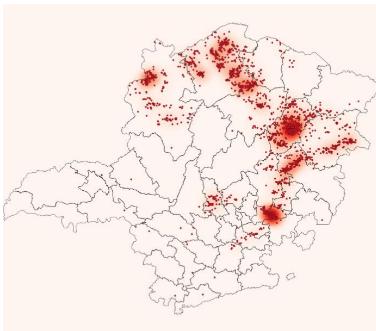
Figura 10 Localização dos raios registrados no dia 22/10/2019
