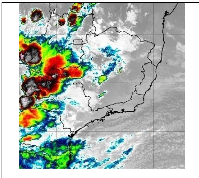
Figura 2 Imagem de Satélite do dia 20/10 as 20:30. Fonte:INPE
