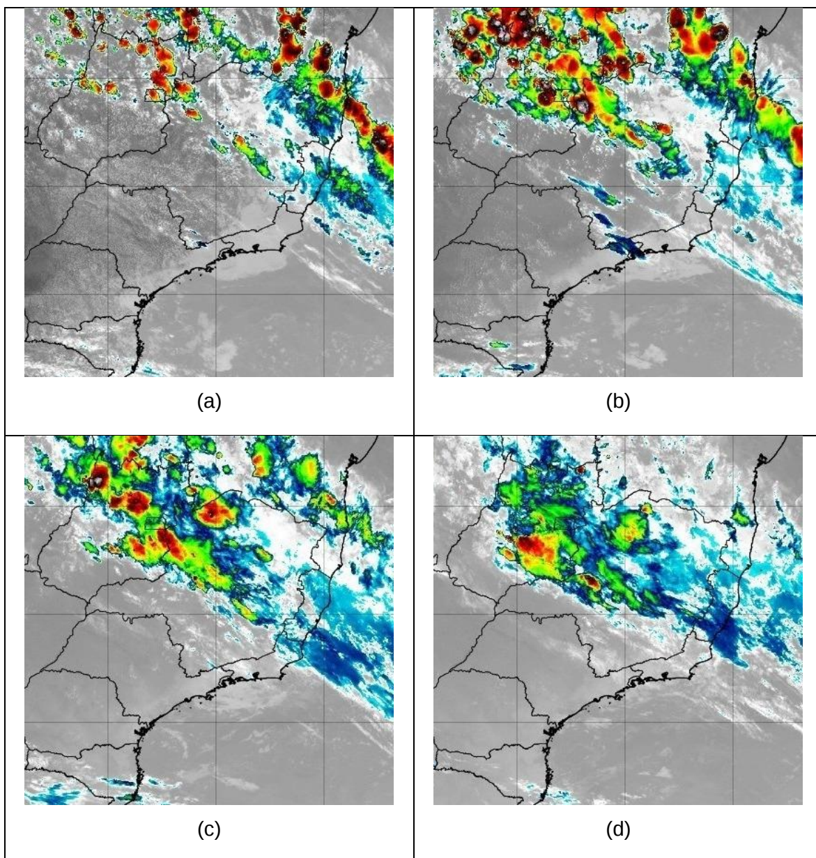
Figura 14 Imagens de Satélite do dia 23/10 as 14:00 (a), 17:00 (b), 20:00 (c) e 23:00 (d). Fonte: INPE.
