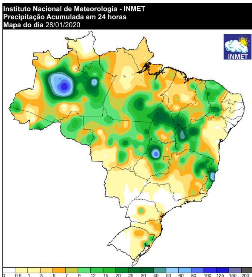
Figura 24 - Precipitação ocorrida no dia 27/01/2020. Fonte: INMET.
