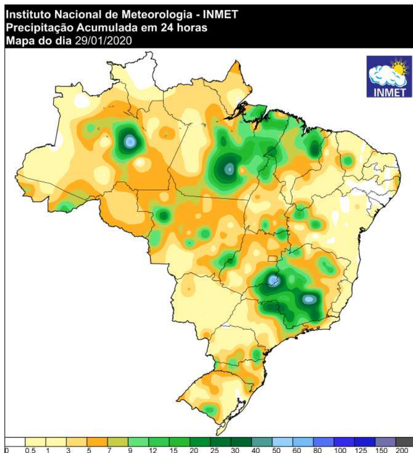
Figura 29 - Precipitação ocorrida no dia 28/01/2020. Fonte: INMET.
