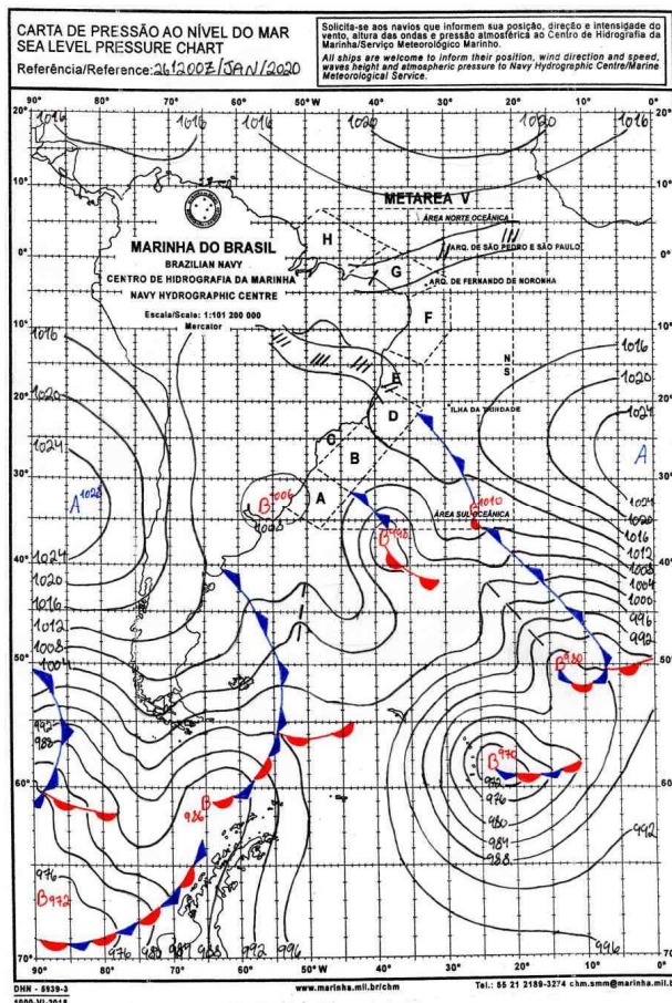
Figura 15 - Carta Sinótica do Dia 26/01/2020. Fonte: Marinha Brasileira.
