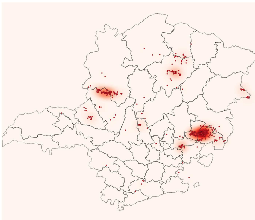
Figura 12 - Raios registrados no dia 25/01/2020. Fonte: RINDAT.
