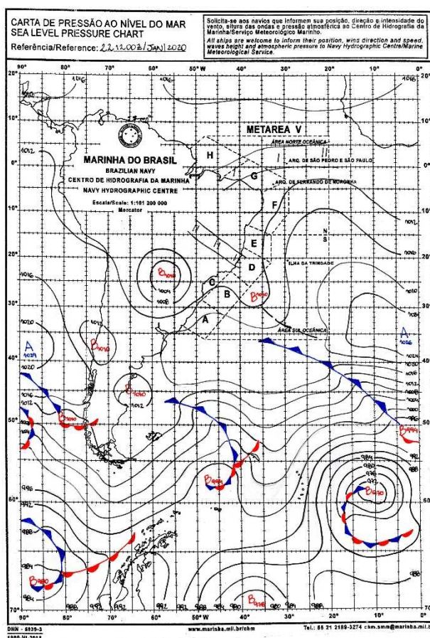
Figura 1 - Carta Sinótica do Dia 22/01/2020. Fonte: Marinha Brasileira.
