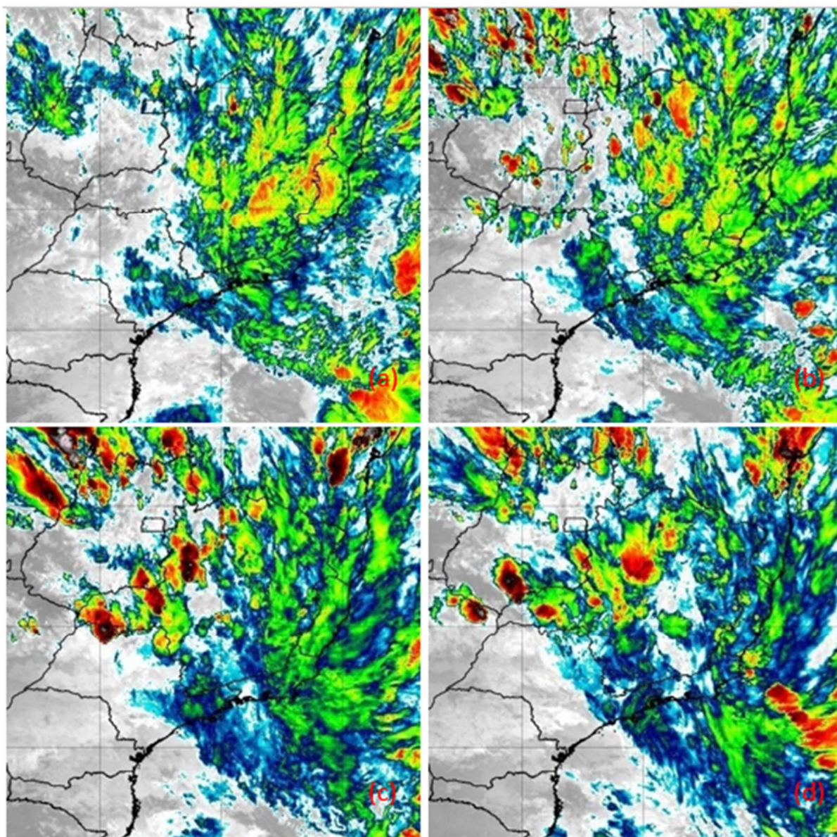
Figura 2 - Imagens do satélite GOES-16 do dia 23/01/2020 as 12:00 (a), 15:00 (b), 18:00 (c) e 21:00 horas local. Fonte: INPE.
