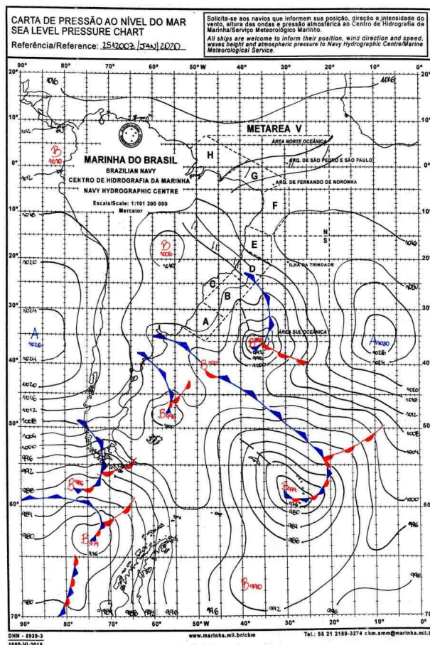
Figura 10 - Carta Sinótica do Dia 25/01/2020. Fonte: Marinha Brasileira.
