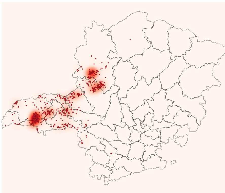
Figura 3 - Raios registrados no dia 23/01/2020. Fonte: RINDAT.
