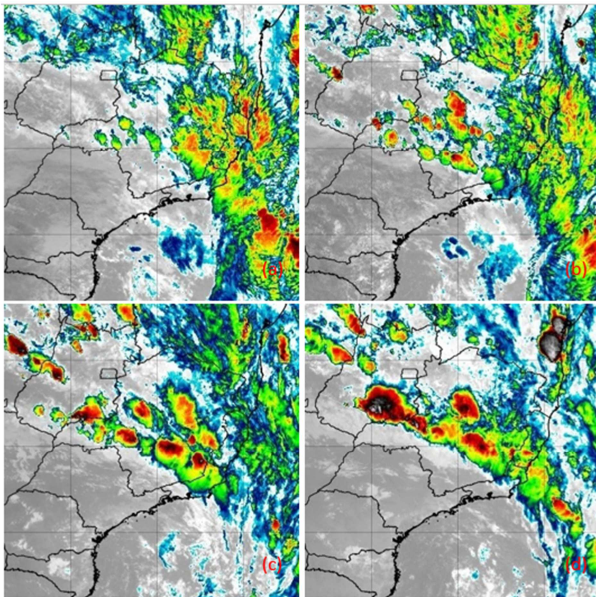
Figura 6 - Imagens do satélite GOES-16 do dia 24/01/2020 as 12:00 (a), 15:00 (b), 18:00 (c) e 21:00 horas local. Fonte: INPE.
