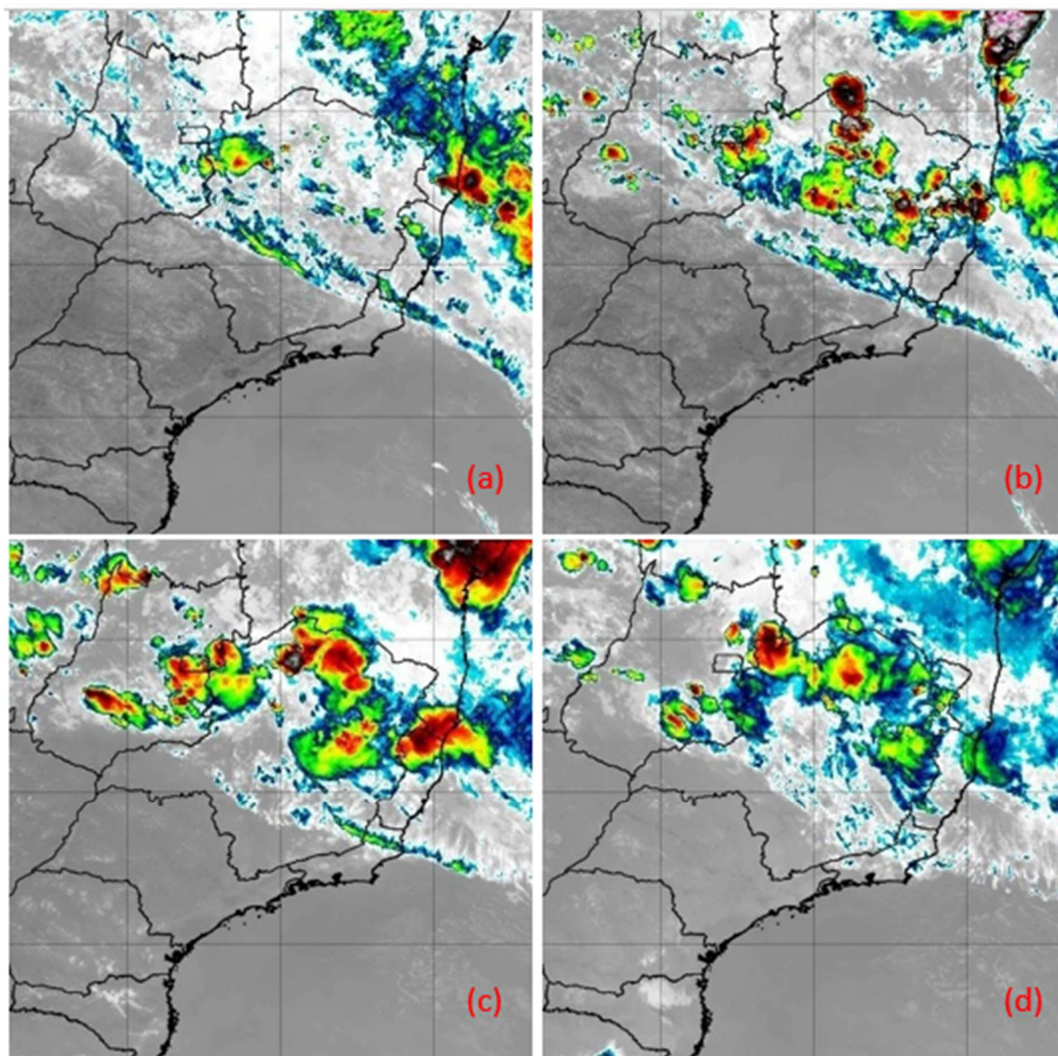
Figura 16 - Imagens do satélite GOES-16 do dia 26/01/2020 as 12:00 (a), 15:00 (b), 18:00 (c) e 21:00 horas local. Fonte: INPE.
