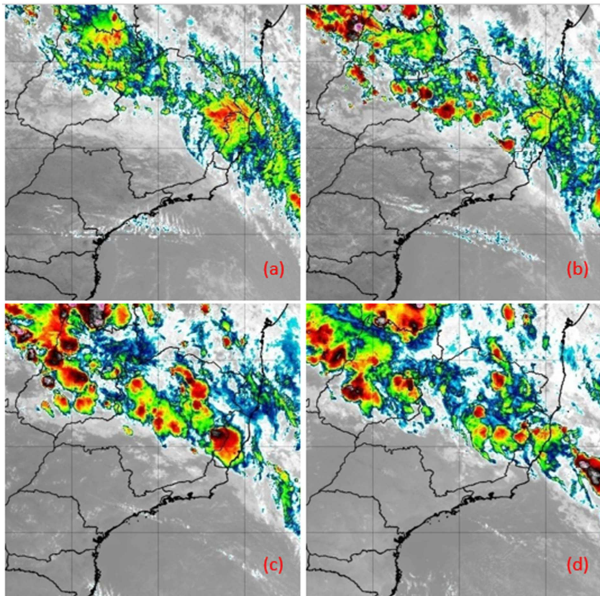
Figura 11 - Imagens do satélite GOES-16 do dia 25/01/2020 as 12:00 (a), 15:00 (b), 18:00 (c) e 21:00 horas local. Fonte: INPE.
