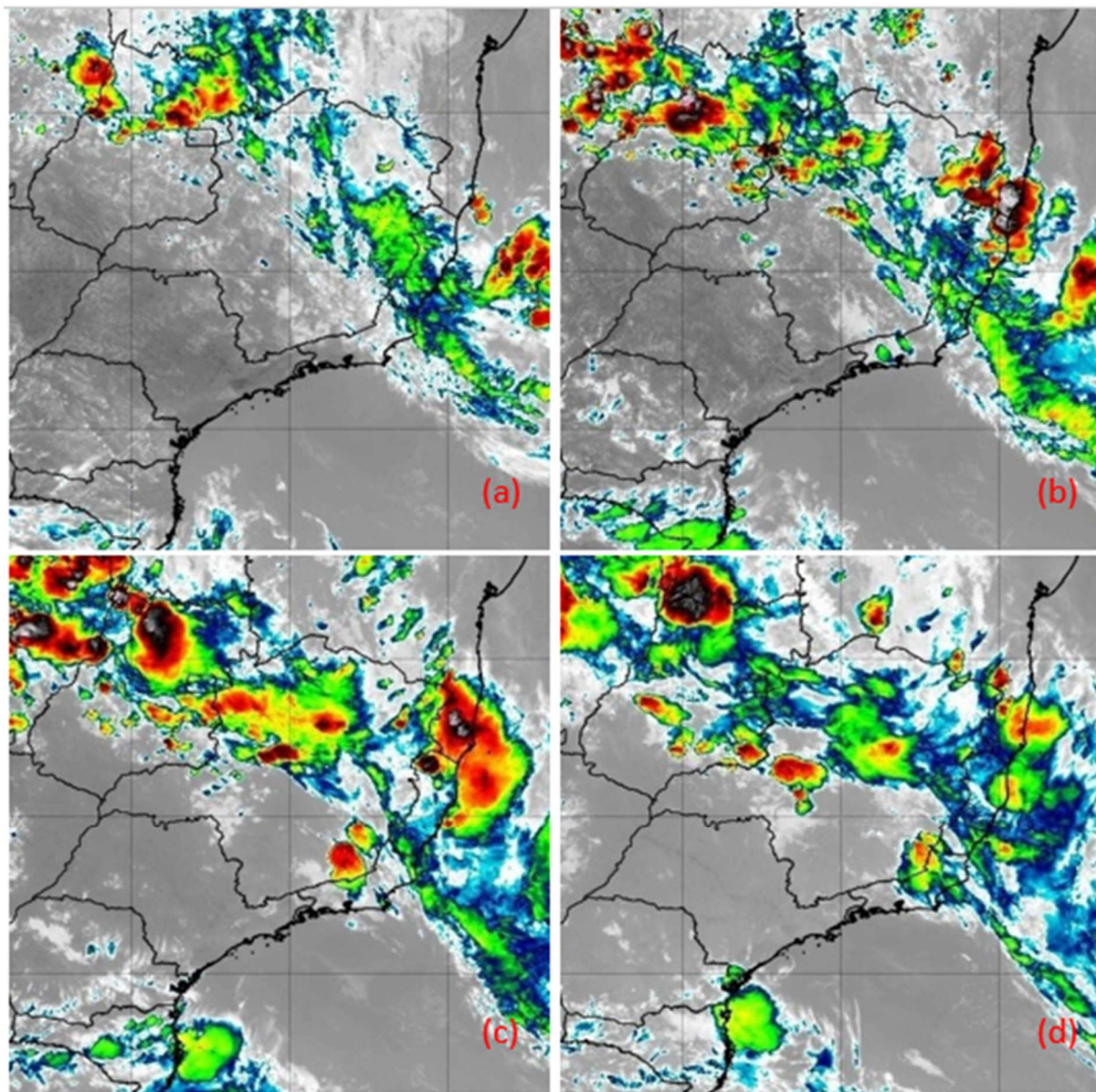
Figura 21 - Imagens do satélite GOES-16 do dia 27/01/2020 as 12:00 (a), 15:00 (b), 18:00 (c) e 21:00 horas local. Fonte: INPE.
