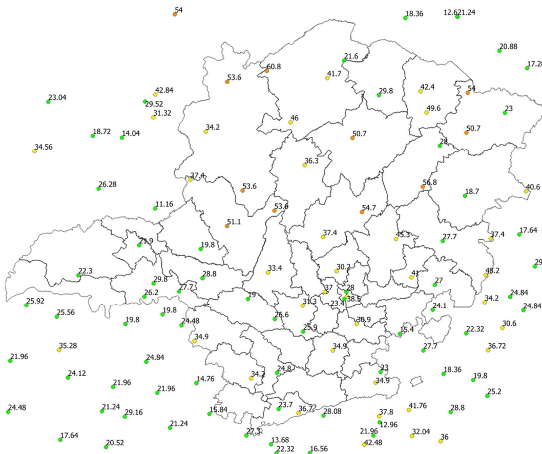
Figura 13 - Rajadas de vento registradas no dia 25/01/2020. Fonte: INMET.
