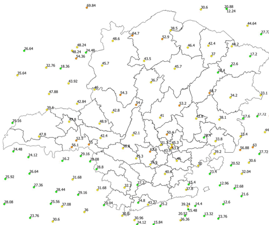
Figura 8 - Rajadas de vento registradas no dia 24/01/2020. Fonte: INMET.
