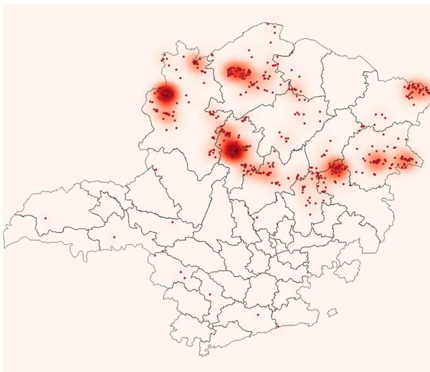
Figura 17 - Raios registrados no dia 26/01/2020. Fonte: RINDAT.
