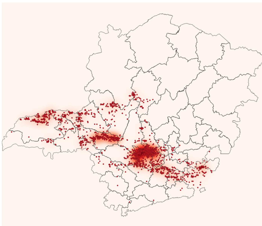
Figura 7 - Raios registrados no dia 24/01/2020. Fonte: RINDAT.
