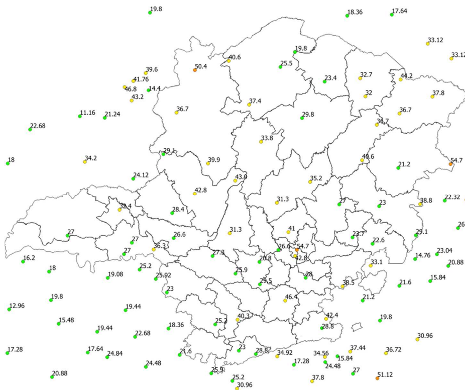
Figura 23 - Rajadas de vento registradas no dia 27/01/2020. Fonte: INMET.
