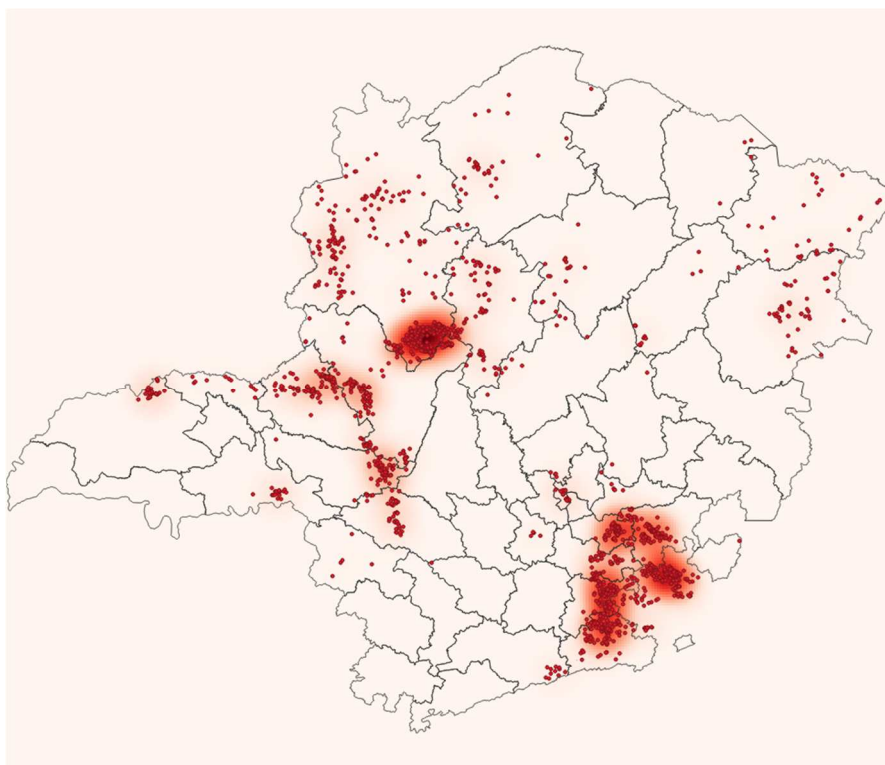
Figura 22 - Raios registrados no dia 27/01/2020. Fonte: RINDAT.
