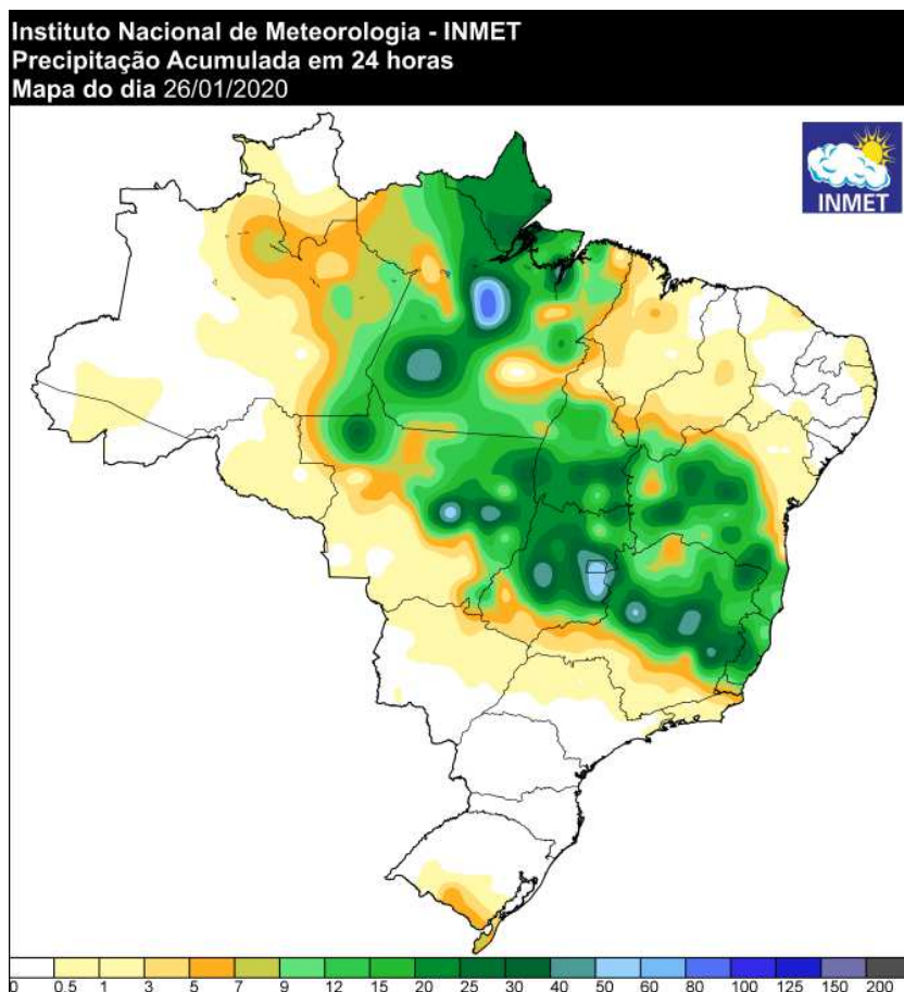
Figura 14 - Precipitação ocorrida no dia 25/01/2020. Fonte: INMET.
