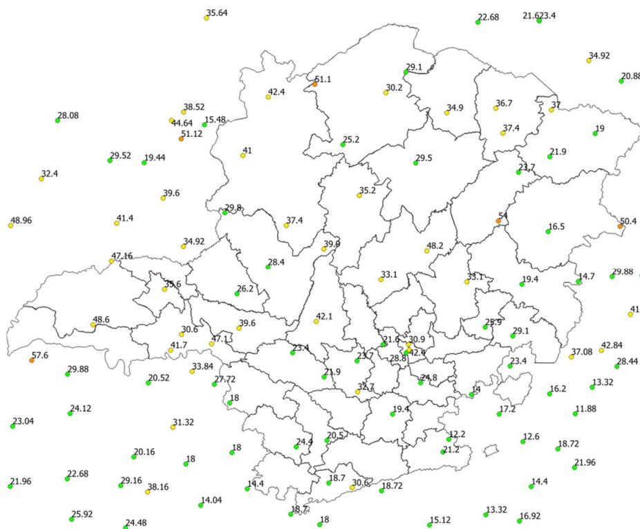
Figura 4 - Rajadas de vento registradas no dia 23/01/2020. Fonte: INMET.
