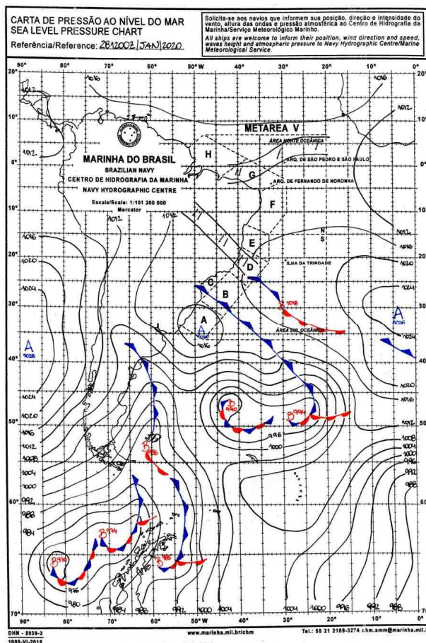
Figura 25 - Carta Sinótica do Dia 28/01/2020. Fonte: Marinha Brasileira.
