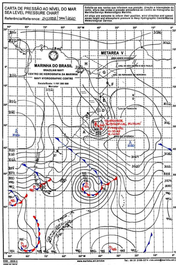
Figura 7 - Carta Sinótica do Dia 24/01/2020. Fonte: Marinha Brasileira.
