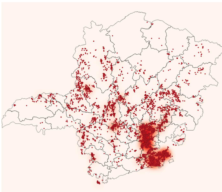
Figura 27 - Raios registrados no dia 28/01/2020. Fonte: RINDAT.
