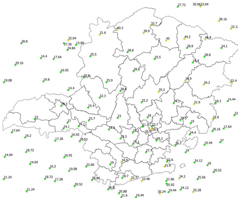
Figura 18 - Rajadas de vento registradas no dia 26/01/2020. Fonte: INMET.
