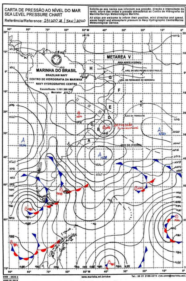
Figura 2 - Carta Sinótica do Dia 23/01/2020. Fonte: Marinha Brasileira.
