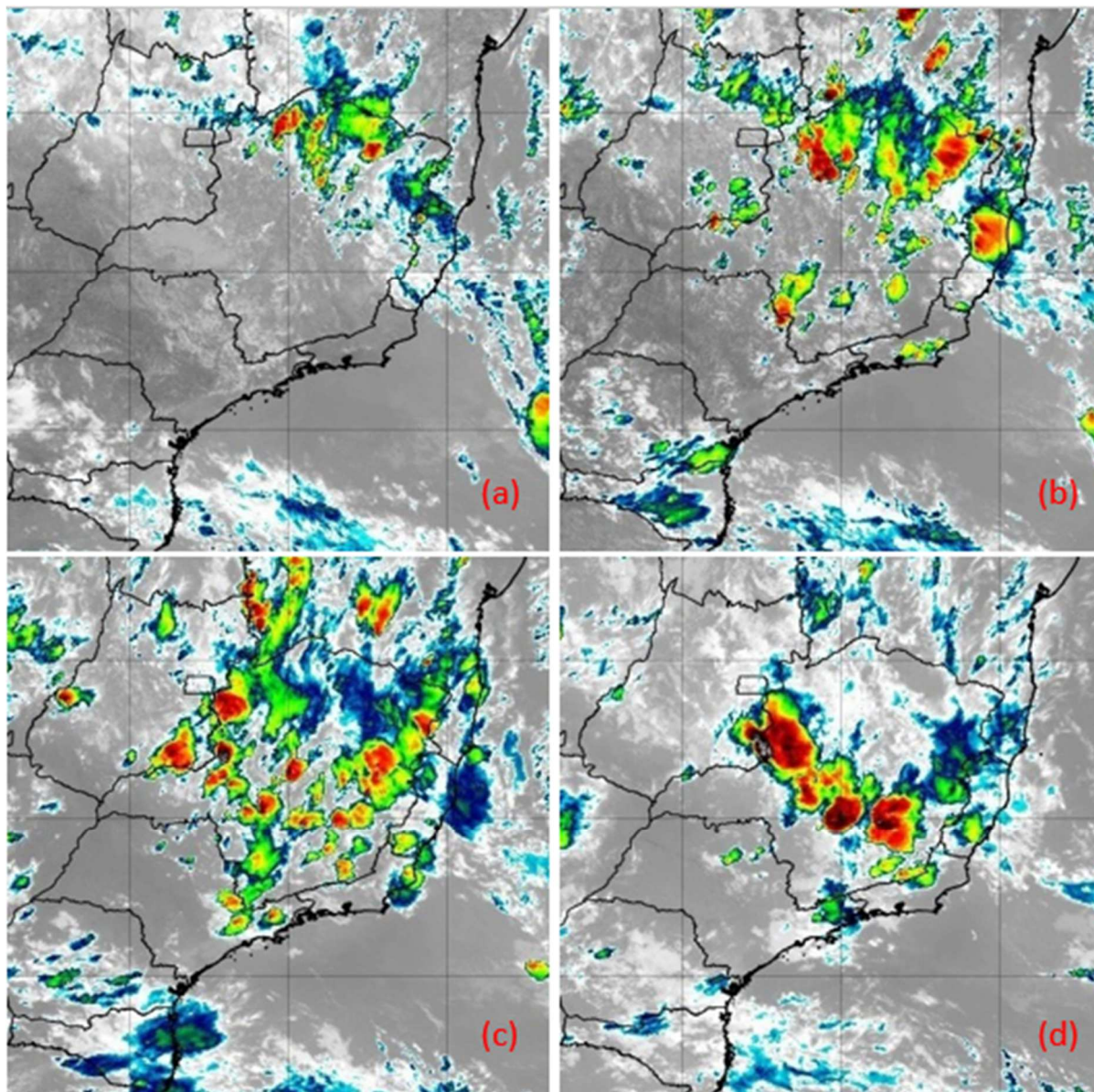
Figura 26 - Imagens do satélite GOES-16 do dia 28/01/2020 as 12:00 (a), 15:00 (b), 18:00 (c) e 21:00 horas local. Fonte: INPE.
