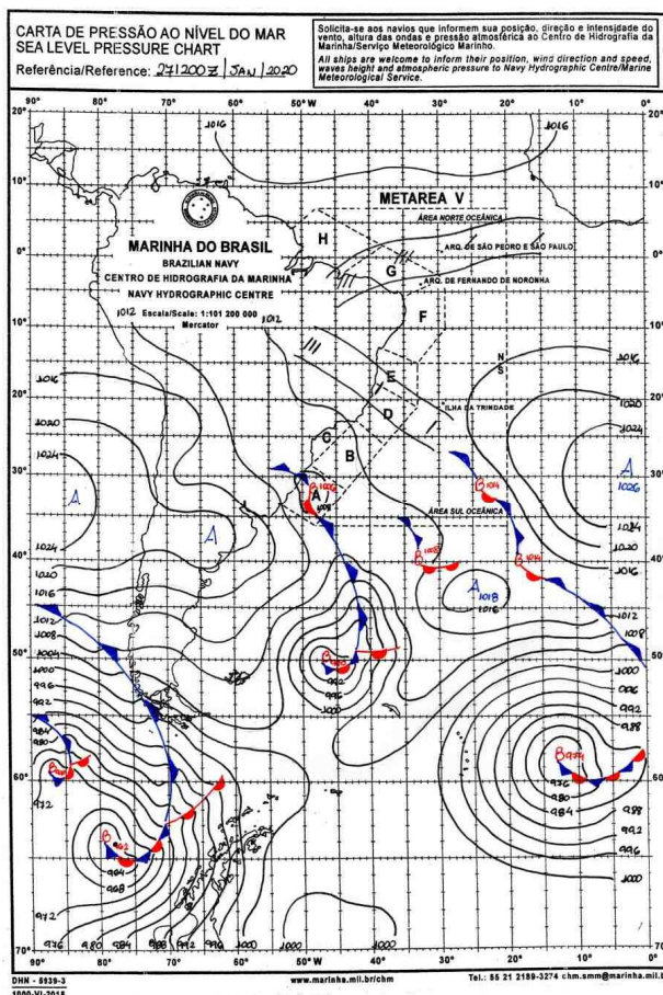
Figura 20 - Carta Sinótica do Dia 27/01/2020. Fonte: Marinha Brasileira.
