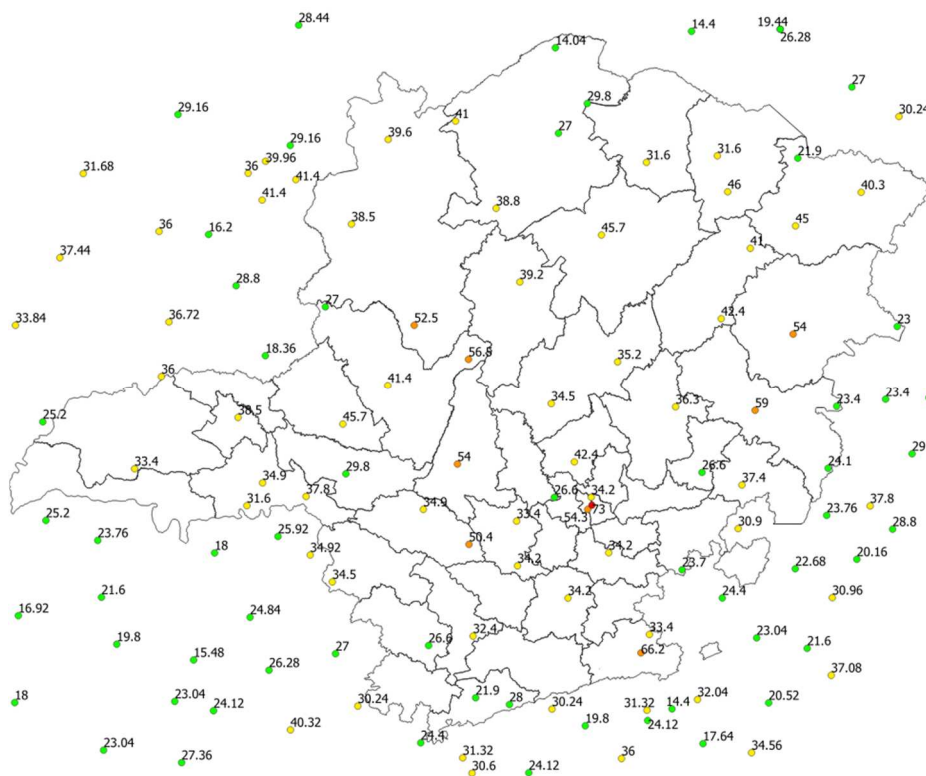
Figura 28 - Rajadas de vento registradas no dia 28/01/2020. Fonte: INMET.
