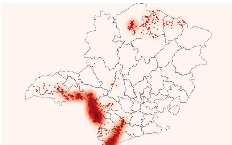
Figura 3 Localização dos raios registrados no dia 24/10/2019. Fonte: RINDAT
