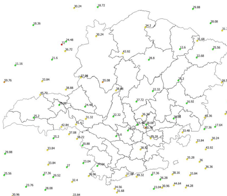
Figura 9 Rajadas de Vento registradas no dia 25/10/2019. Fonte: INMET.
