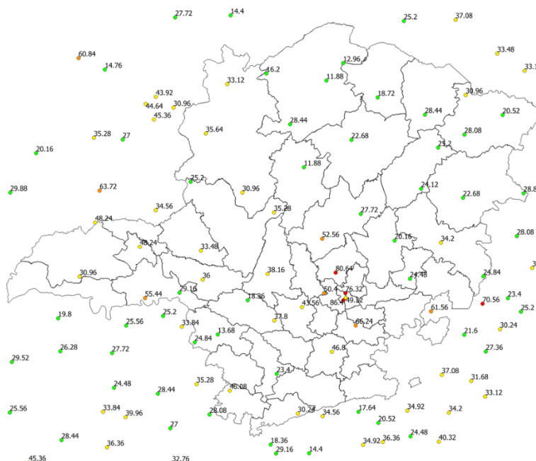
Figura 14 Rajadas de Vento registradas no dia 26/10/2019
