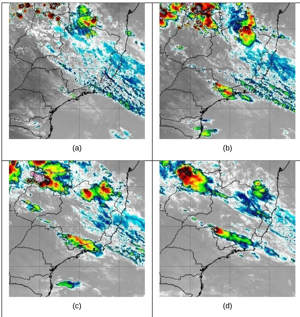
Figura 2 Imagens de Satélite do dia 24/10 as 13:00 (a), 16:00 (b), 19:00 (c) e 22:00 (d). Fonte: INPE
