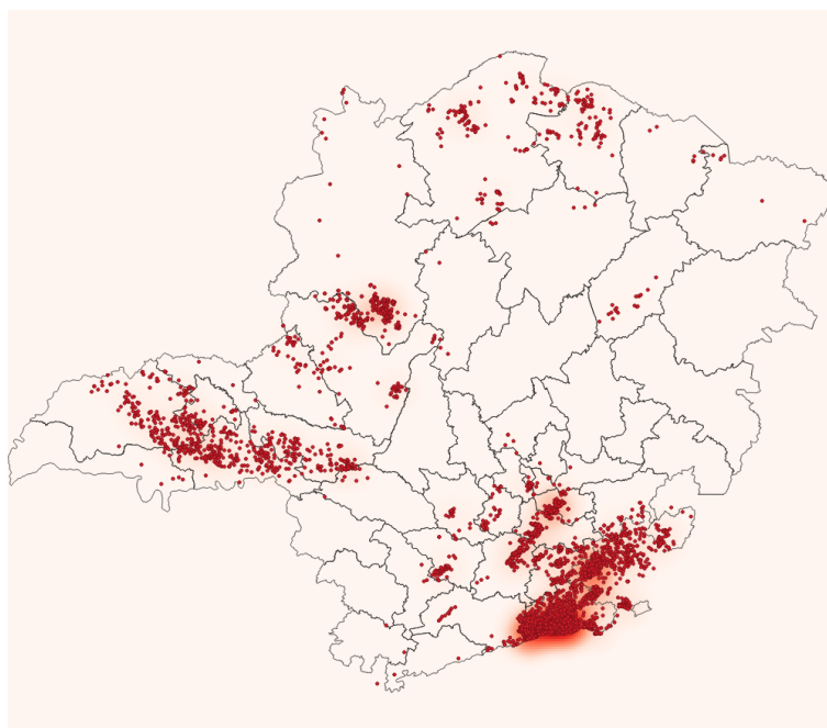
Figura 8 Localização dos raios registrados no dia 25/10/2019. Fonte: RINDAT
