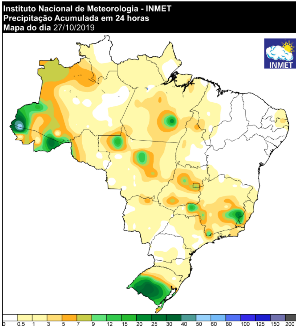
Figura 15 Pluviometria do dia 26/10/2019
