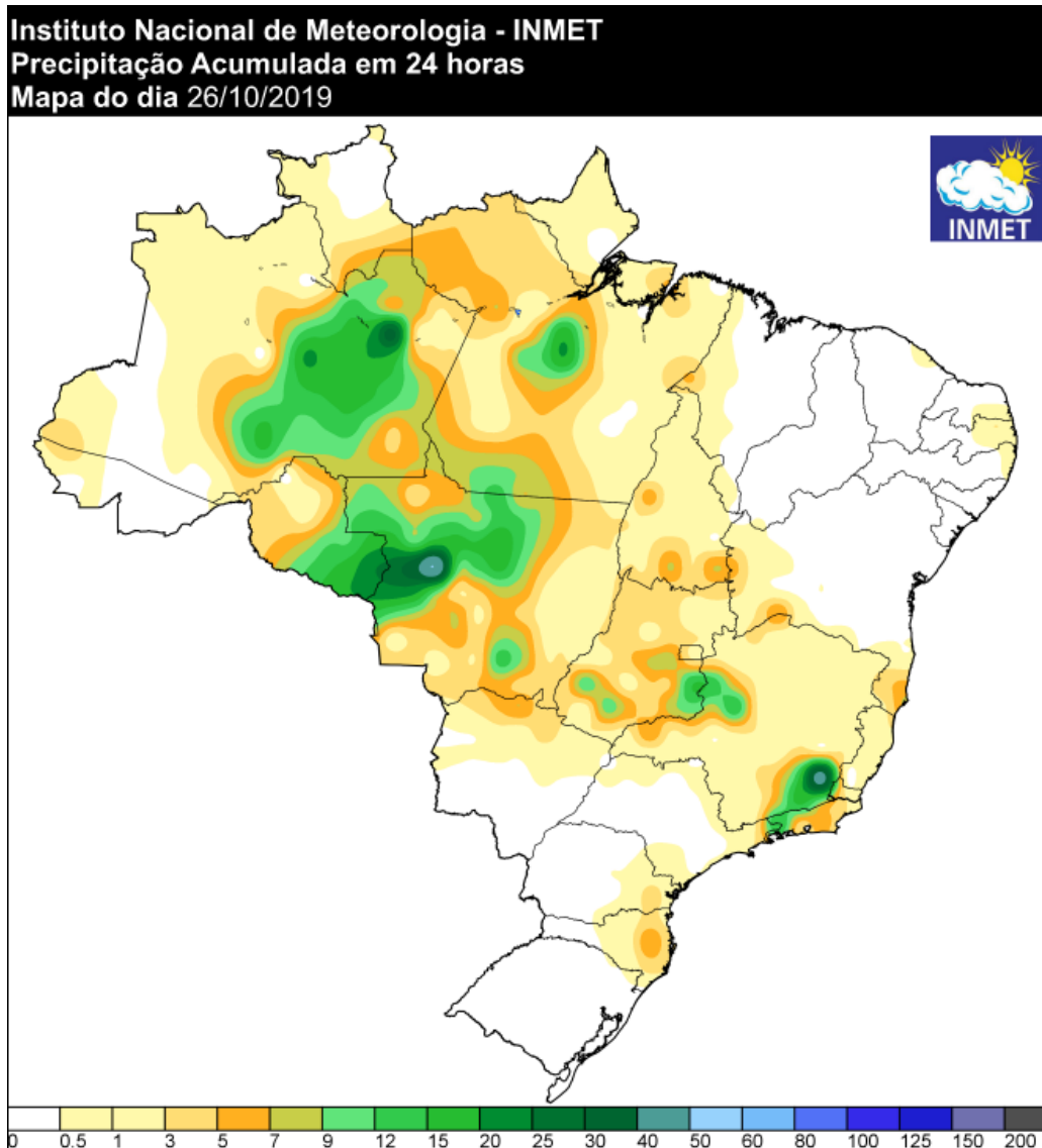
Figura 10 Pluviometria do dia 25/10/2019.
