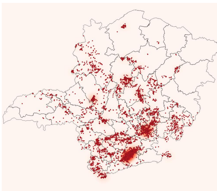
Figura 13 Localização dos raios registrados no dia 26/10/2019
