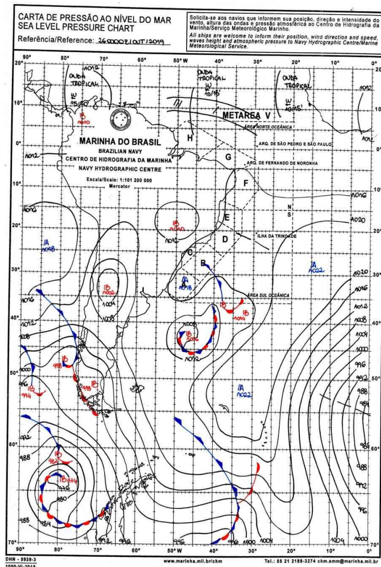
Figura 11 Carta Sinótica do dia 26/10/2019. Fonte: Marinha Brasileira.
