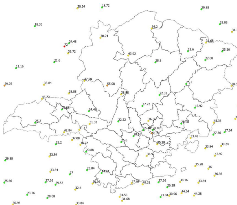
Figura 4 Rajadas de Vento registradas no dia 24/10/2019. Fonte: INMET.
