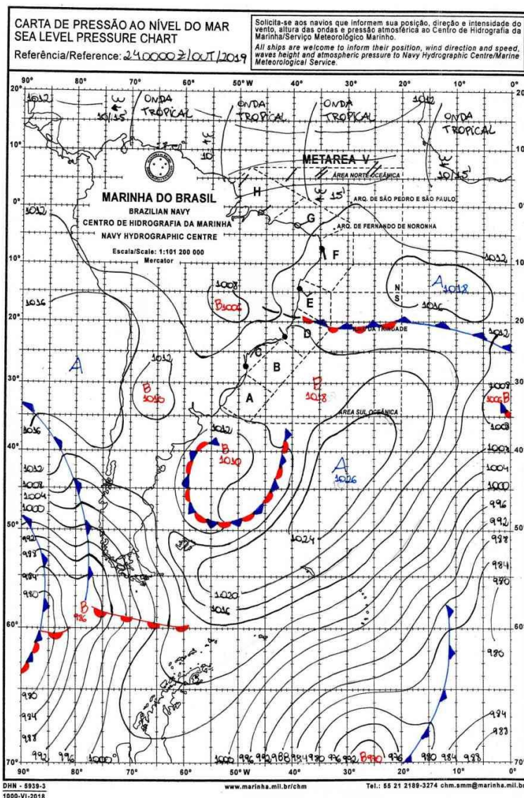
Figura 1 - Carta Sinótica do dia 24/10/2019. Fonte: Marinha Brasileira
