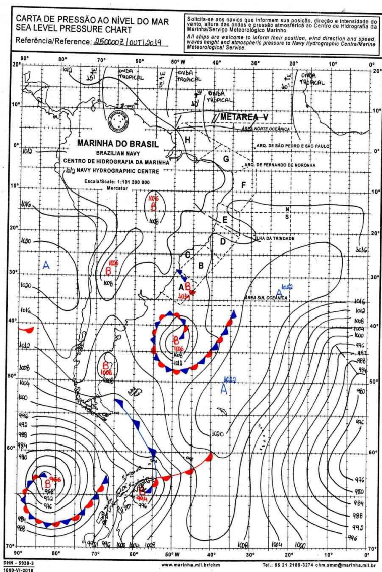
Figura 6 Carta Sinótica do dia 21/10/2019. Fonte: Marinha Brasileira
