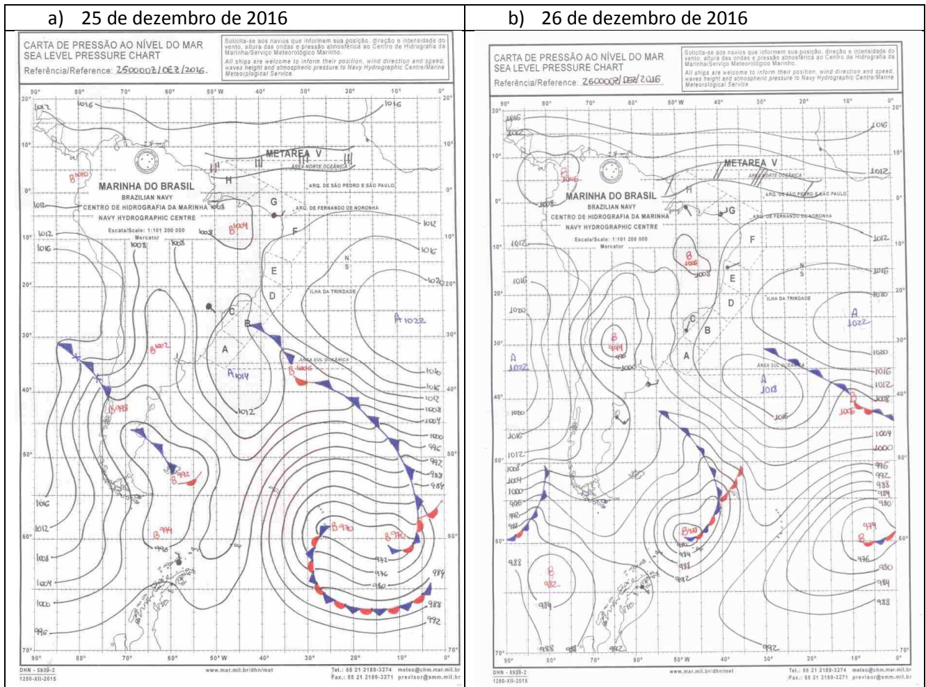
Figura 1 - Cartas Sinóticas elaboradas pela Marinha do Brasil para os dias 25 a 28 de dezembro de 2016.
