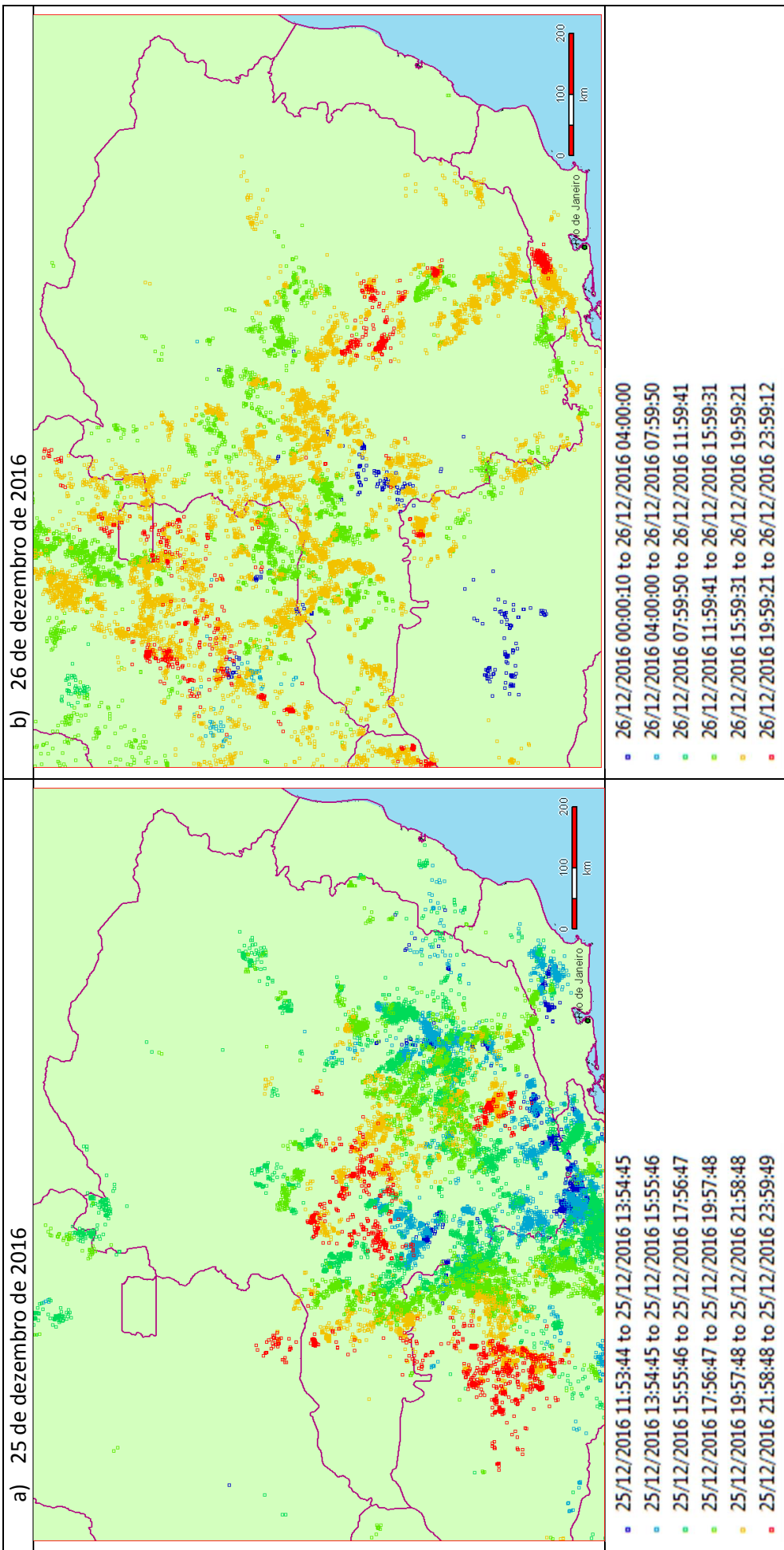
Figura 8 – Descargas atmosféricas registradas em Minas Gerais nos dias 25 a 28 de dezembro de 2016.
