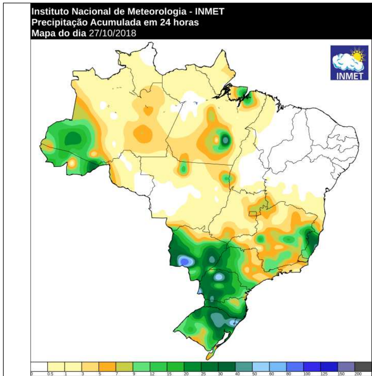
Figura 2 – Acumulado de precipitação (mm) no dia 27 de outubro de 2018.
