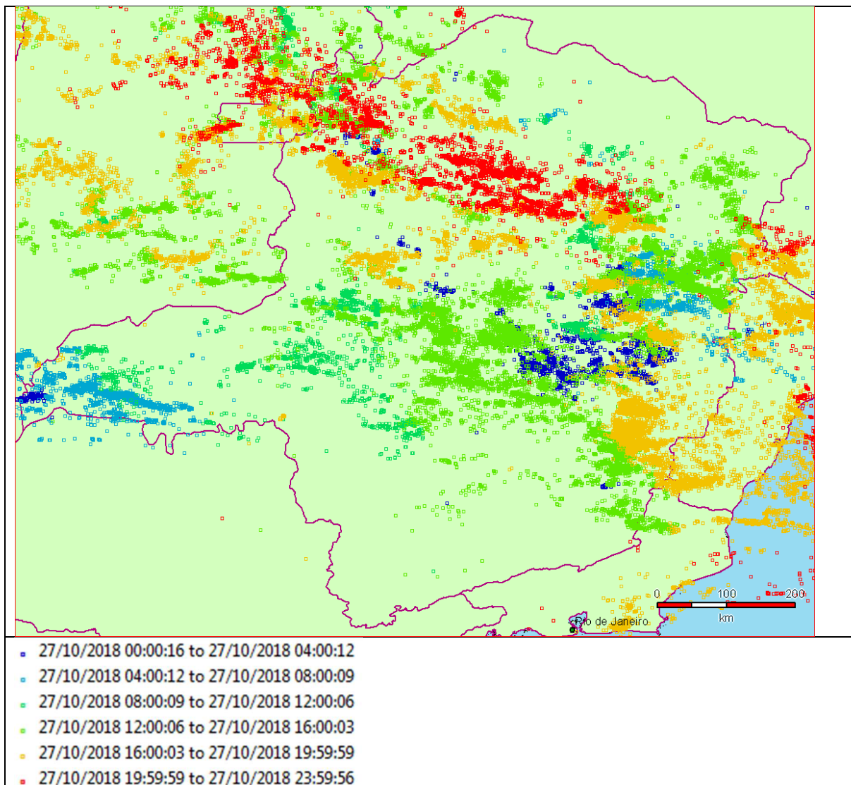
Figura 4 – Descargas atmosféricas registradas em Minas Gerais no dia 27 de outubro de 2018
