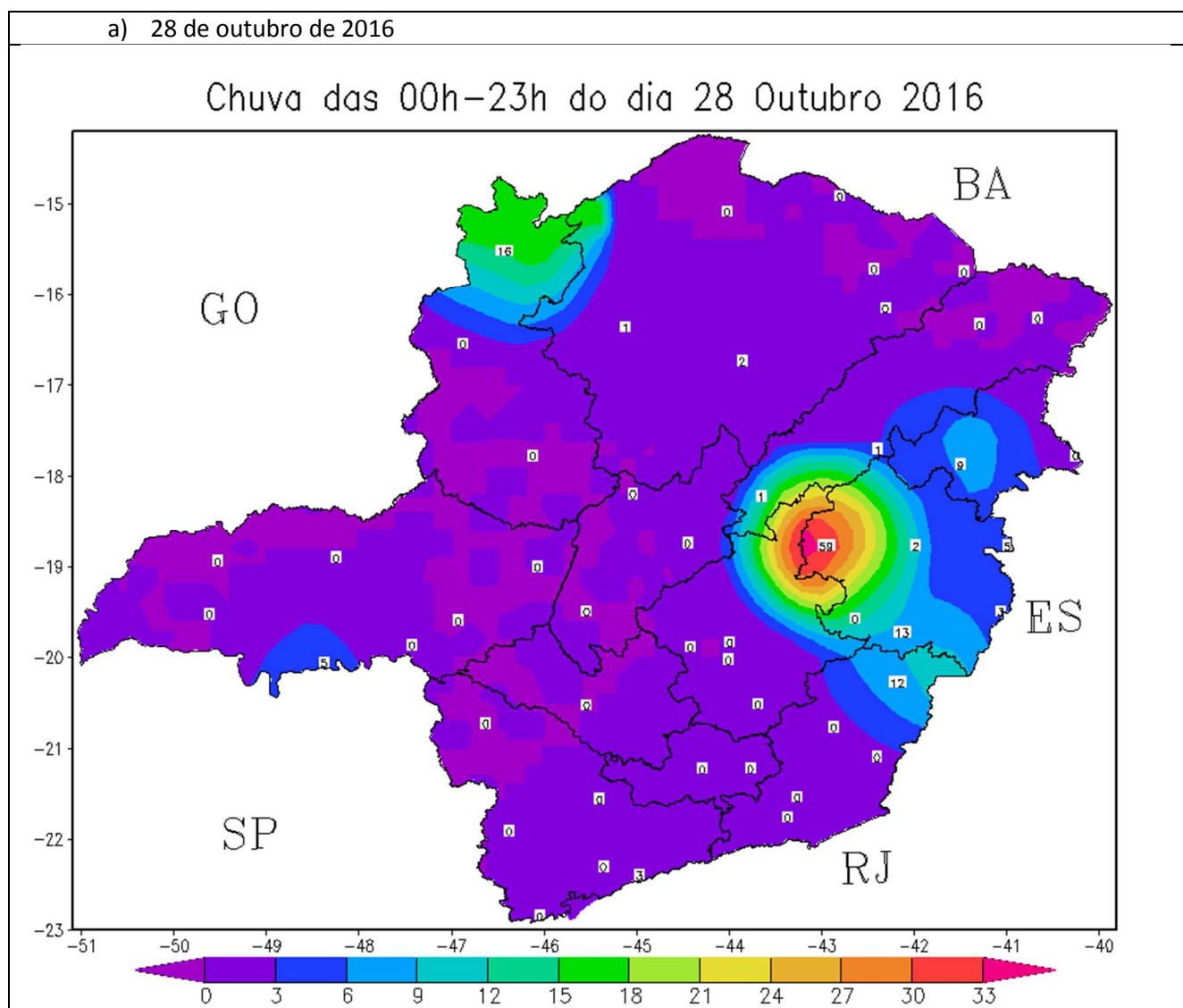
Figura 2 – Acumulado de precipitação (mm) nos dias 28 e 29 de outubro de 2016.
