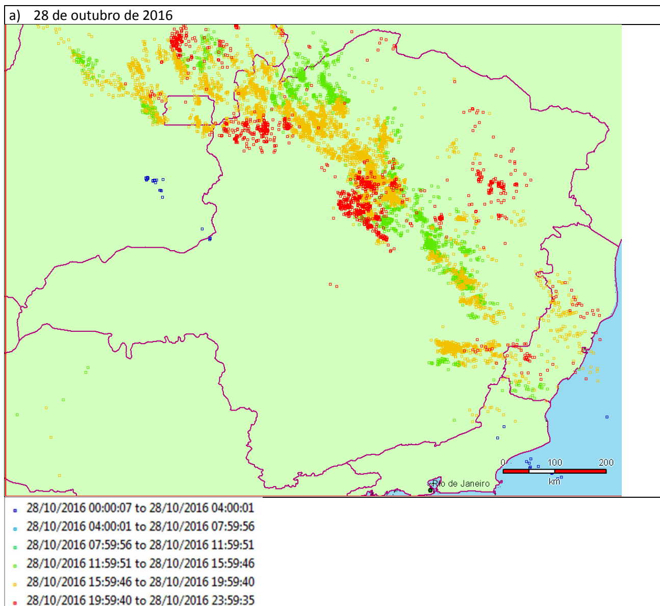
Figura 6 – Descargas atmosféricas registradas em Minas Gerais nos dias 28 e 29 de outubro de 2016.
