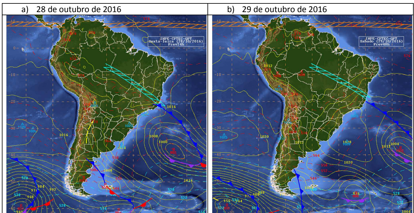
Figura 1 - Cartas Sinóticas elaboradas pelo Centro de Previsão de Tempo e Estudos Climáticos - CPTEC para os dias 28 e 29 de outubro de 2016.
