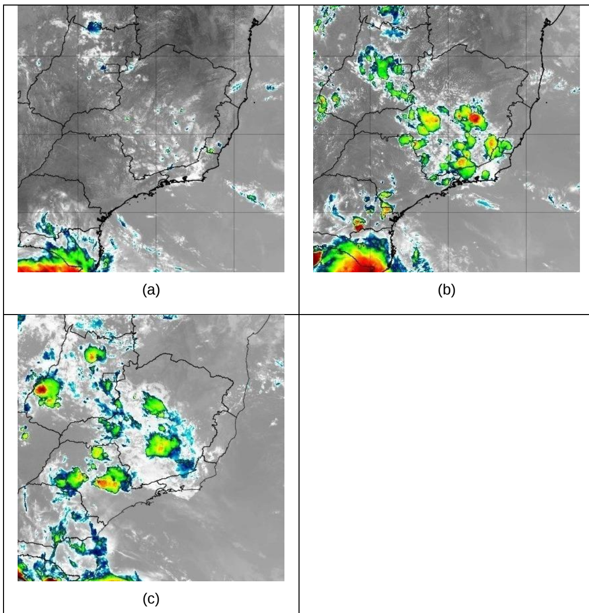
Figura 11 Imagens de Satélite do dia 30/10 as 15:30 (a), 19:00 (b) e (c) 23:00 (h)
