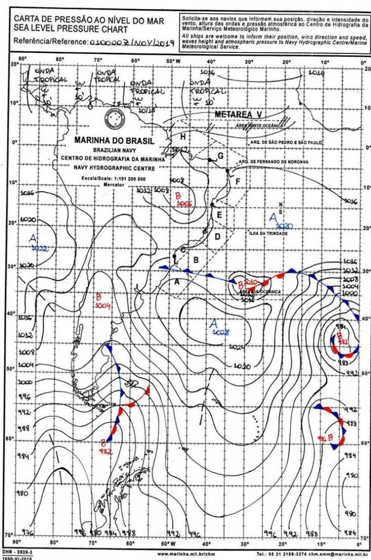
Figura 18 Carta Sinótica do dia 01/11/2019. Fonte: Marinha Brasileira.
