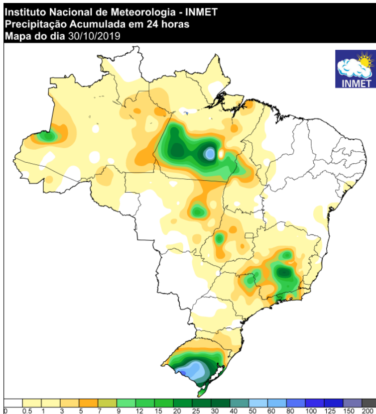
Figura 9 Pluviometria do dia 29/10/2019
