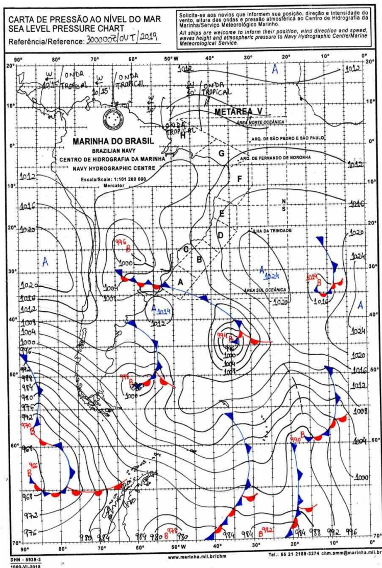
Figura 10 Carta Sinótica do dia 30/10/2019. Fonte: Marinha Brasileira.
