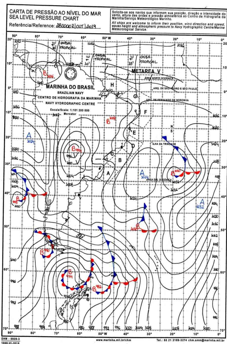
Figura 2 Carta Sinótica do dia 28/10/2019. Fonte: Marinha Brasileira
