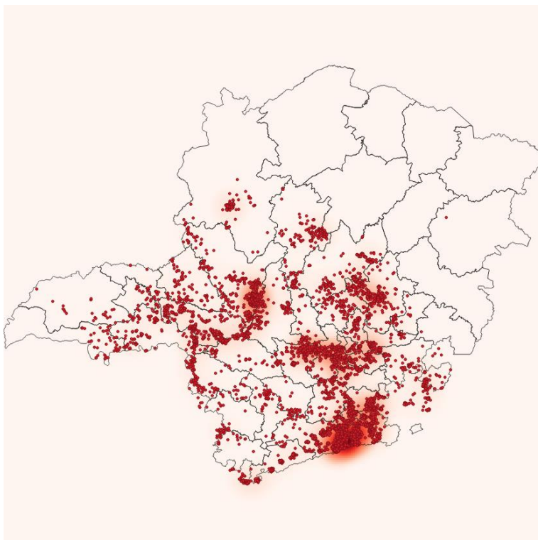
Figura 12 Localização dos raios registrados no dia 30/10/2019
