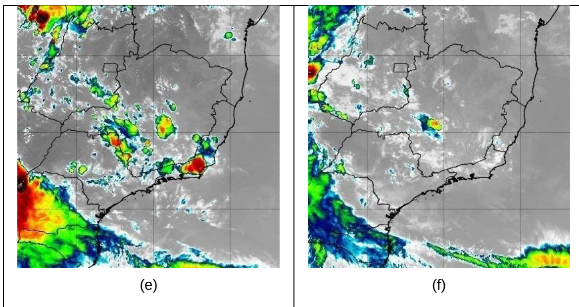
Figura 15 Imagens de Satélite do dia 31/10 as 11:00 (a), 13:00 (b), 15:00 (c), 17:00 (d), 19:00 (e) e 21:00 (f) Estas tempestades levaram a uma quantidade de raios significativa (figura 16) e chuvas no centro-sul de Minas (figura 17).
