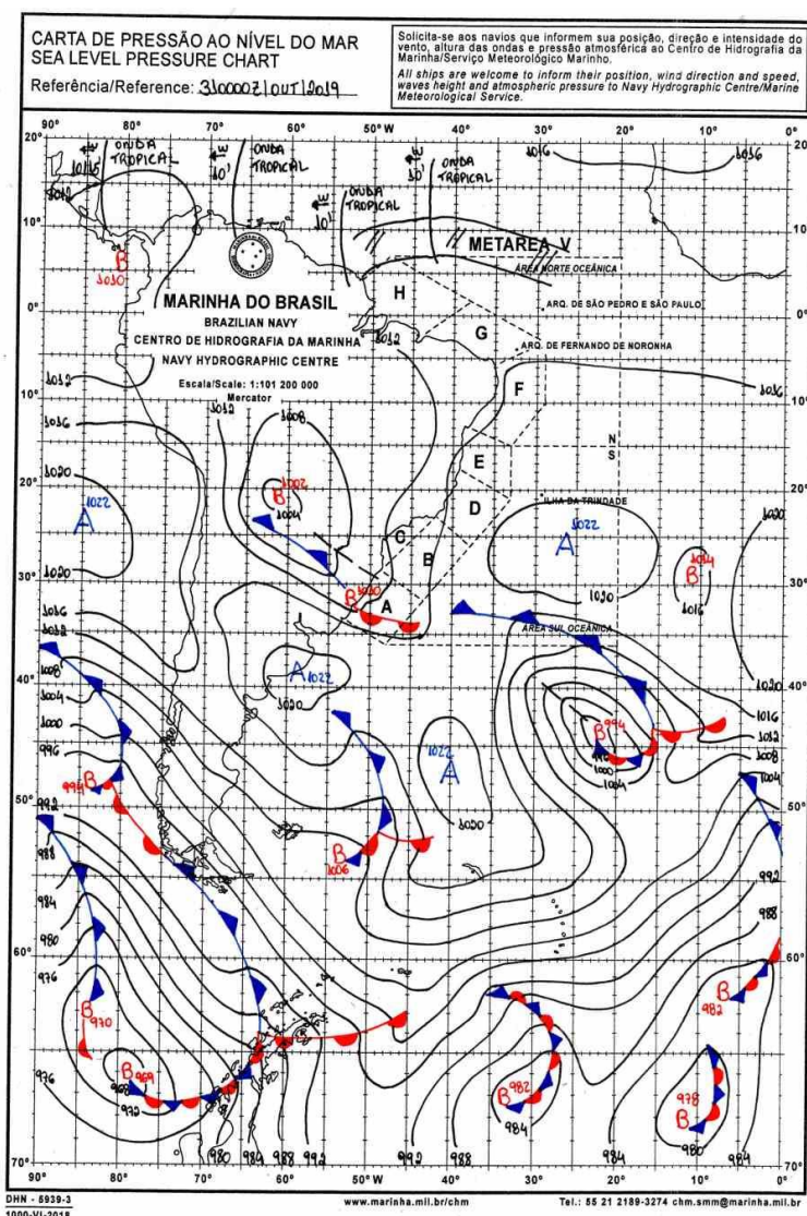
Figura 14 Carta Sinótica do dia 31/10/2019. Fonte: Marinha Brasileira.
