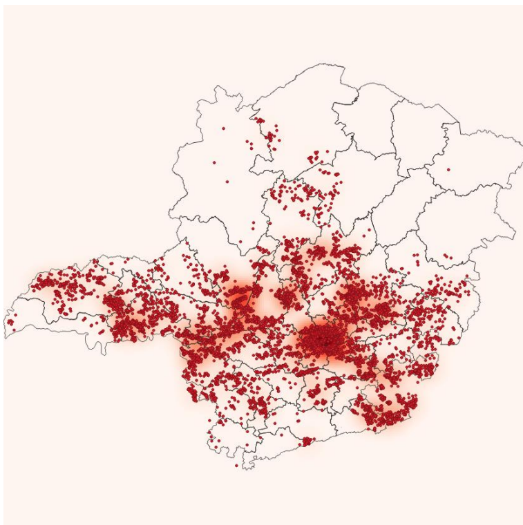
Figura 20 Localização dos raios registrados no dia 01/11/2019
