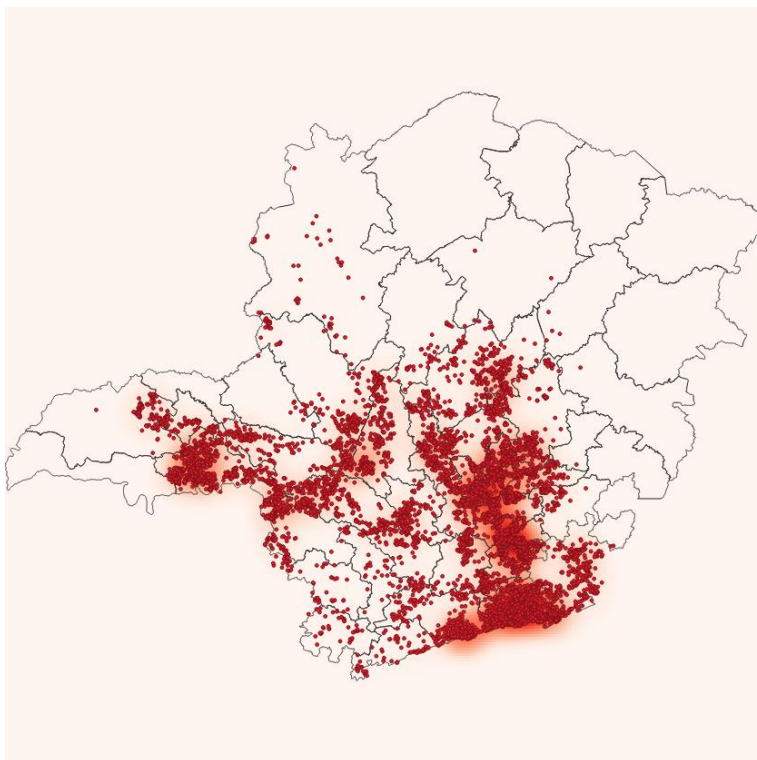
Figura 8 Localização dos raios registrados no dia 29/10/2019
