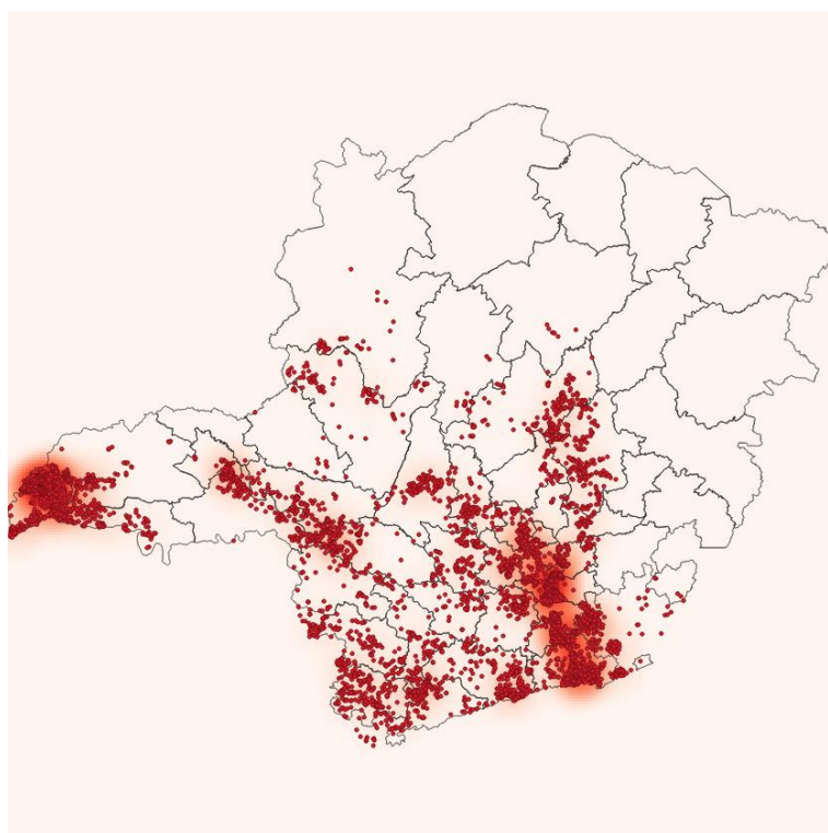
Figura 4 Localização dos raios registrados no dia 28/10/2019.
