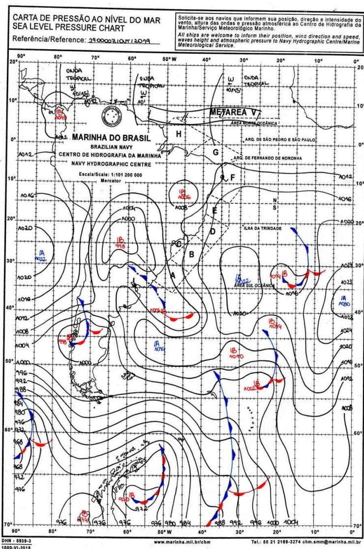
Figura 6 Carta Sinótica do dia 29/10/2019. Fonte: Marinha Brasileira.
