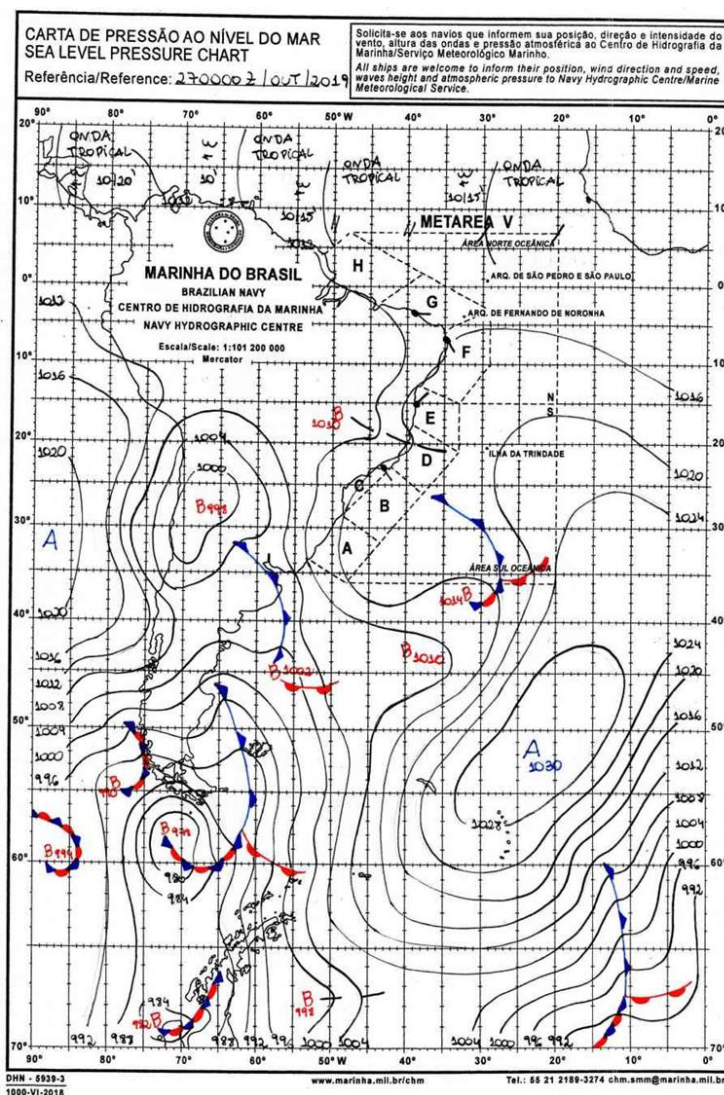
Figura 1 - Carta Sinótica do dia 27/10/2019. Fonte: Marinha Brasileira
