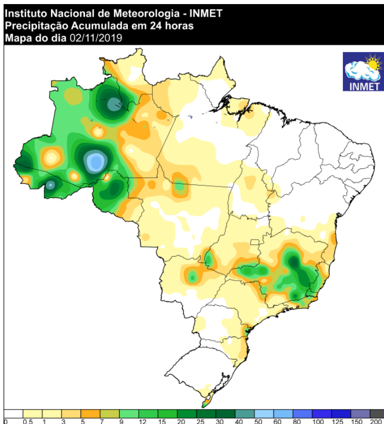
Figura 21 Pluviometria do dia 01/11/2019
