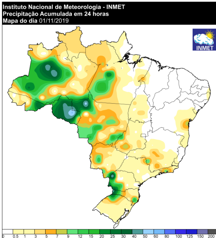
Figura 17 Pluviometria do dia 31/10/2019
