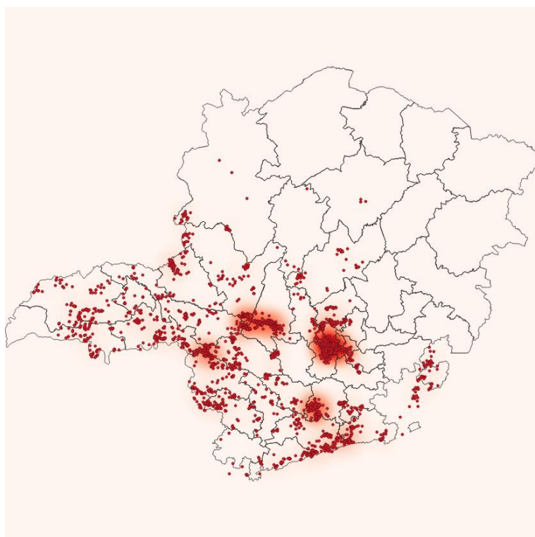
Figura 16 Localização dos raios registrados no dia 31/10/2019
