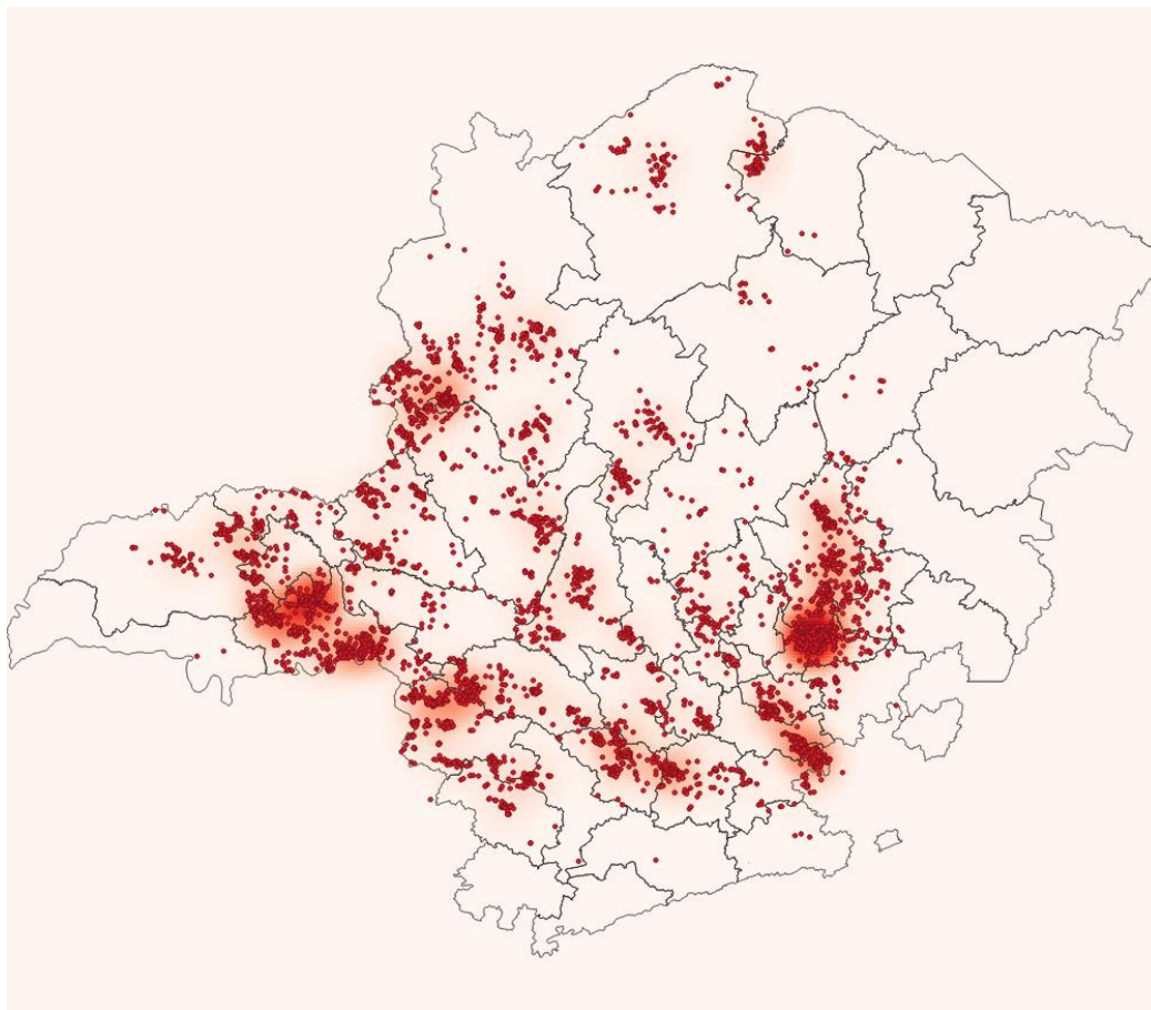
Figura 4 - Raios registrados no dia 28/11/2019. Fonte: RINDAT.
