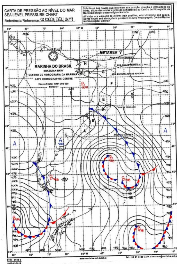
Figura 22 - Carta Sinótica do Dia 02/12/2019. Fonte: Marinha Brasileira.
