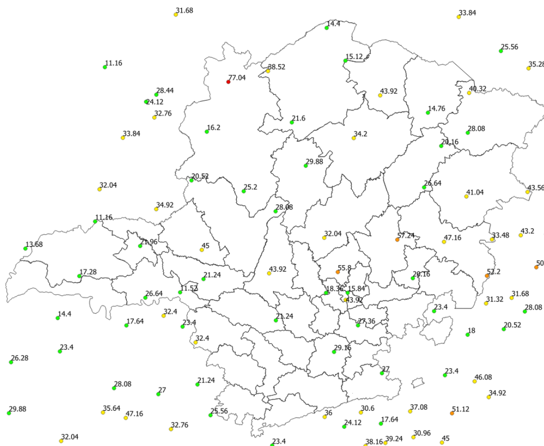
Figura 25 - Rajadas de vento registradas no dia 02/12/2019. Fonte: INMET.
