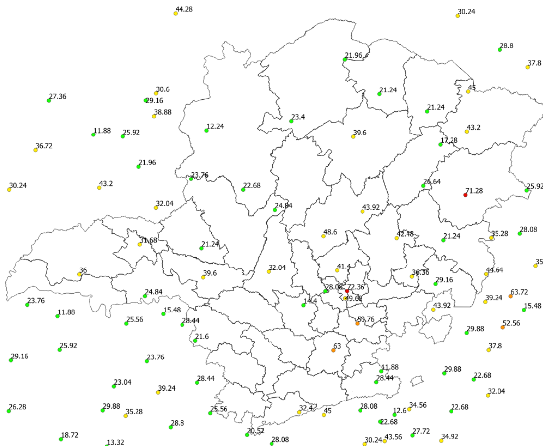
Figura 20 - Rajadas de vento registradas no dia 01/12/2019. Fonte: INMET.
