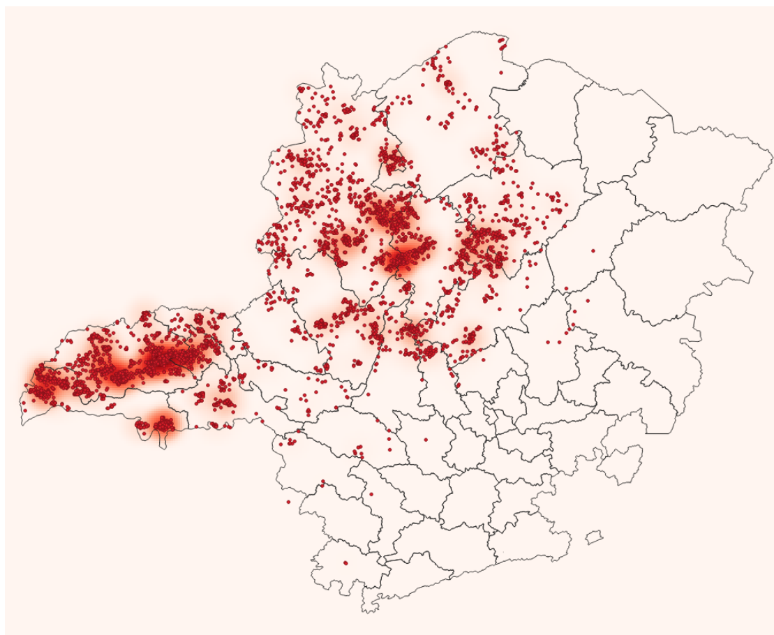
Figura 28 - Raios registrados no dia 03/12/2019. Fonte: RINDAT.
