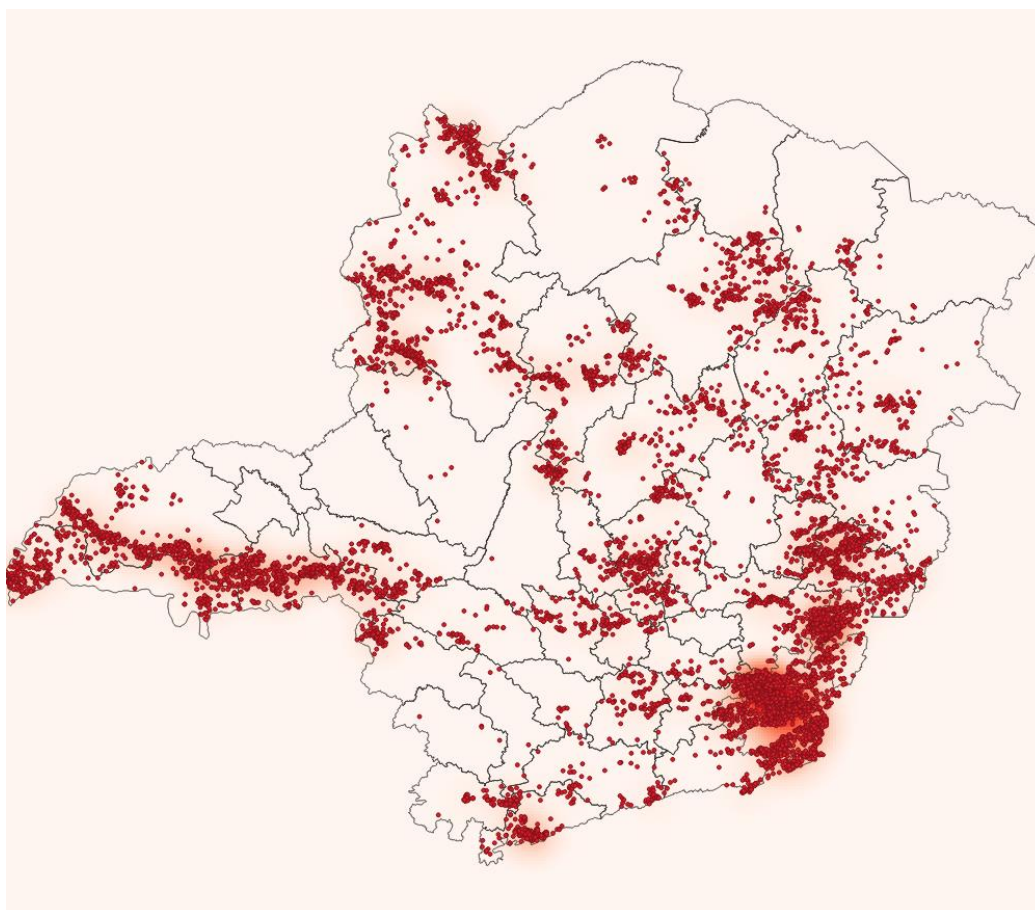
Figura 19 - Raios registrados no dia 01/12/2019. Fonte: RINDAT.
