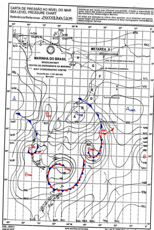
Figura 7 - Carta Sinótica do Dia 29/11/2019. Fonte: Marinha Brasileira.
