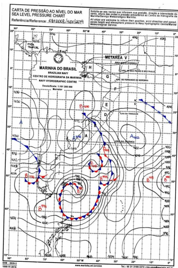
Figura 2 - Carta Sinótica do Dia 28/11/2019. Fonte: Marinha Brasileira.
