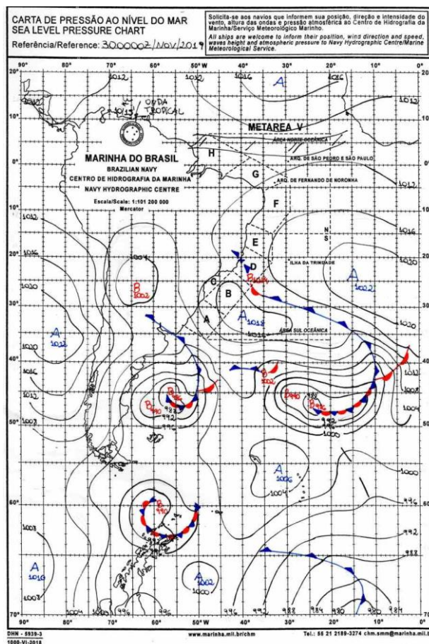
Figura 12 - Carta Sinótica do Dia 30/11/2019. Fonte: Marinha Brasileira.
