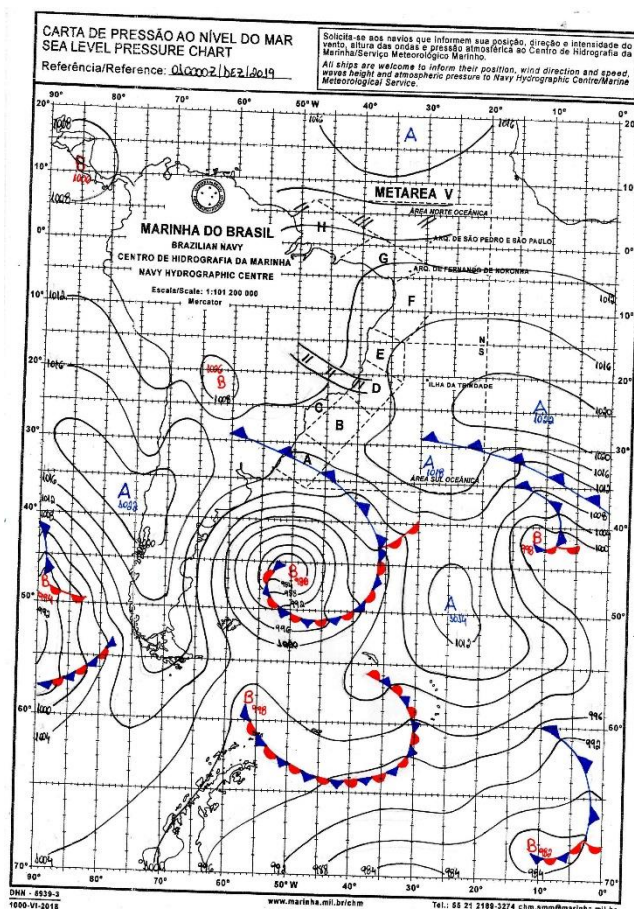
Figura 17 - Carta Sinótica do Dia 01/12/2019. Fonte: Marinha Brasileira.
