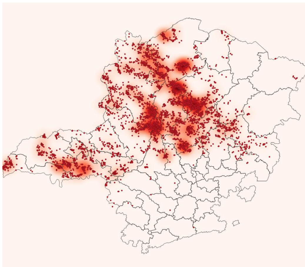
Figura 9 - Raios registrados no dia 29/11/2019. Fonte: RINDAT.
