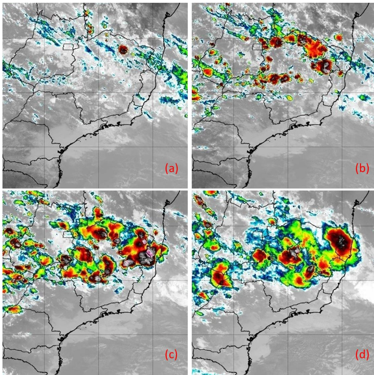
Figura 23 - Imagens do satélite GOES-16 do dia 02/12/2019 as 12:00 (a), 15:00 (b), 18:00 (c) e 21:00 horas local. Fonte: INPE.
