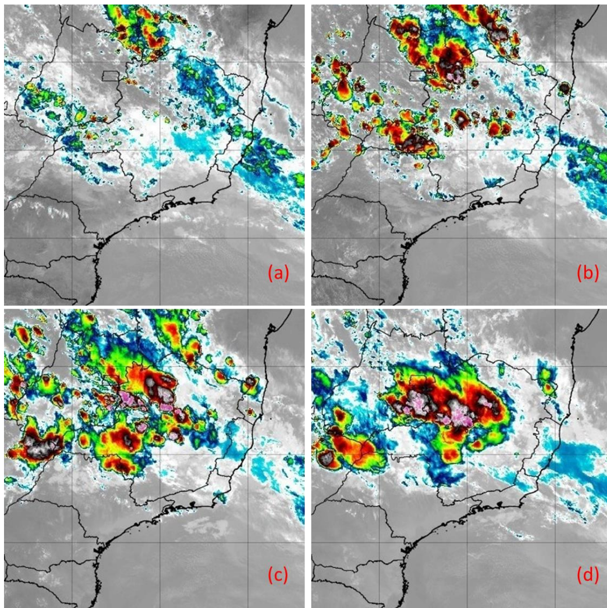
Figura 8 - Imagens do satélite GOES-16 do dia 29/11/2019 as 12:00 (a), 15:00 (b), 18:00 (c) e 21:00 horas local. Fonte: INPE.
