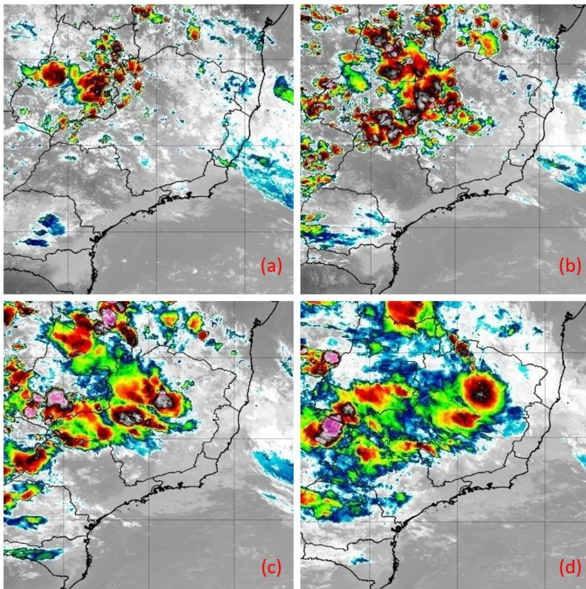
Figura 278 - Imagens do satélite GOES-16 do dia 03/12/2019 as 12:00 (a), 15:00 (b), 18:00 (c) e 21:00 horas local. Fonte: INPE.
