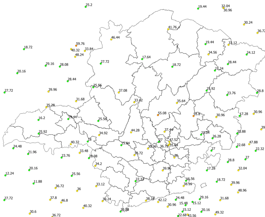
Figura 5 - Rajadas de vento registradas no dia 28/11/2019. Fonte: INMET.
