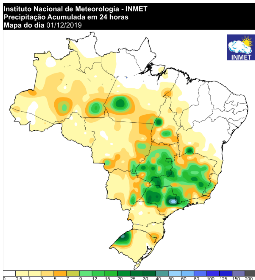
Figura 16 - Precipitação ocorrida no dia 30/11/2019. Fonte: INMET.
