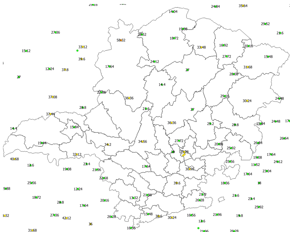
Figura 30 - Rajadas de vento registradas no dia 03/12/2019. Fonte: INMET.
