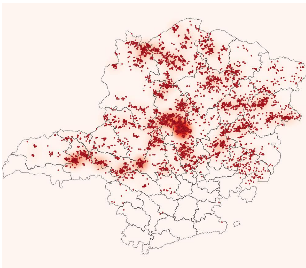
Figura 24 - Raios registrados no dia 02/12/2019. Fonte: RINDAT.
