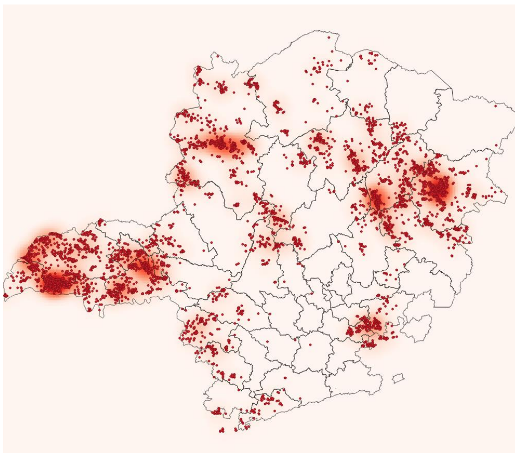
Figura 14 - Raios registrados no dia 30/11/2019. Fonte: RINDAT.
