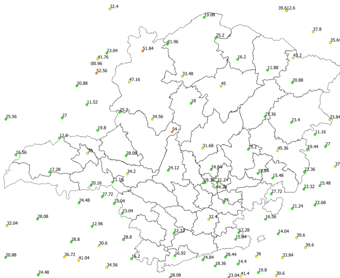
Figura 10 - Rajadas de vento registradas no dia 29/11/2019. Fonte: INMET.
