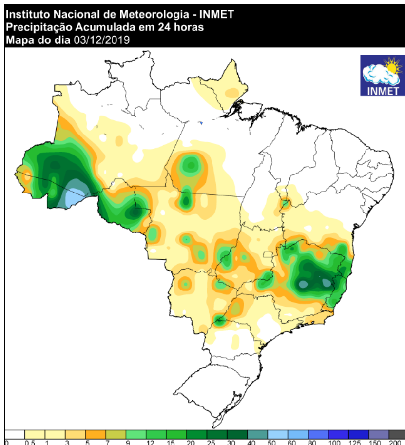
Figura 26 - Precipitação ocorrida no dia 02/12/2019. Fonte: INMET.
