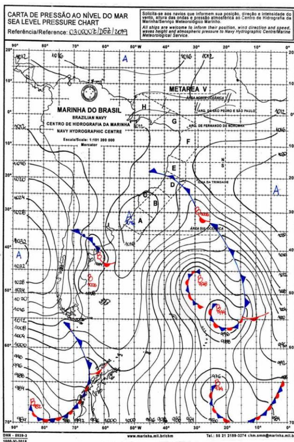
Figura 27 - Carta Sinótica do Dia 03/12/2019. Fonte: Marinha Brasileira.
