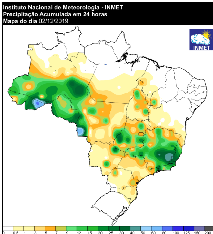
Figura 21 - Precipitação ocorrida no dia 01/12/2019. Fonte: INMET.
