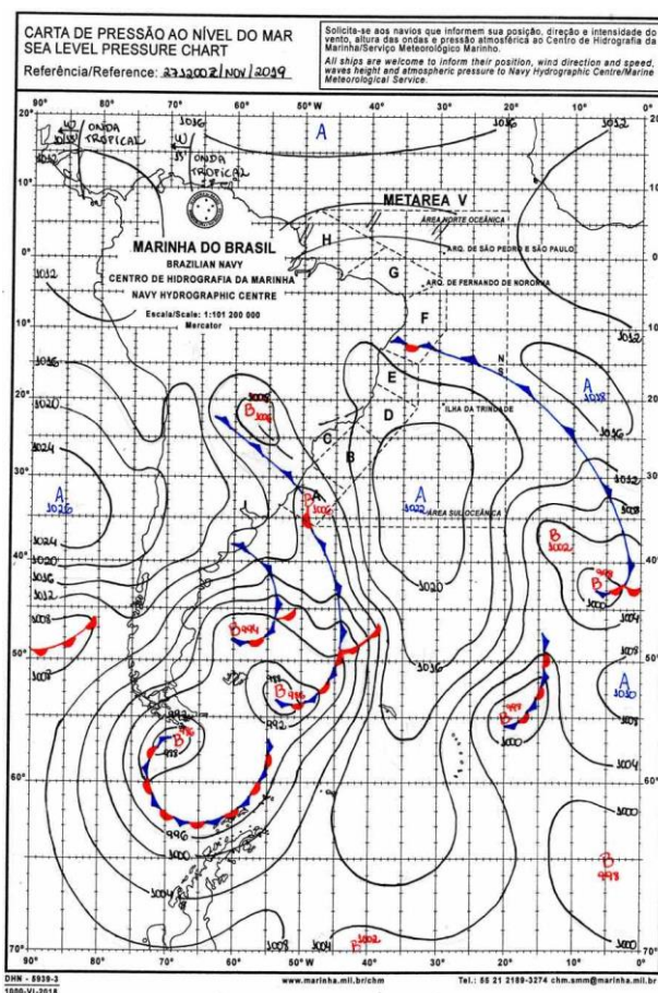
Figura 1 - Carta Sinótica do Dia 27/11/2019. Fonte: Marinha Brasileira.
