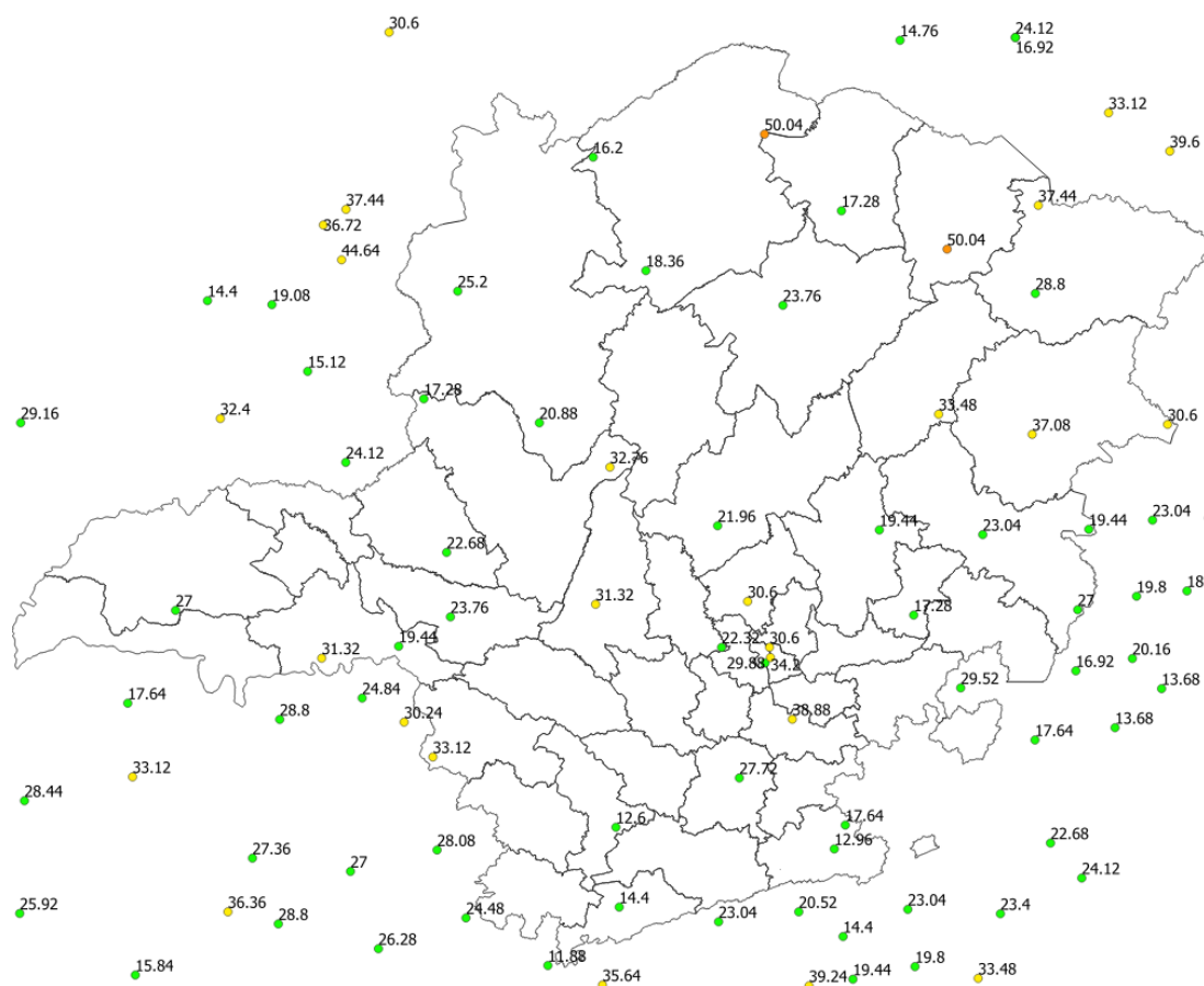
Figura 15 - Rajadas de vento registradas no dia 30/11/2019. Fonte: INMET.
