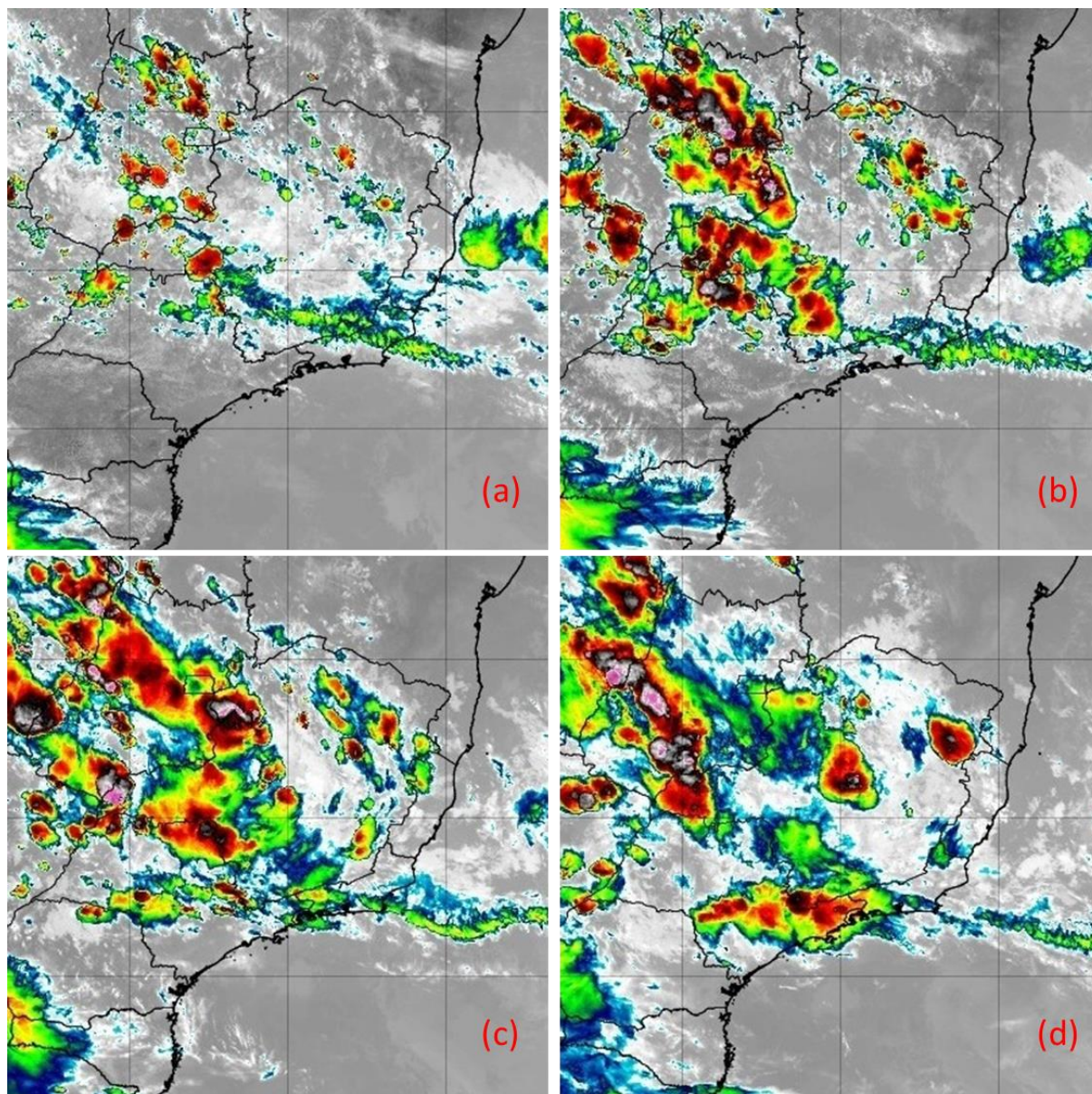
Figura 13 - Imagens do satélite GOES-16 do dia 30/11/2019 as 12:00 (a), 15:00 (b), 18:00 (c) e 21:00 horas local. Fonte: INPE.
