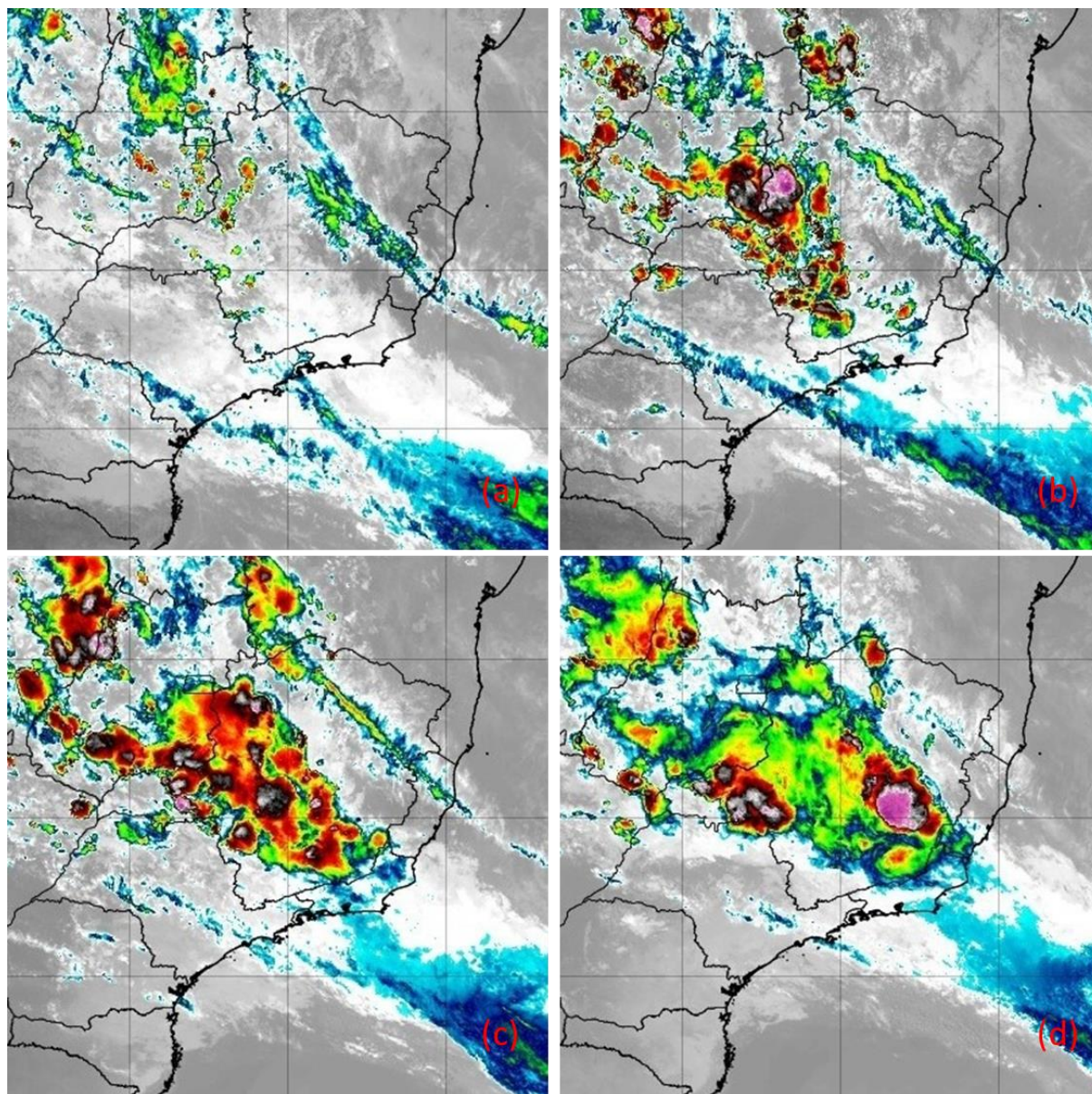
Figura 3 - Imagens do satélite GOES-16 do dia 28/11/2019 as 12:00 (a), 15:00 (b), 18:00 (c) e 21:00 horas local. Fonte: INPE.
