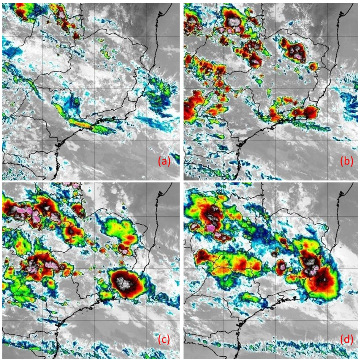
Figura 18 - Imagens do satélite GOES-16 do dia 01/12/2019 as 12:00 (a), 15:00 (b), 18:00 (c) e 21:00 horas local. Fonte: INPE.
