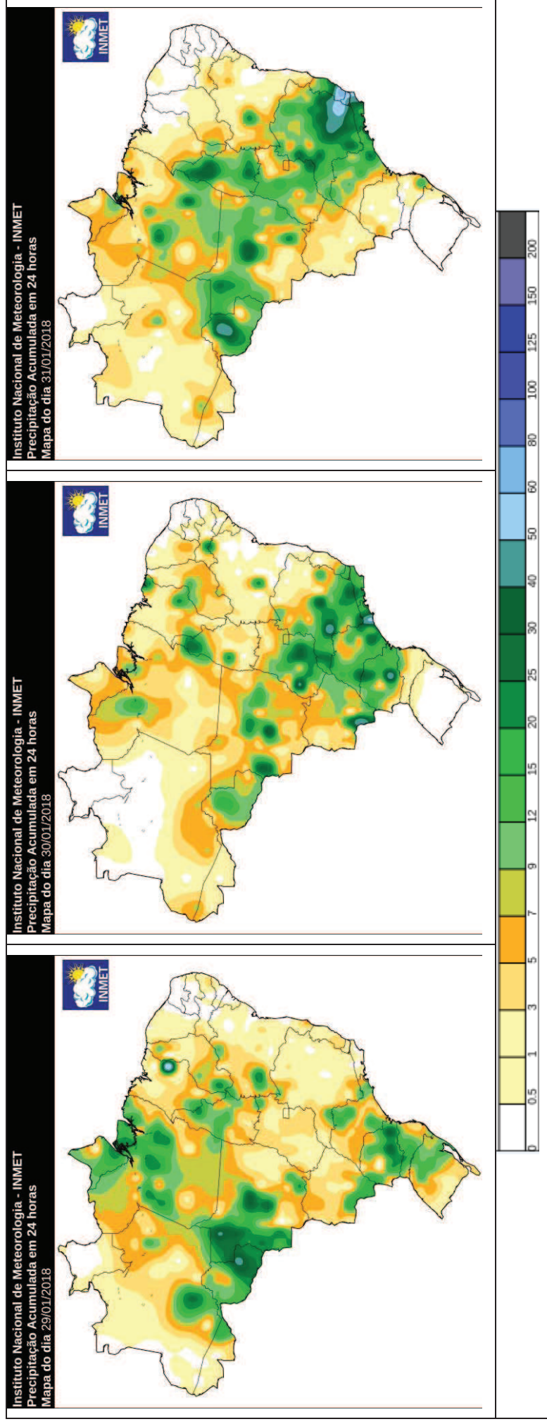
Figura 2 - Acumulado de precipitação (mm) nos dias 29, 30 e 31 de janeiro de 2018.
