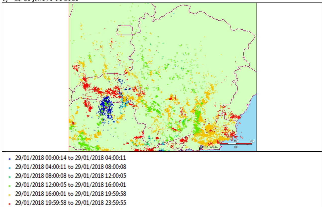
Figura 4 – Descargas atmosféricas registradas em Minas Gerais nos dias 29, 30 e 31 de janeiro de 2018.
