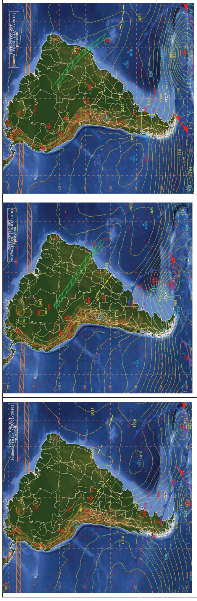
Figura 1 - Cartas Sinóticas elaboradas pelo Centro de Previsão de Tempo e Estudos Climáticos para os dias 29, 30 e 31 de janeiro de 2018.
