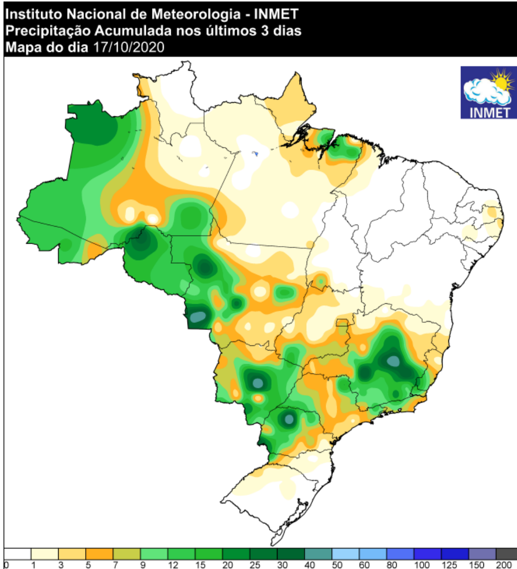
Figura 5 - Pluviometria acumulada dos dias 14, 15 e 16 de outubro de 2020.
