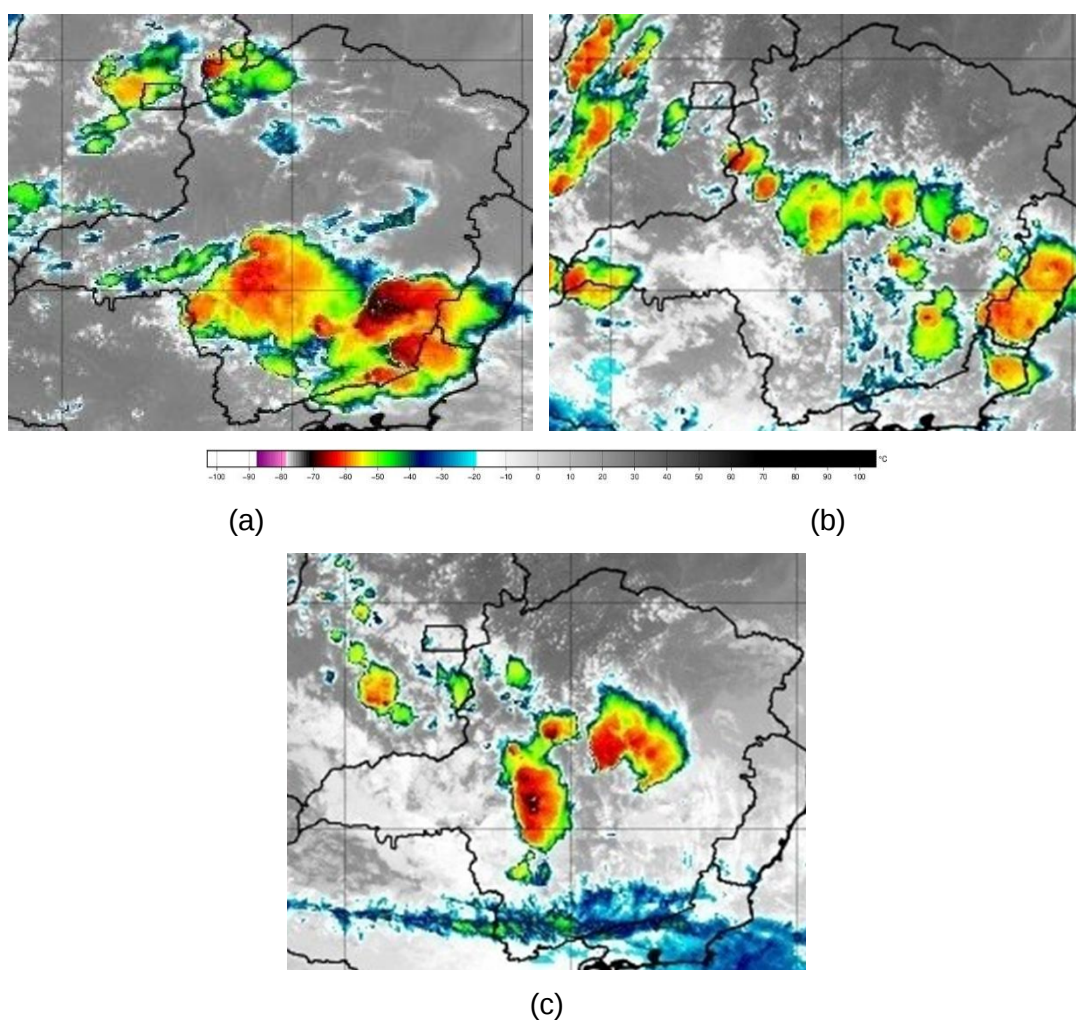
Figura 2 – Exemplo de Imagem de Satélite dos dias 14 (a), 15 (b) e 16 (c) de outubro de 2020. Fonte: INPE.
