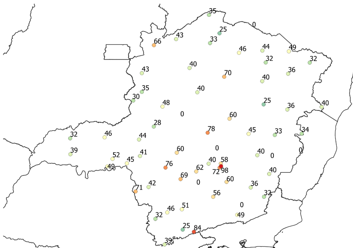
Figura 4 – Rajadas de vento máximas registradas entre os dias 14 e 16 de outubro de 2020. Fonte: INMET
