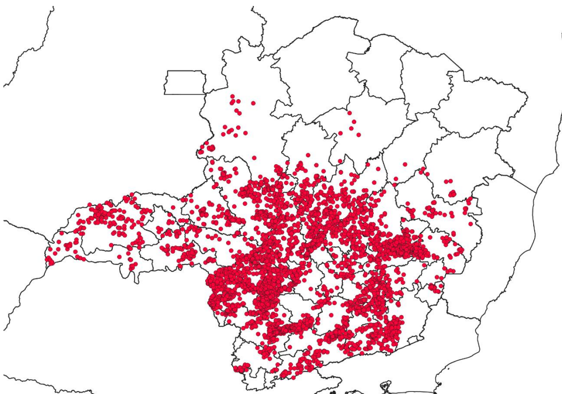
Figura 3 - Localização dos raios registrados entre os dias 14 e 16 de outubro de 2020. Fonte: RINDAT
