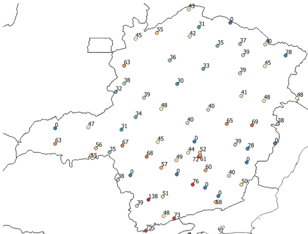
Figura 4 – Rajadas de vento máximas registradas entre os dias 16 e 18 de novembro de 2020. Fonte: INMET
