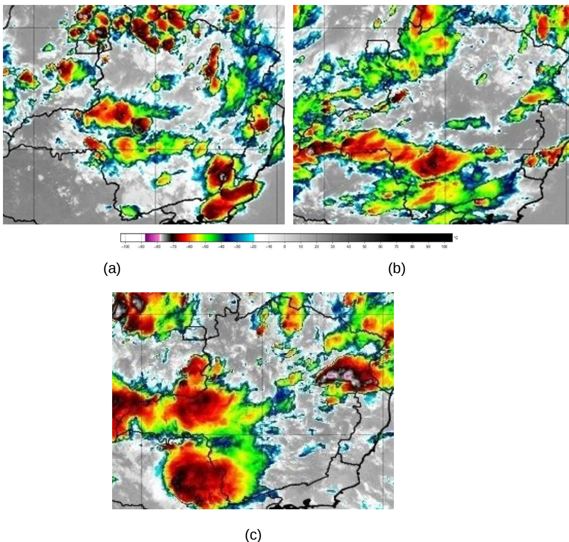
Figura 2 – Exemplo de Imagem de Satélite dos dias 16 (a), 17 (b) e 18 (c) de novembro de 2020. Fonte: INPE.
