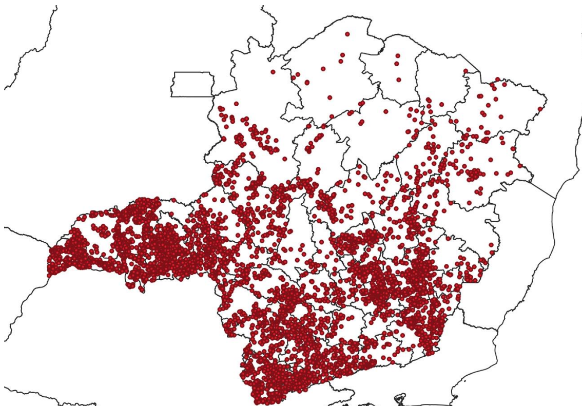
Figura 3 - Localização dos raios registrados entre os dias 16 e 18 de novembro de 2020. Fonte: RINDAT
