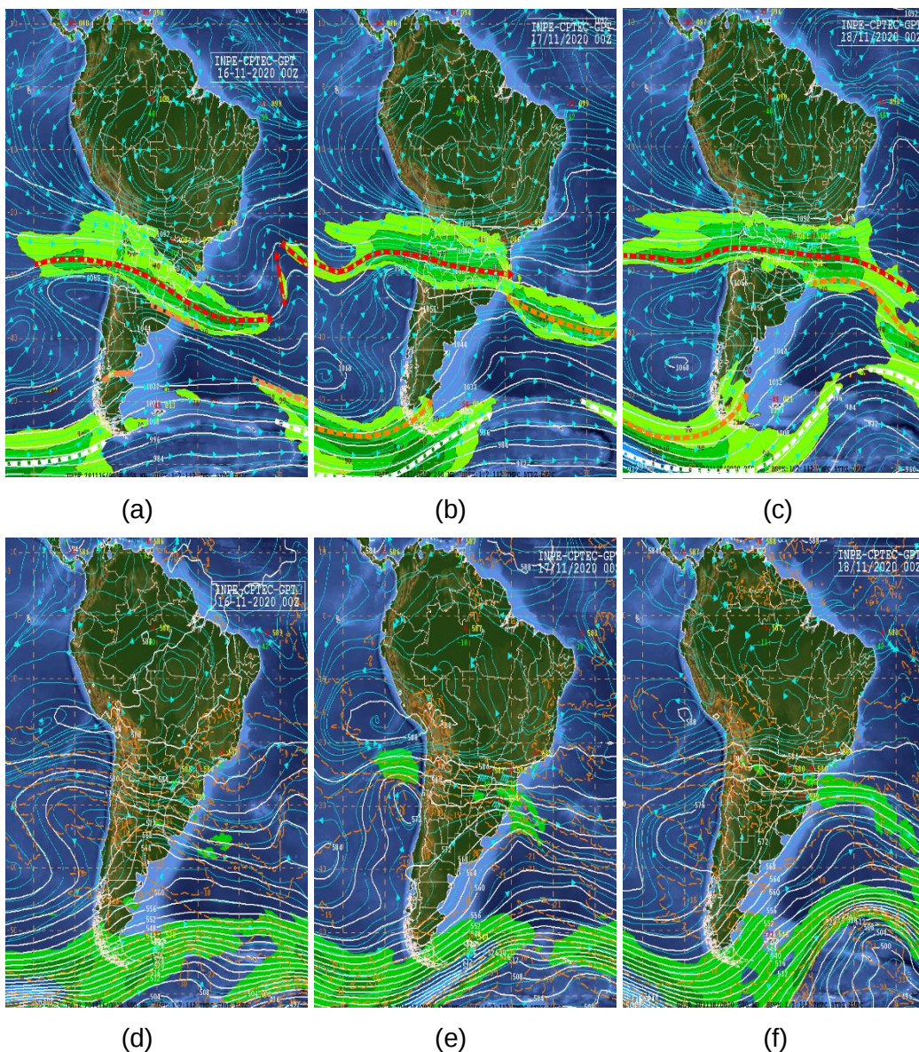
Figura 1 - Carta Sinótica dos dias 16, 17 e 18 em 250 hPa (a), (b) e (c) e em 500 hPa (d), (e) e (f), respectivamente. Fonte: CPTEC/INPE.
