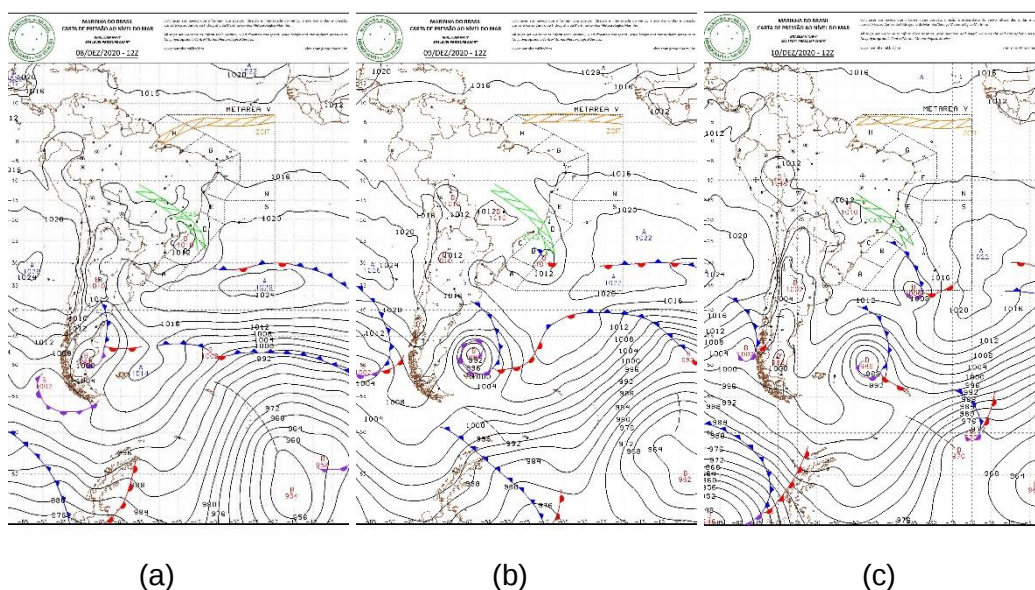
Figura 1 - Carta Sinótica dos dias 08, 09 e 10 de dezembro de 2020 (a), (b) e (c), respectivamente. Fonte: Marinha Brasileira.
