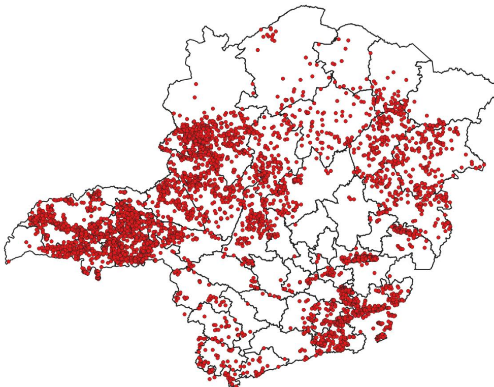
Figura 3 - Localização dos raios registrados entre os dias 08 e 10 de dezembro de 2020. Fonte: RINDAT
