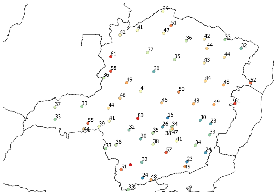
Figura 4 – Rajadas de vento máximas registradas entre os dias 08 e 10 de dezembro de 2020. Fonte: INMET
