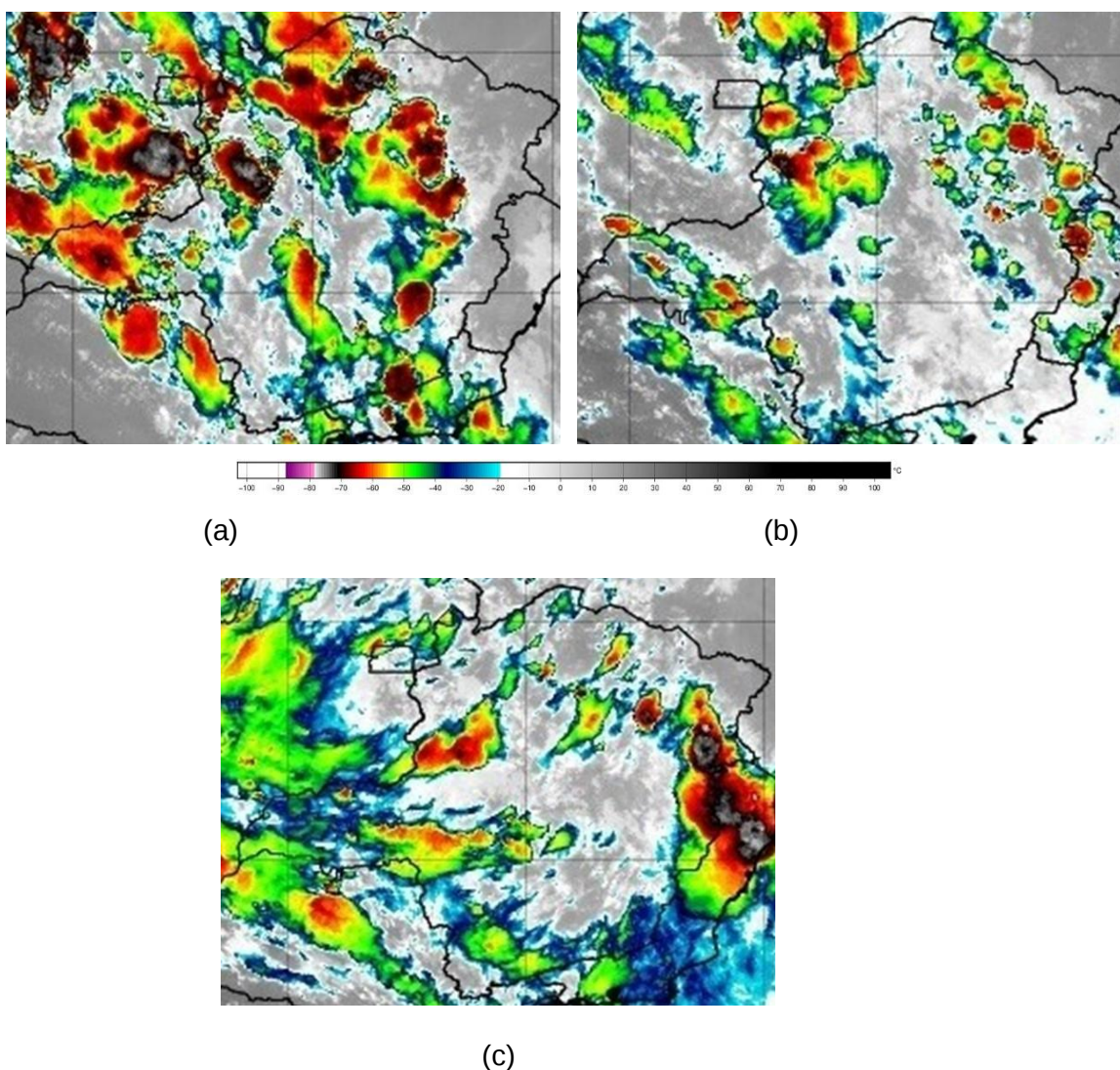
Figura 2 – Exemplo de Imagem de Satélite dos dias 08 (a), 09 (b) e 10 (c) de dezembro de 2020 as 19:00 UTC. Fonte: INPE.
