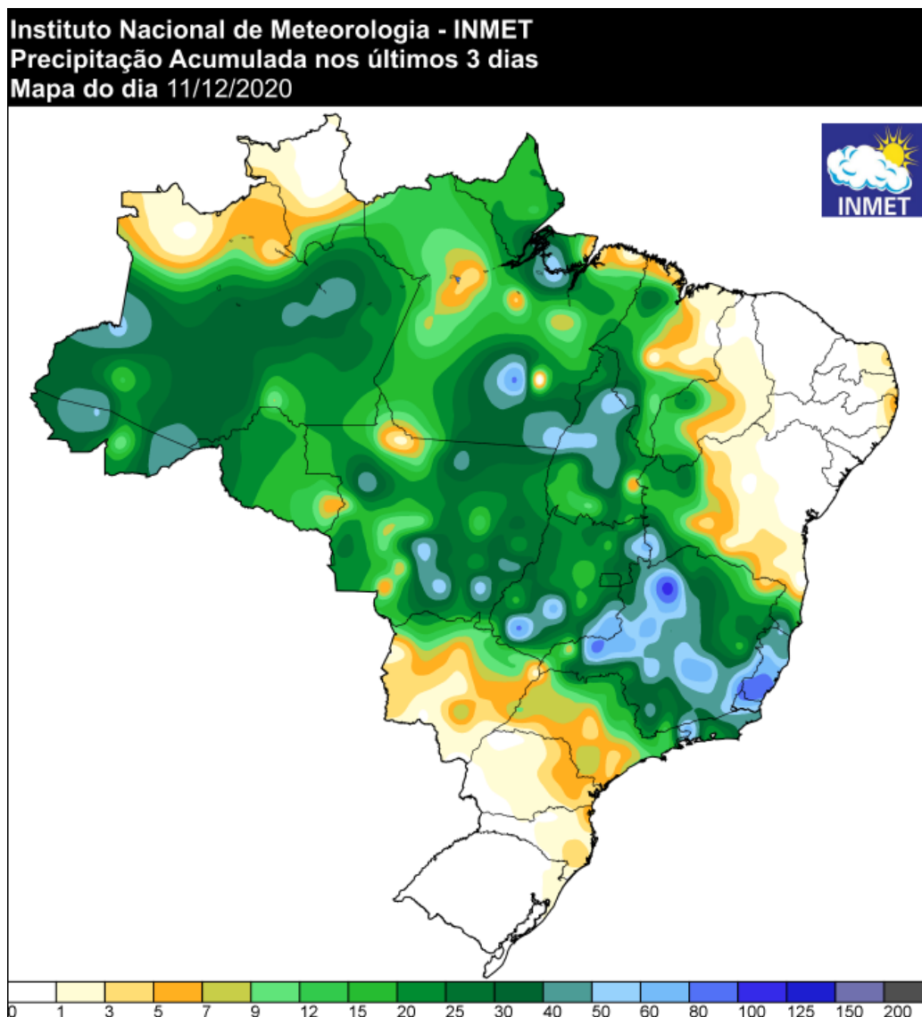
Figura 5 - Pluviometria acumulada dos dias 08, 09 e 10 de dezembro de 2020.
