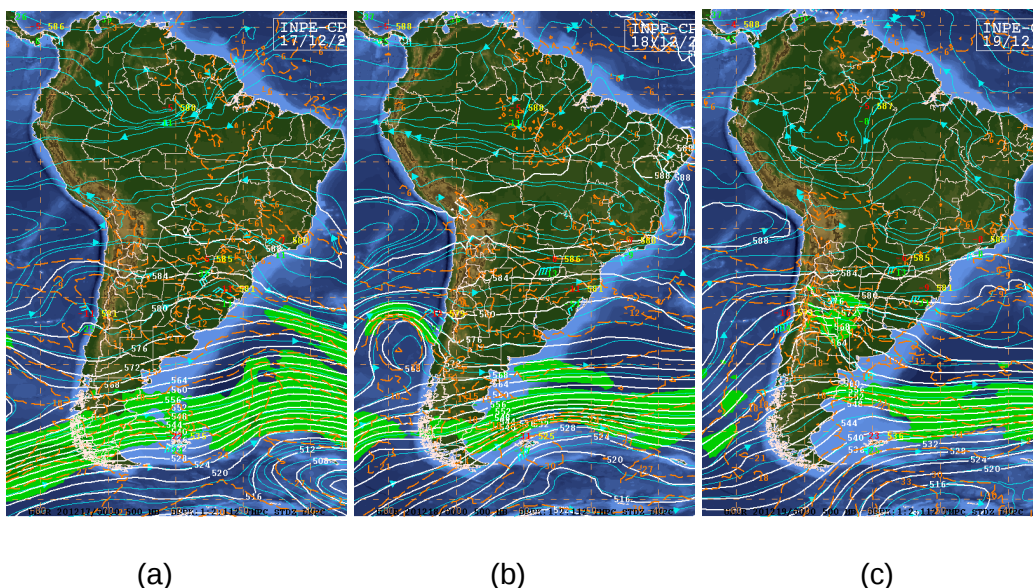
Figura 1 - Carta Sinótica dos dias 17, 18 e 19 de dezembro de 2020 em 500 hPa (a), (b) e (c), respectivamente. Fonte: CPTEC/INPE.
