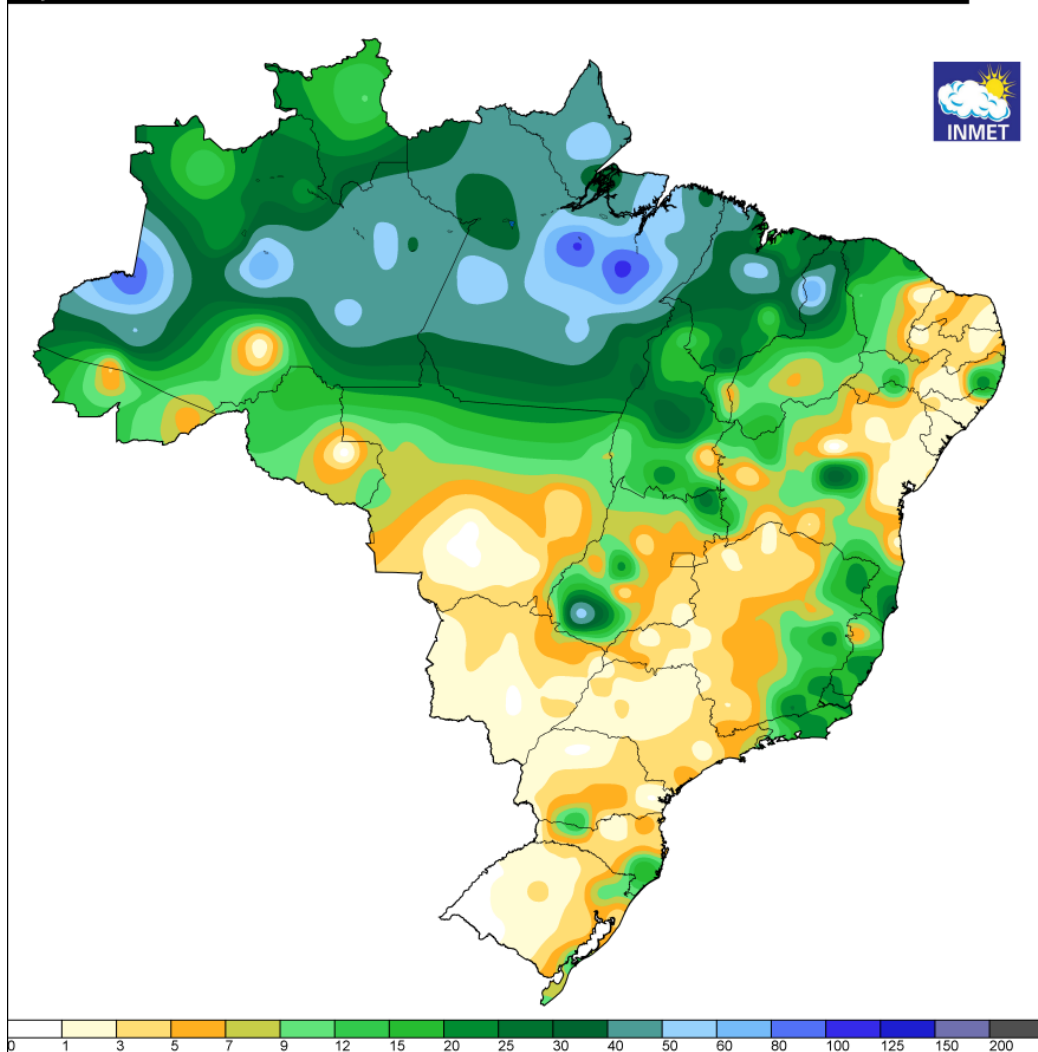
Figura 5 - Pluviometria acumulada dos dias 30 e 31 de março e 01 de abril de 2021.
