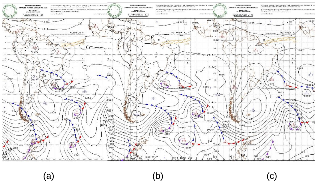
Figura 1 - Cartas Sinóticas em superfície dos dias 30 e 31 de março e 01 de abril de 2021 (a), (b) e (c), respectivamente. Fonte: Marinha do Brasil.
