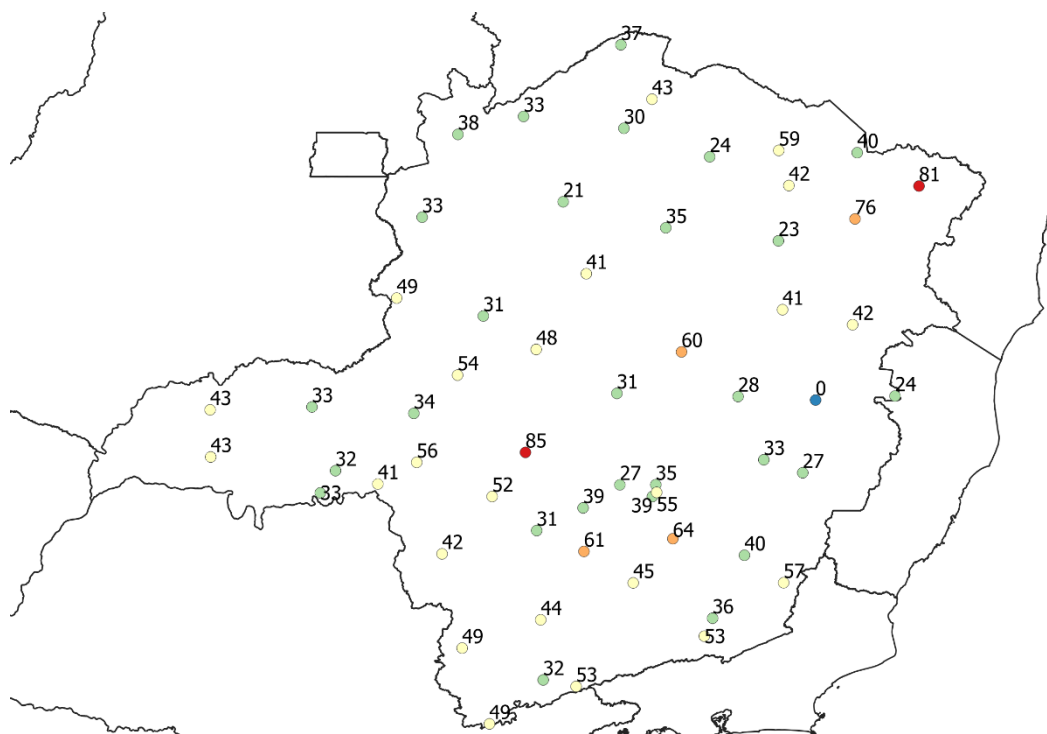
Figura 4 – Rajadas de vento máximas registradas entre os dias 30 e 31 de março e 01 de abril de 2021. Fonte: INMET
