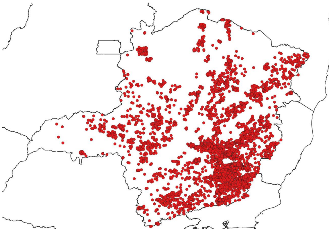
Figura 3 - Localização dos raios registrados entre os dias 30 e 31 de março e 01 de abril de 2021. Fonte: RINDAT
