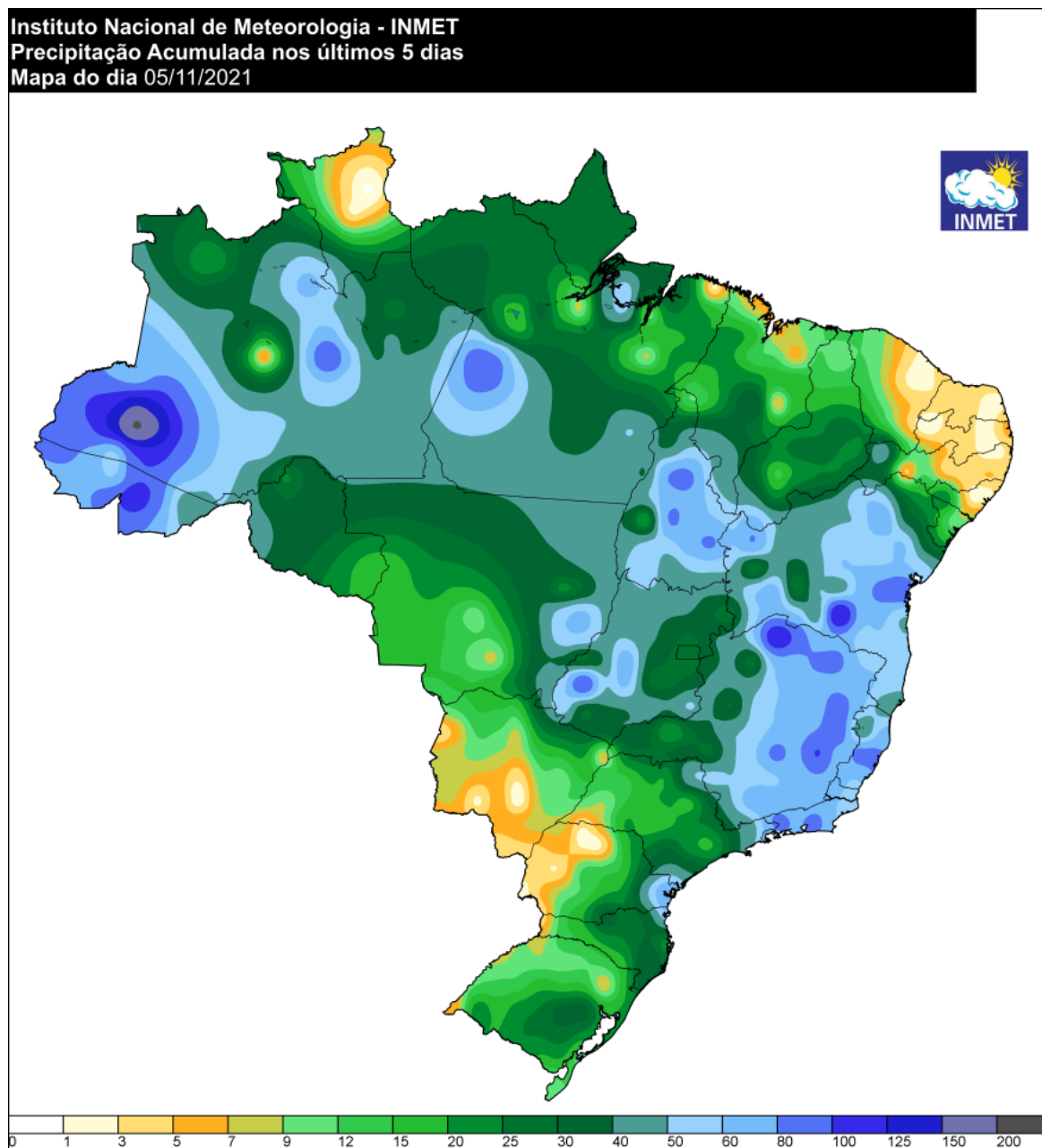
Figura 5a - Pluviometria acumulada dos dias 31/10 e 04 de novembro de 2021.
