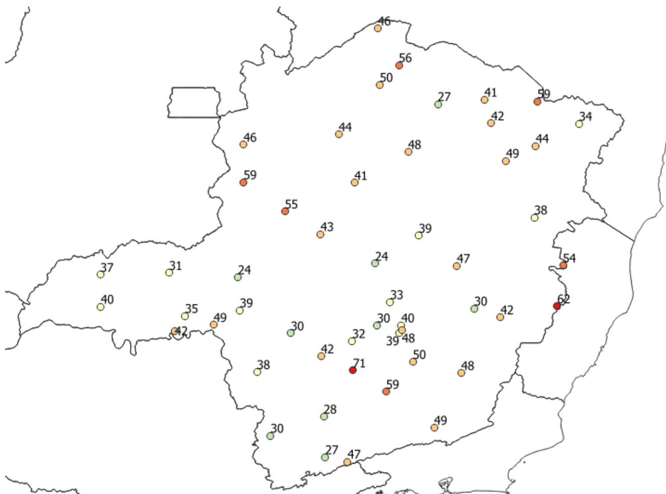
Figura 4 – Rajadas de vento máximas registradas entre os dias 01 e 04 de novembro de 2021. Fonte: INMET
