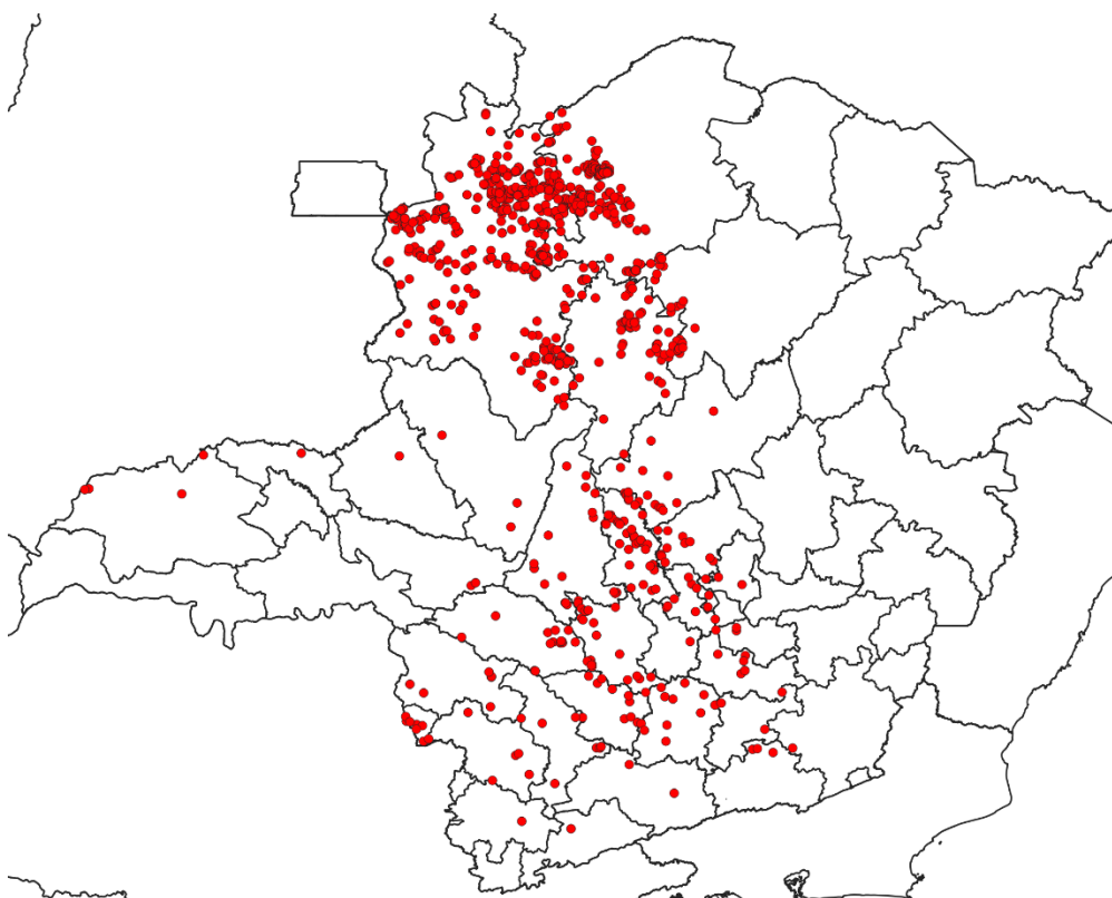
Figura 3 - Localização dos raios registrados entre os dias 01 e 04 de novembro de 2021. Fonte: RINDAT
