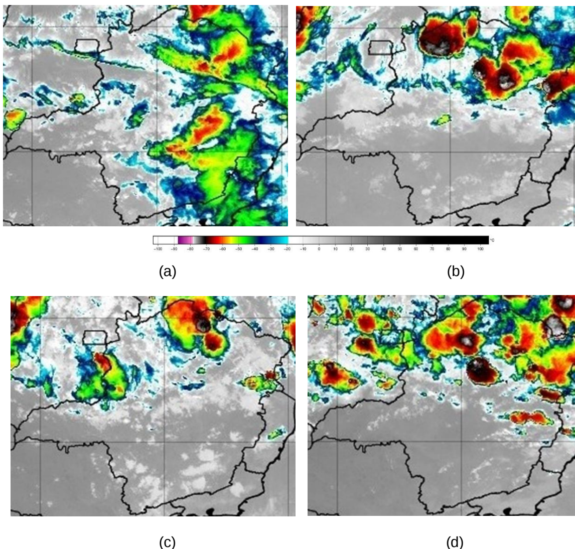
Figura 2 – Seleção de Imagem de Satélite dos dias 01/11 as 18:00 (a), 02/11 as 20:00 (b), 03/11 as 18:00 (c) e 04/11 as 18:00 de novembro de 2021 (Horário Local). Fonte: INPE.
