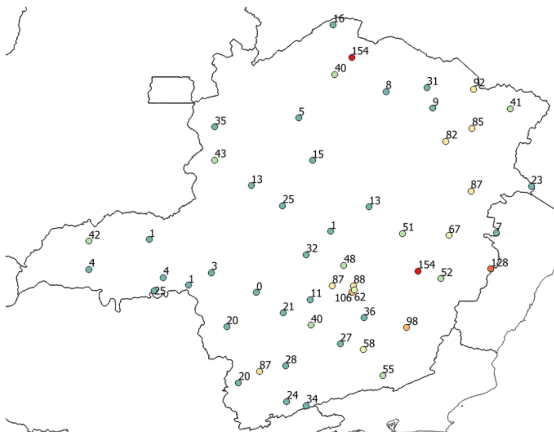
Figura 5b - Pluviometria acumulada dos dias 01 e 04 de novembro de 2021.
