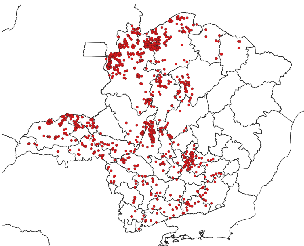
Figura 3 - Localização dos raios registrados entre os dias 01 e 04 de dezembro de 2021. Fonte: RINDAT
