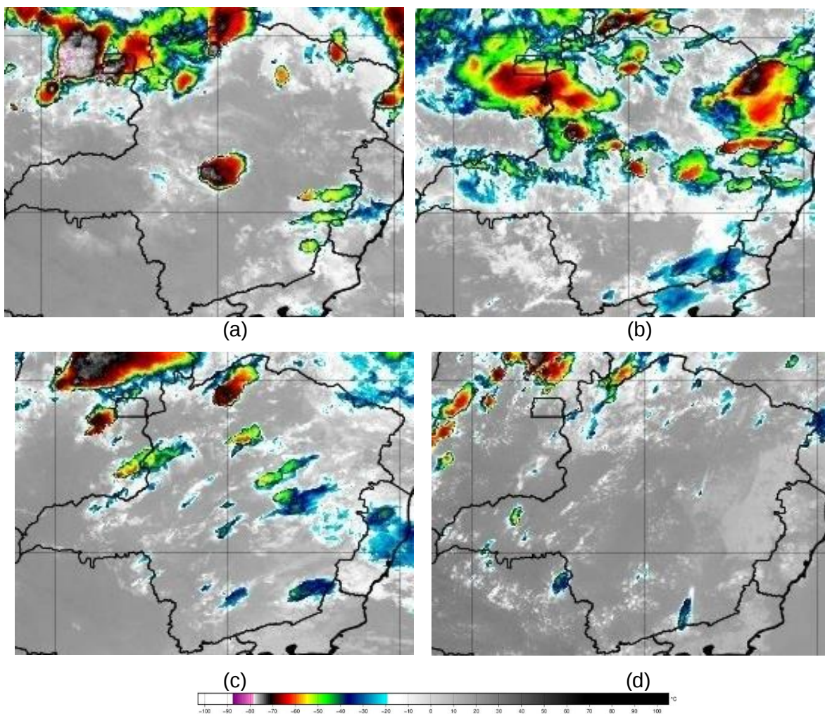
Figura 2 – Seleção de Imagem de Satélite dos dias 01 as 20:00 (a), 02 as 18:00 (b), 03 as 20:00 (c) e 04 as 18:00 de dezembro de 2021 (Horário Local). Fonte: INPE.
