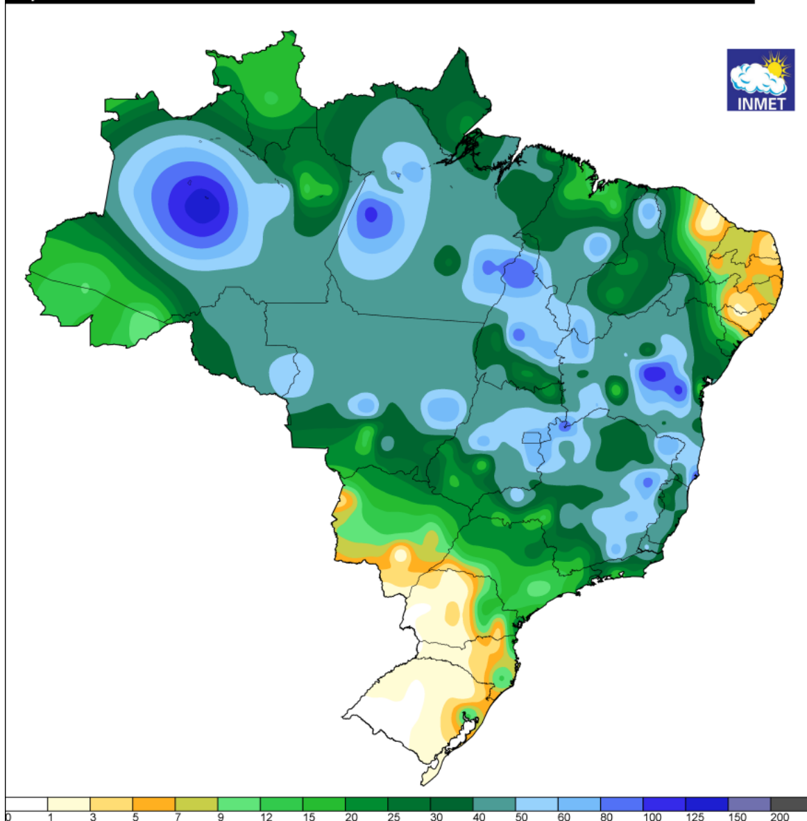
Figura 5a - Pluviometria acumulada entre os dias 30 de novembro e 04 de dezembro de 2021.
