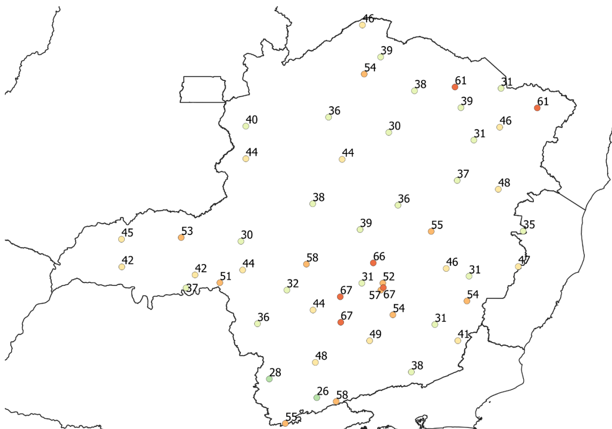
Figura 4 – Rajadas de vento máximas registradas entre os dias 01 e 04 de dezembro de 2021. Fonte: INMET
