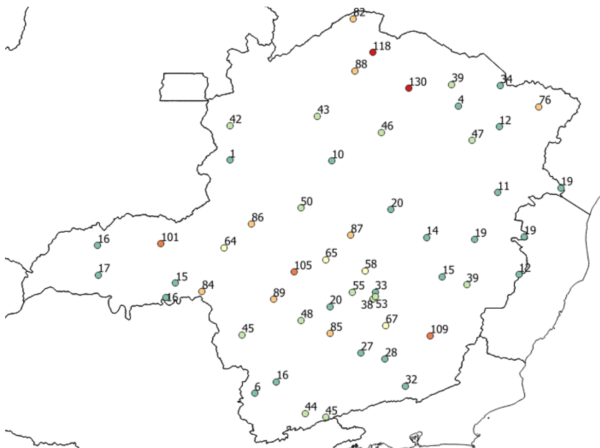
Figura 5b - Pluviometria acumulada entre os dias 27 e 30 de novembro de 2021.
