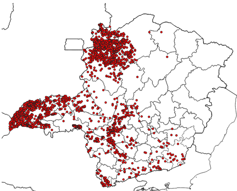
Figura 3 - Localização dos raios registrados entre os dias 27 e 30 de novembro de 2021. Fonte: RINDAT
