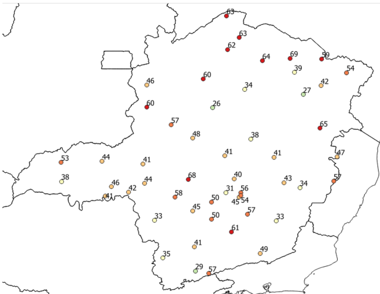
Figura 4 – Rajadas de vento máximas registradas entre os dias 27 e 30 de novembro de 2021. Fonte: INMET
