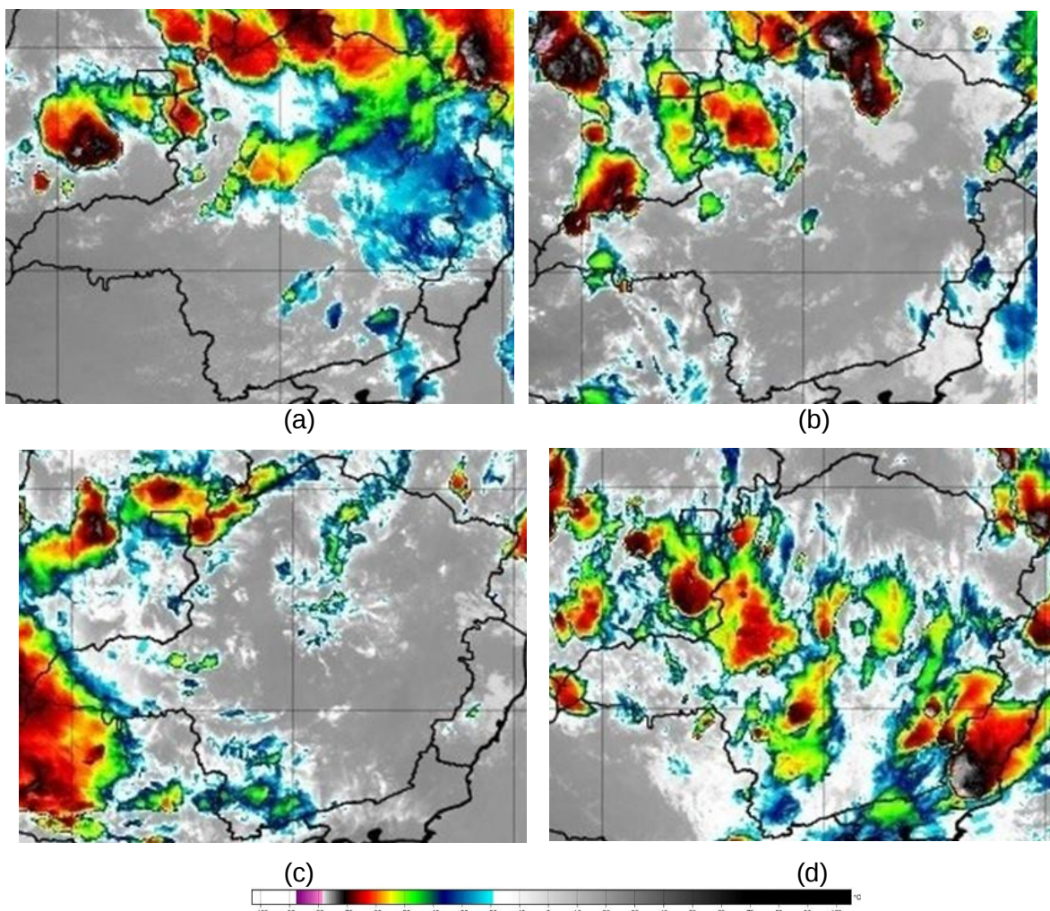
Figura 2 – Seleção de Imagem de Satélite dos dias 27 as 18:00 (a), 28 as 18:00 (b), 29 as 18:00 (c) e 30 as 18:00 de novembro de 2021 (Horário Local). Fonte: INPE.
