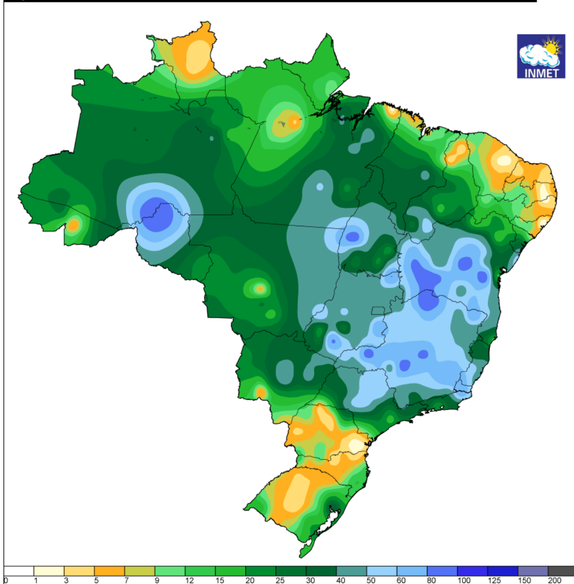
Figura 5a - Pluviometria acumulada entre os dias 26 e 30 de novembro de 2021.
