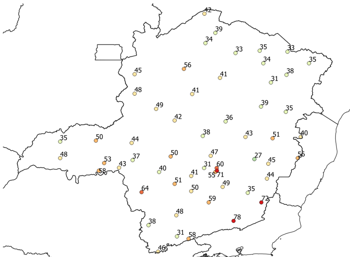
Figura 4 – Rajadas de vento máximas registradas entre os dias 27/12/2021 e 01/01/2022. Fonte: INMET
