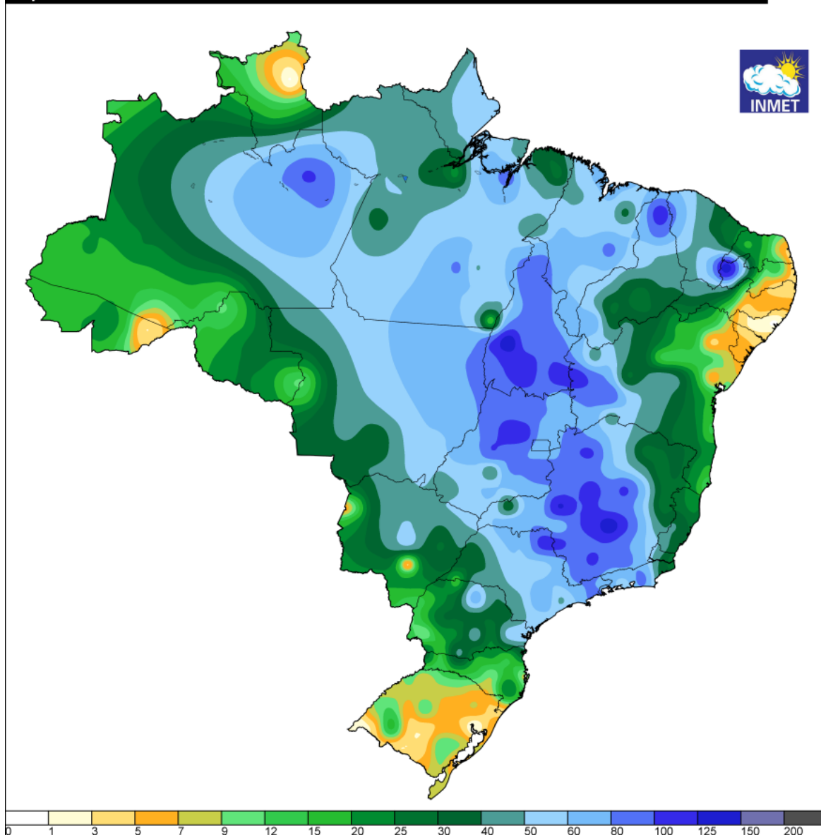
Figura 5a - Pluviometria acumulada entre os dias 28/12/2021 e 01/01/2022. Fonte: INMET.
