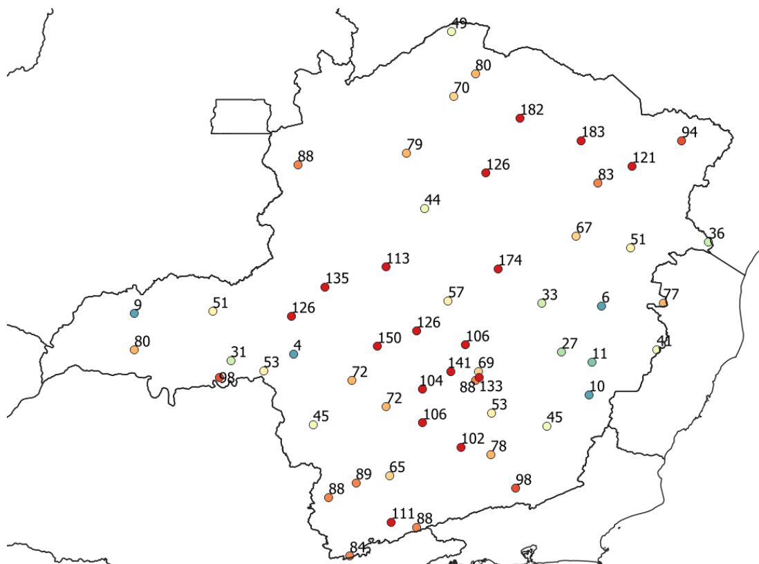
Figura 5b - Pluviometria acumulada entre os dias 27/12/2021 e 01/01/2022. Fonte dos dados: INMET.
