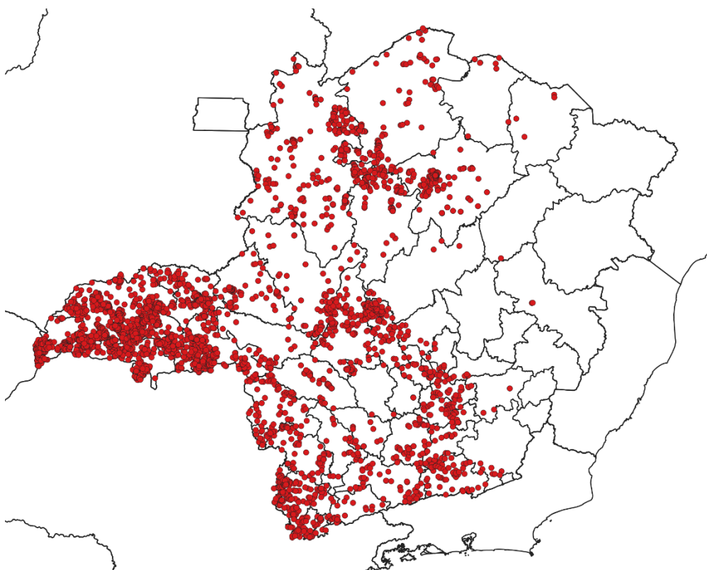
Figura 3 - Localização dos raios registrados entre os dias 27/12/2021 e 01/01/2022. Fonte: RINDAT
