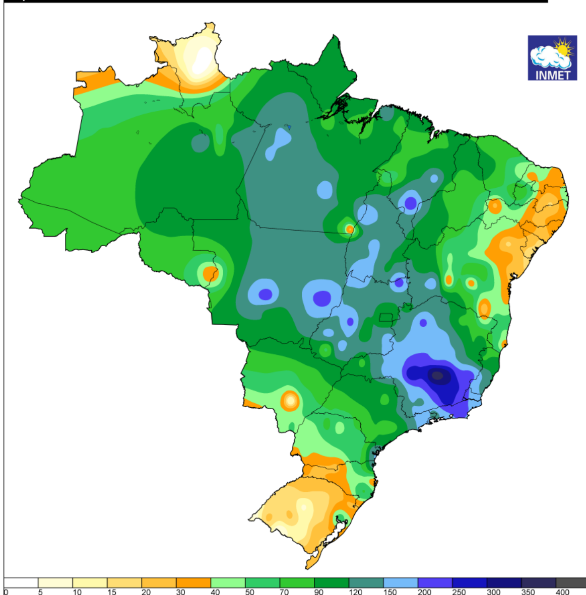
Figura 5a - Pluviometria acumulada entre os dias 03 a 13 de janeiro de 2022. Fonte: INMET.
