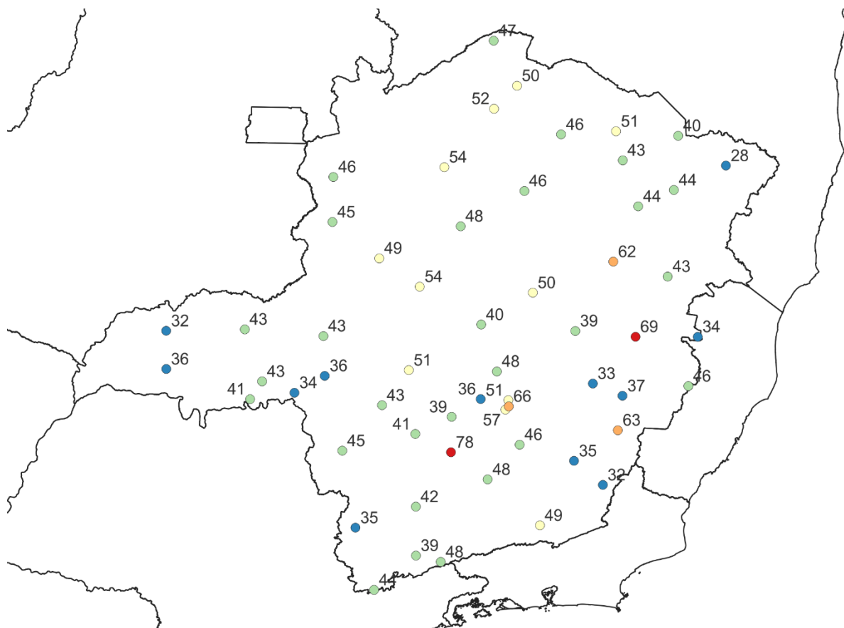
Figura 4 – Rajadas de vento máximas registradas entre os dias 06 e 13 de janeiro de 2022. Fonte: INMET
