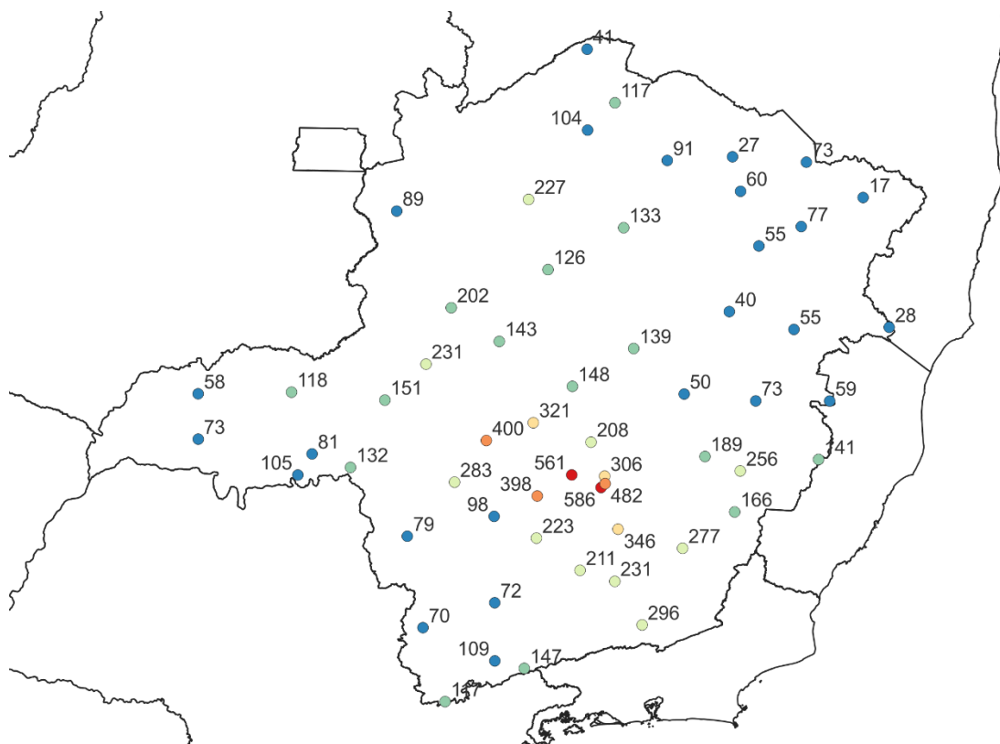
Figura 5b - Pluviometria acumulada entre os dias 06 e 13 de janeiro de 2022. Fonte dos dados: INMET.
