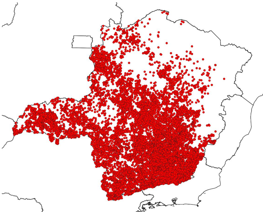
Figura 3 - Localização dos raios registrados entre os dias 06 e 13 de janeiro de 2022. Fonte: RINDAT
