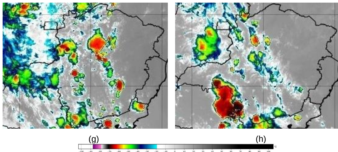
Figura 2 – Seleção de Imagem de Satélite dos dias 06 as 19:00 (a), 07 as 16:00 (b), 08 as 20:00 (c), 09 as 17:00 (d), 10 as 20:00 (e), dia 11 às 17:00 (f), dia 12 às 17:00 (g) e dia 13 às 19:00 (h) horas local, de janeiro de 2022. Fonte: INPE.
