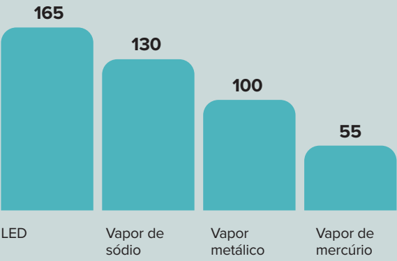
Figura 1 - Imagem ilustrativa da comparação entre a eficiência luminosa média de acordo com os tipos de lâmpadas utilizadas na iluminação pública.
