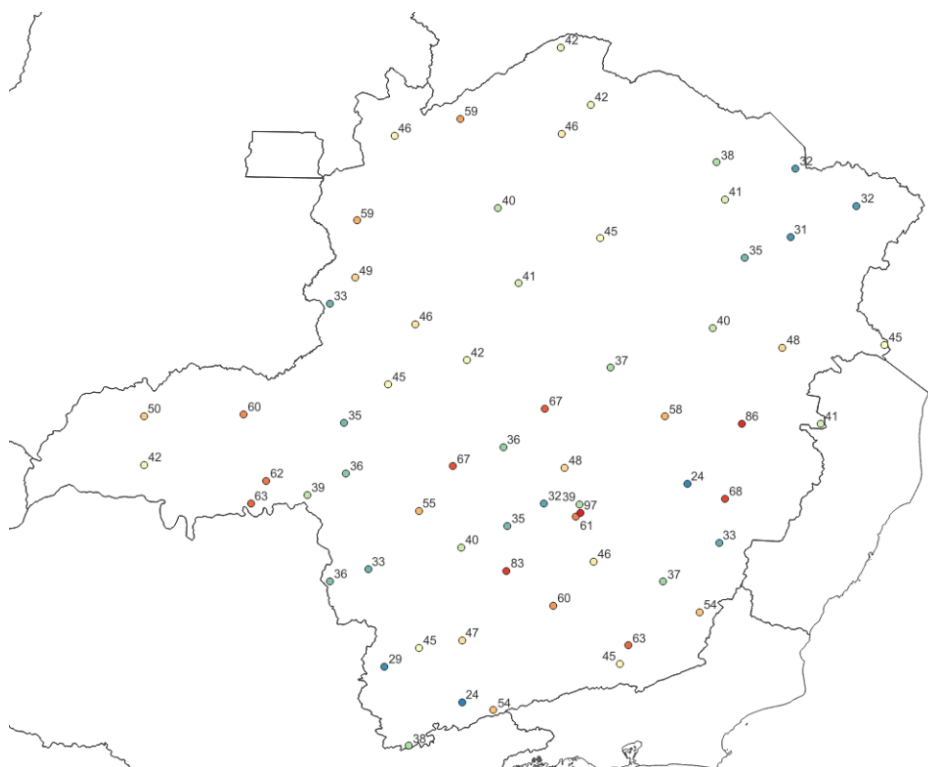
Figura 4 – Rajadas de vento (Km/h) máximas registradas entre os dias 29 e 31 de dezembro de 2023. Fonte: INMET
