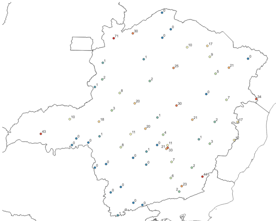
Figura 5b - Pluviometria acumulada entre os dias 29 e 31 de dezembro de 2023. Fonte dos dados: INMET.
