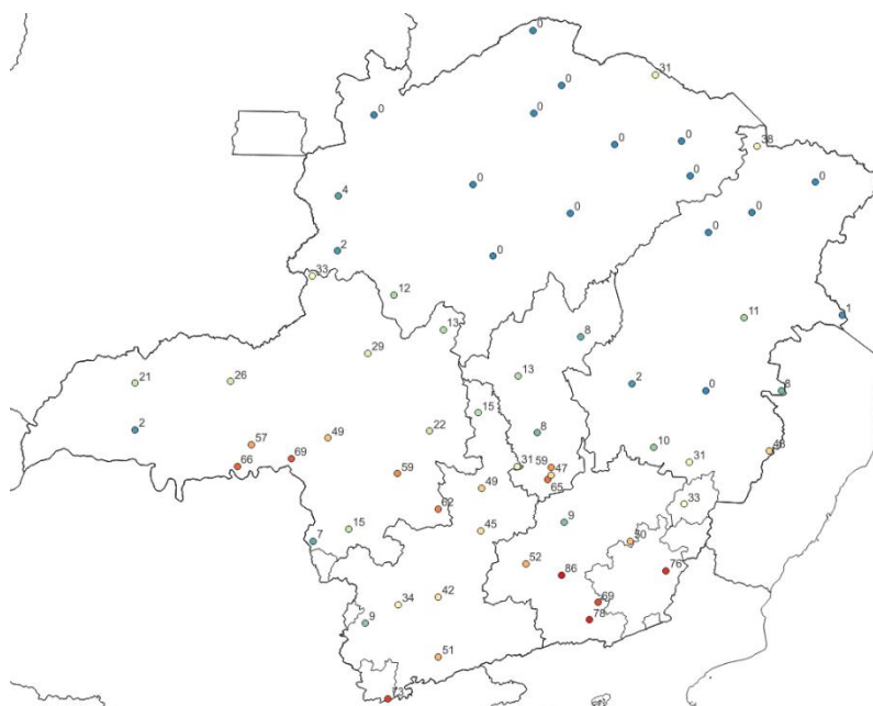
Figura 5b - Pluviometria acumulada entre os dias 17 e 20 de março de 2025. Fonte dos dados: INMET.
