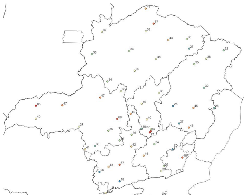
Figura 4 – Rajadas de vento (Km/h) máximas registradas entre os dias 17 e 20 de março de 2025. Fonte: INMET
