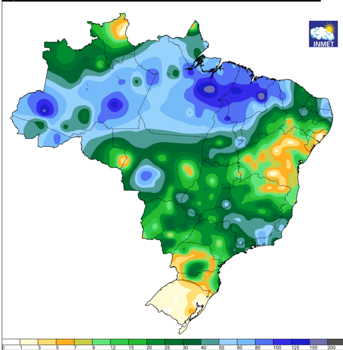
Figura 5a - Pluviometria acumulada (mm) entre os dias 16 e 20 de março de 2025. Fonte: INMET.
