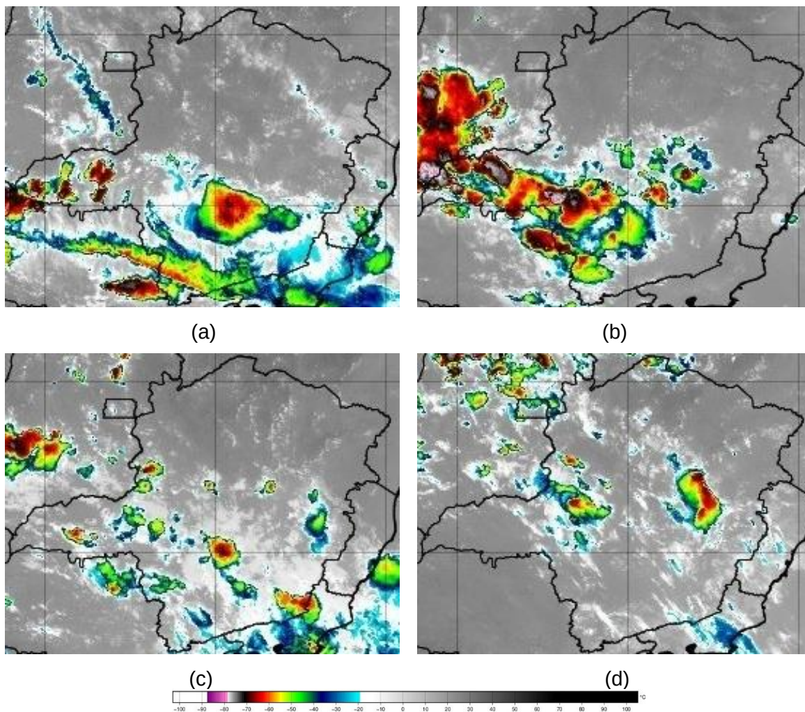
Figura 2 – Seleção de Imagens de Satélite dos dias 17 (a), 18 (b), 19 (c) e 20 (d) de março de 2025. Fonte: INPE.
