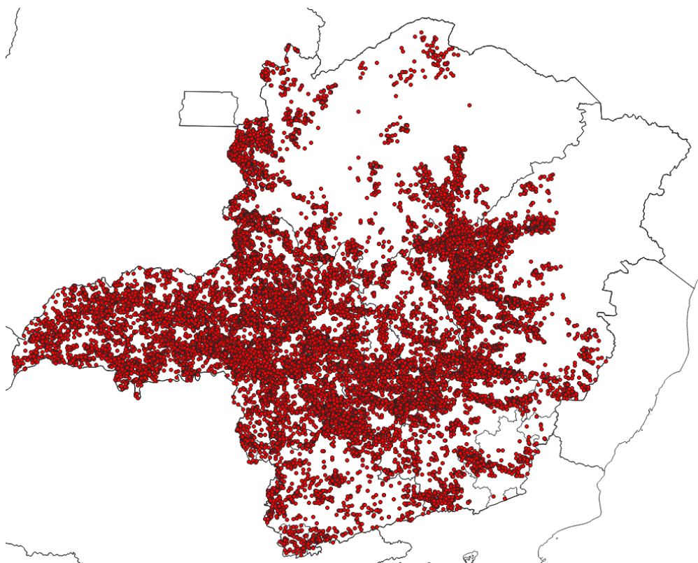
Figura 3 - Localização dos raios registrados entre os dias 17 e 20 de março de 2025. Fonte: RINDAT
