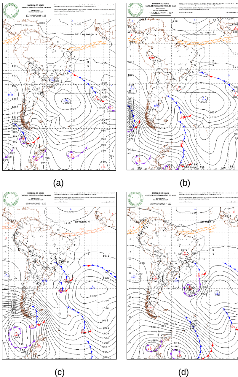
Figura 1 - Carta Sinótica em superfície dos dias 17 (a), 18 (b), 19 (c) e 20 (d) de março de 2025. Fonte: Marinha do Brasil.
