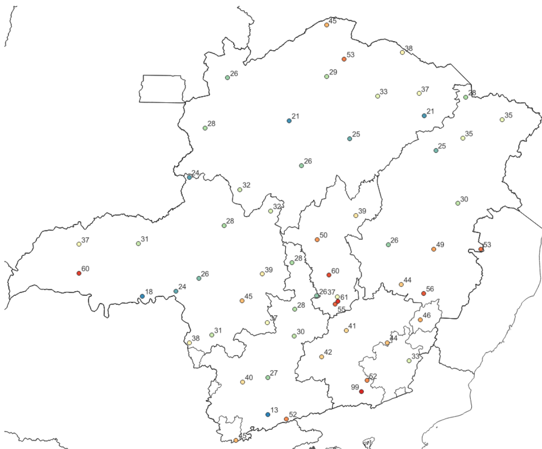
Figura 4 – Rajadas de vento (Km/h) máximas registradas entre os dias 10 e 11 de abril de 2025. Fonte: INMET
