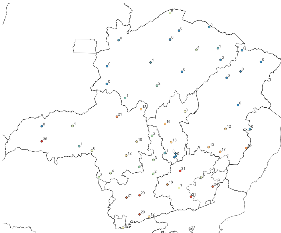
Figura 5b - Pluviometria acumulada entre os dias 10 e 11 de abril de 2025. Fonte dos dados: INMET.
