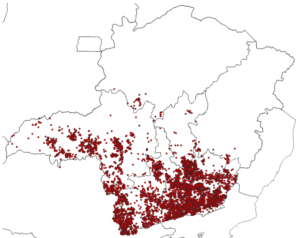
Figura 3 - Localização dos raios registrados entre os dias 10 e 11 de abril de 2025. Fonte: RINDAT
