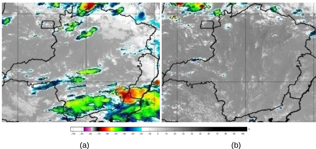
Figura 2 – Seleção de Imagem de Satélite dos dias 10 (a) e 11 (b) de abril de 2025. Fonte: INPE.
