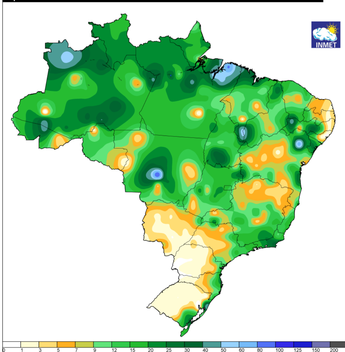
Figura 5a - Pluviometria acumulada (mm) entre os dias 09 e 11 de abril de 2025. Fonte: INMET.
